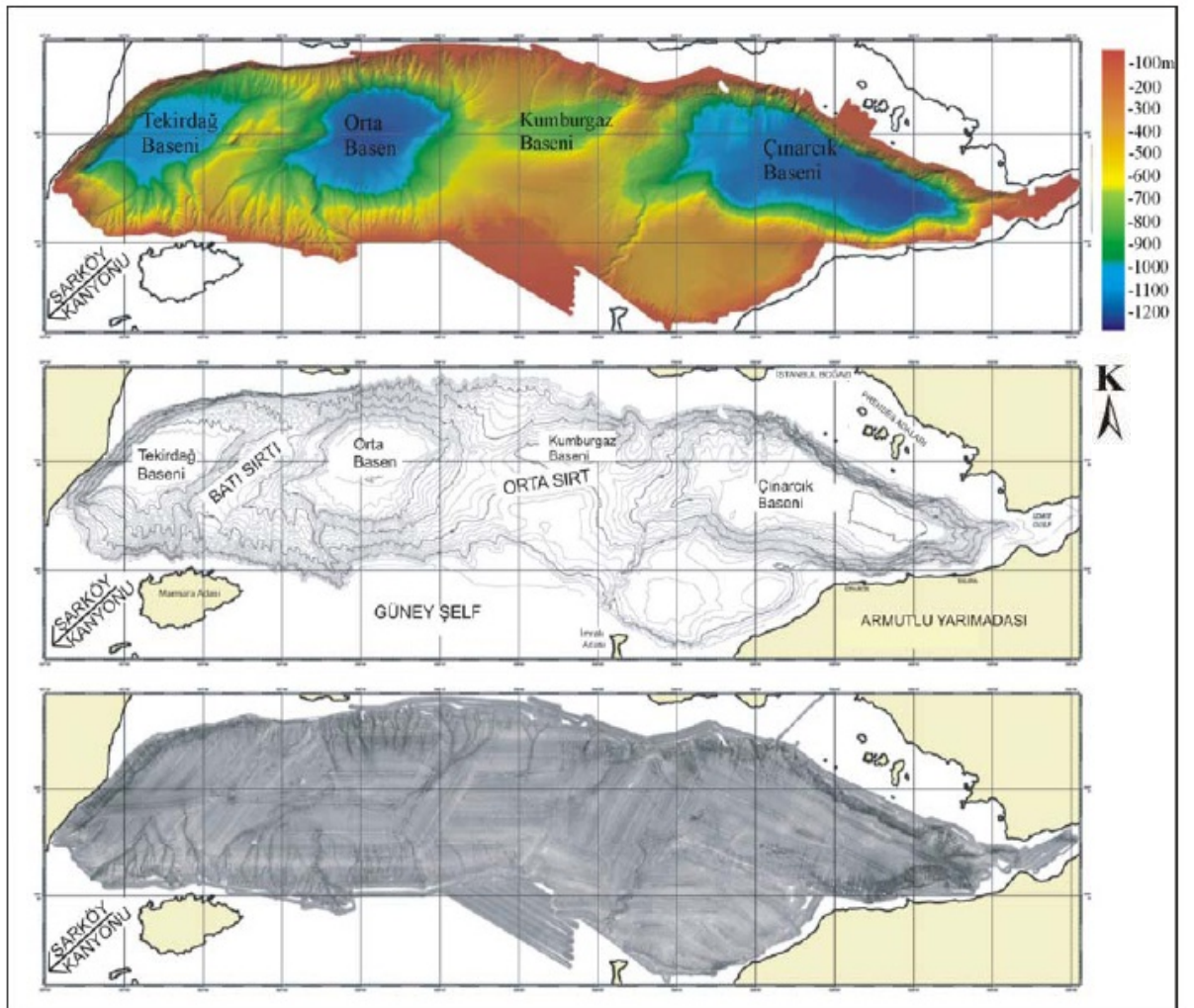
Şekil 1.2 Marmara Denizi'nin önemi morfolojik yapıları (Le Pichon vd. 2001)
