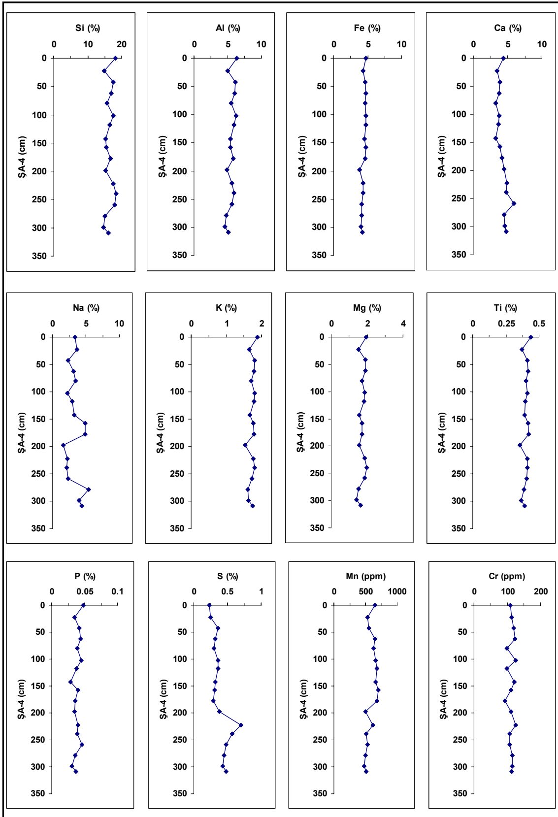
Şekil 4.1 ŞA-4 karotu derinliğe göre element dağılımı
