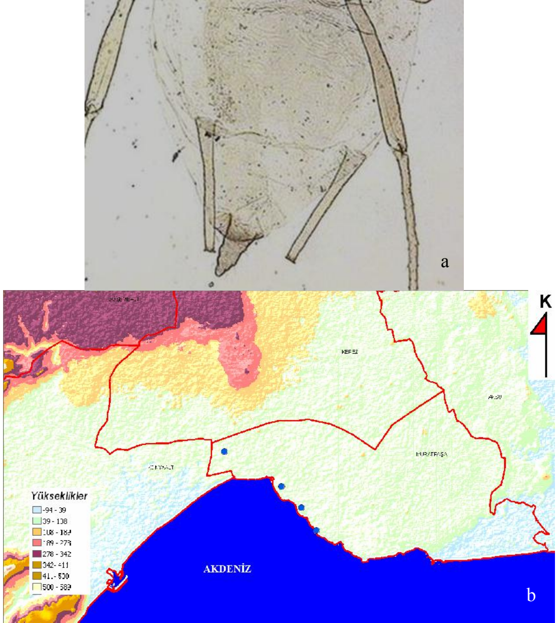
Şekil 4.24 Aulacorthum solani (Kaltenbach)’nin: a. kanatsız bireyinde abdomen, b. Antalya şehrinde yüksekliğe göre dağılımı
