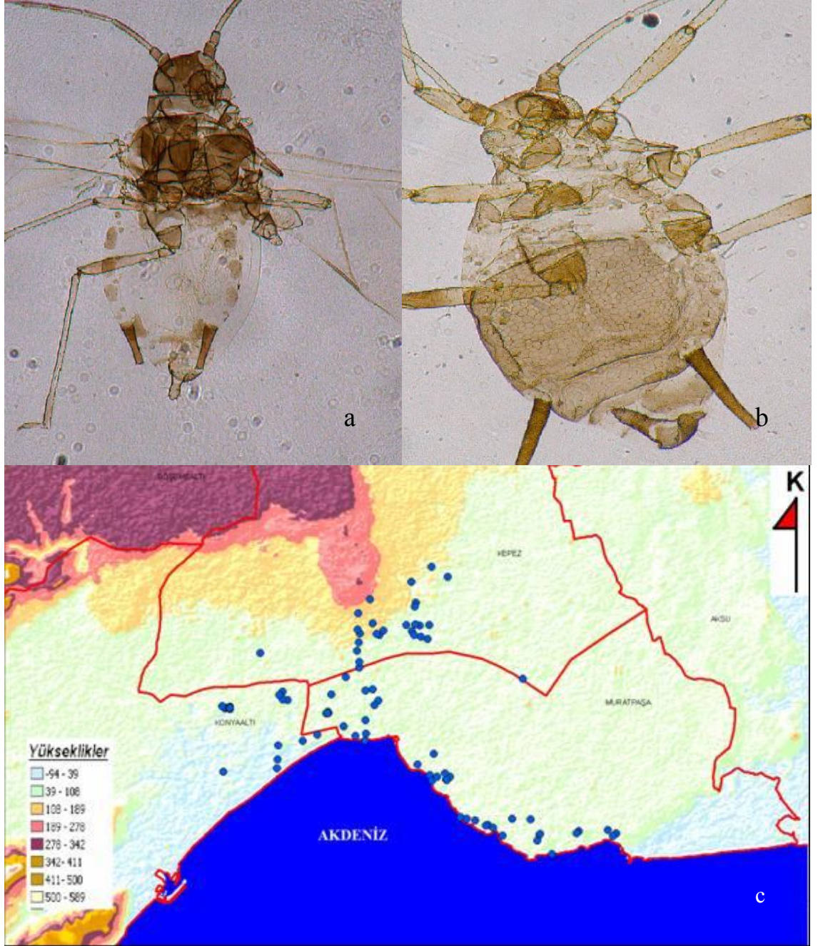
Şekil 4.4. Aphis craccivora Koch'nın: a. kanatlı bireyi, b. kanatsız bireyi, c. Antalya şehrinde yüksekliğe göre dağılımı
