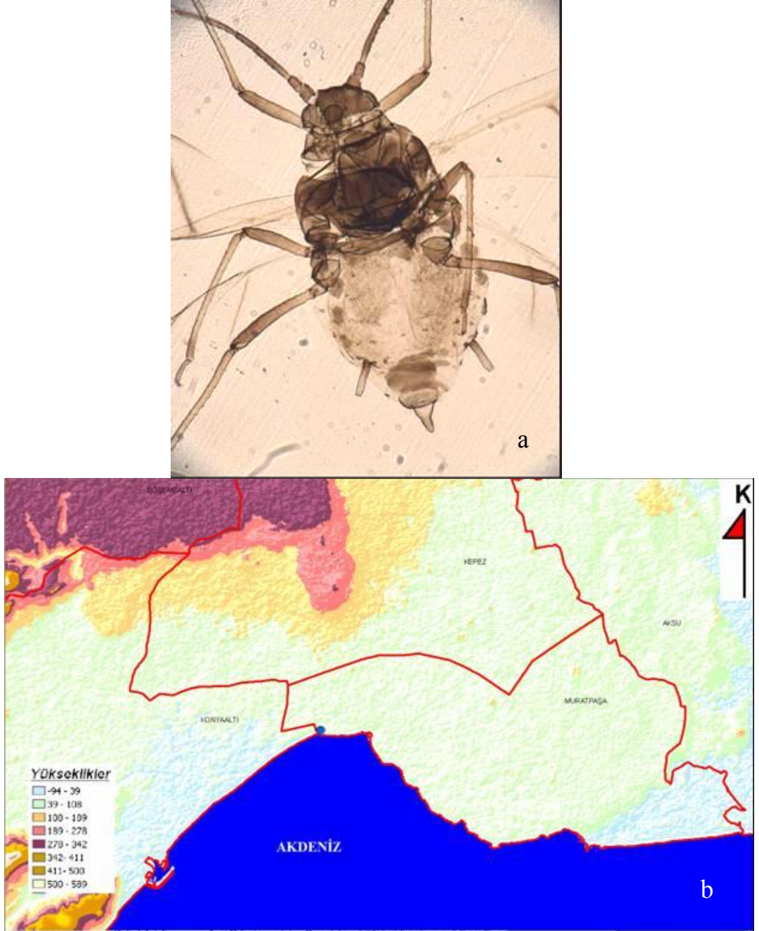
Şekil 4.37 Lipaphis erysimi (Kaltenbach)’nin: a. kanatlı bireyi, b. Antalya şehrinde yüksekliğe göre dağılımı
