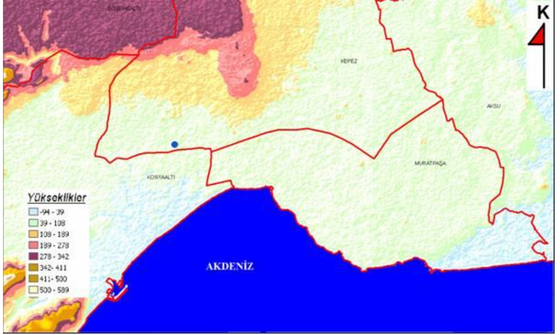
Şekil 4.30 Capitophorus inulae (Passerini)'nın Antalya şehrinde yüksekliğe göre dağılımı
