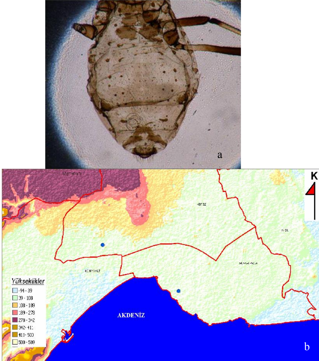
Şekil 4.54 Cinara pinea (Mordvilko)'nın: a. kanatsız bireyinde abdomen, b. Antalya şehrinde yüksekliğe göre dağılımı
