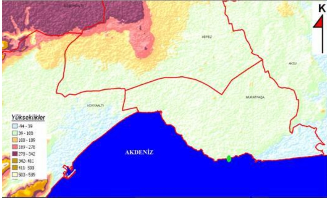
Şekil 4.59 Pemphigus immunis Buckton’ın Antalya şehrinde yüksekliğe göre dağılımı
