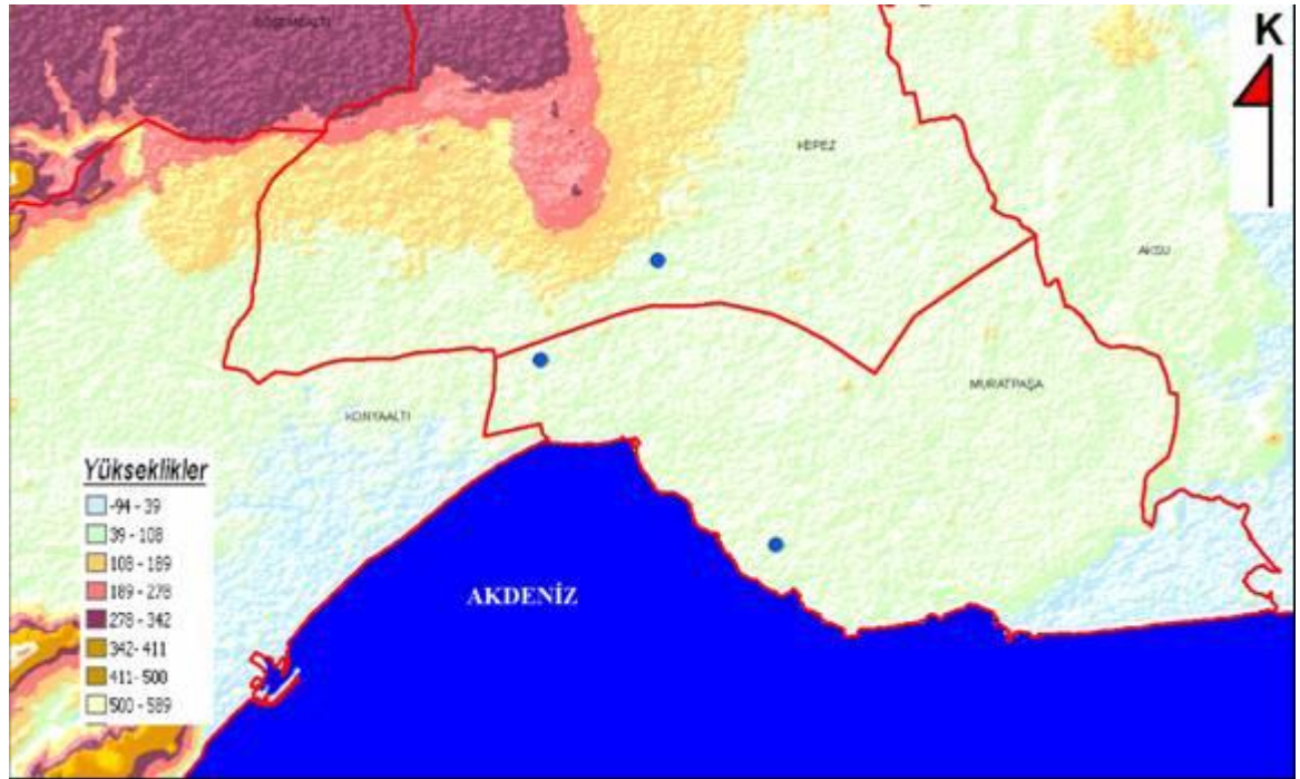
Şekil 4.22 Rhapalosiphum nymphaeae (Linnaeus) ’nin Antalya şehrinde yüksekliğe göre dağılımı
