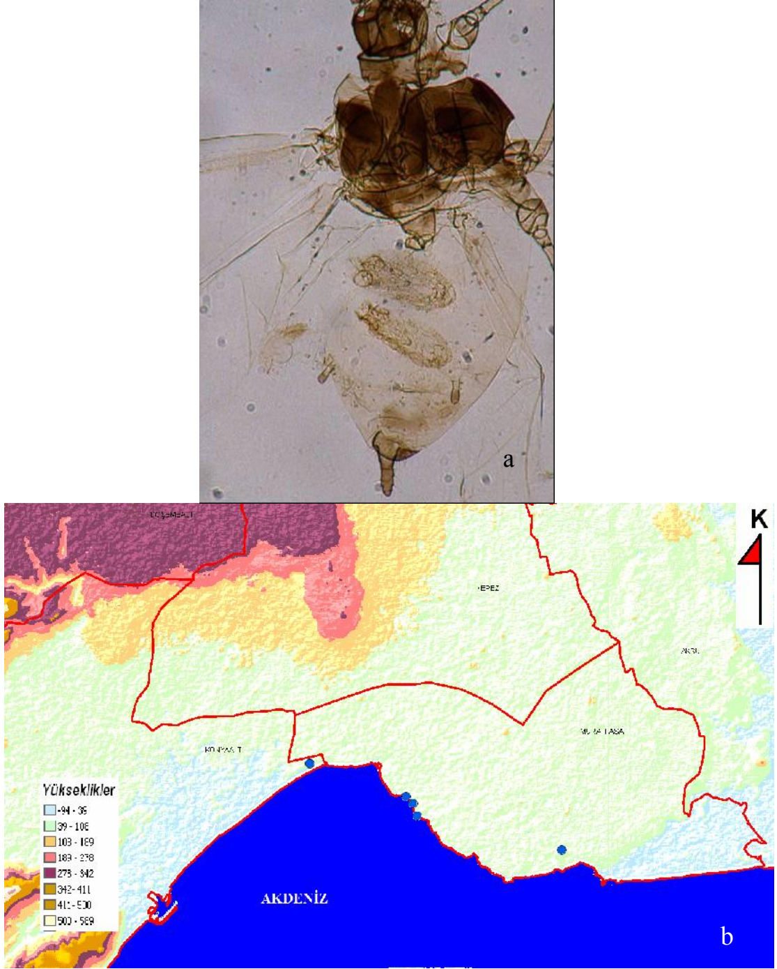
Şekil 4.21 Melanaphis sacchari (Zehntner)'nin: a. kanatlı bireyi, b. Antalya şehrinde yüksekliğe göre dağılımı
