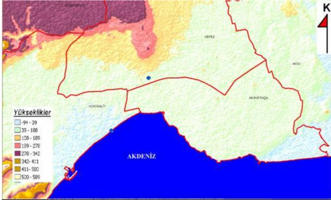
Şekil 4.42 Myzus ornatus Laing'un Antalya şehrinde yüksekliğe göre dağılımı
