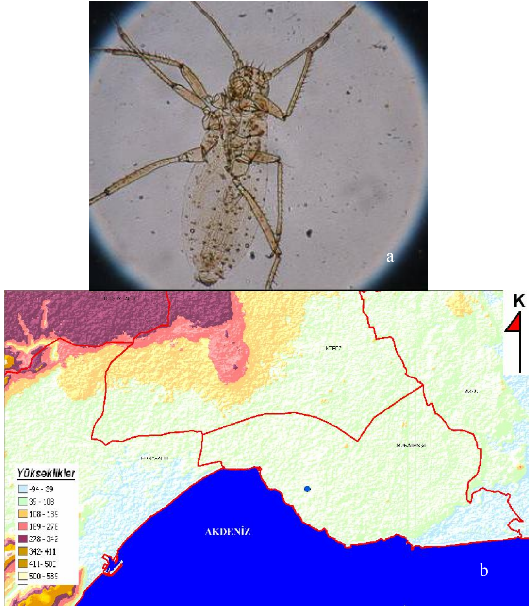
Şekil 4.56 Eulachnus rileyi (Williams)'nin: a. kanatsız bireyi, b. Antalya şehrinde yüksekliğe göre dağılımı
