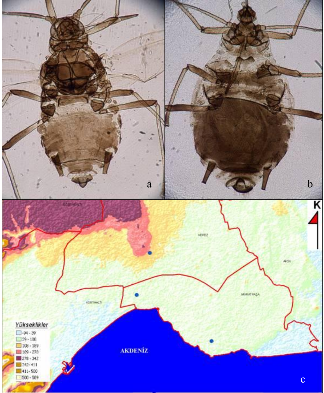
Şekil 4.26 Brachycaudus (Acaudus) cardui (Linnaeus)'nin: a. kanatlı bireyi, b. kanatsız bireyi, c. Antalya şehrinde yüksekliğe göre dağılımı
