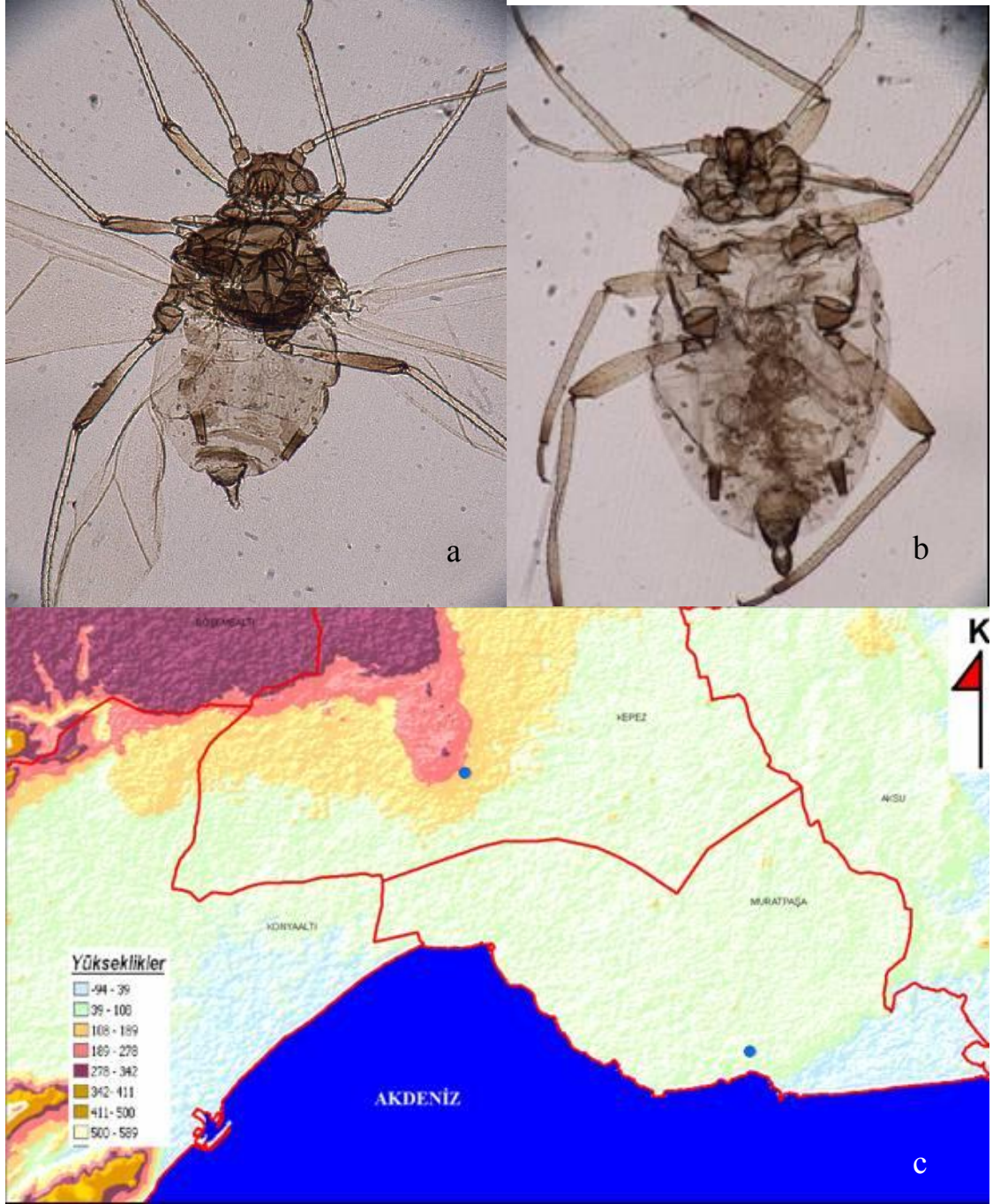
Şekil 4.15 Aphis tirucallis Hille Ris Lambers'in: a. kanatlı bireyi, b. kanatsız bireyi, c. Antalya şehrinde yüksekliğe göre dağılımı
