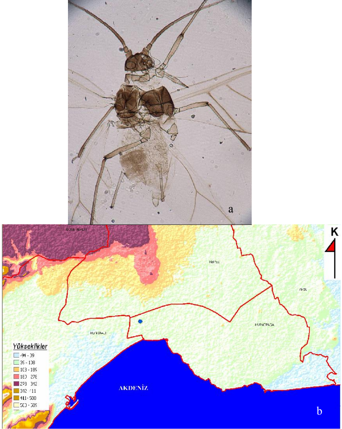
Şekil 4.29 Capitophorus elaeagni (del Guercio)'nin: a. kanatlı bireyi, b. Antalya şehrinde yüksekliğe göre dağılımı
