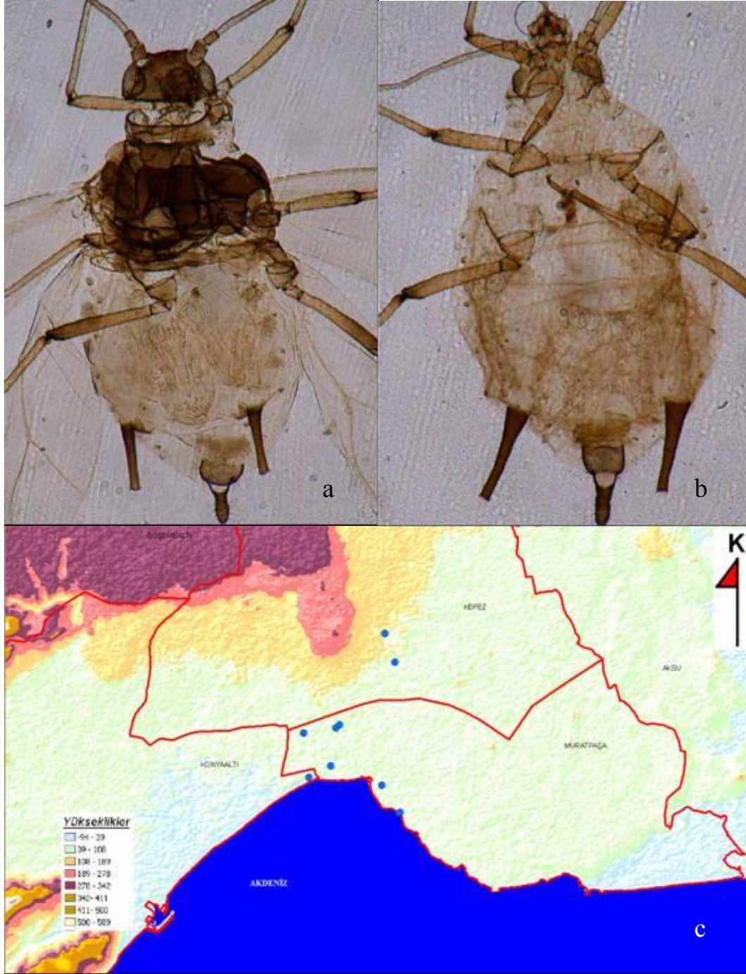
Şekil 4.11 Aphis pomi de Geer'in: a. kanatlı bireyi, b. kanatsız bireyi, c. Antalya şehrinde yüksekliğe göre dağılımı
