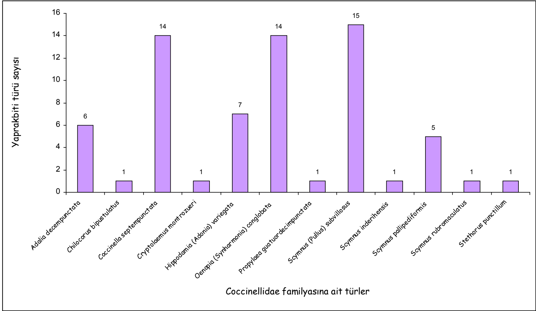
Şekil 4.60 Coccinellidae familyasına ait türlerin beslendiği yaprakbiti türlerinin sayısı
