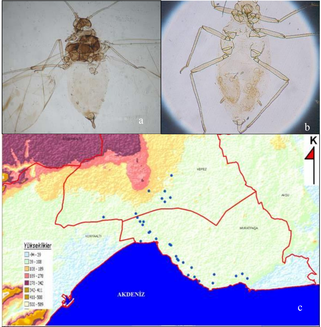
Şekil 4.20 Hyalopterus pruni (Geoffroy)'nin: a. kanatlı bireyi, b. kanatsız bireyi, c. Antalya şehrinde yüksekliğe göre dağılımı
