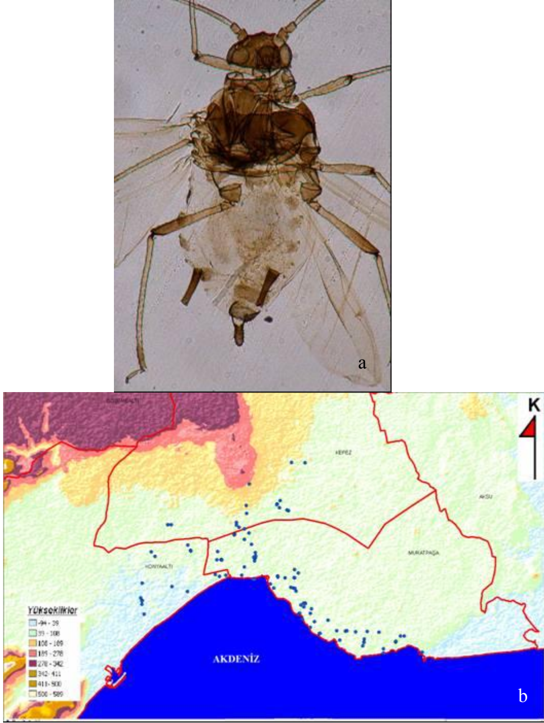
Şekil 4.14 Aphis spiraecola Patch'ın: a. kanatlı bireyi, b. Antalya şehrinde yüksekliğe göre dağılımı
