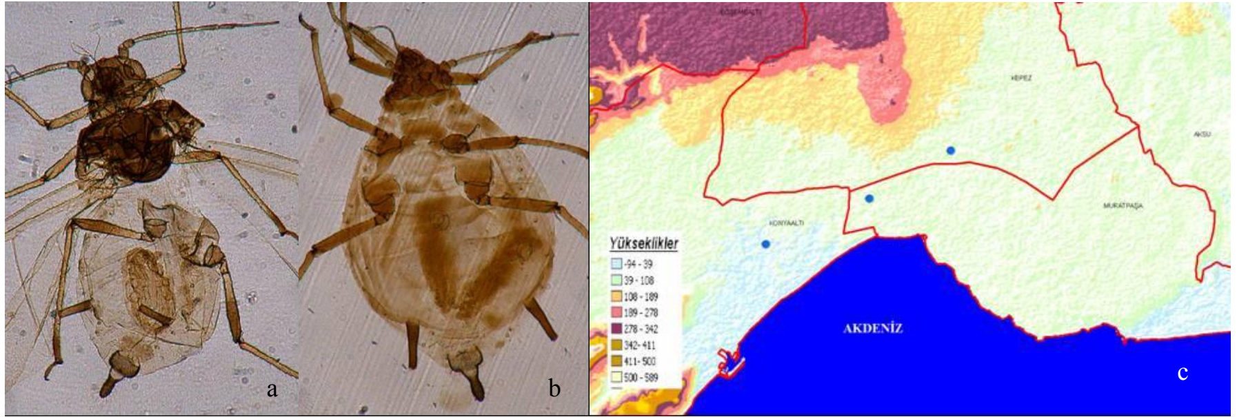
Şekil 4.9 Aphis hederae Kalténbach'ın: a. kanatlı bireyi, b. kanatsız bireyi, c. Antalya şehrinde yüksekliğe göre dağılımı.
