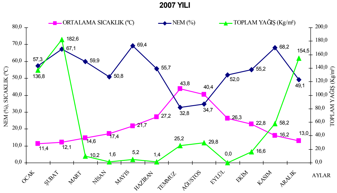
EK 4 Antalya şehrine ait 2007, 2008 ve 2009 yıllarına ait ortalama sıcaklık, nem (%) ve toplam yağış miktarlarını gösteren grafikler
