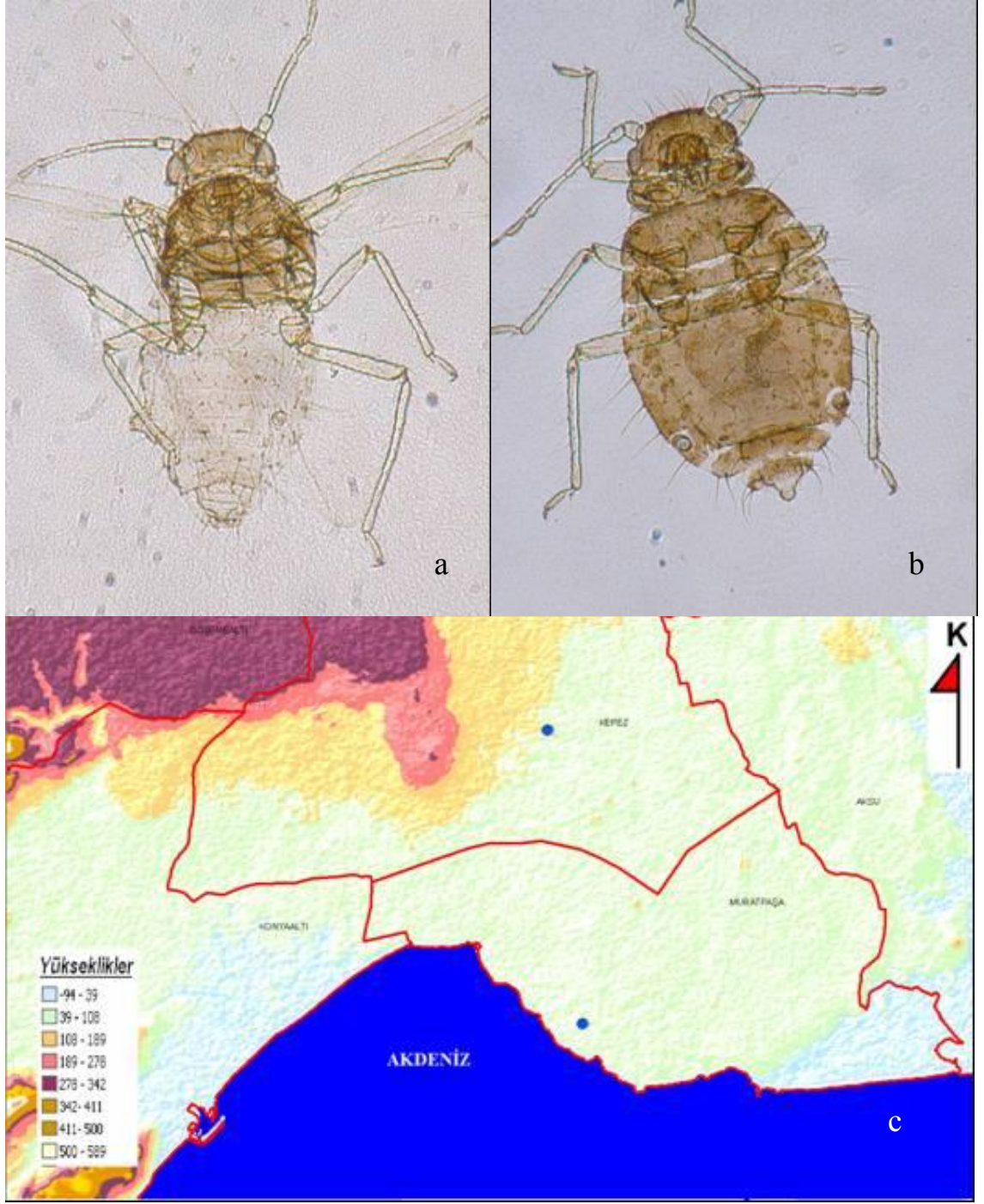
Şekil 4.52 Chaitophorus populeti (Panzer)'nin: a. kanatlı bireyi, b. kanatsız bireyi, c. Antalya şehrinde yüksekliğe göre dağılımı
