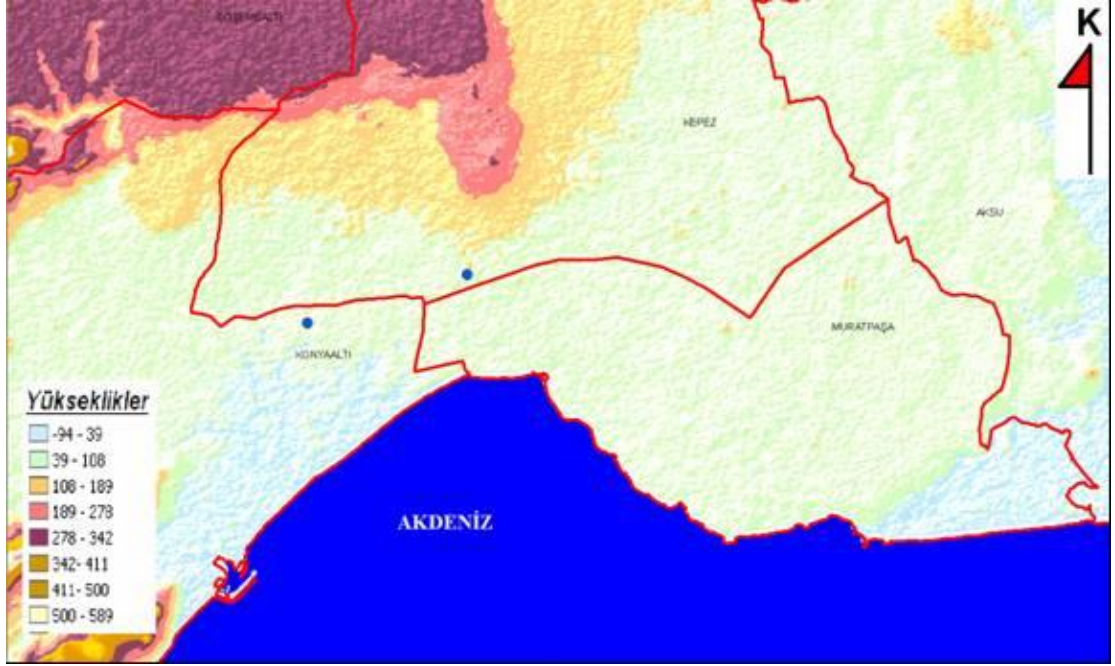
Şekil 4.6. Aphis fabae subsp. cirsiacanthoidis Scopoli 'in Antalya şehrinde yüksekliğe göre dağılımı
