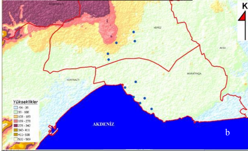
Şekil 4.16 Aphis umbrella (Börner)'nın: a. kanatsız bireyi, b. Antalya şehrinde yüksekliğe göre dağılımı
