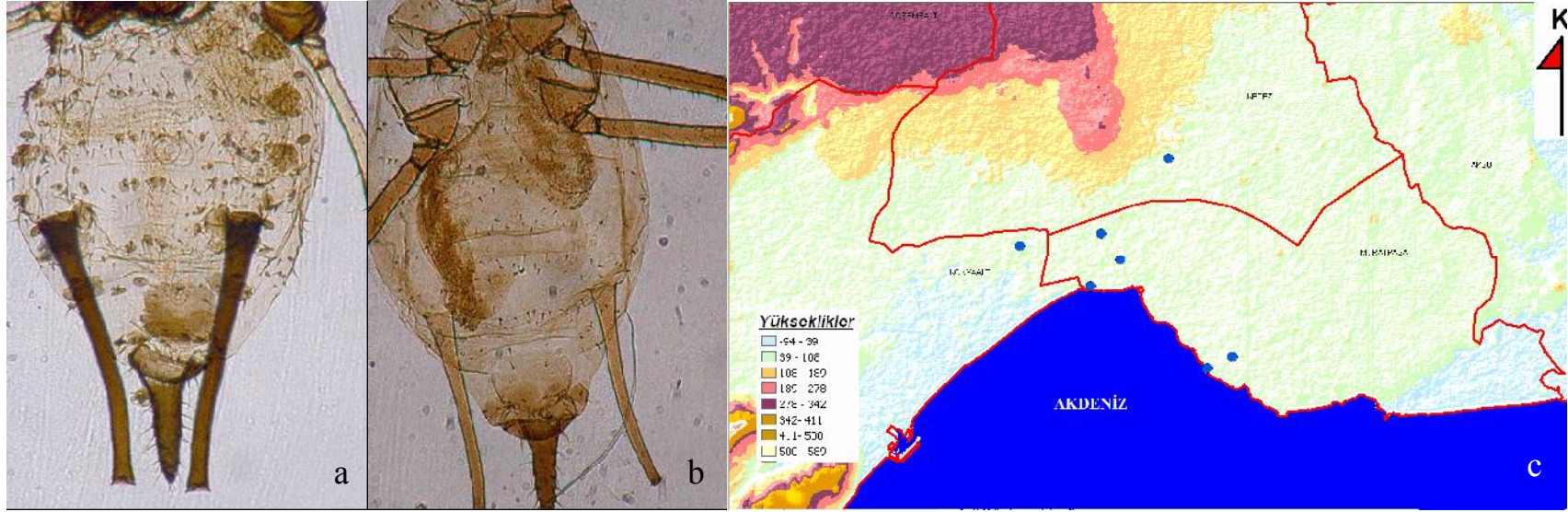
Şekil 4.39 Macrosiphum euphorbiae (Thomas)'nın: a. kanatlı bireyinde abdomen, b. kanatsız bireyinde abdomen, c. Antalya şehrinde yüksekliğe göre dağılımı
