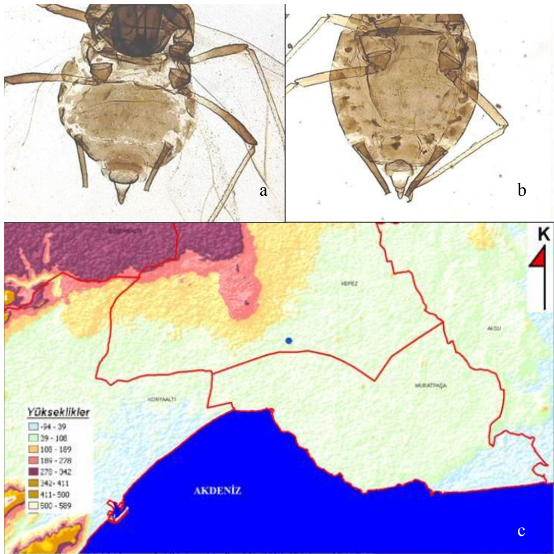
řekil 4.41 Myzus cerasi (Fabricius)’nin: a. kanatlı bireyi, b. kanatsız bireyinde abdomen, c. Antalya řehrinde yüksekliđe göre dađılımı
