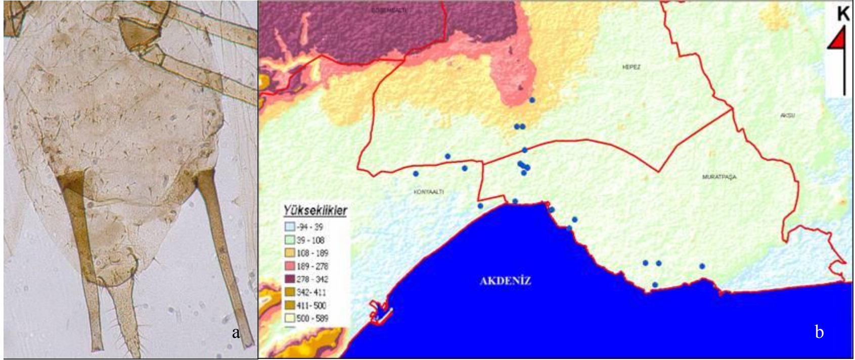
Şekil 4.46 Uroleucon sonchi (Linnaeus)'nin: a. kanatlı bireyinde abdomen, b. Antalya şehrinde yüksekliğe göre dağılımı
