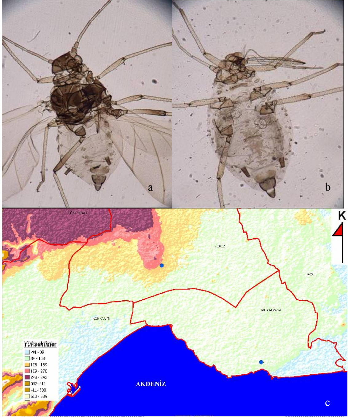
Şekil 4.17 Aphis vallei Hille Ris Lambers & Stroyan'ın: a. kanatlı bireyi, b. kanatsız bireyi, c. Antalya şehrinde yüksekliğe göre dağılımı.
