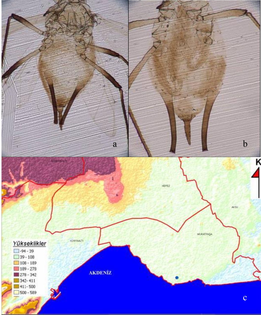
Şekil 4.48 Uroleucon (Lambersius) erigeronense (Thomas)'nin: a. kanatlı bireyi, b. kanatsız bireyi, c. Antalya şehrinde yüksekliğe göre dağılımı
