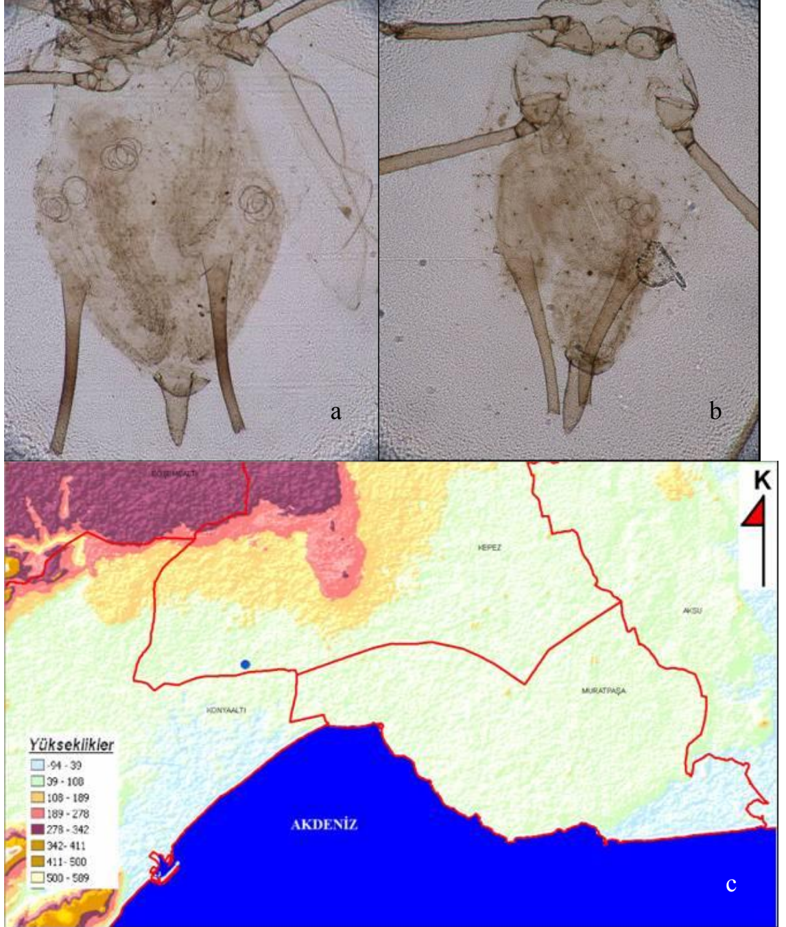
Şekil 4.47 Uroleucon (Belochilum) inulae (Ferrari)’nın: a. kanatlı bireyinde abdomen, b. kanatsız bireyinde abdomen, c. Antalya şehrinde yüksekliğe göre dağılımı
