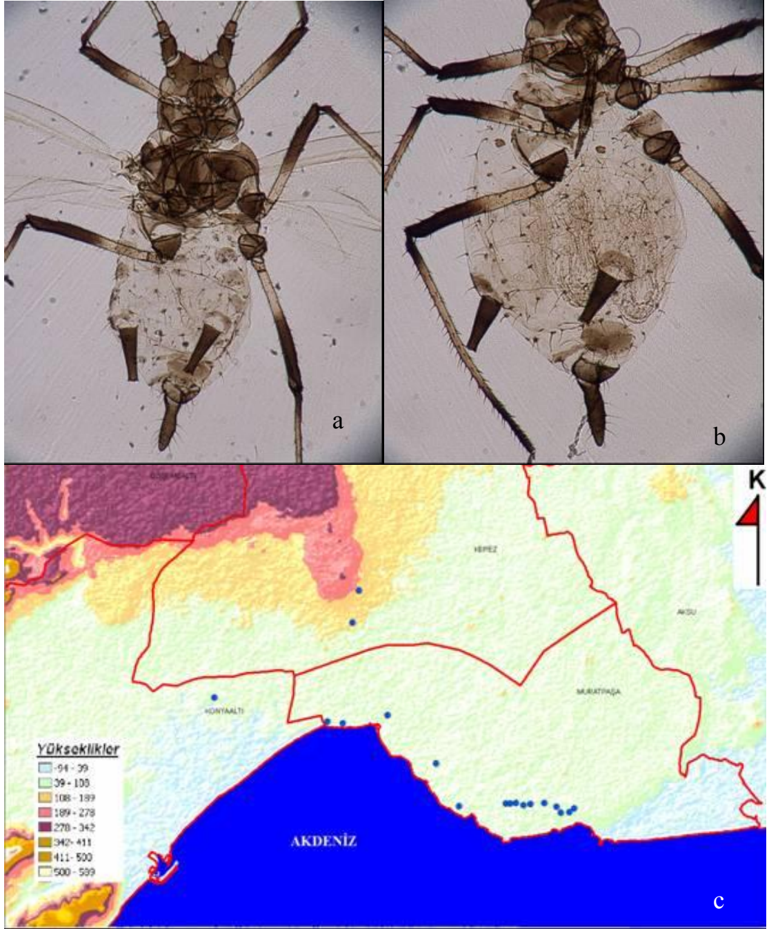
Şekil 4.38 Macrosiphoniella sanborni (Gillette)'nin: a. kanatlı bireyi, b. kanatsız bireyi, c. Antalya şehrinde yüksekliğe göre dağılımı
