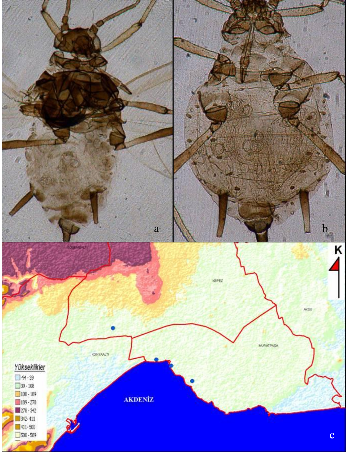
Şekil 4.7 Aphis fabae subsp. solanella Theobald'ın: a. kanatlı bireyi, b. kanatsız bireyi, c. Antalya şehrinde yüksekliğe göre dağılımı
