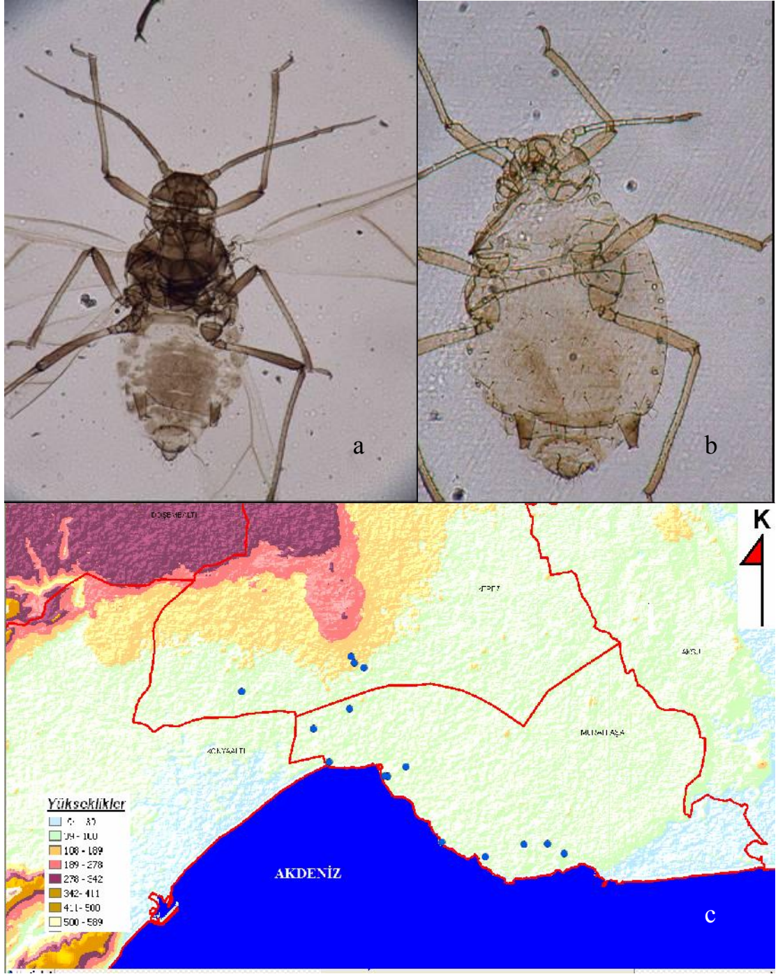
Şekil 4.25 Brachycaudus helichrysi (Kaltenbach)'nin: a. kanatlı bireyi, b. kanatsız bireyi, c. Antalya şehrinde yüksekliğe göre dağılımı
