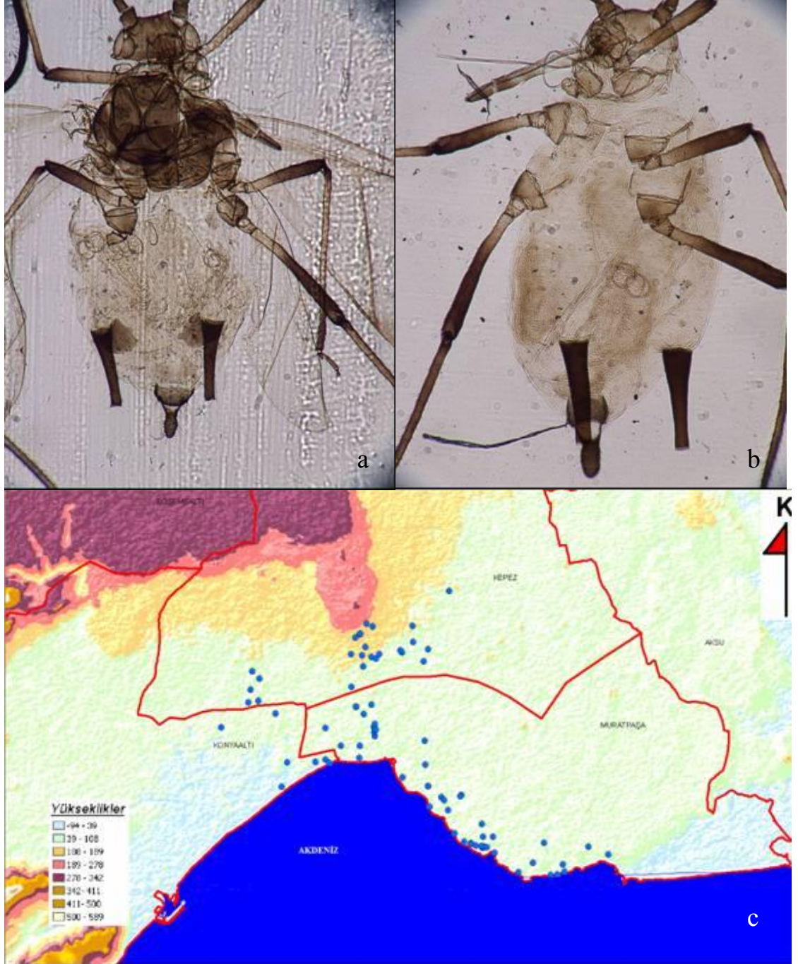
Şekil 4.10 Aphis nerii Boyer de Fonscolombe'nin: a. kanatlı bireyi, b. kanatsız bireyi, c. Antalya şehrinde yüksekliğe göre dağılımı.
