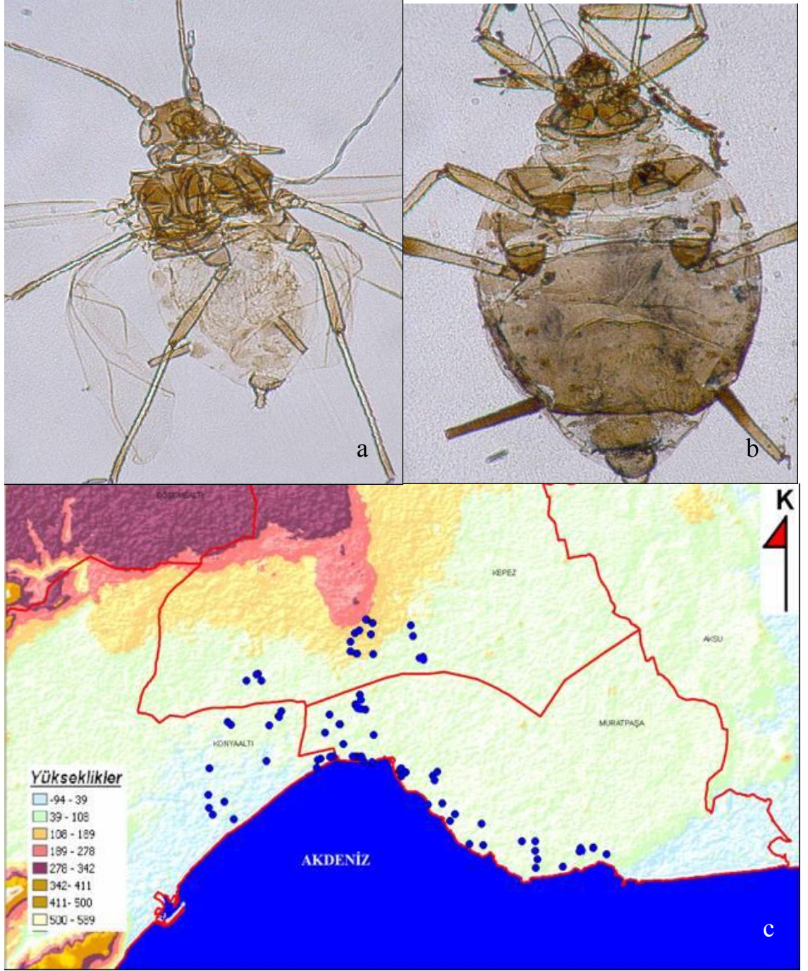
Şekil 4.5 Aphis fabae Scopoli'nin: a. kanatlı bireyi, b. kanatsız bireyi, c. Antalya şehrinde yüksekliğe göre dağılımı
