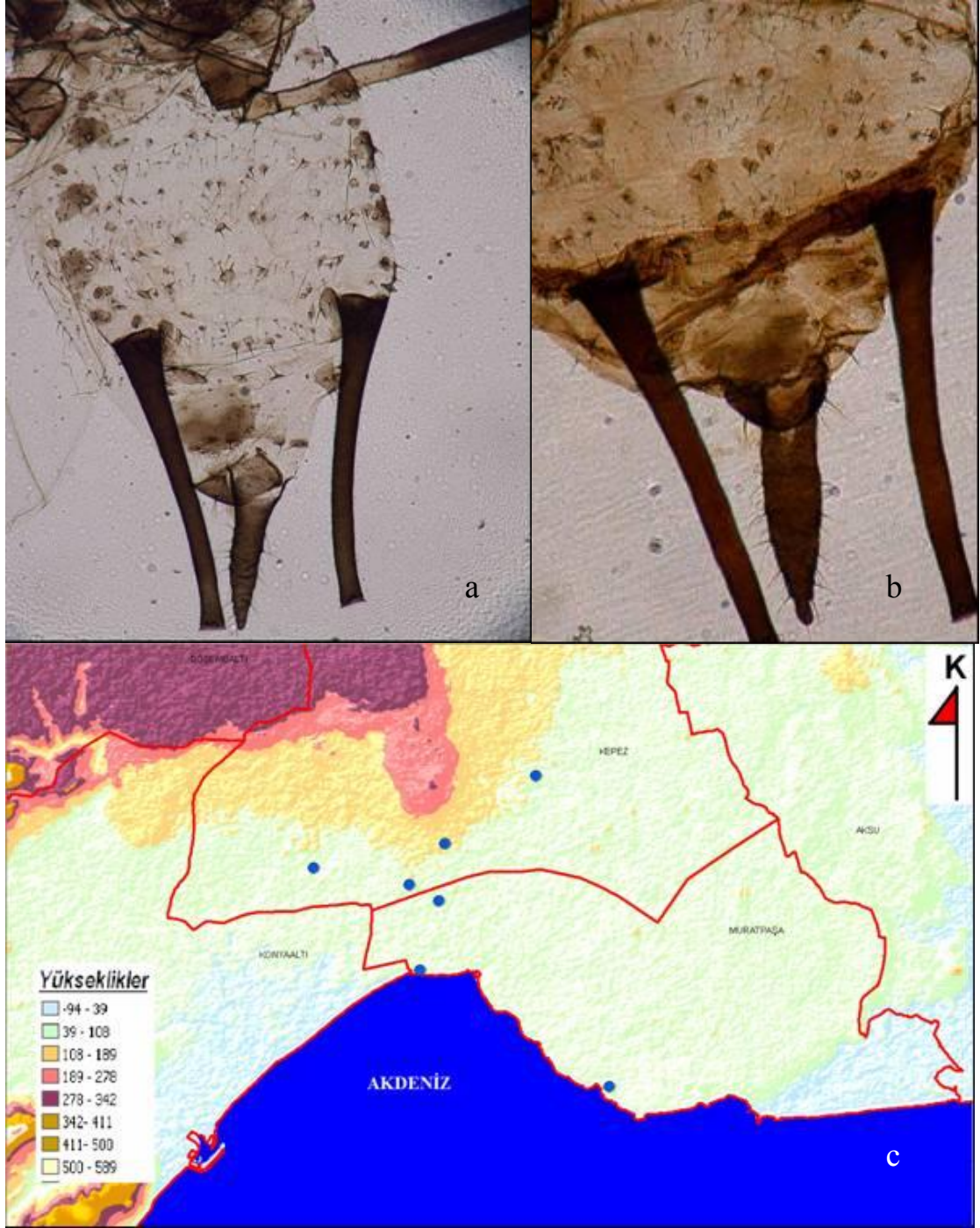
Şekil 4.50 Uroleucon (Uromelan) jaceae (Linnaeus)'nin: a. kanatlı bireyinde abdomen, b. kanatsız bireyinde abdomen, c. Antalya şehrinde yüksekliğe göre dağılımı
