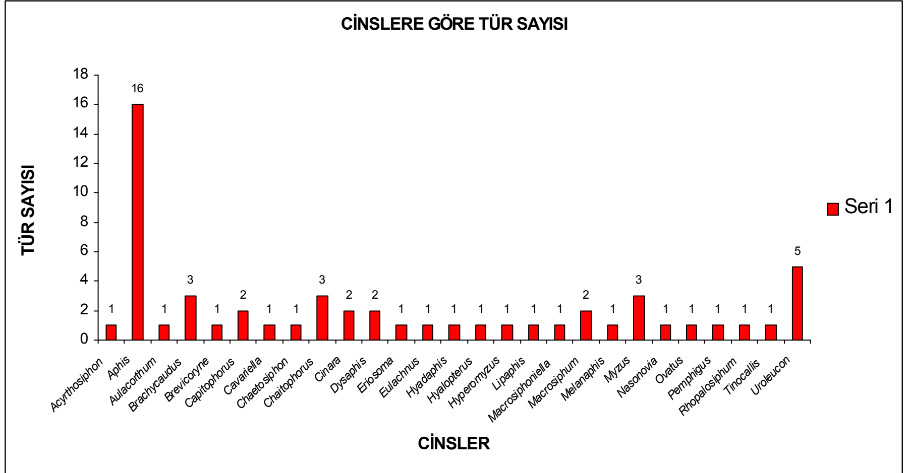
Şekil 4.2. Çalışmada saptanan cinslerde bulunan yaprakbiti tür sayısının dağılımı
