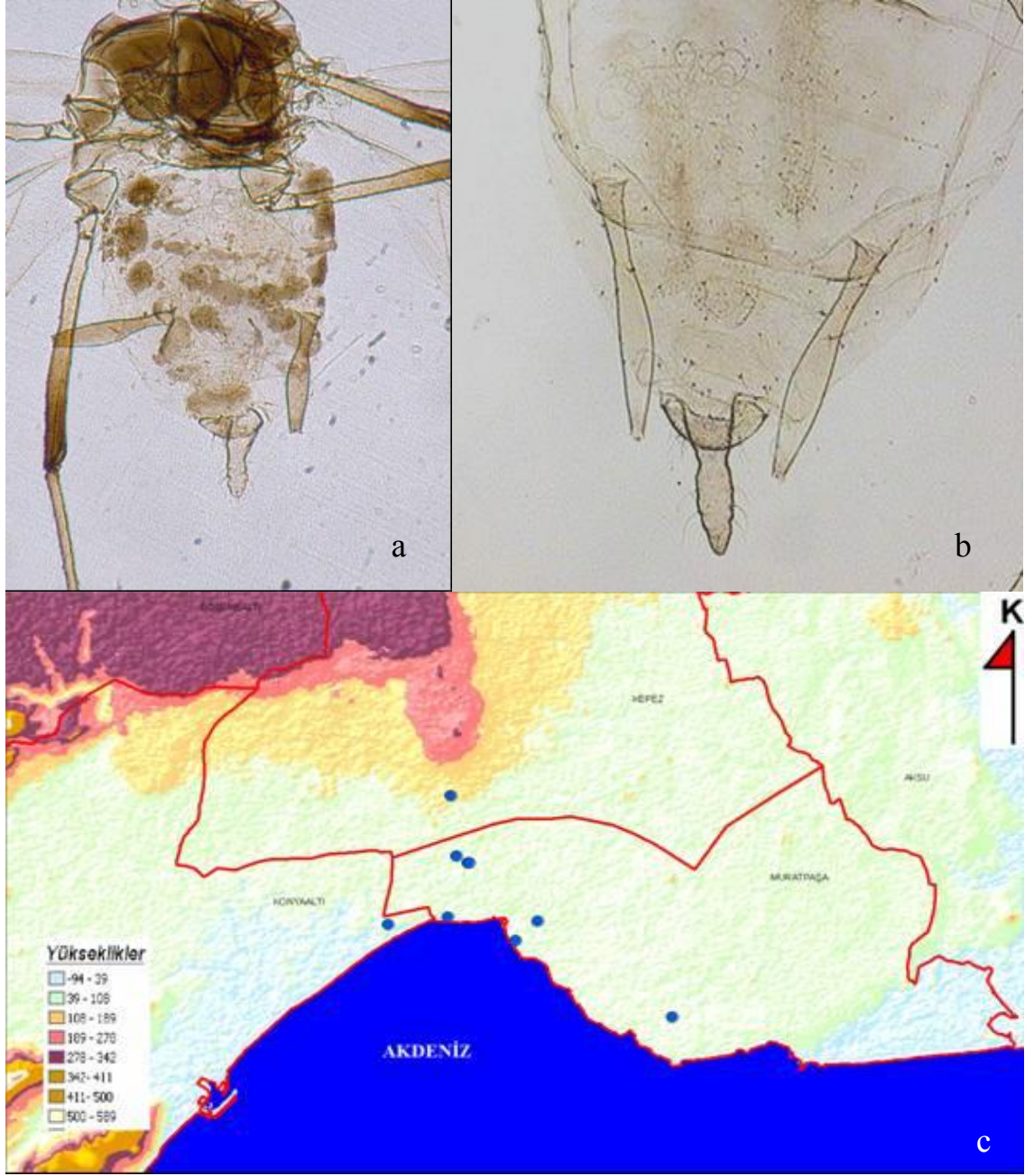
Şekil 4.36 Hyperomyzus lactucae (Linnaeus)'nin: a. kanatlı bireyi, b. kanatsız bireyinde abdomen, c. Antalya şehrinde yüksekliğe göre dağılımı
