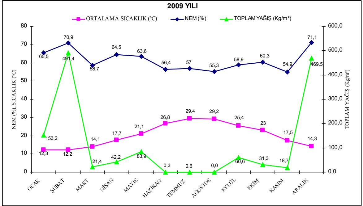
EK 4 Antalya şehrine ait 2007, 2008 ve 2009 yıllarına ait ortalama sıcaklık, nem (%) ve toplam yağış miktarlarını gösteren grafikler (devam)
