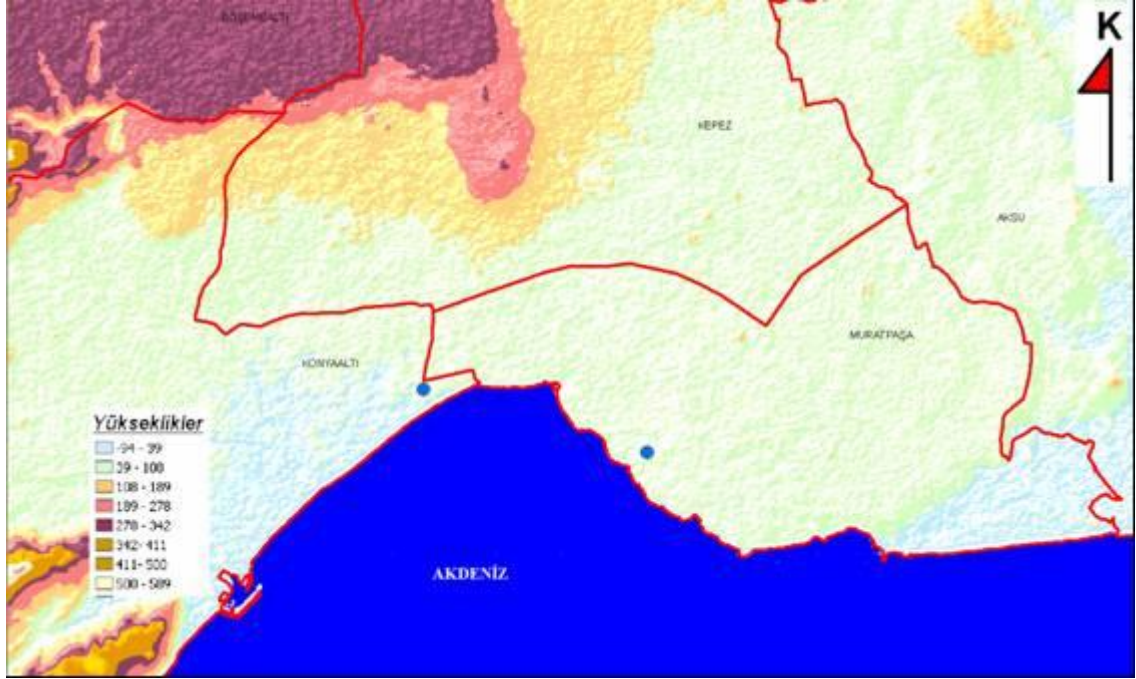
Şekil 4.13 Antalya şehrinde yüksekliğe göre dağılımı
