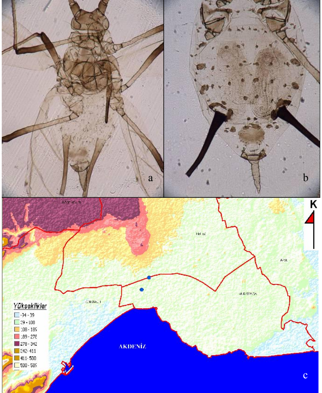
Şekil 4.49 Uroleucon (Uromelan) aeneum Hille Ris Lambers'un: a. kanatlı bireyi, b. kanatsız bireyinde abdomen, c. Antalya şehrinde yüksekliğe göre dağılımı
