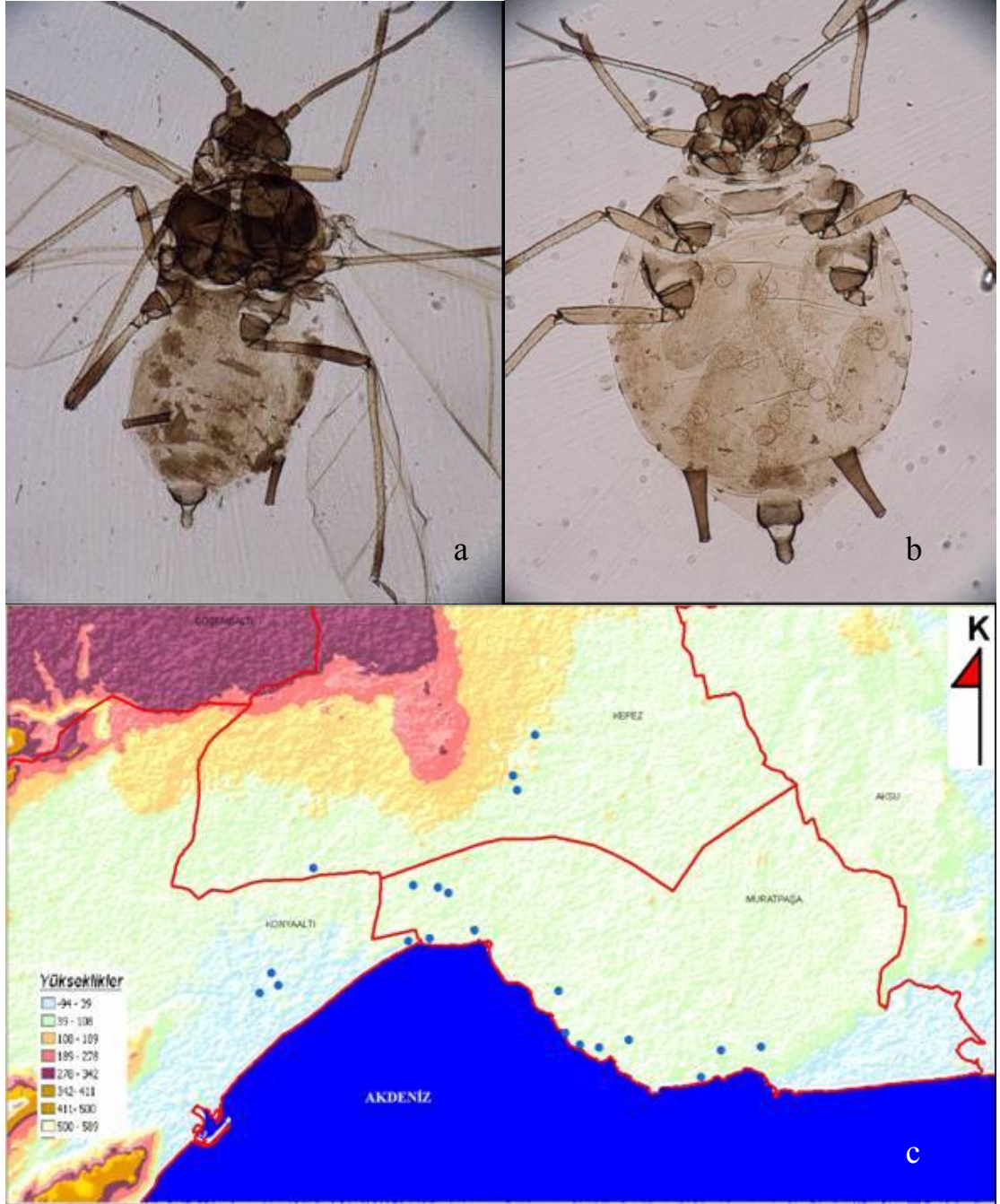
Şekil 4.12 Aphis punicae Passerini'nin: a. kanatlı bireyi, b. kanatsız bireyi, c. Antalya şehrinde yüksekliğe göre dağılımı.
