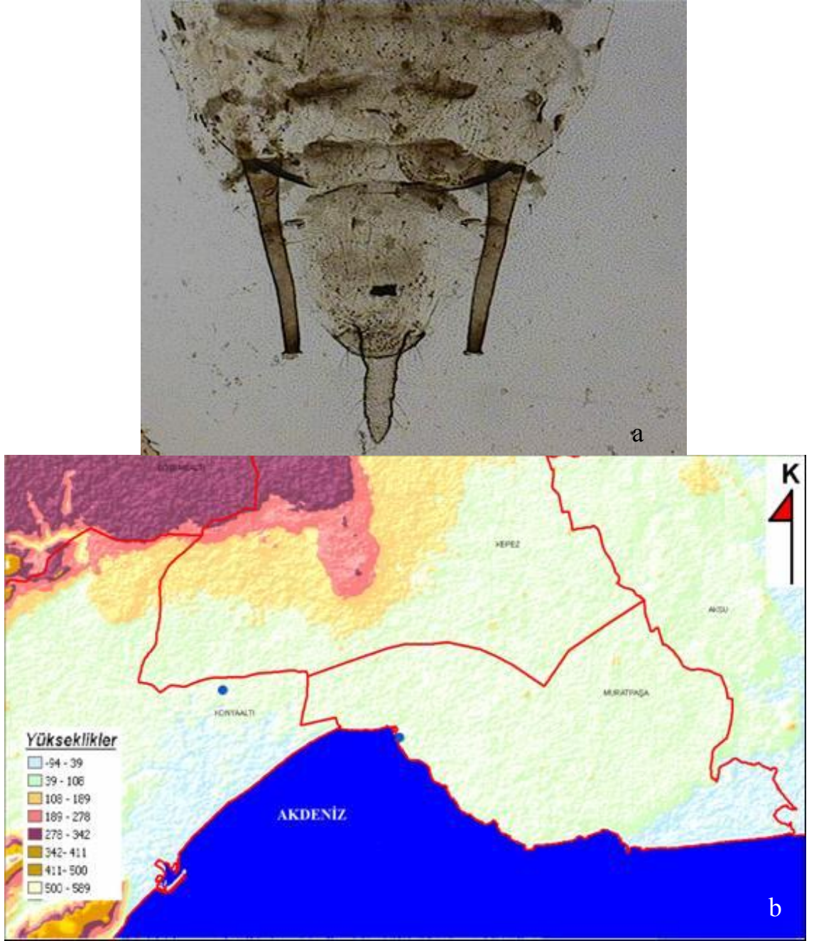
Şekil 4.44 Nasonovia ribisnigri (Mosley)'nin: a. kanatsız bireyinde kauda ve kornikıl, b. Antalya şehrinde yüksekliğe göre dağılımı
