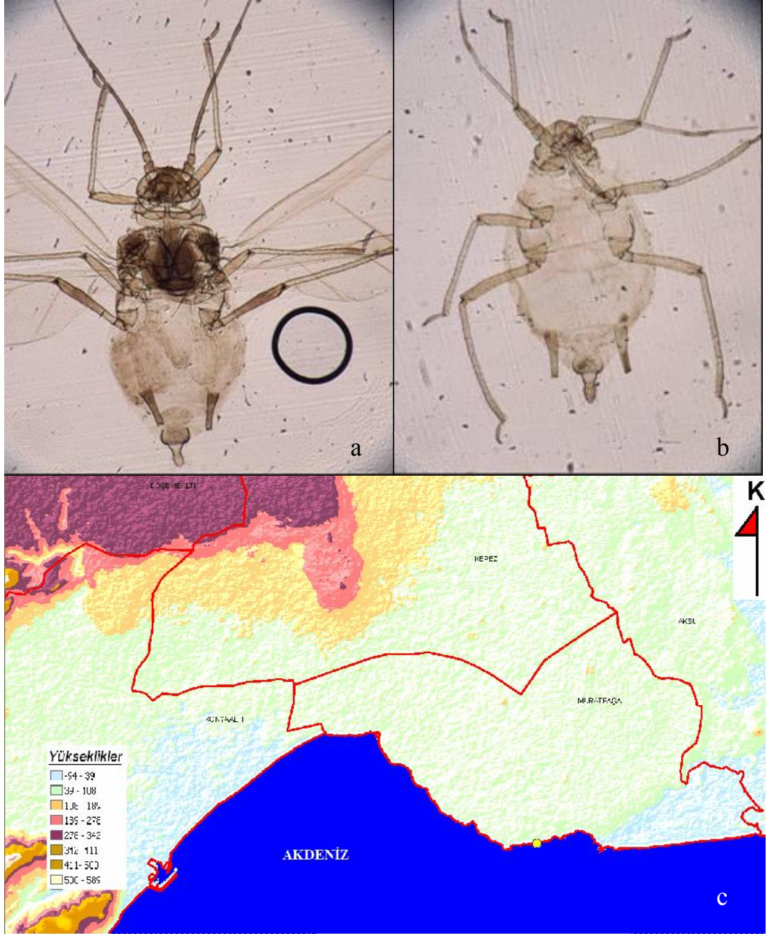
Şekil 4.19 Aphis viticis Ferrari'nin: a. kanatlı bireyi, b. kanatsız bireyi, c. Antalya şehrinde yüksekliğe göre dağılımı
