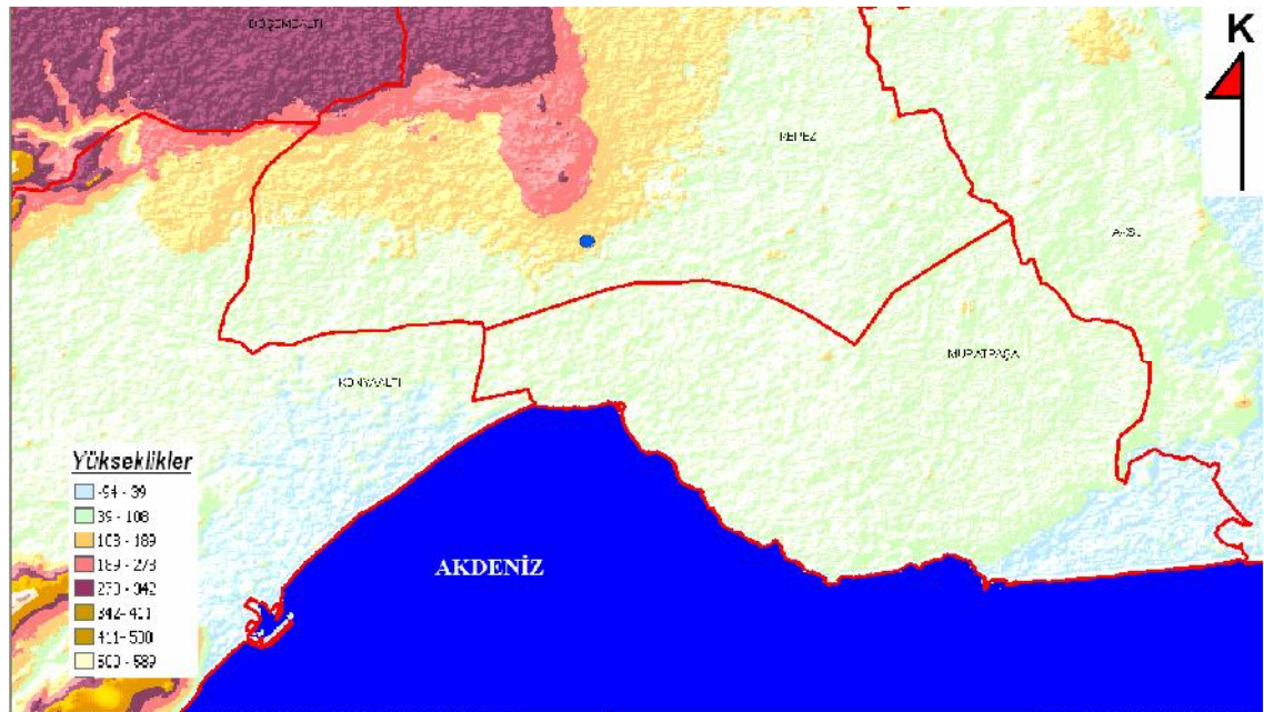
Şekil 4.27 Brachycaudus (Acaudus) persicae (Passerini)'nin Antalya şehrinde yüksekliğe göre dağılımı
