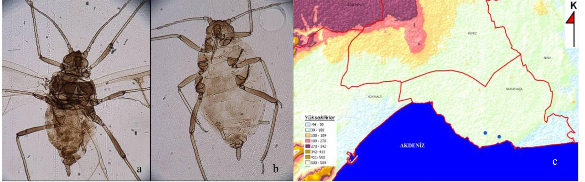
Şekil 4.35 Hyadaphis coriandri (B. Das)'nin: a. kanatlı bireyi, b. kanatsız bireyi, c. Antalya şehrinde yüksekliğe göre dağılımı
