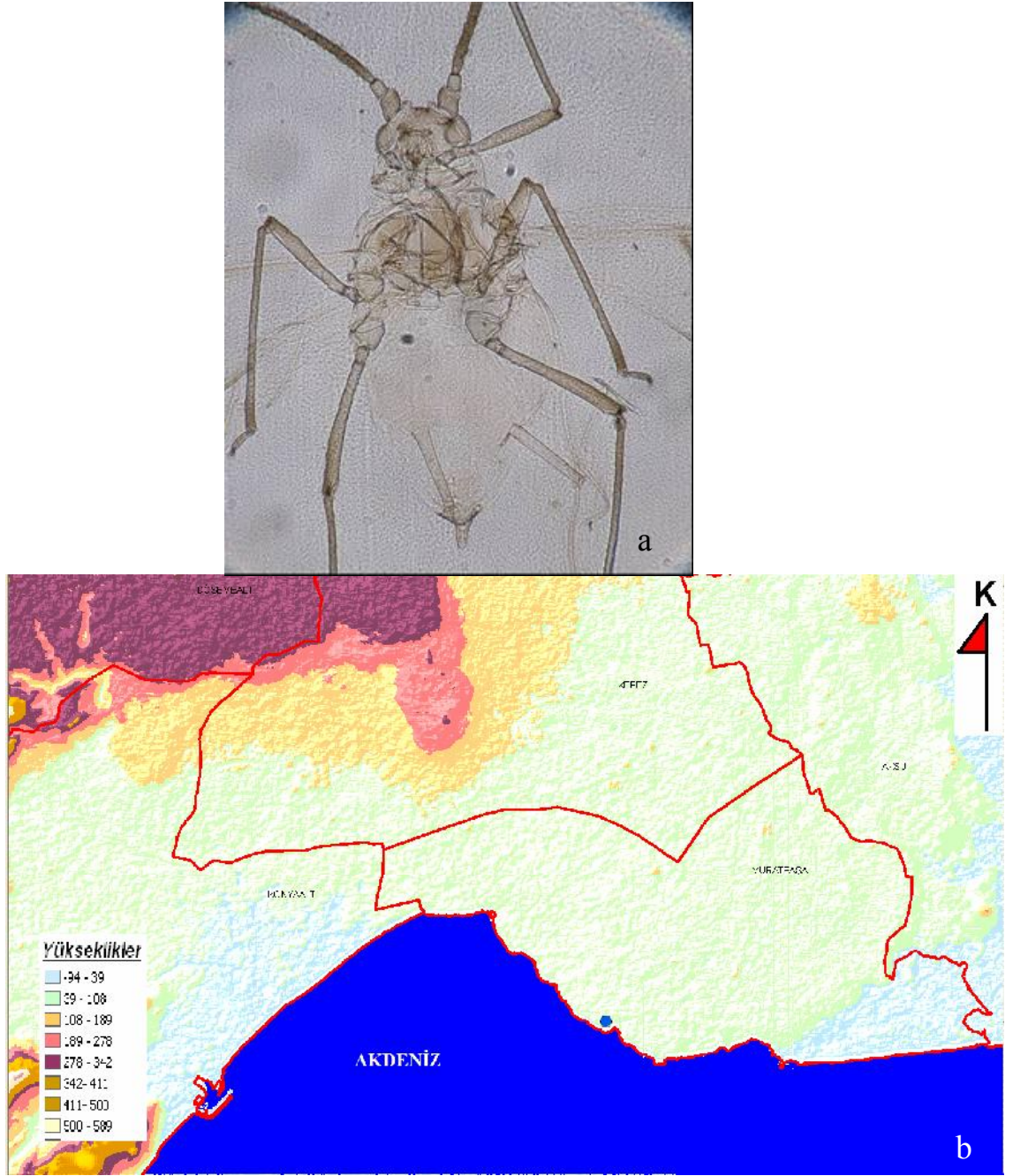
Şekil 4.45 Ovatus crataegarius (Walker)'un: a. kanatlı bireyi, b. Antalya şehrinde yüksekliğe göre dağılımı
