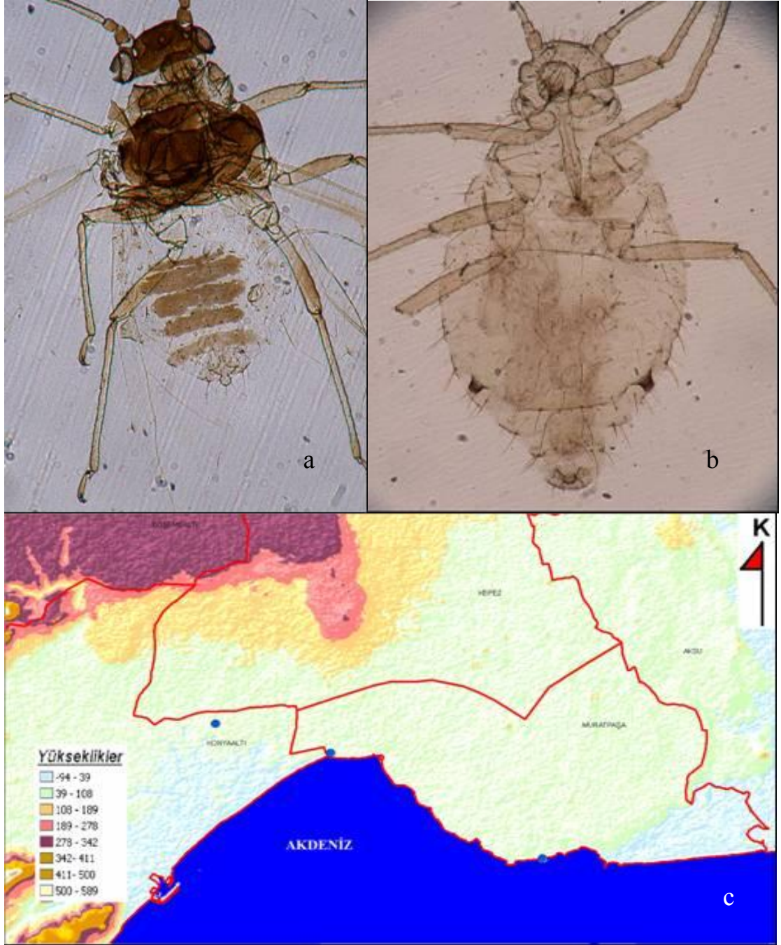
Şekil 4.51 Chaitophorus leucomelas Koch'ın: a. kanatlı bireyi, b. kanatsız bireyi, c. Antalya şehrinde yüksekliğe göre dağılımı
