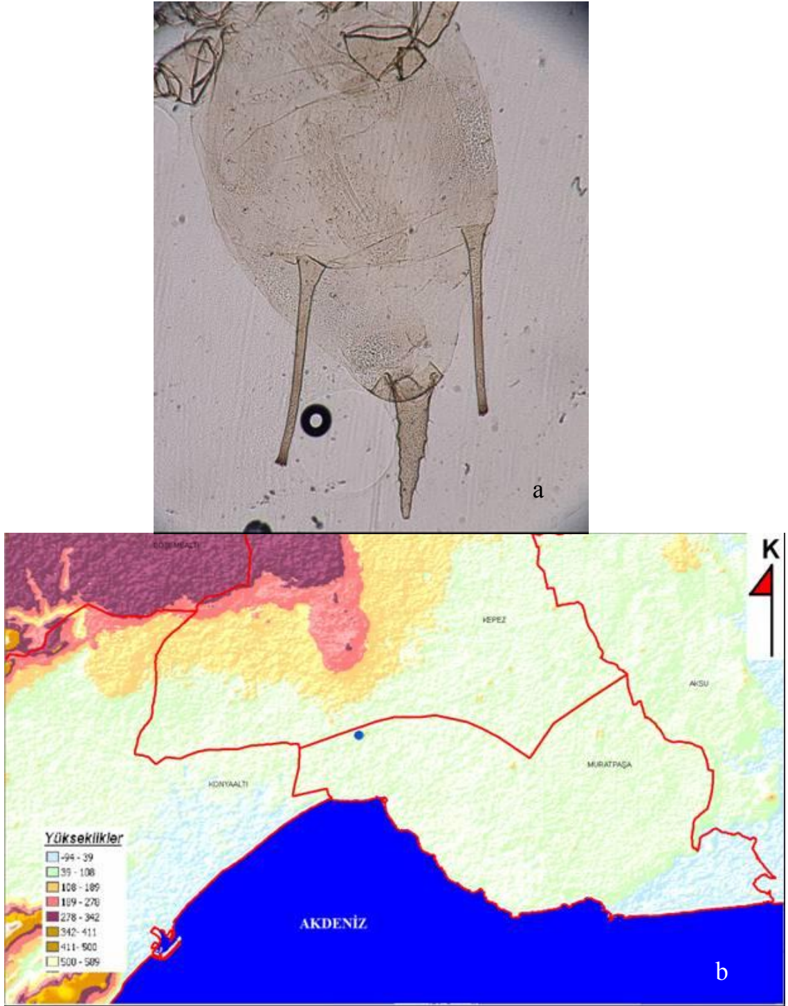
Şekil 4.23 Acyrthosiphon pisum (Harris)'un: a. kanatsız bireyinde abdomen, b. Antalya şehrinde yüksekliğe göre dağılımı.
