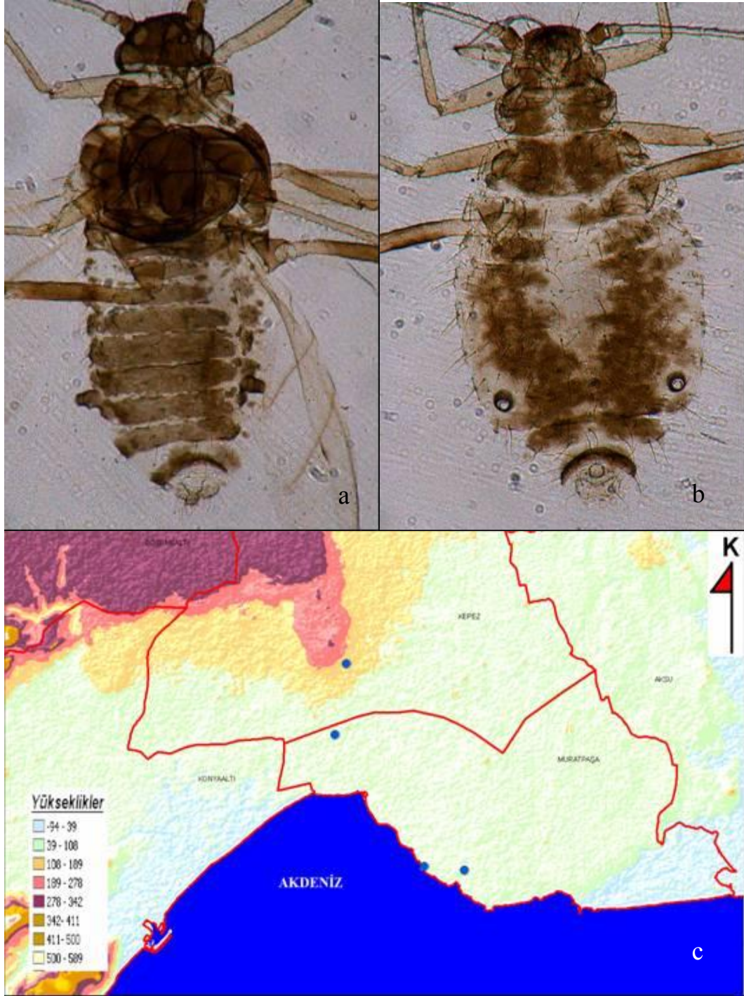
Şekil 4.53 Chaitophorus populialbae (Boyer de Fonscolombe)'nın: a. kanatlı bireyi, b. kanatsız bireyi, c.) Antalya şehrinde yüksekliğe göre dağılımı
