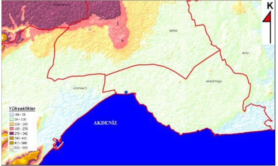
Şekil 4.33 Dysaphis crataegi (Kaltenbach)'nin Antalya şehrinde yüksekliğe göre dağılımı
