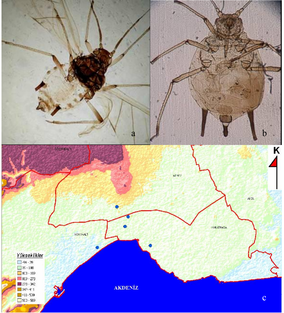
Şekil 4.18 Aphis verbasci Schrank'ın: a. kanatlı bireyi, b. kanatsız bireyi, c. Antalya şehrinde yüksekliğe göre dağılımı.
