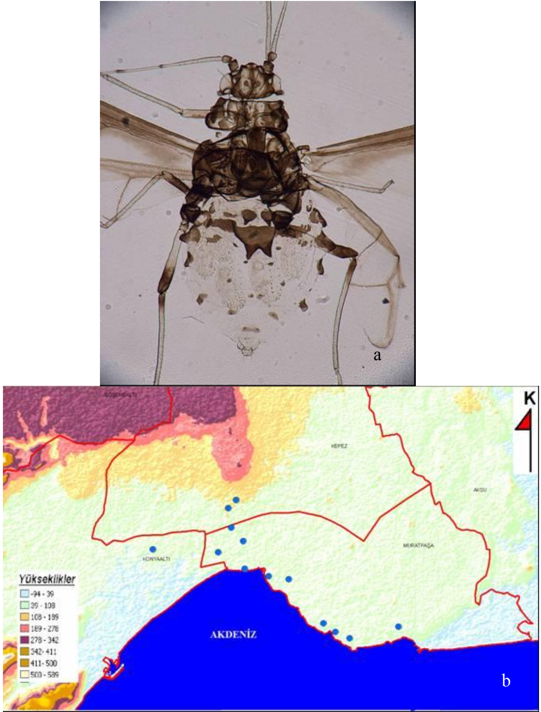
Şekil 4.57 Tinocallis kahawaluokalani (Kirkaldy)'nin: a. kanatlı bireyi, b. Antalya şehrinde yüksekliğe göre dağılımı
