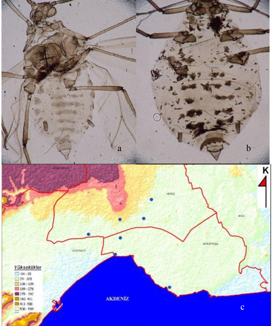
Şekil 4.28 Brevicoryne brassicae (Linnaeus)’nin: a. kanatlı bireyi, b. kanatsız bireyi, c. Antalya şehrinde yüksekliğe göre dağılımı
