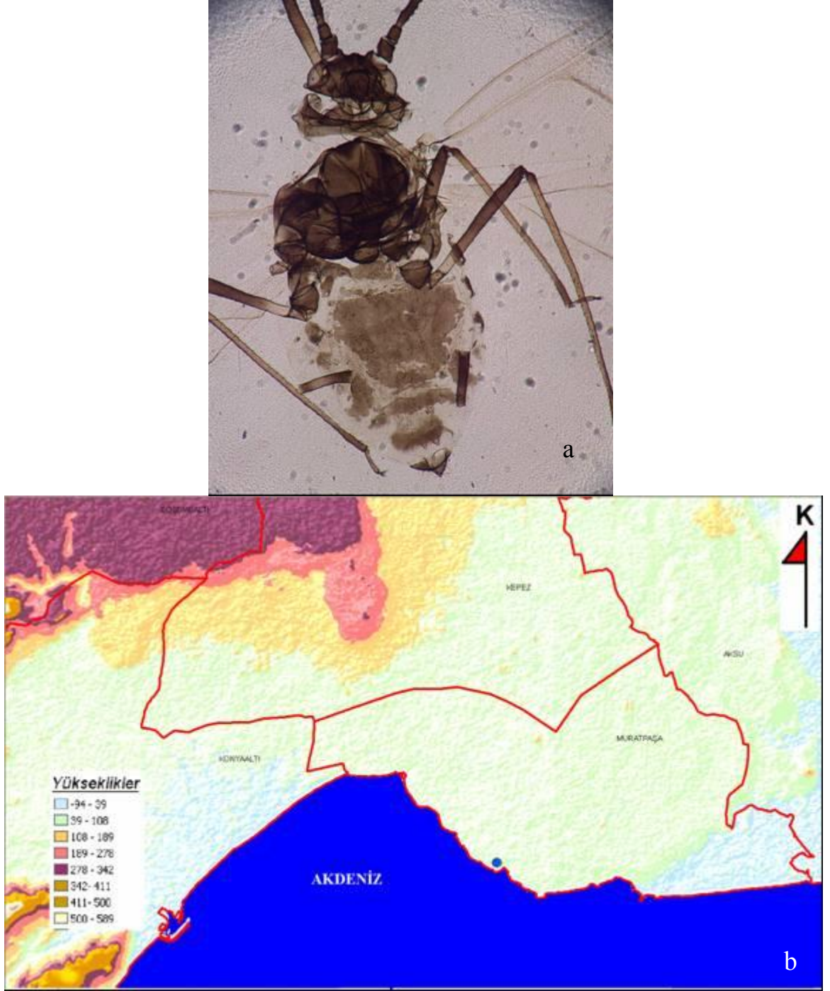
Şekil 4.34 Dysaphis (Pomaphis) plantaginea (Passerini)'nin: a. kanatlı bireyi, b. Antalya şehrinde yüksekliğe göre dağılımı.
