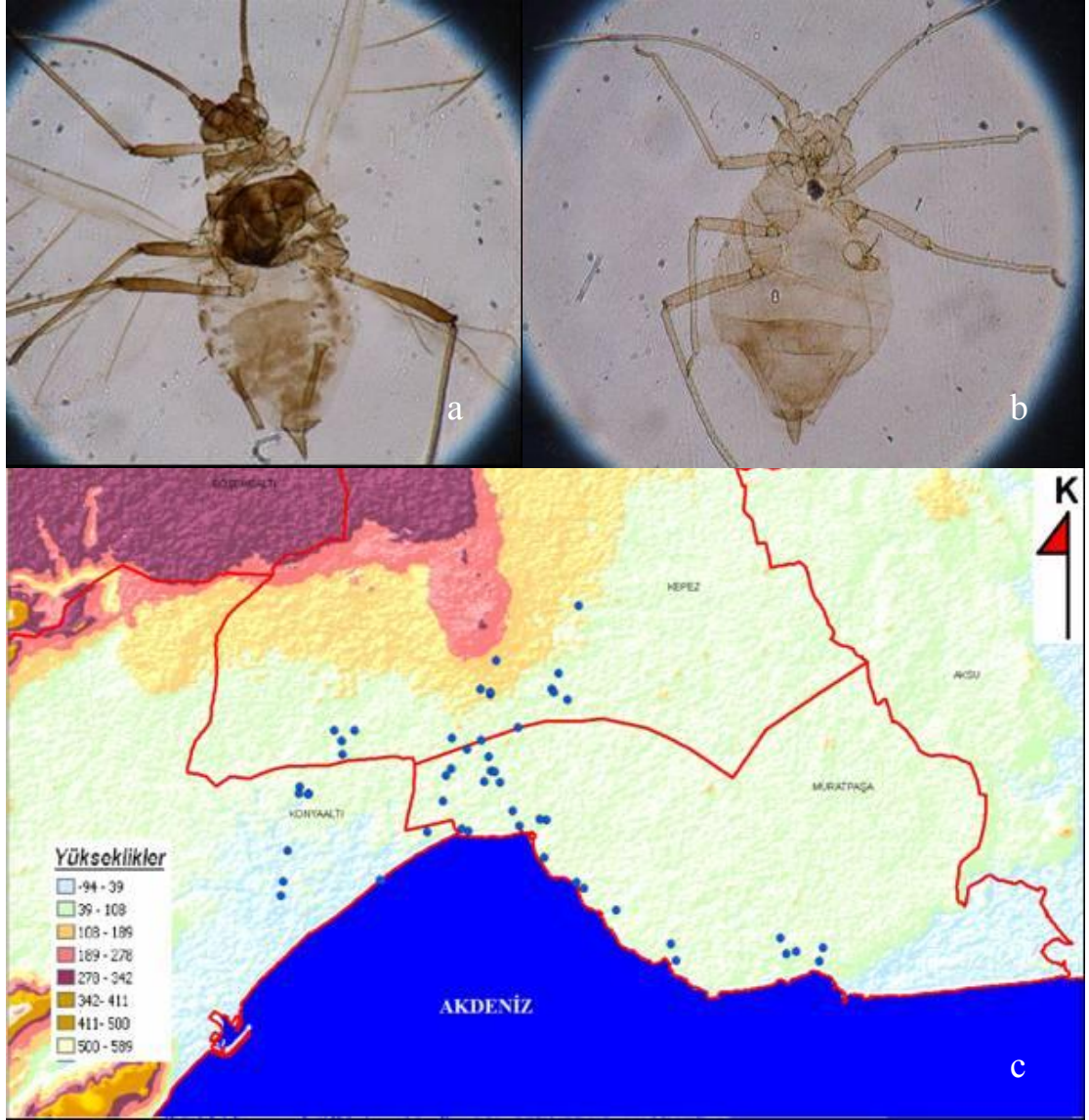
Şekil 4.43 Myzus (Nectarosiphon) persicae (Sulzer)'nin: a. kanatlı bireyi, b. kanatsız bireyi, c. Antalya şehrinde yüksekliğe göre dağılımı
