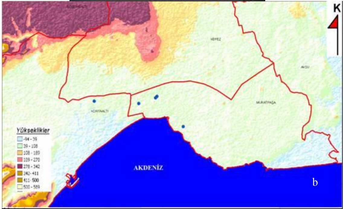
Şekil 4.32 Chaetosiphon (Pentatrachopus) tetrahodum Walker'un: a. kanatlı bireyi, b. Antalya şehrinde yüksekliğe göre dağılımı.
