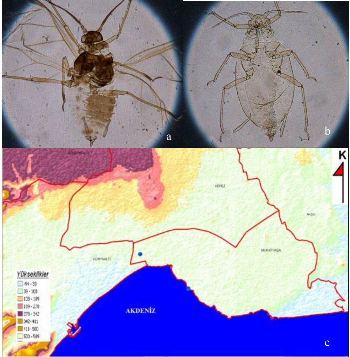
Şekil 4.31 Cavariella aegopodii (Scopoli)'nin: a. kanatlı bireyi, b. kanatsız bireyi, c. Antalya şehrinde yüksekliğe göre dağılımı
