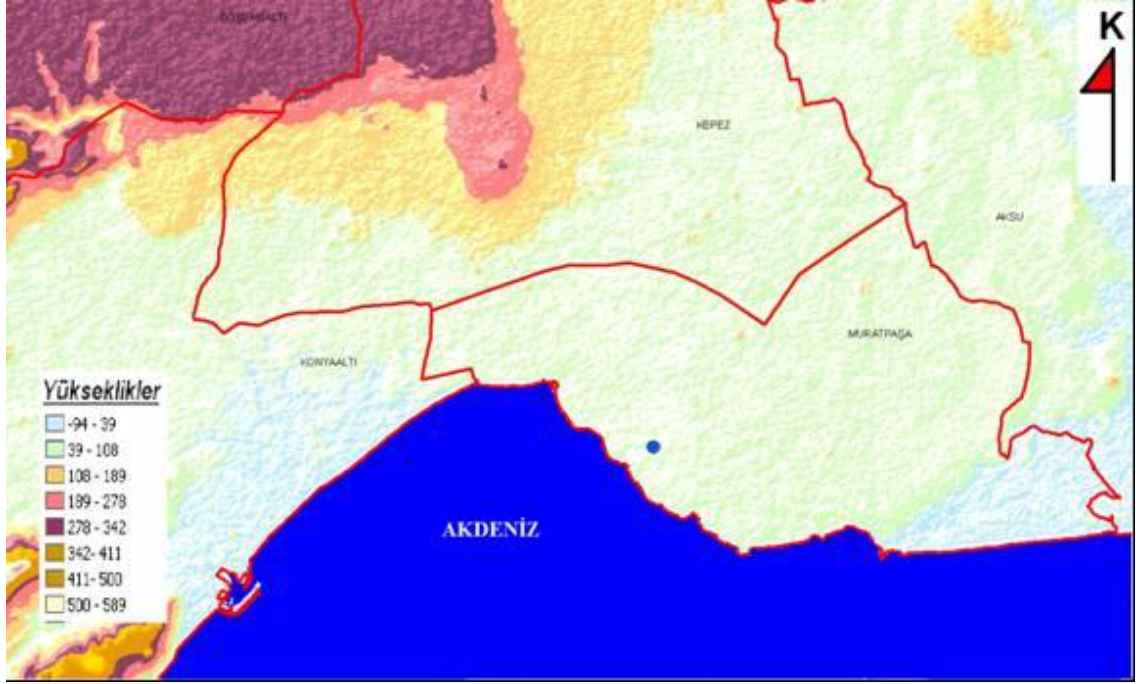
Şekil 4.58 Eriosoma lanigerum (Hausmann)'un Antalya şehrinde yüksekliğe göre dağılımı
