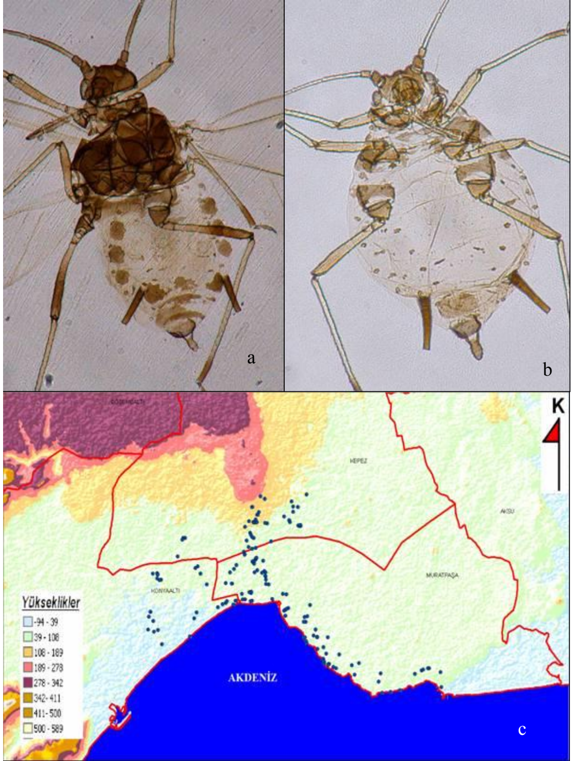
Şekil 4.8 Aphis gossypii Glover'in: a. kanatlı bireyi, b. kanatsız bireyi, c. Antalya şehrinde yüksekliğe göre dağılımı
