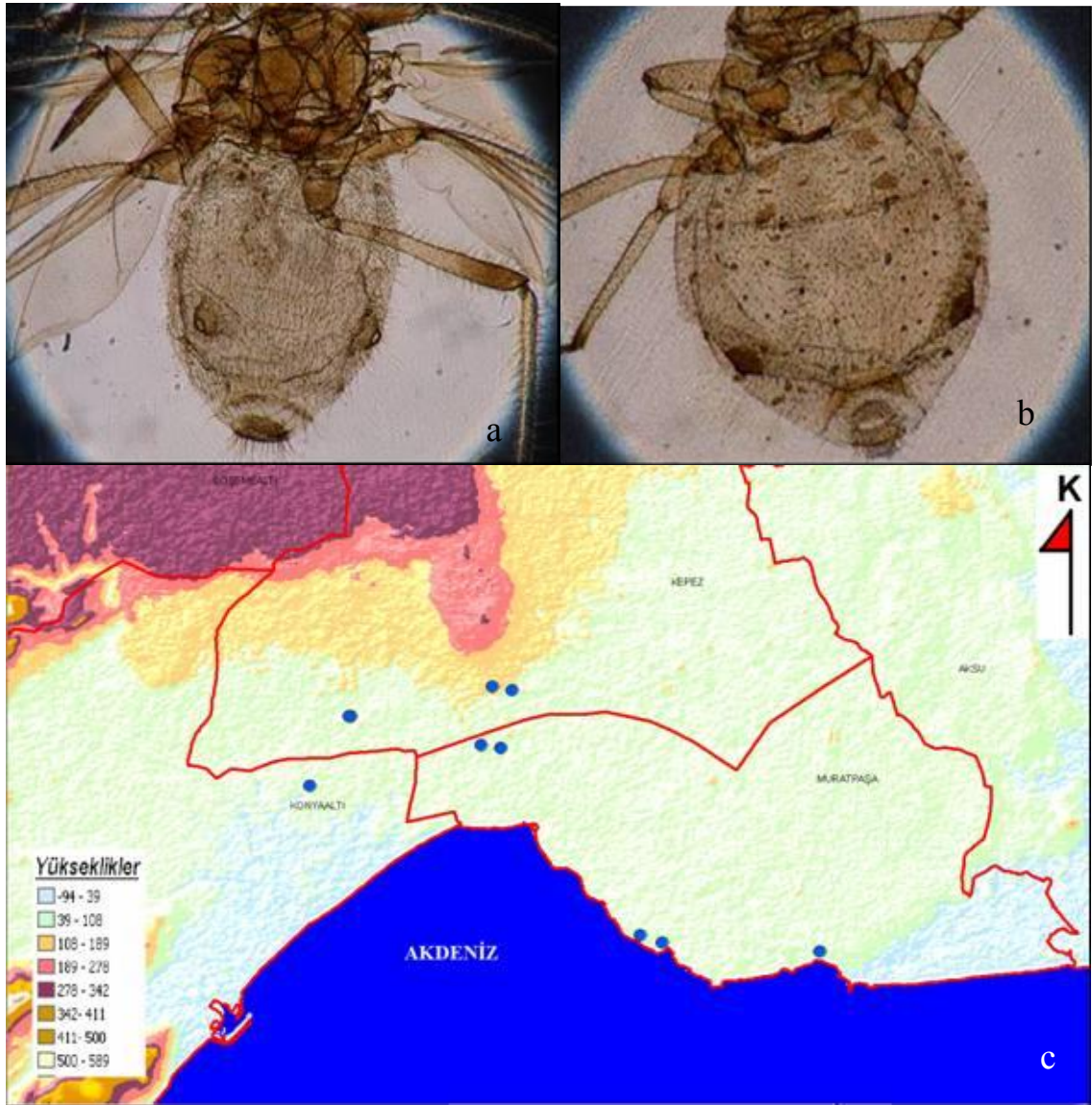
Şekil 4.55 Cinara (Cupressobium) cupressi (Buckton)’nin: a. kanatlı bireyi, b. kanatsız bireyi, c. Antalya şehrinde yüksekliğe göre dağılımı
