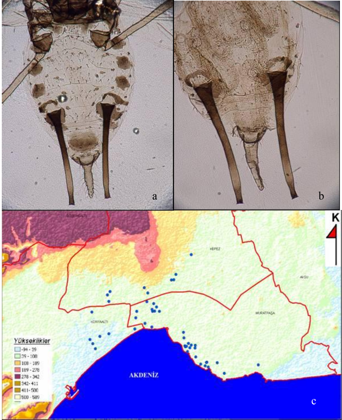
Şekil 4.40 Macrosiphum rosae (Linnaeus)'nin: a. kanatlı bireyinde abdomen, b. kanatsız bireyinde abdomen, c. Antalya şehrinde yüksekliğe göre dağılımı
