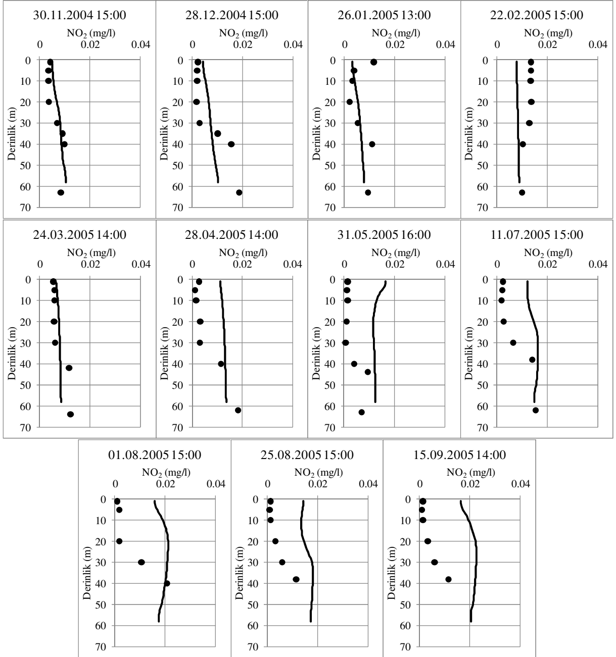
Şekil 6.133 B7 İstasyonunda \text{NO}_2 veri seti için model sonuçları ile ölçümlerin düşey profiller üzerinde karşılaştırılması. •: ölçüm verileri —: model sonuçları.
