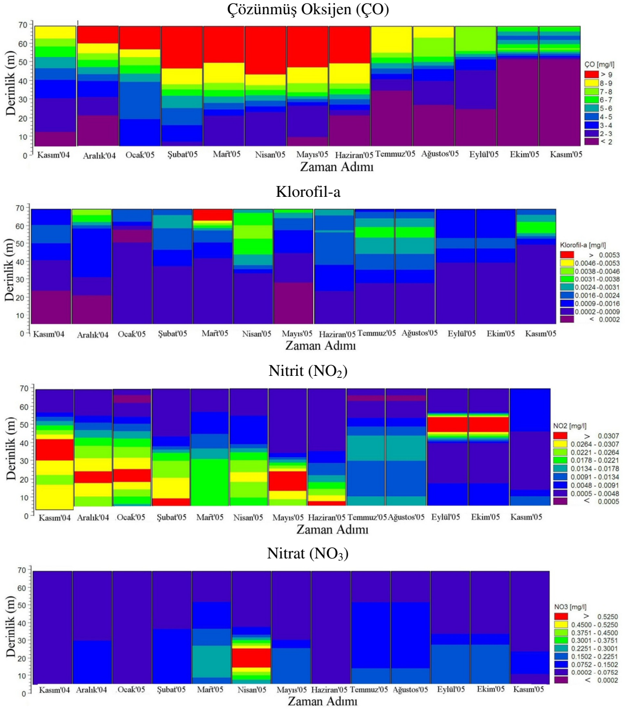
Şekil 6.96 Marmara Denizi Sınırında durum değişkenlerine ait konsantrasyon sınır şartları.
