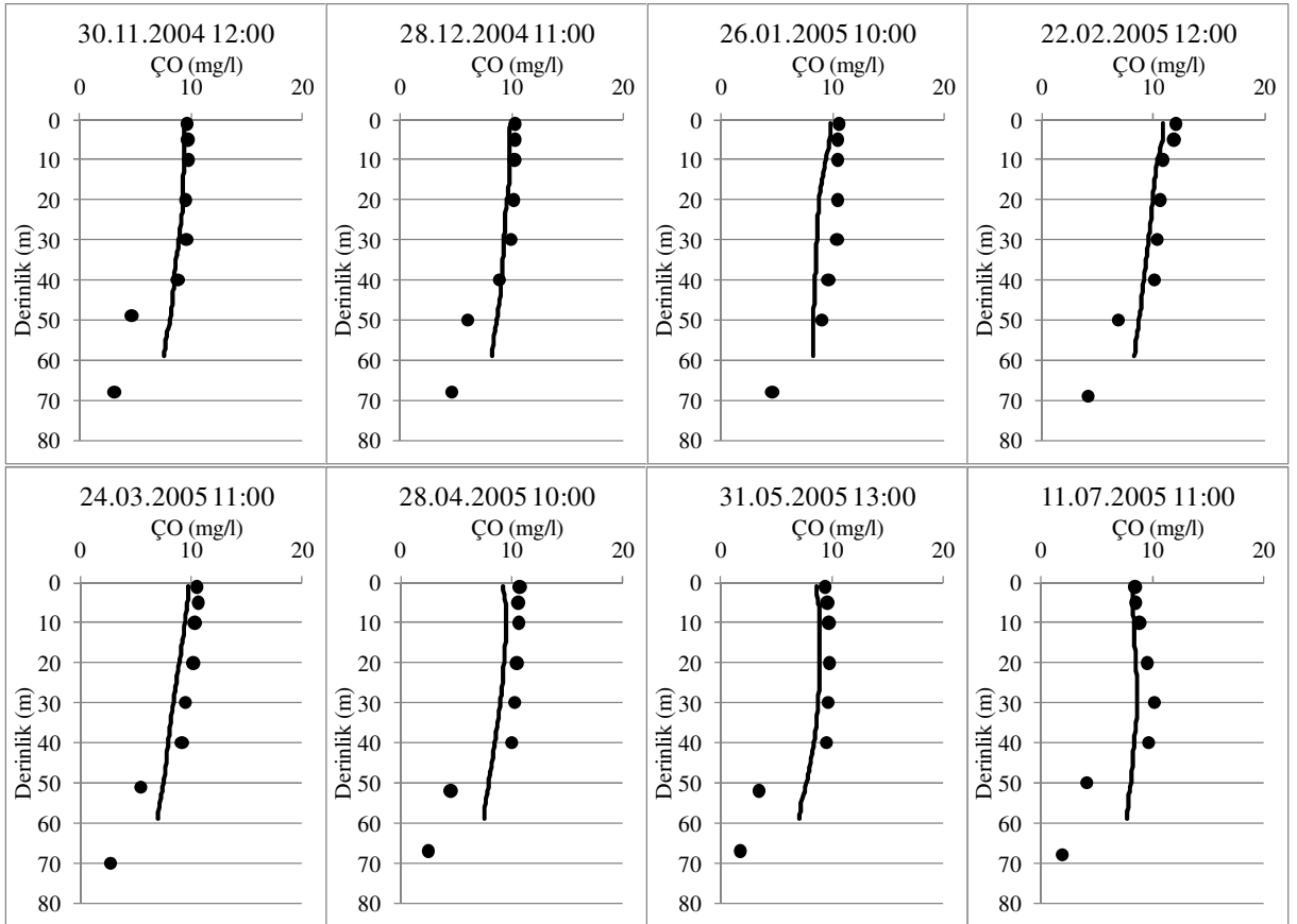
Şekil 6.120 K0 İstasyonunda \dot{C}O veri seti için model sonuçları ile ölçümlerin düşey profiller üzerinde karşılaştırılması. •: ölçüm verileri —: model sonuçları.
