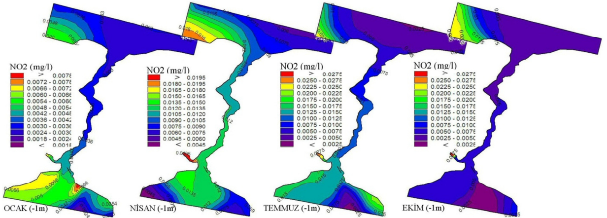
Şekil 6.159 Ocak, Nisan, Temmuz ve Ekim aylarında NO 2 konsantrasyonlarının yüzeyden 1 m, 10 m, 20 m ve 40 m derinliklerde model alanı içerisindeki değişimleri.
