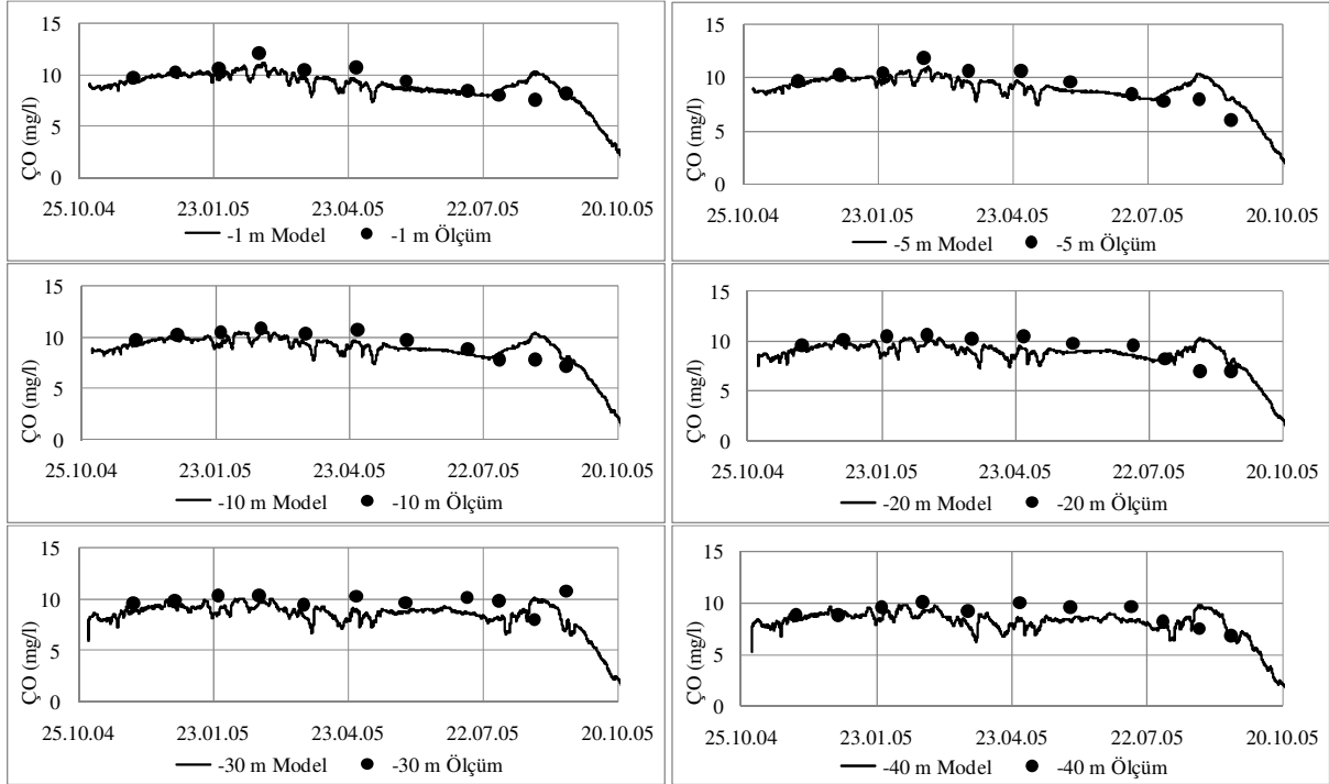
Şekil 6.115 K0 İstasyonunda tüm veri seti için farklı derinliklerde \text{ÇO} konsantrasyonlarının değişimine dair zaman serileri. •: ölçüm verileri —: model sonuçları.
