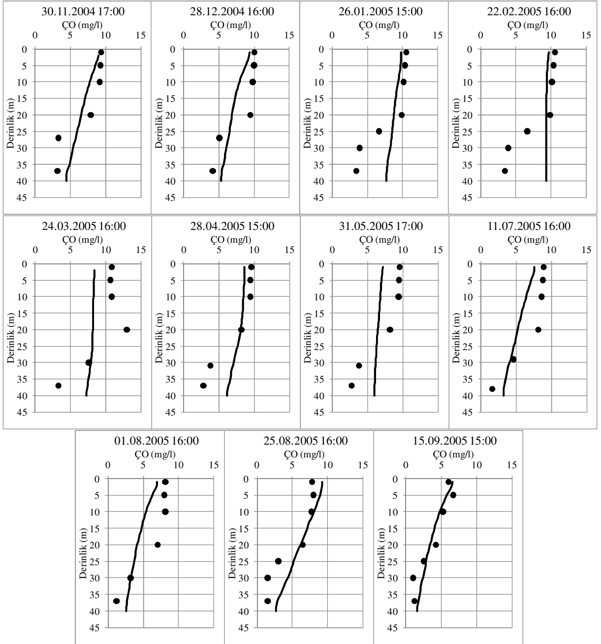
Şekil 6.142 B2 İstasyonunda \text{CO} veri seti için model sonuçları ile ölçümlerin düşey profiller üzerinde karşılaştırılması. •: ölçüm verileri —: model sonuçları.
