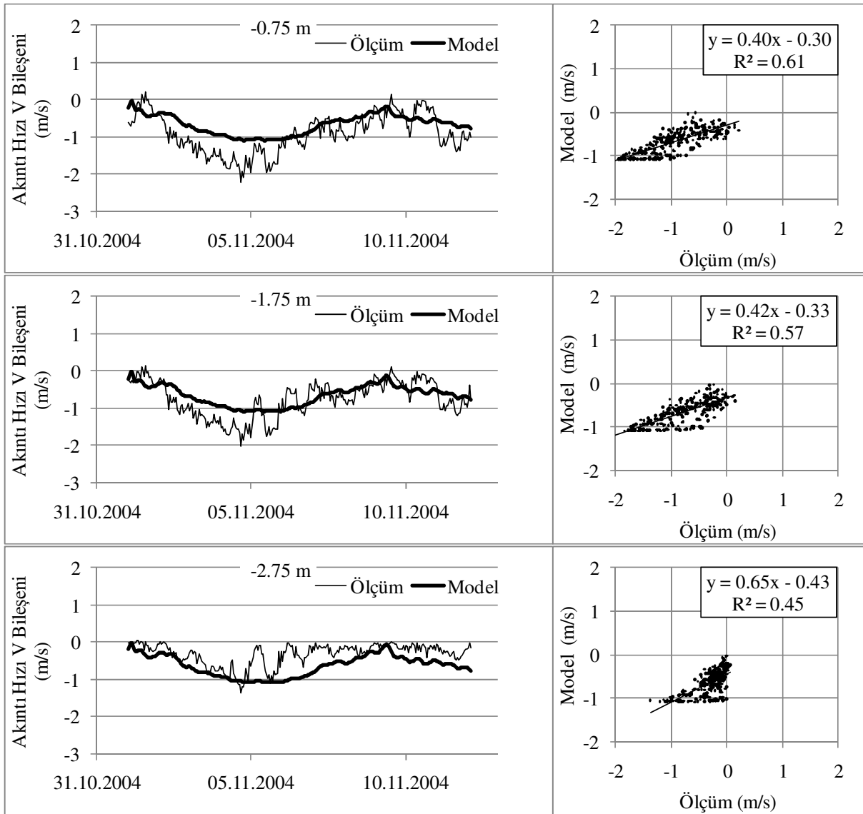
Şekil 6.61 Kalibrasyon dönemi içerisinde B istasyonundaki V akıntı hız bileřenlerinin ölçülen ve modellenen deęerlerinin karşılaştırılması için yüzeyden (-0.75 m), tabana (-23.75 m) kadar bir metrelik aralıklarla tüm derinliklerdeki zaman serileri, daęılım grafikleri ve determinasyon katsayıları.
