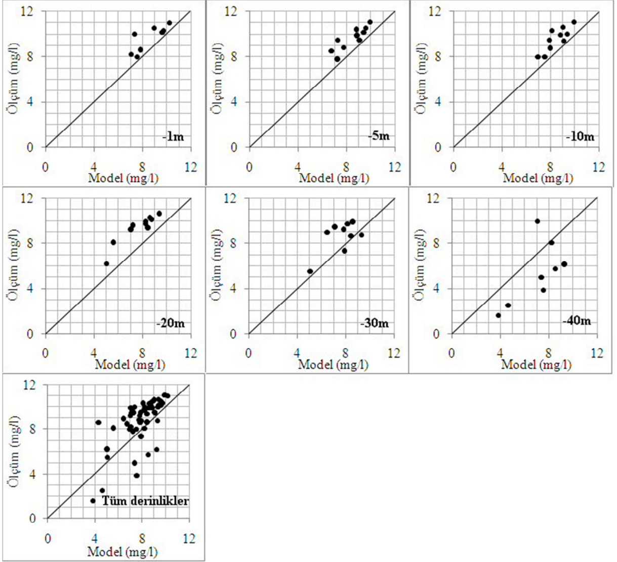
Şekil 6.136 B7 İstasyonunda tüm veri seti ve tüm su kalitesi durum değişkenleri için model sonuçları-ölçüm verileri saçılım diyagramları.
