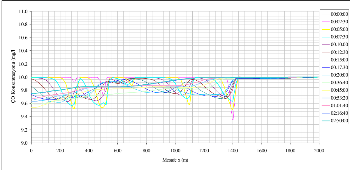
Şekil 6.38 7. Benzetimin çeşitli zaman adımlarında ÇO konsantrasyonunun kanal ekseninde yüzeyde değişimi.
