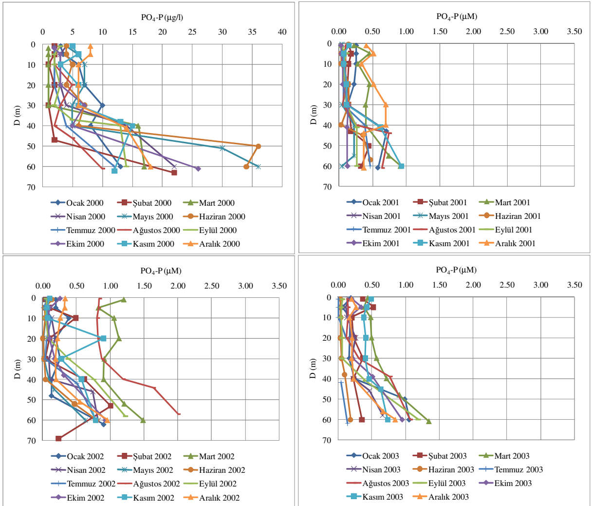
Şekil 4.18 B13 istasyonunda 2000-2006 yılları arasında PO_4\text{-P} konsantrasyonlarının değişimi.
