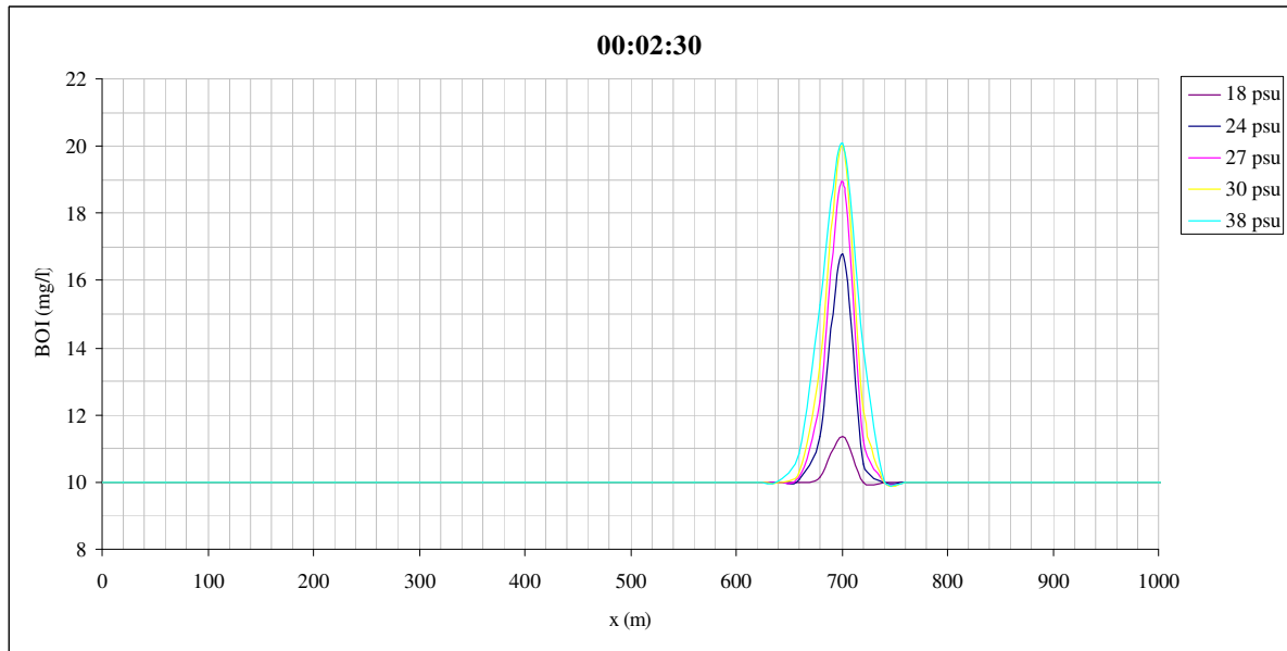
Şekil 6.35 Kanalındaki farklı tuzluluk değerleri için benzetimin başlamasından 2 dak. 30 s. sonra BOİ ve ÇO konsantrasyonunun değişimi.
