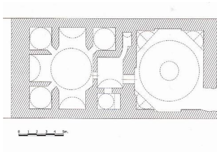
Şekil 3.53 : Saray Hamamı: (a) batıdan görünüm, (b) sıcaklık, (c) plan 35 , (d) vaziyet planı
