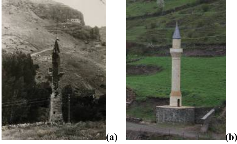
Şekil 4. 8 : Minare I, Çarşı Camii: restorasyon öncesi (a) 51 ve sonrası (b)
