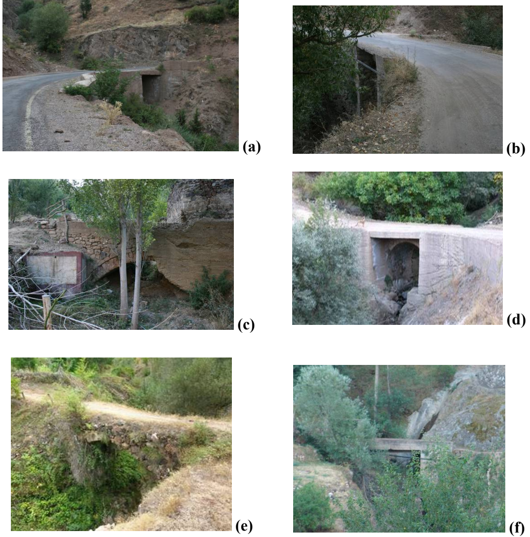
Şekil 3.59 : Köprüler: (a) 138 Env.No'lu yerleşim girişindeki köprü, (b) 118 Env. No'lu Musalla Deresi üzerindeki köprü, (c) 42 Env.No'lu Dabakhane Köprüsü, (d) 44 Env.No'lu Musalla Deresi üzerinde Çarşı mahallesindeki köprü, (e) 98 Env.No'lu Musalla Deresi üzerindeki müdahale edilmemiş köprü, (f) 81 Env.No'lu Koroçim Mevkii'ndeki köprü
