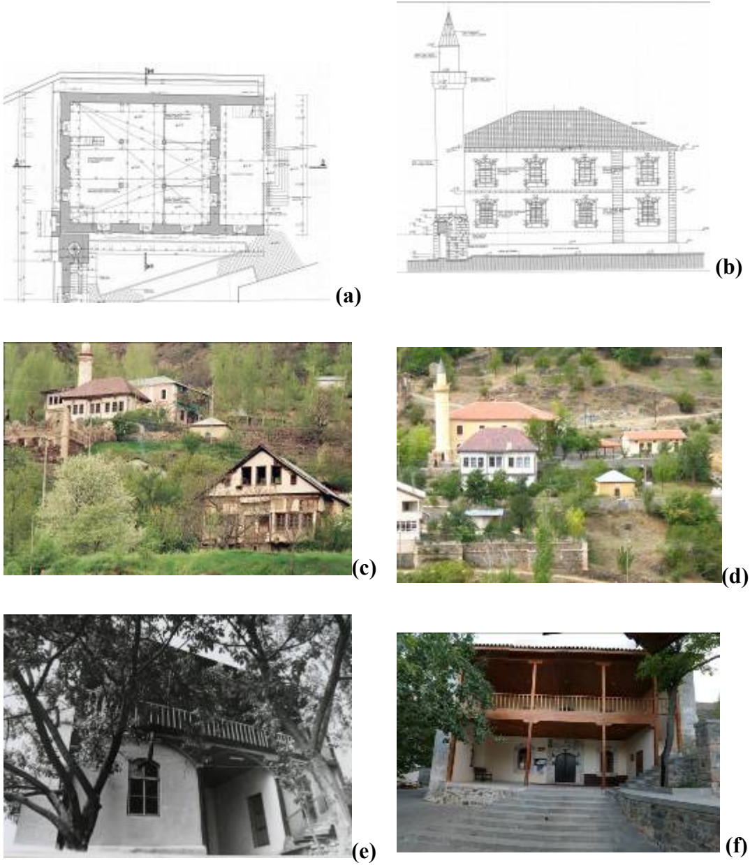
Şekil 4. 6 : Süleymaniye Camisi Restorasyon Projesi zemin kat planı (a) ve doğu cephesi (b) 45 ; cami ve bahçesinin 1990’lardaki görünümü (c) 46 ve restorasyon sonrası görünümü (d); son cemaat yerinin restorasyon öncesi (e) 47 ve sonrası (f) görünüşü
