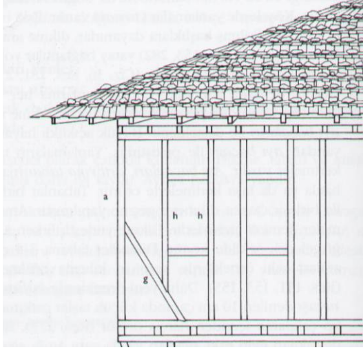
Şekil 3.71 : Hartama (Pedavra) çatı kaplaması (Günay, 1998, s.302)
