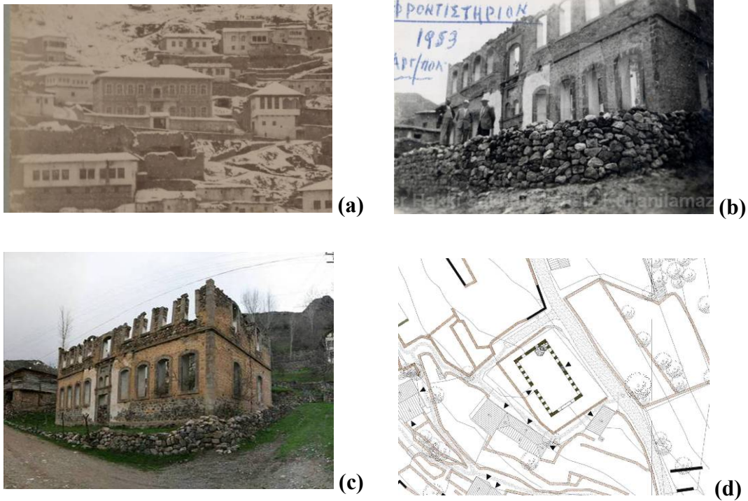
Şekil 3.49 : Rum Erkek Okulu (Frontistirion): (a) 19. yüzyıl sonlarında (Yıldız Albümleri), (b) 1953'te (Kostas Papadopoulos Arşivi), (c) günümüze, (d) vaziyet planı
