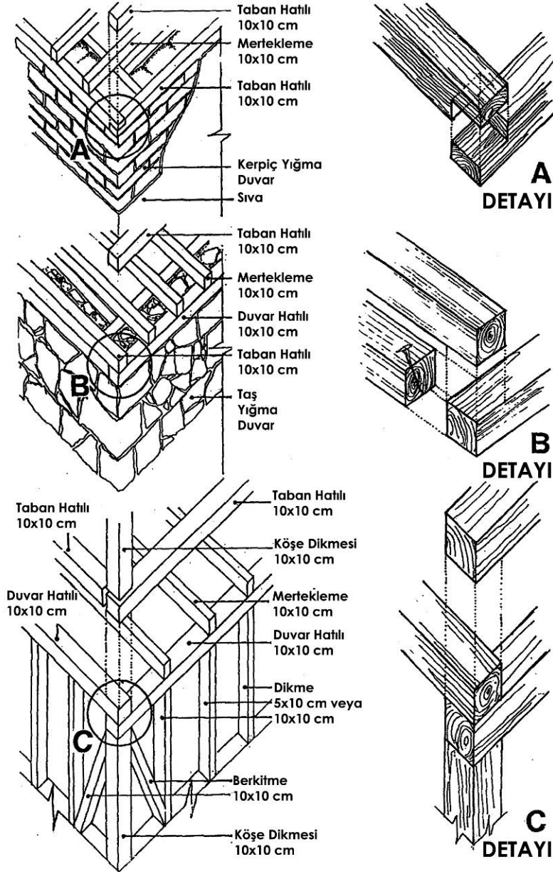
Şekil 3.70 : Ahşap ve taş bölümler arası birleşim detayları (Şahin, 1995, s.186)
