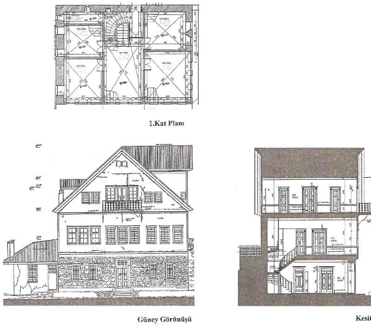
Şekil 3.67 : Yeni Gümüşhane’de 1920’lerde yapılan Hasan (Fehmi Ataç) Bey Konağı (Sağsöz, 2005, s. 1151-1153)
