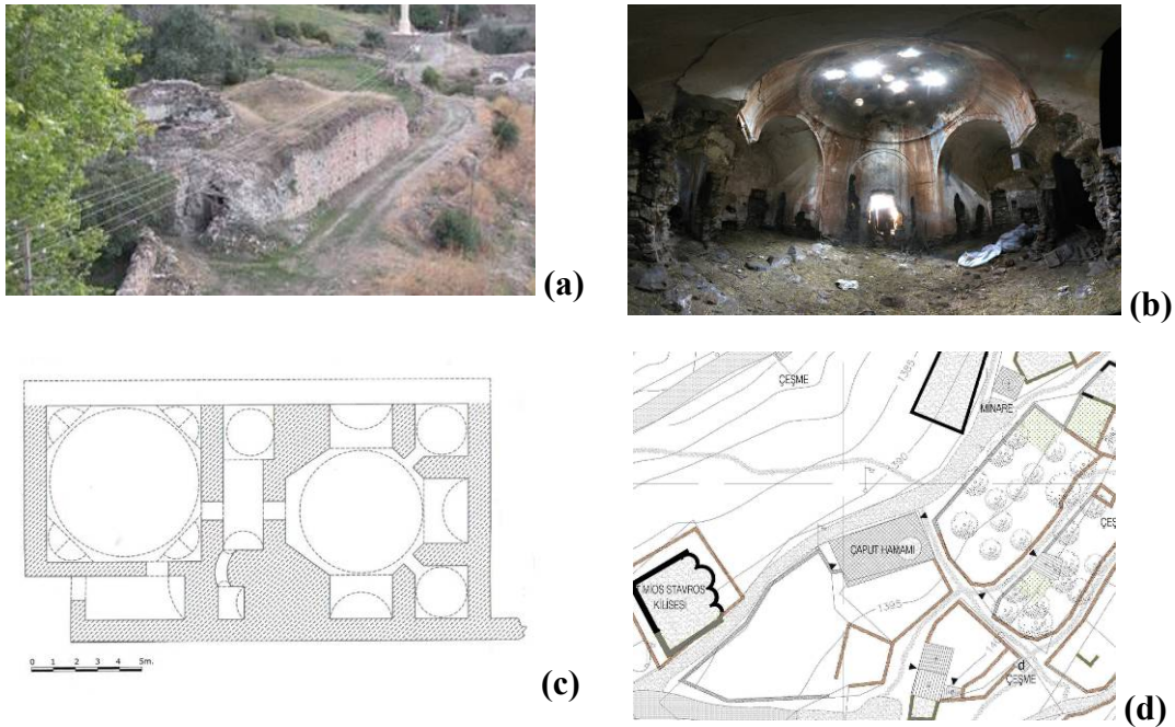
Şekil 3.55 : Çaput Hamamı: (a) kuzeyden/Cami-i Sagir minaresinden görünüm, (b) sıcaklık, (c) plan 37 , (d) vaziyet planı
