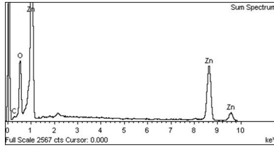
Şekil 4.105 150 mg/L VSA varlığında üretilen kristallerin sinterleme sonrasındaki EDX analizi sonucu
