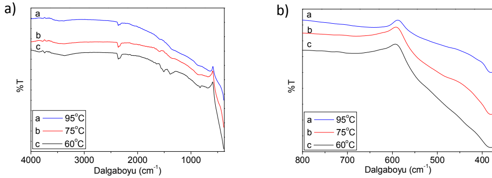
Şekil 4.4 Katkısız üretilen ZnO malzemelerinin FT-IR spektrumları
