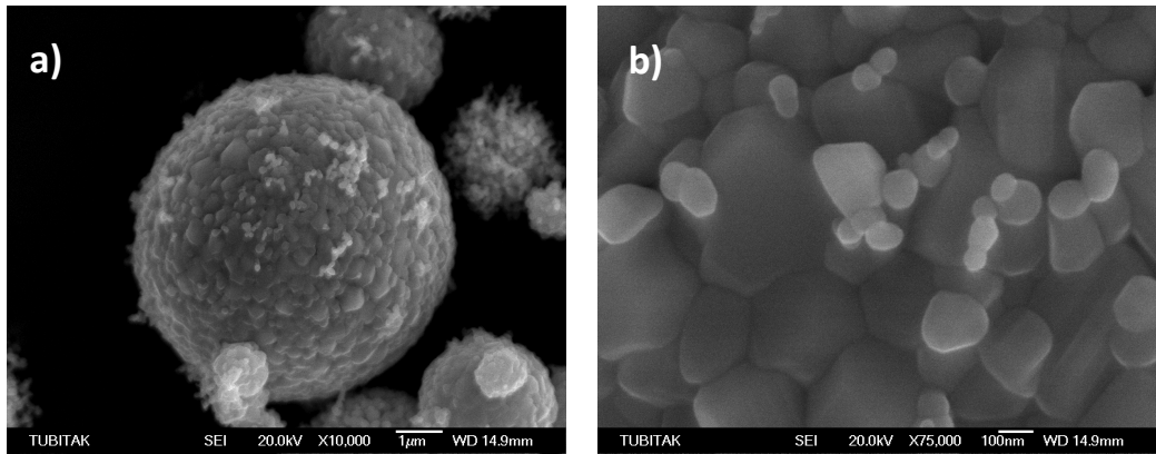
Şekil 4.64 95°C’de 3000 mg/L KI-15 varlığında üretilen kristallerin (SD135) 700°C’de sinterlenmesi sonrasındaki SEM fotoğrafları
