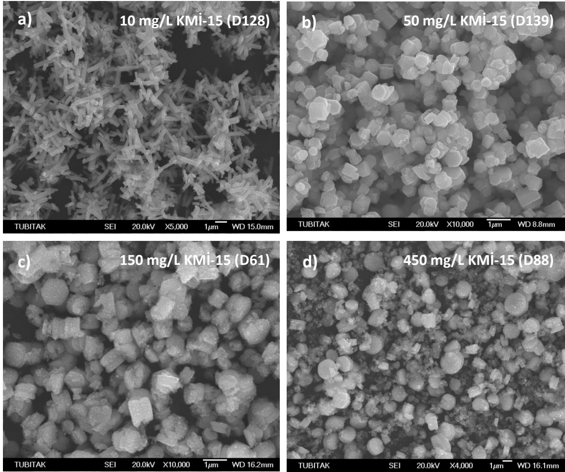
Şekil 4.52 95°C’de KMi-15 varlığında üretilen kristallerin SEM fotoğrafları
