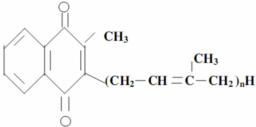
Şekil 7: K2 Vitamini (Menakinon-n, MK-n)
