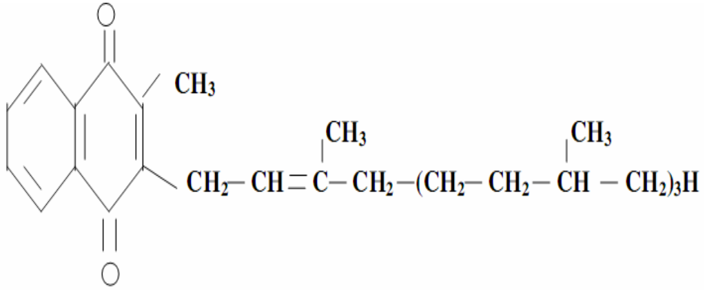
Şekil 6: K1 Vitamini (Fillokinon)
