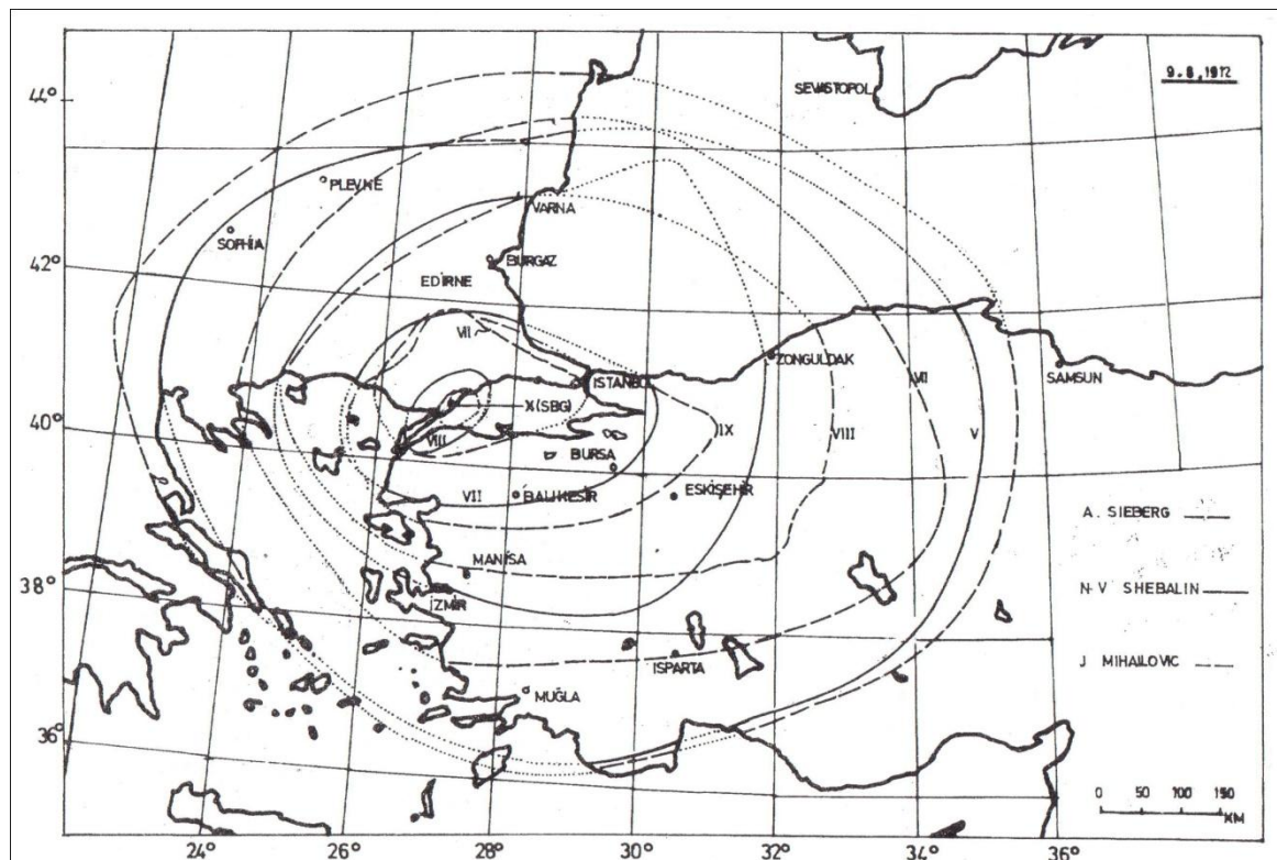
Şekil 1. Şarköy-Mürefte depreminin izozeismik haritası.
