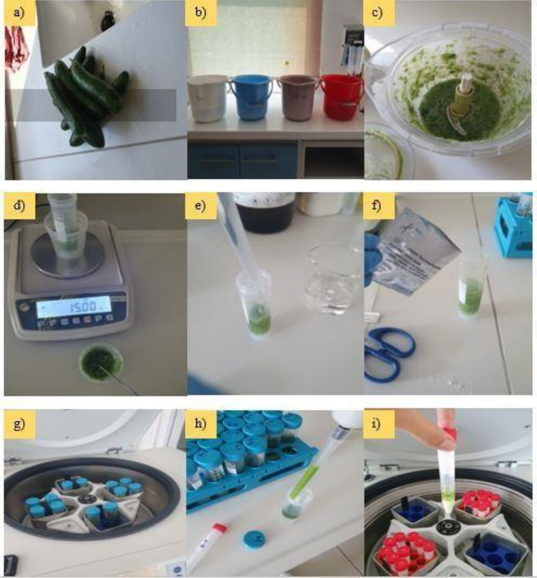
Şekil 3.3. a) Salatalıkların yıkanması, b) Çözeltilerin kovalara hazırlanması, c) Blenderle homojenizasyon, d) 15g numune tartılması, e) 15ml acetonitril çözeltisi eklenmesi, f) 6g susuz MgSO_4 , 1,5g NaAcetate eklenmesi, g) 10dk santrifüjleme h) Süpernatant fazından 4ml alınarak 1200mg MgO_4 ve 400mg PSA ekleme, i) 10 dk santrifüjleme
