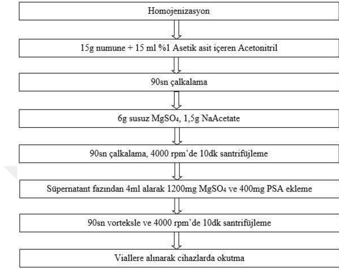
Şekil 3.4. QuEChERS (AOAC 2007.01) analiz yönteminin işlem akış şeması (Çiftçi 2019)
