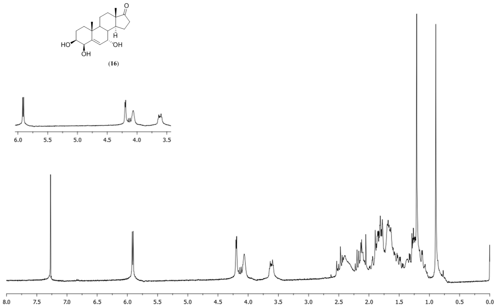
EK 14: 3 \beta ,4 \beta ,7 \alpha -Trihidroksiestandrost-5-en-17-on ( 16 ) için ^1\text{H} NMR spektrumu
