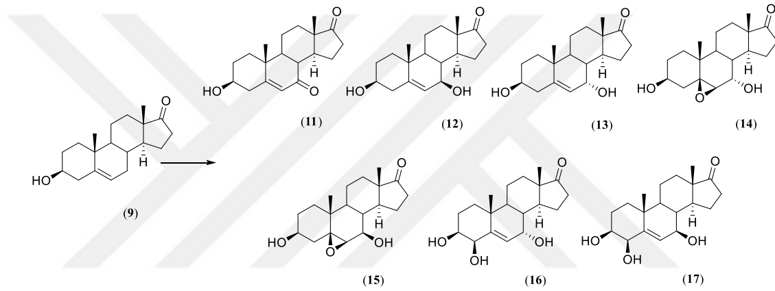
Şekil 5.1. Substratın U. chartarum ile biyotransformasyonu.
