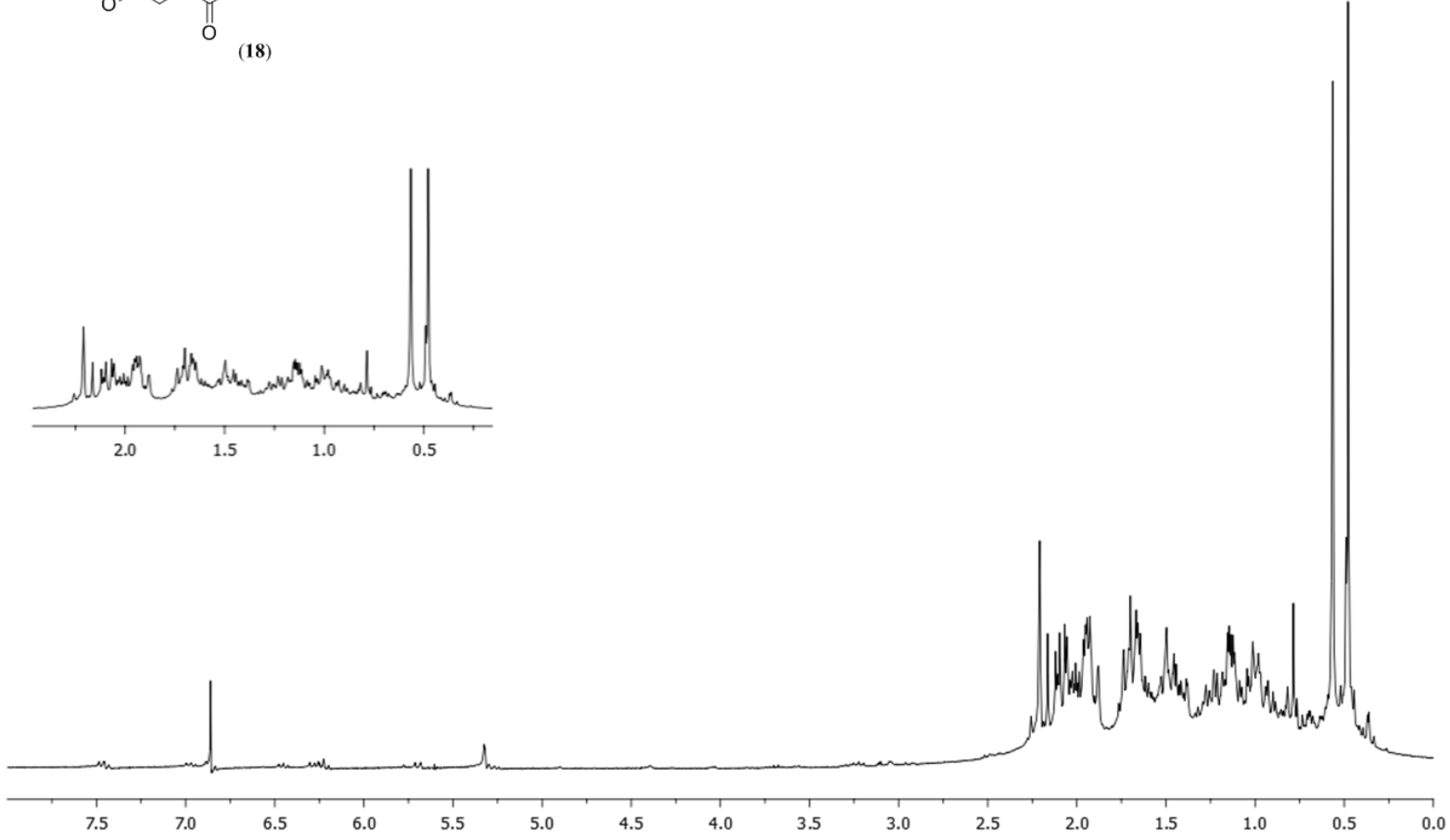
EK 20: 5 \alpha -Androstan-3,6,17-trion (18) için ^1\text{H} NMR spektrumu
