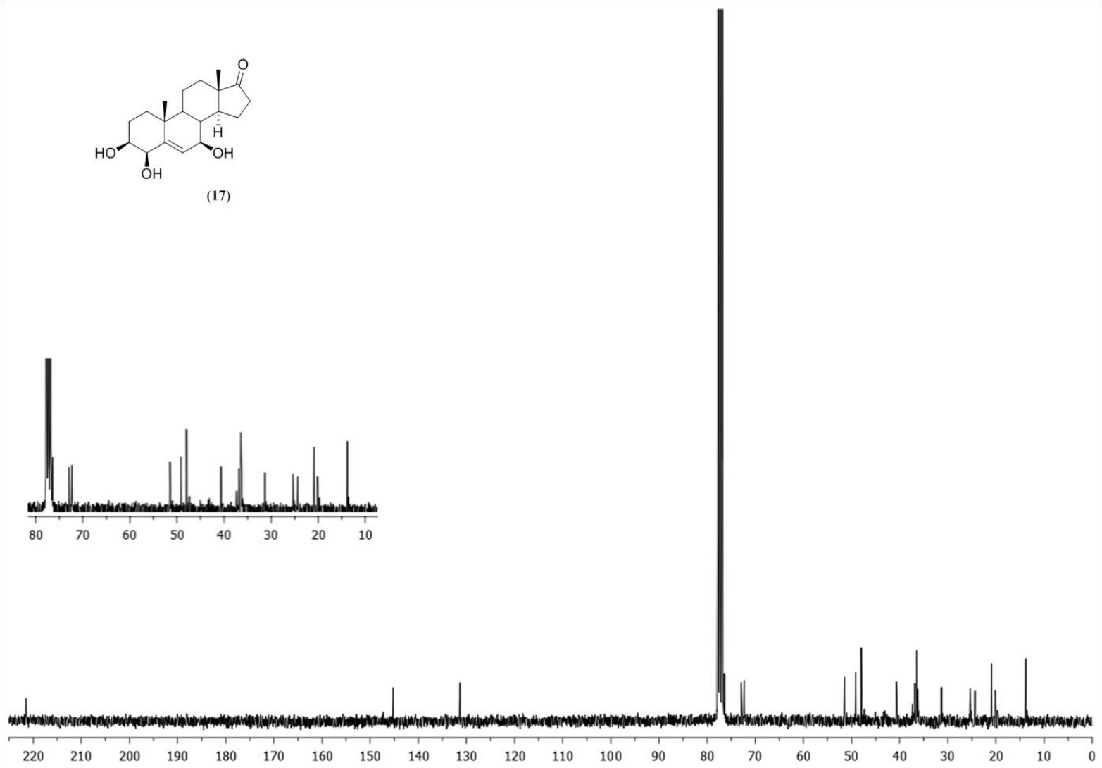
EK 18: 3 \beta ,4 \beta ,7 \beta -Trihidroksiandrosteron-5-en-17-on ( 17 ) için ^{13}\text{C} NMR spektrumu
