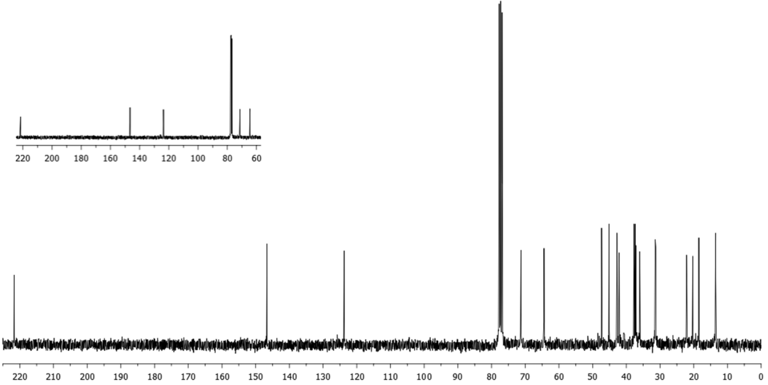
EK 8: 3 \beta ,7 \alpha -Dihidroksiandroster-5-en-17-on (13) için ^{13}\text{C} NMR spektrumu
