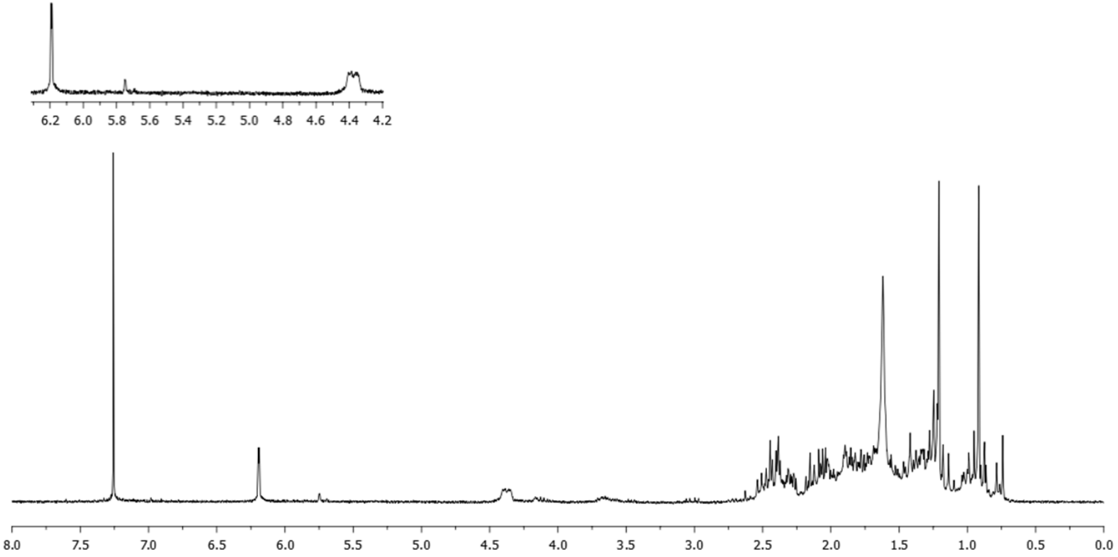
EK 24: 6 \alpha -Hidroksiandroster-4-en-3,17-dion (20) için ^1\text{H} NMR spektrumu
