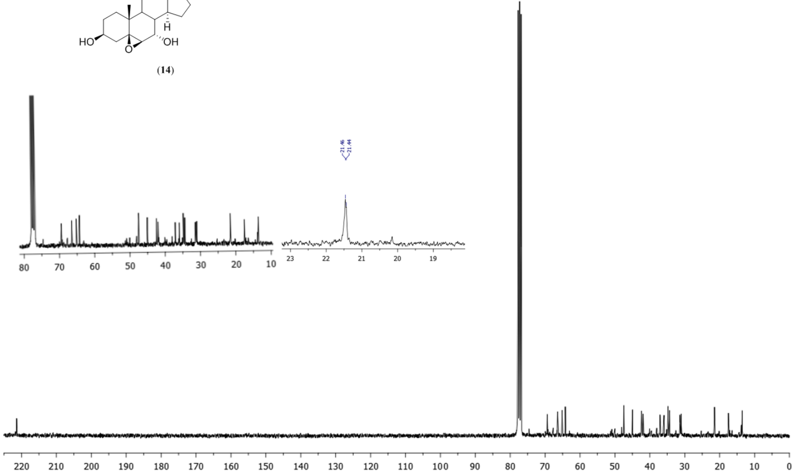
EK 10: 3 \beta ,7 \alpha -Dihidroksi-5 \beta ,6 \beta -epoksiandrostan-17-on (14) için ^{13}\text{C} NMR spektrumu
