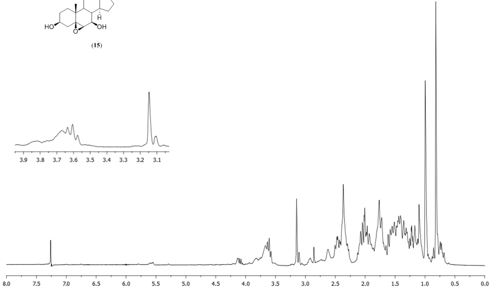
EK 11: 3 \beta ,7 \beta -dihidroksi-5 \beta ,6 \beta -epoksiandrostan-17-on (15) için ^1\text{H} NMR spektrumu
