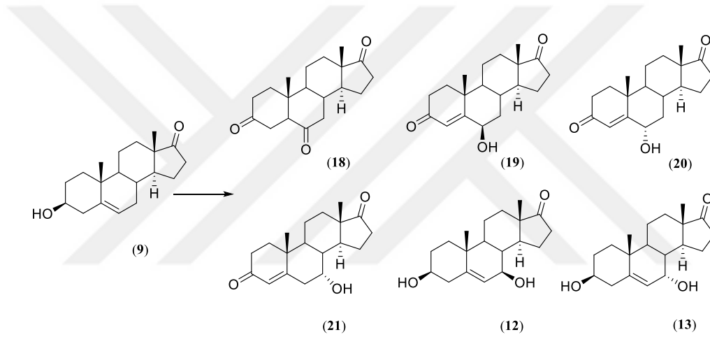
Şekil 5.2. Substratın C. sphaerospermum ile biyotransformasyonu.
