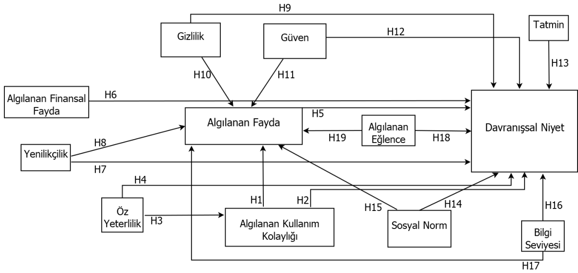
Şekil 6 Araştırmanın Modeli
