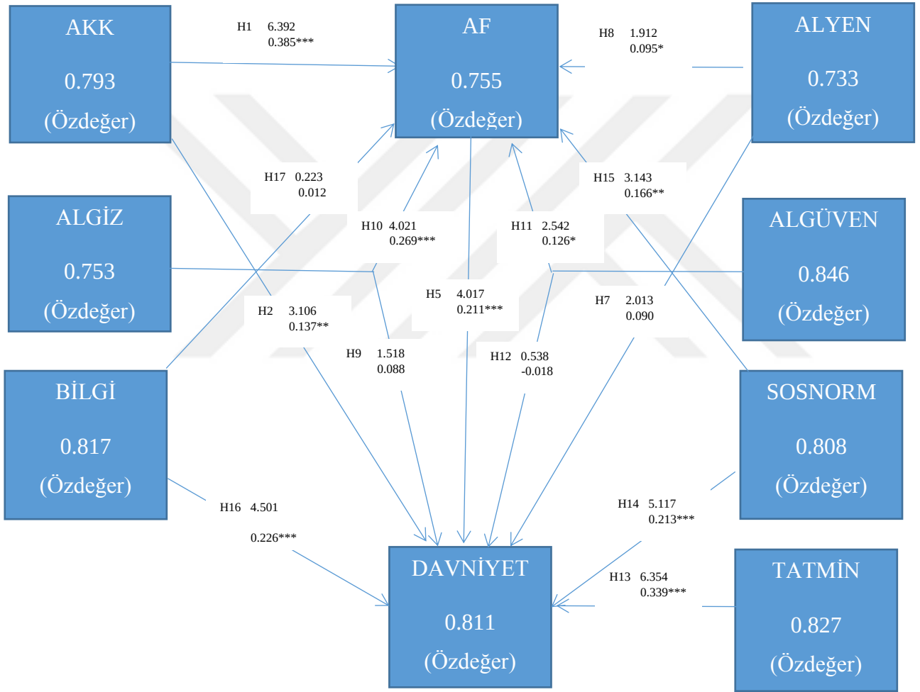
Şekil 9 Yapısal Model
