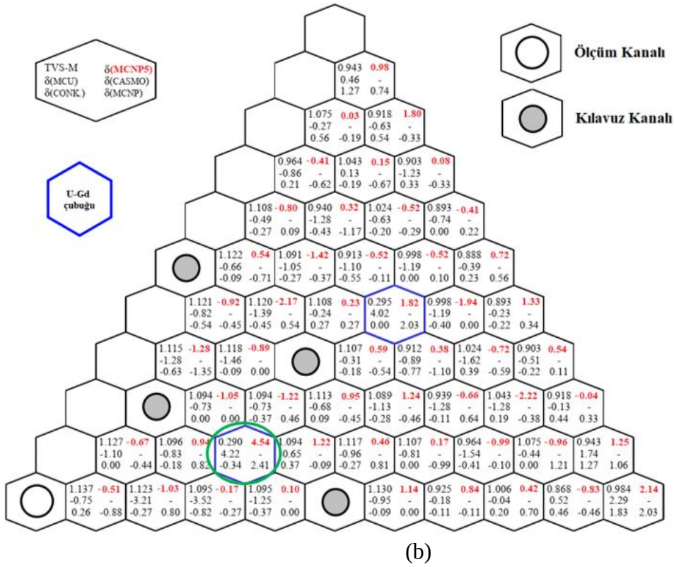
Şekil 5.5. Yakıt demeti 4 için bağıl güç yoğunluk değeri ve diğer kodlar ile sapma yüzdelerinin karşılaştırılması
