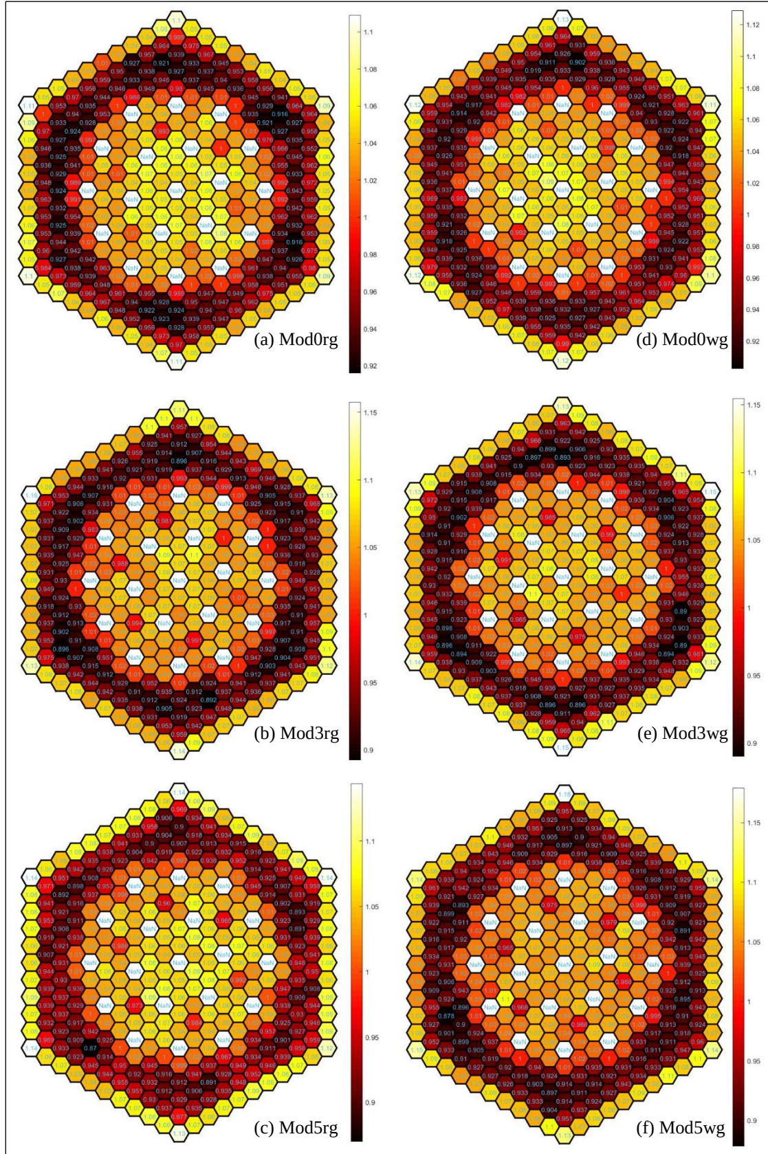
Şekil 6.9. Homojen bir şekilde dağılmış ( \text{PuO}_2 + \text{ThO}_2 ) yakıt bileşimlerinin D12 işletme koşullarında bağlı güç yoğunluğu dağılımı
