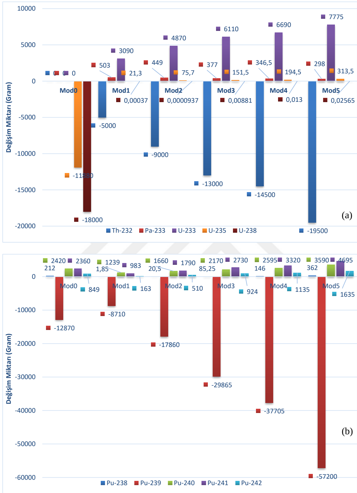
Şekil 6.15. Homojen bir şekilde dağılmış ( wgPuO_2+ThO_2 ) yakıt bileşimi için D12 işletme koşullarında Th-232, Pa-233, U-233, U-235, U-238 ve Plütonyum izotopların değişimleri
