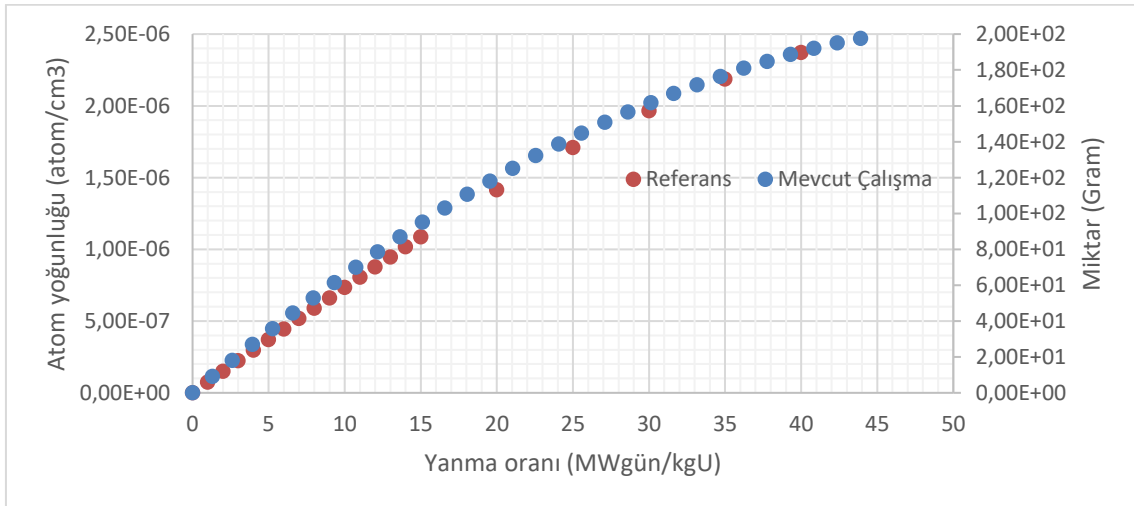
Şekil 5.17. YD4 düzeninde U-236 miktarı ile yanma oranı arasındaki ilişki
