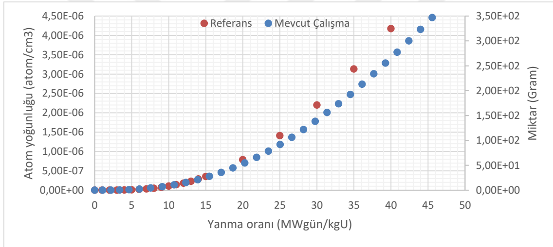
Şekil 5.13. YD3 düzeninde Pu-242 miktarı ile yanma oranı arasındaki ilişki
