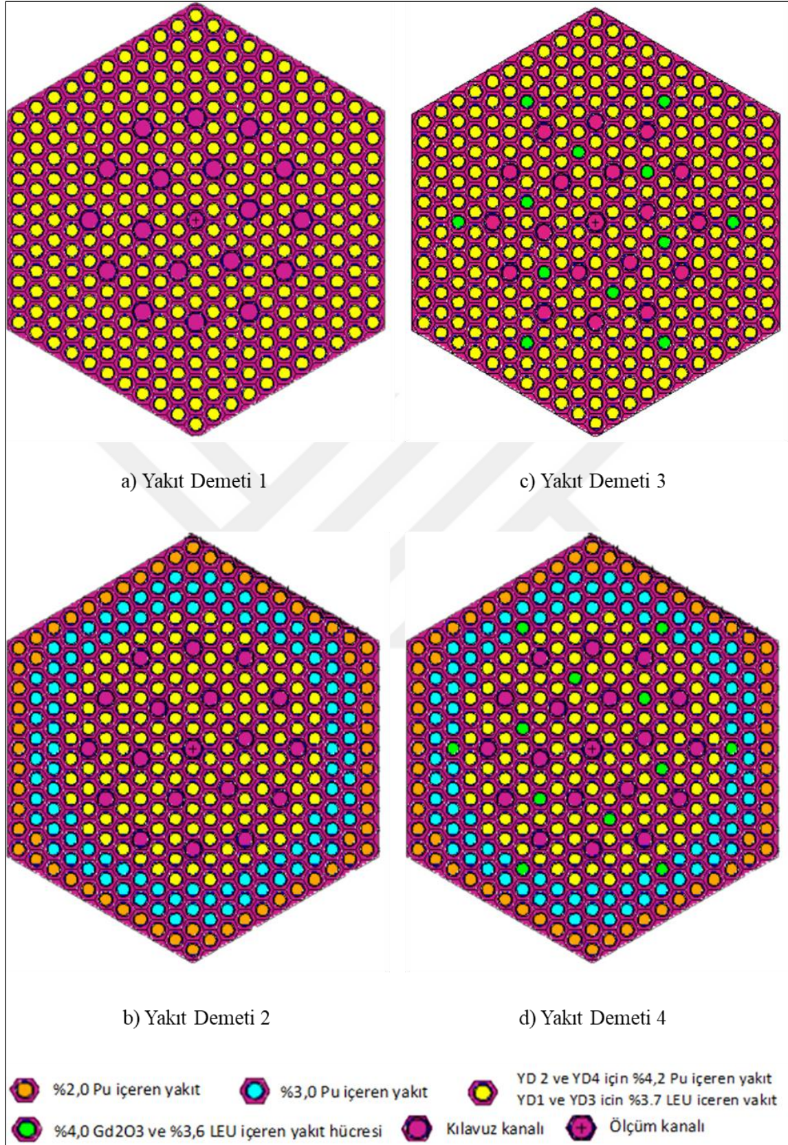
Şekil 5.1. YD1 (Homojen %3,7 LEU), YD2 (%2, %3, %4,2 Pu), YD3 (Homojen %3,7 LEU ve %3,6 LEU ile %4 Gd 2 O 3 ) ve YD4 (%2, %3, %4,2 Pu ve %3,6 LEU ile %4 Gd 2 O 3 ) yakıt demeti düzenleri
