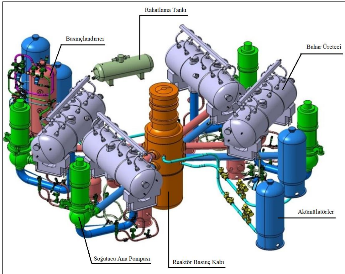
Şekil 2.6. VVER-1200 birincil döngü ve ana bileşenleri [16]
