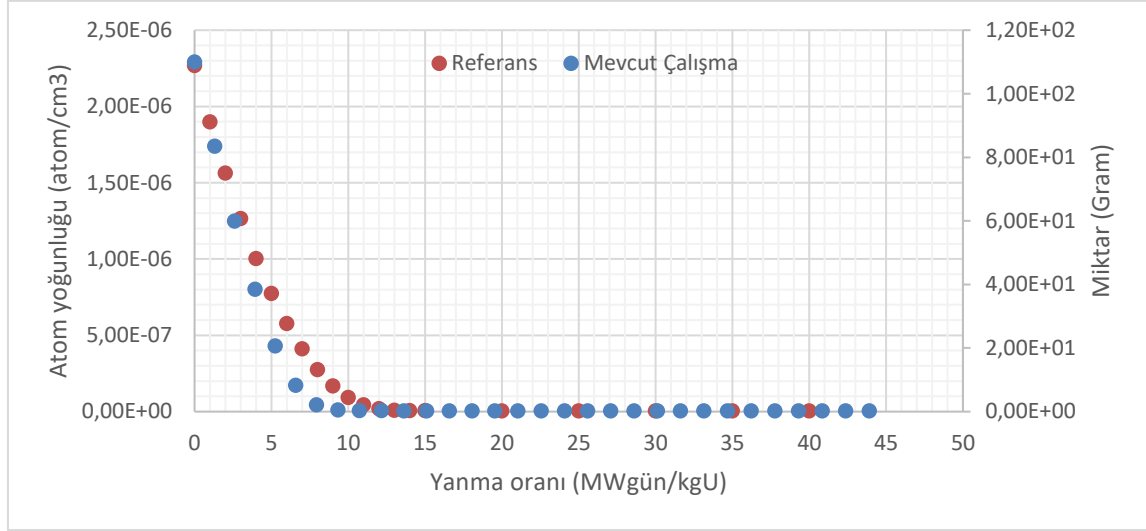
Şekil 5.24. YD4 yakıt düzeninde Gd-157 miktarı ile yanma oranı arasındaki ilişki
