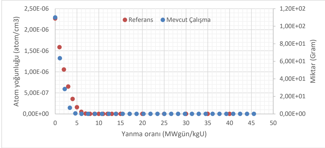
Şekil 5.15. YD3 düzeninde Gd-157 miktarı ile yanma oranı arasındaki ilişki
