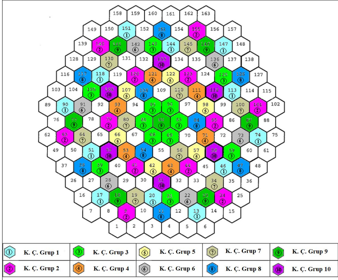
Şekil 2.5. Kontrol çubuğu kümelerinin VVER-1000 koru içerisinde konumları [22]
