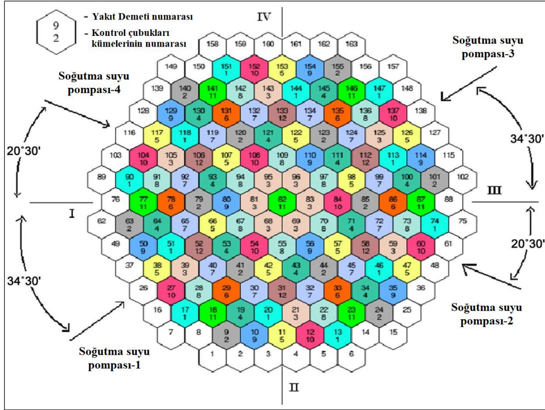
Şekil 2.8. VVER-1200 reaktör korunda kontrol çubukları kümesinin yerleşimi [25]
