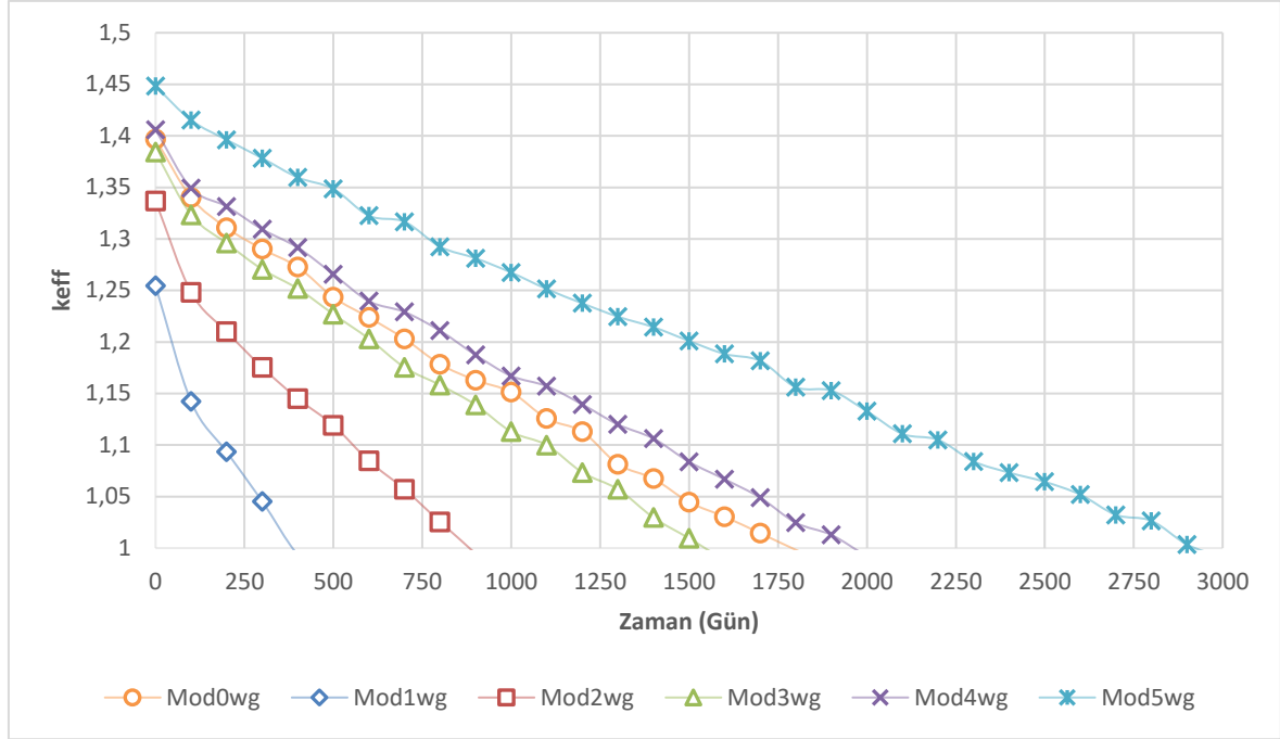
Şekil 6.5. Homojen dağılımlı ( wgPuO_2+ThO_2 ) yakıt bileşiminin D12 işletme koşullarında zamana bağlı olarak etkin çoğaltma faktörünün değişimi
