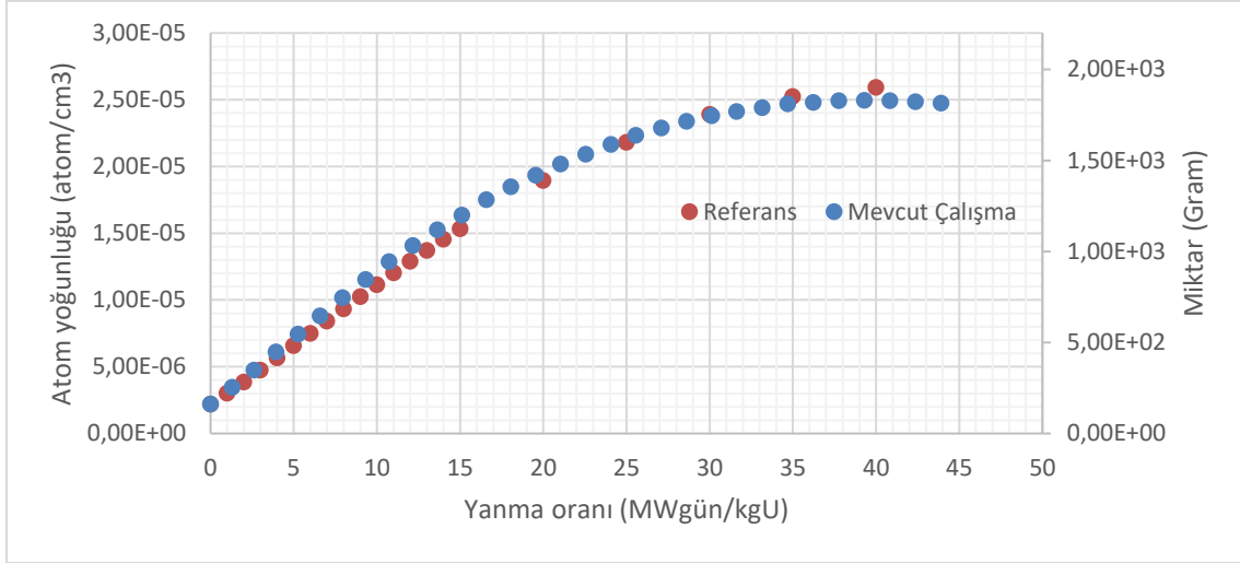
Şekil 5.21. YD4 düzeninde Pu-241 miktarı ile yanma oranı arasındaki ilişki
