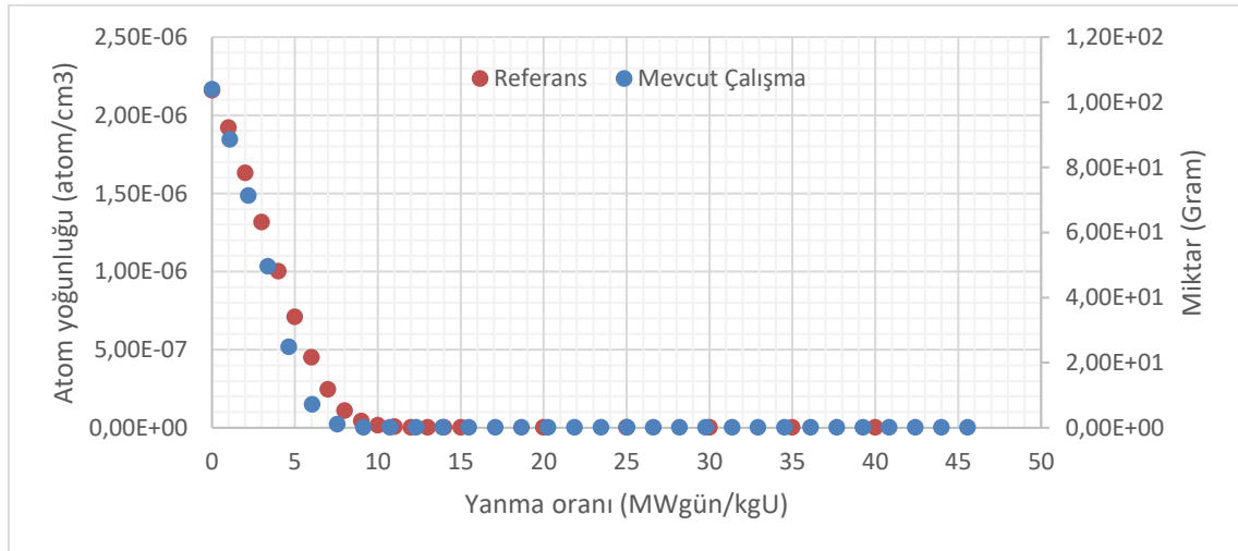
Şekil 5.14. YD3 düzeninde Gd-155 miktarı ile yanma oranı arasındaki ilişki
