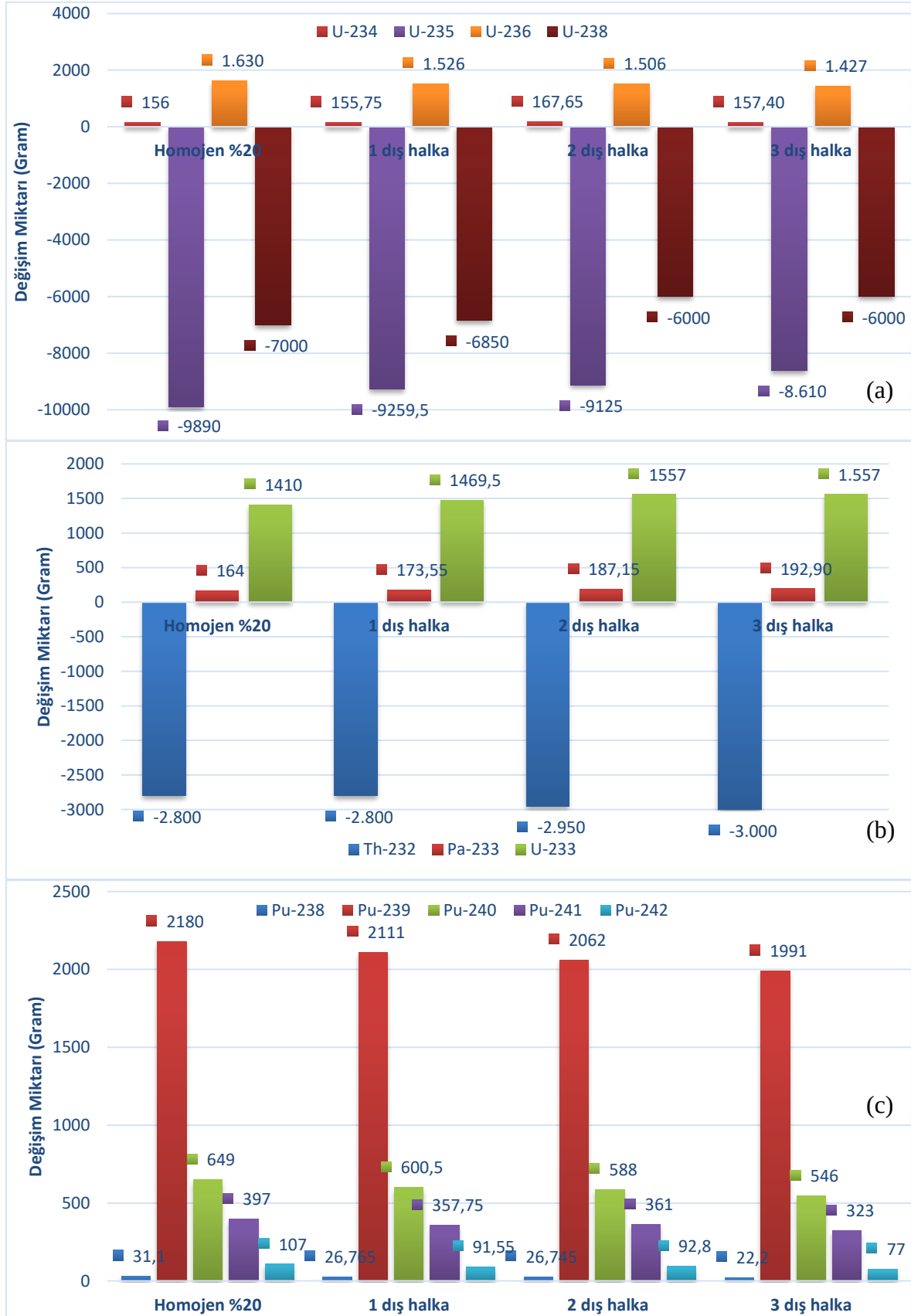
Şekil 6.13. Heterojen dizilime sahip ( \text{UO}_2 + \text{ThO}_2 ) yakıt bileşimleri için D12 işletme koşullarında Uranyum izotopları, Th-232, Pa-233, U-233 ve Pu izotoplarının değişimleri
