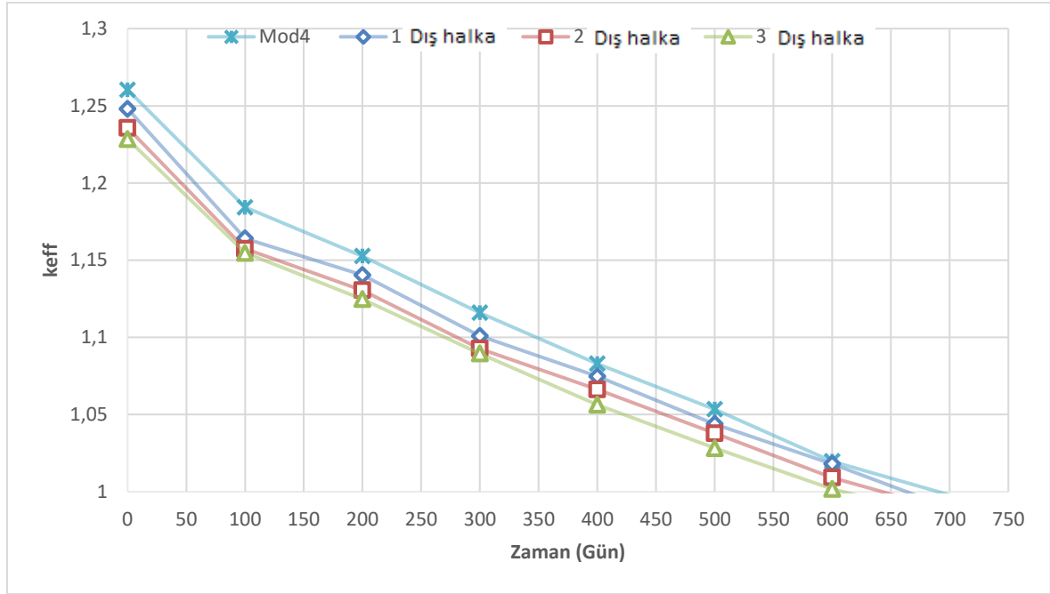
Şekil 6.3. Heterojen dizilime sahip ( UO_2+ThO_2 ) yakıt bileşiminin D12 işletme koşullarında zamana bağlı olarak etkin çoğaltma faktörünün değişimi
