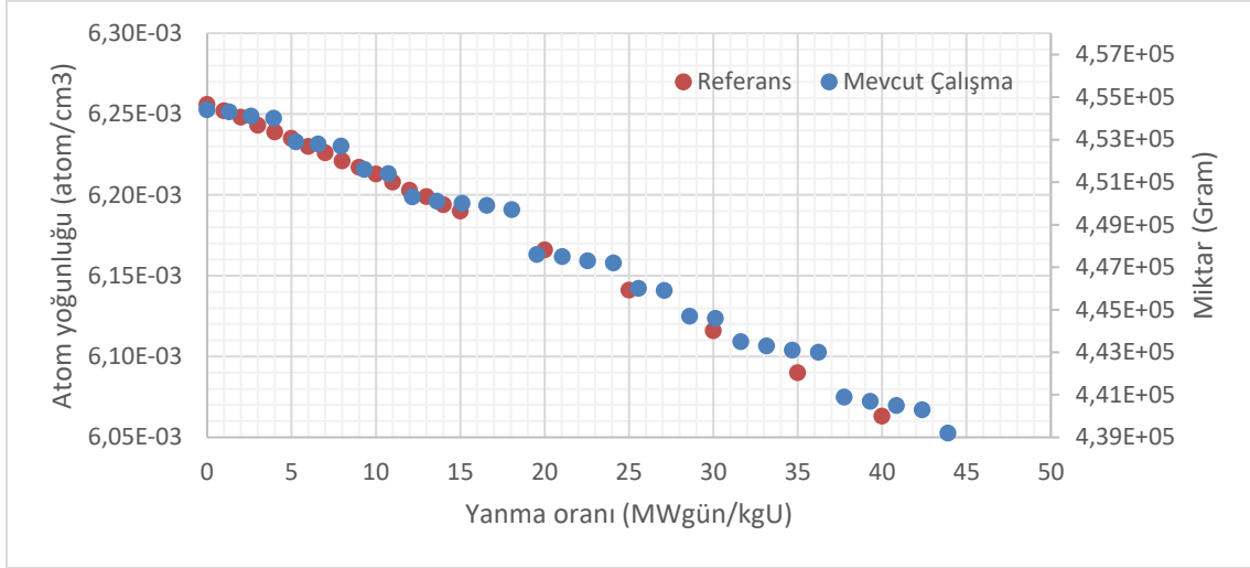
Şekil 5.18. YD4 düzeninde U-238 miktarı ile yanma oranı arasındaki ilişki
