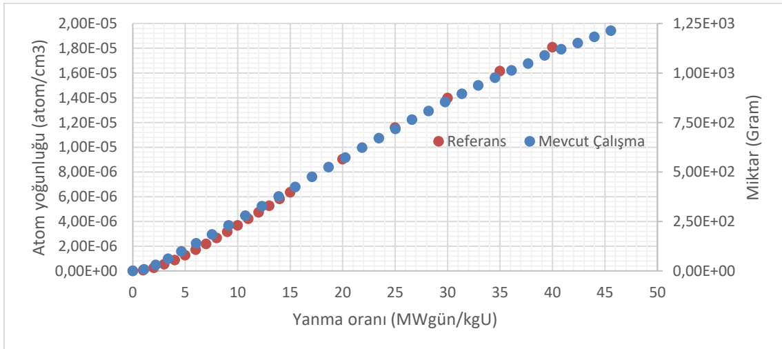
Şekil 5.11. YD3 düzeninde Pu-240 miktarı ile yanma oranı arasındaki ilişki
