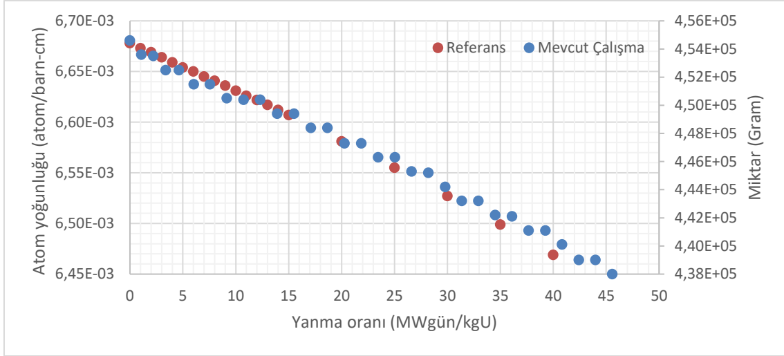
Şekil 5.9. YD3 düzeninde U-238 miktarı ile yanma oranı arasındaki ilişki
