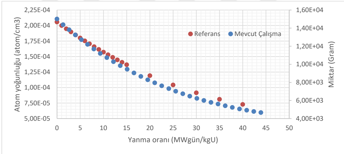
Şekil 5.19. YD4 düzeninde Pu-239 miktarı ile yanma oranı arasındaki ilişki
