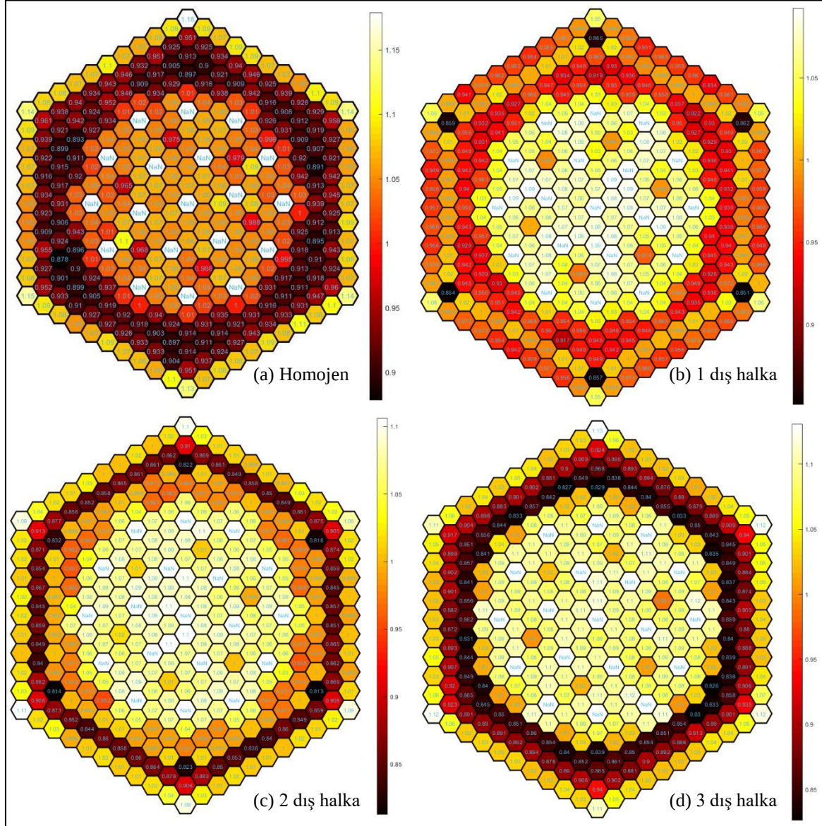
Şekil 6.11. Heterojen bir şekilde dağılmış ( wgPuO_2+ThO_2 ) yakıt bileşiminin D12 işletme koşullarında bağıl güç yoğunluğu dağılımı
