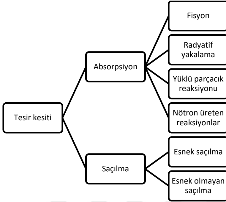
Şekil 4.2. Nötronun madde ile etkileşimi ve nötron tesir kesiti [15]
