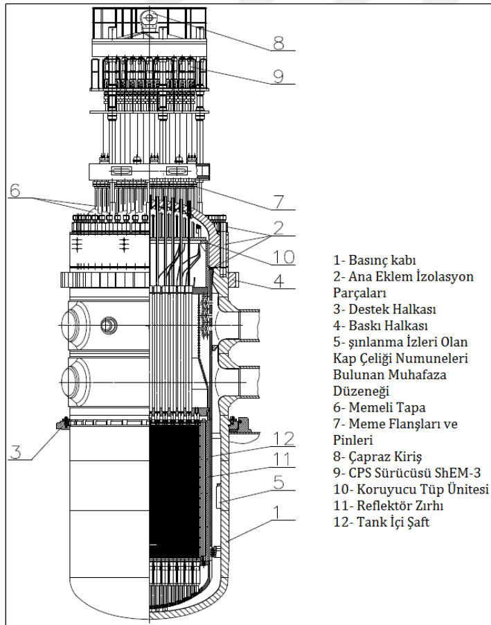
Şekil 2.2. Reaktör basınç kabının genel bir görünümü [17]
