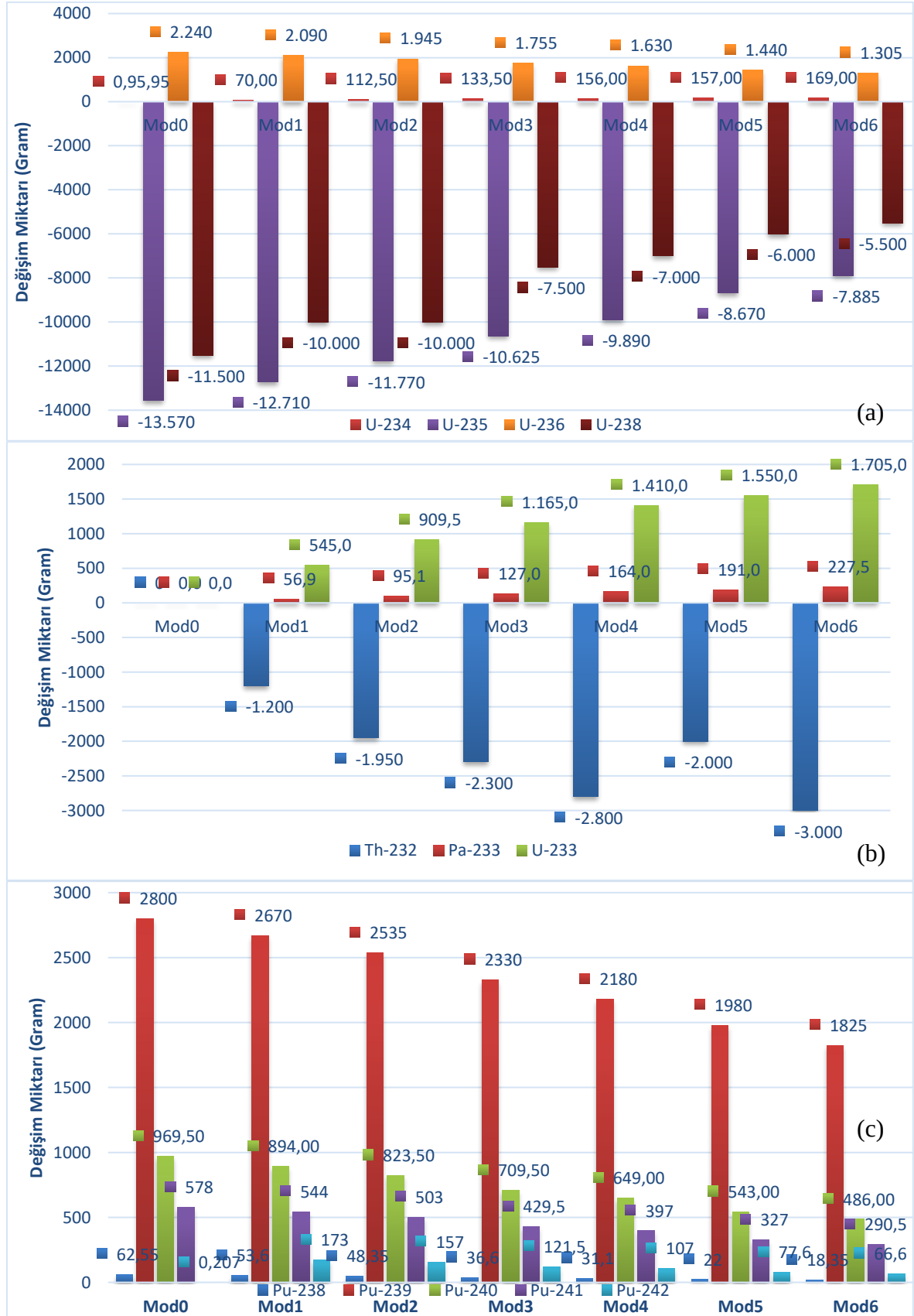
Şekil 6.12. Homojen bir şekilde dağılmış ( \text{UO}_2 + \text{ThO}_2 ) yakıt bileşimi için D12 işletme koşullarında Uranyum izotopları, Th-232, Pa-233, U-233 ve Pu izotoplarının değişimleri
