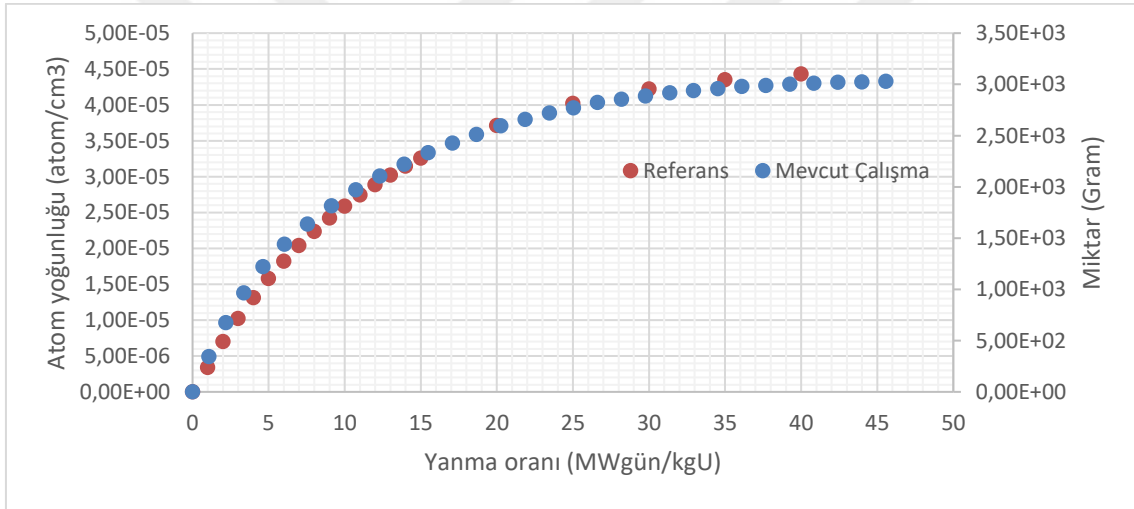
Şekil 5.10. YD3 düzeninde Pu-239 miktarı ile yanma oranı arasındaki ilişki
