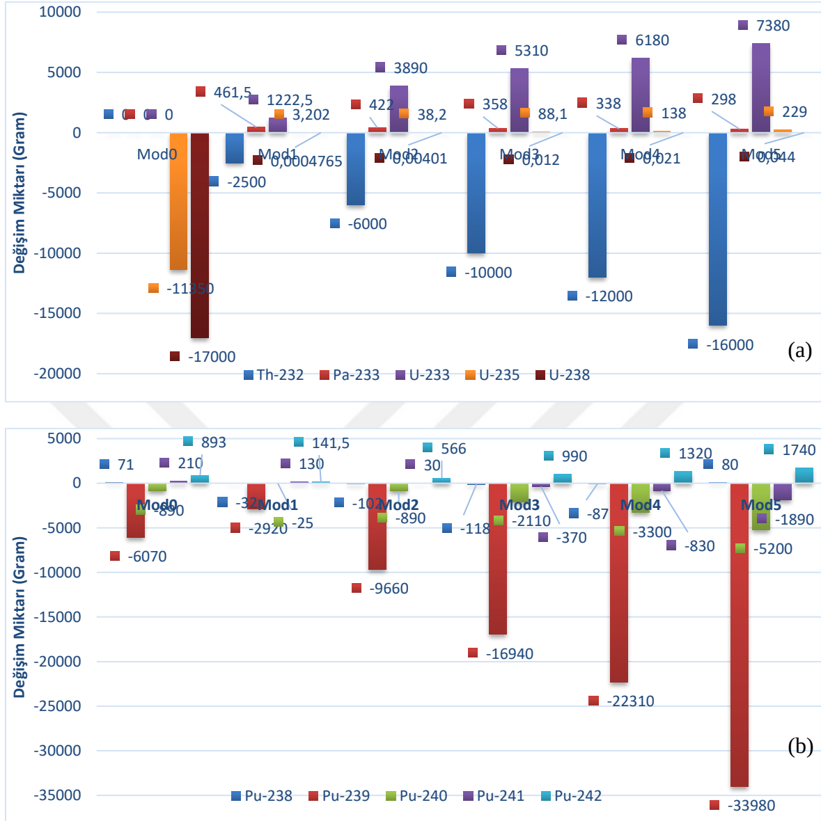
Şekil 6.14. Homojen bir şekilde dağılmış (rgPuO 2 +ThO 2 ) yakıt bileşimi için D12 işletme koşullarında Th-232, Pa-233, U-233, U-235, U-238 ve Plütonyum izotopların değişimleri
