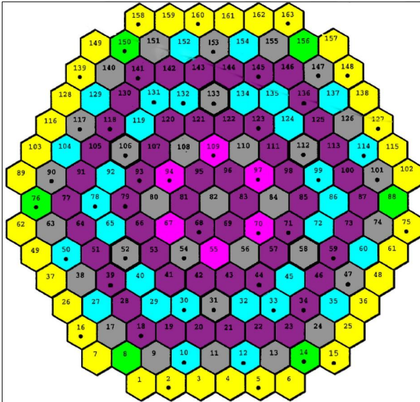
Şekil 2.3. VVER kuru yakıt düzeni [19]
