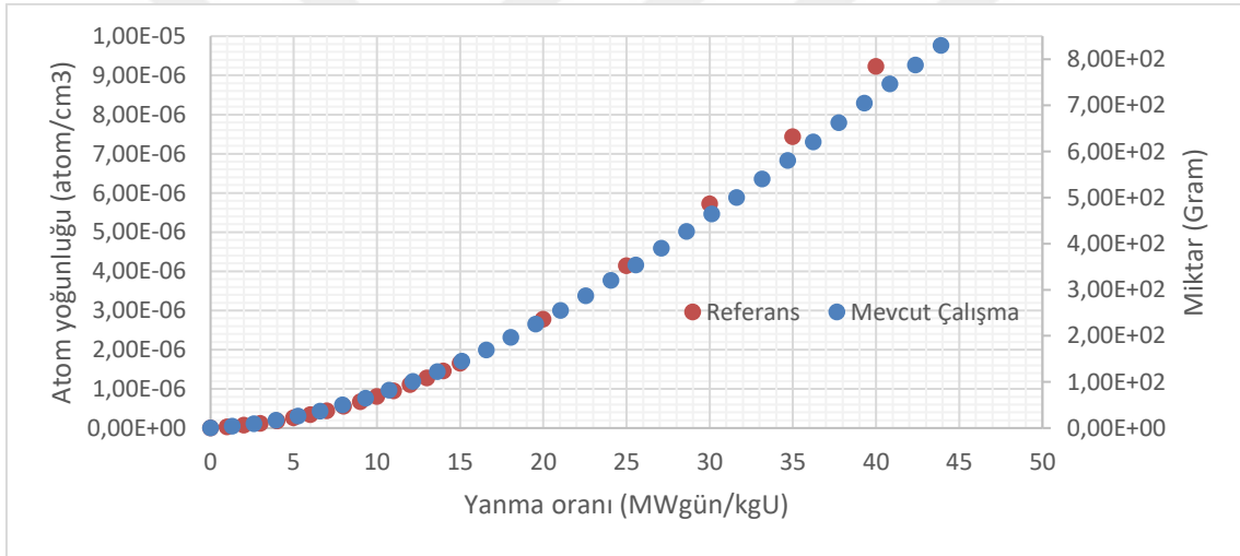
Şekil 5.22. YD4 düzeninde Pu-242 miktarı ile yanma oranı arasındaki ilişki
