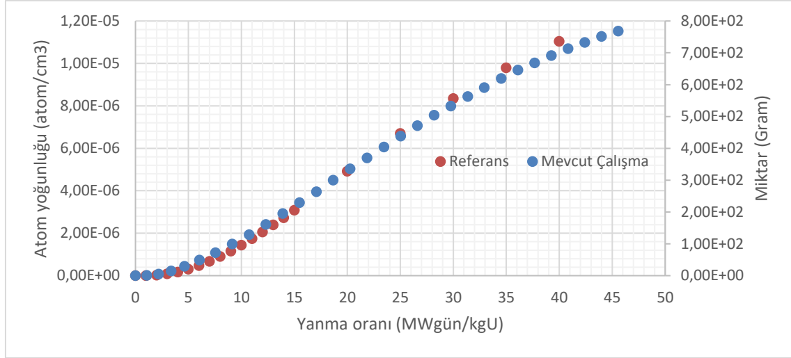
Şekil 5.12. YD3 düzeninde Pu-241 miktarı ile yanma oranı arasındaki ilişki
