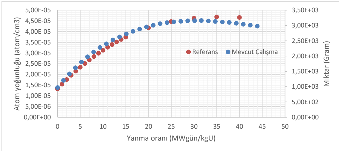
Şekil 5.20. YD4 düzeninde Pu-240 miktarı ile yanma oranı arasındaki ilişki
