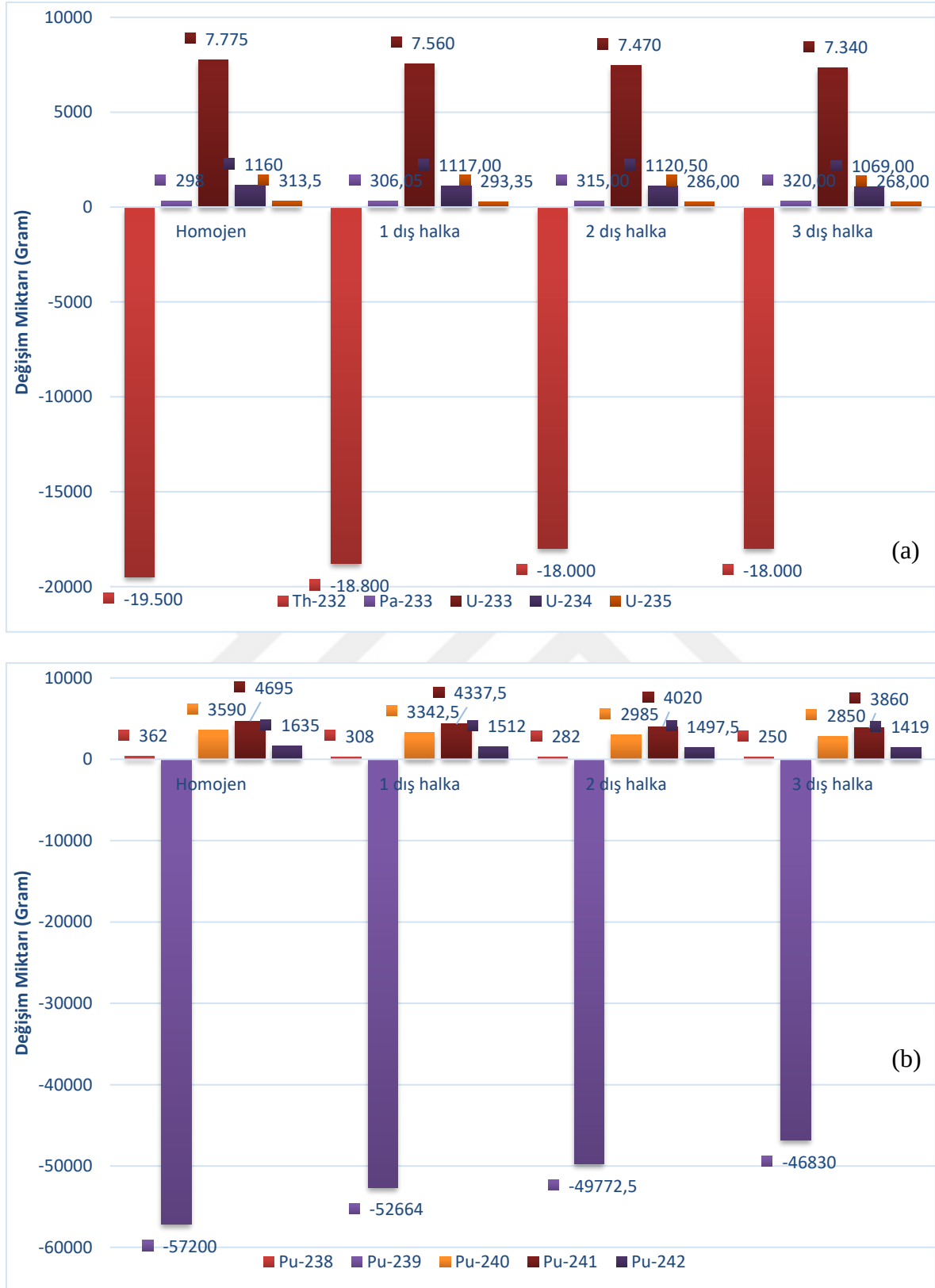
Şekil 6.17. Heterojen bir dizilime sahip ( w_{\text{PuO}_2} + \text{ThO}_2 ) yakıt bileşimi için D12 işletme koşullarında Th-232, Pa-233, U-233, U-235, U-238 ve Plütonyum izotopların değişimleri
