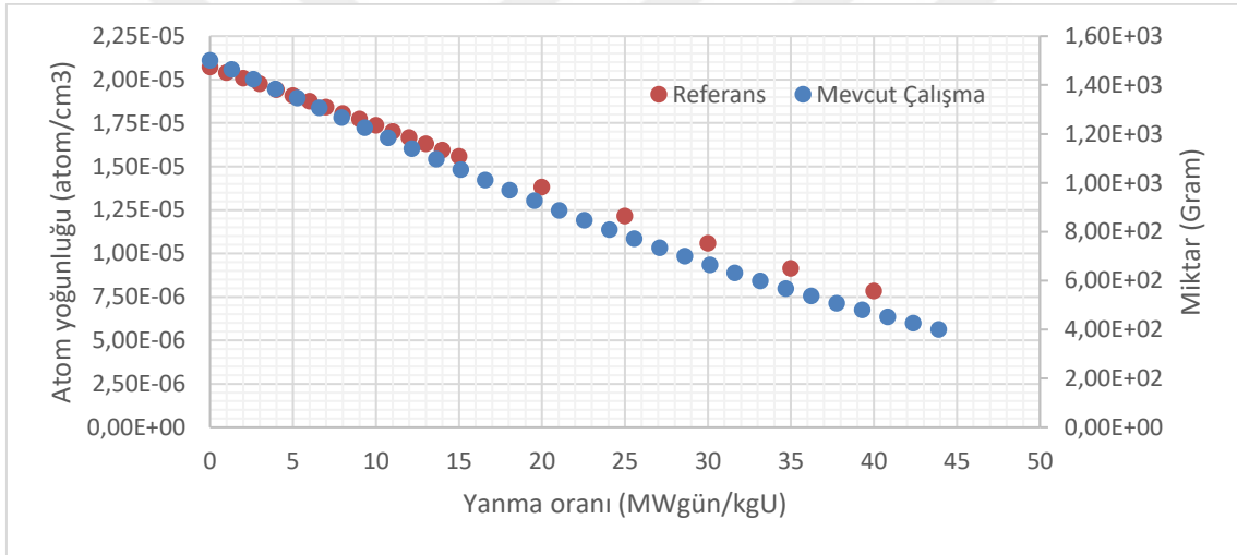
Şekil 5.16. YD4 düzeninde U-235 miktarı ile yanma oranı arasındaki ilişki
