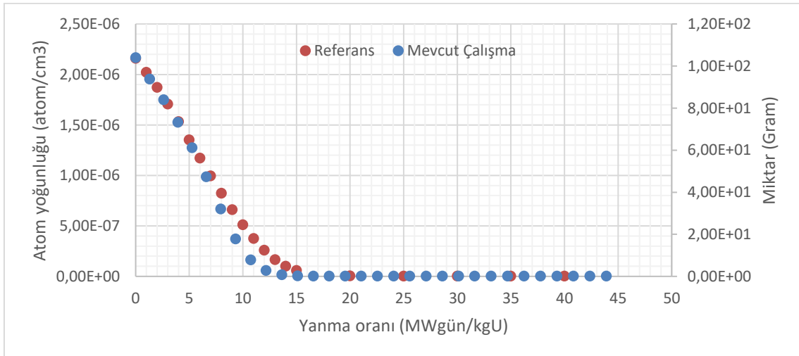
Şekil 5.23. YD4 düzeninde Gd-155 miktarı ile yanma oranı arasındaki ilişki
