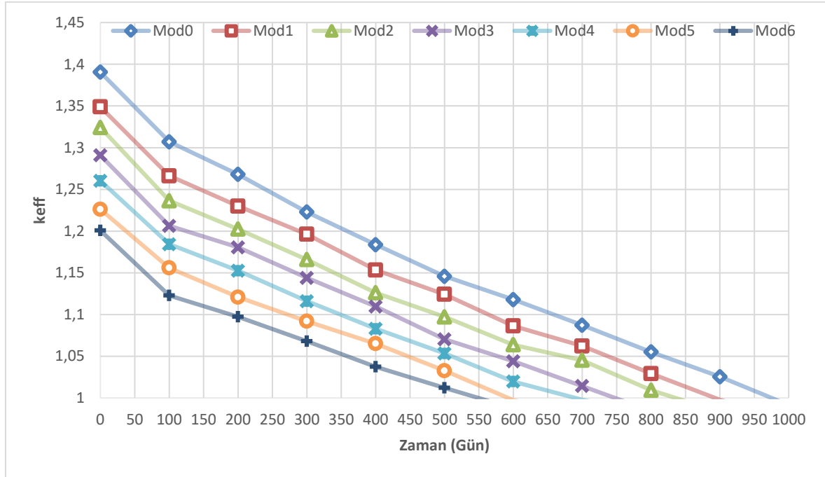
Şekil 6.2. Homojen bir şekilde dağılmış ( \text{UO}_2 + \text{ThO}_2 ) yakıt bileşimlerinin D12 işletme koşullarında zamana bağlı olarak etkin çoğaltma faktörünün değişimi
