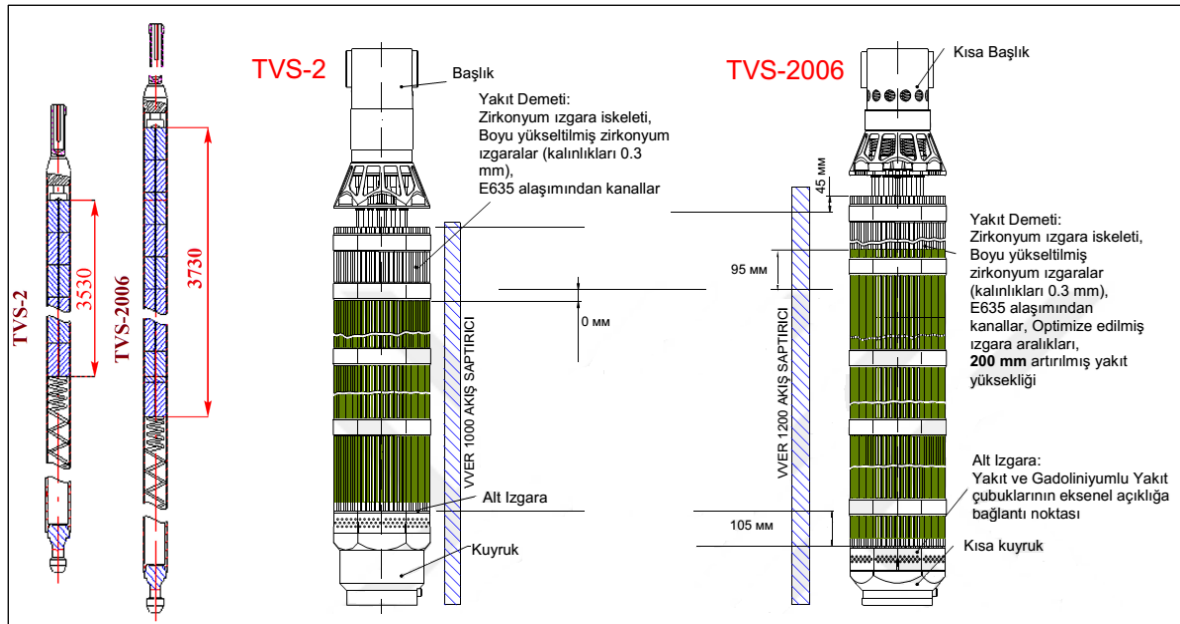
Şekil 2.7. VVER-1000'de kullanılan TVS-2 isimli ve VVER-1200'de kullanılan TVS-2006 isimli yakıt tasarımı [26, 63]
