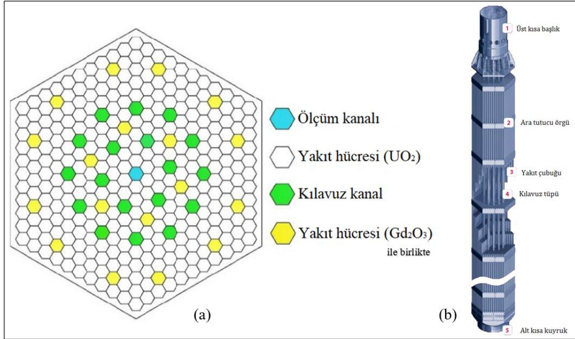
Şekil 2.4. Tipik bir VVER-1000 yakıt demeti içerisinde yakıt hücreleri ile ölçüm ve kontrol elemanlarının yerleşimi ve yakıt demetinin genel görünüşü [20]
