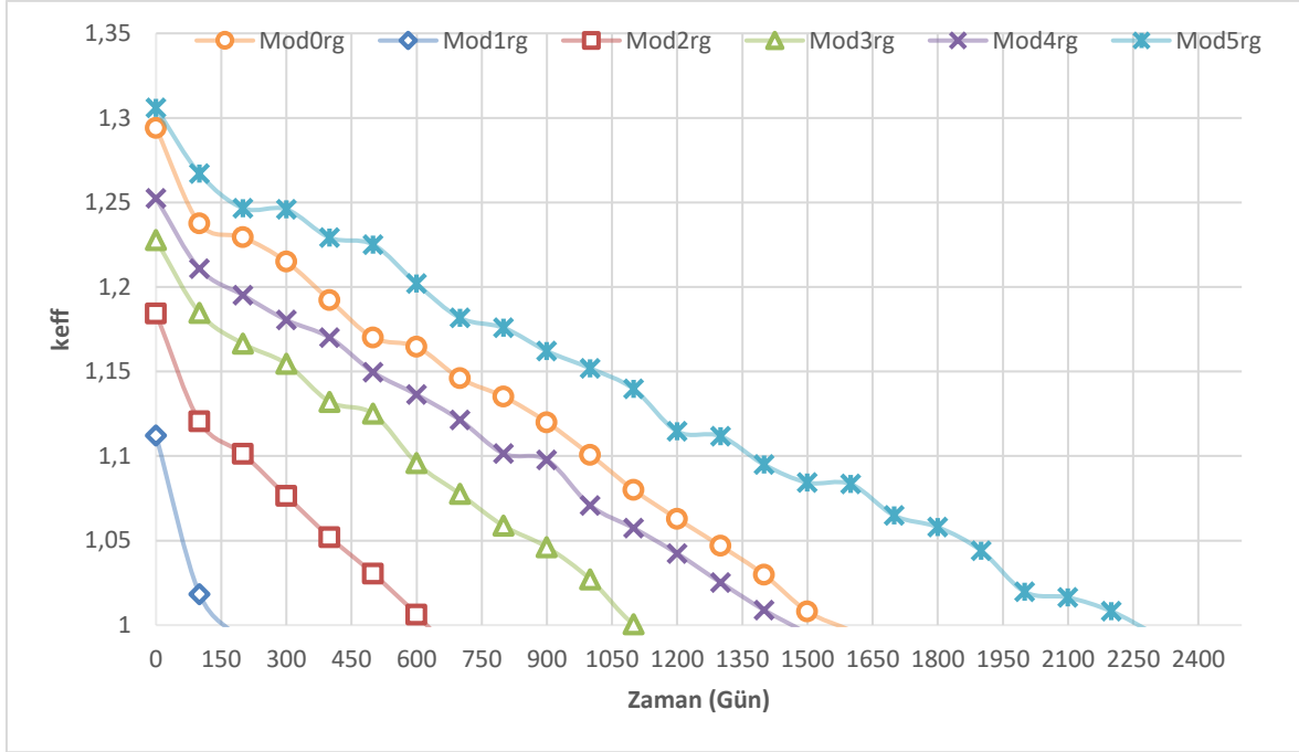
Şekil 6.4. Homojen dağılımlı (rgPuO 2 +ThO 2 ) yakıt bileşiminin D12 işletme koşullarında zamana bağlı olarak etkin çoğaltma faktörünün değişimi
