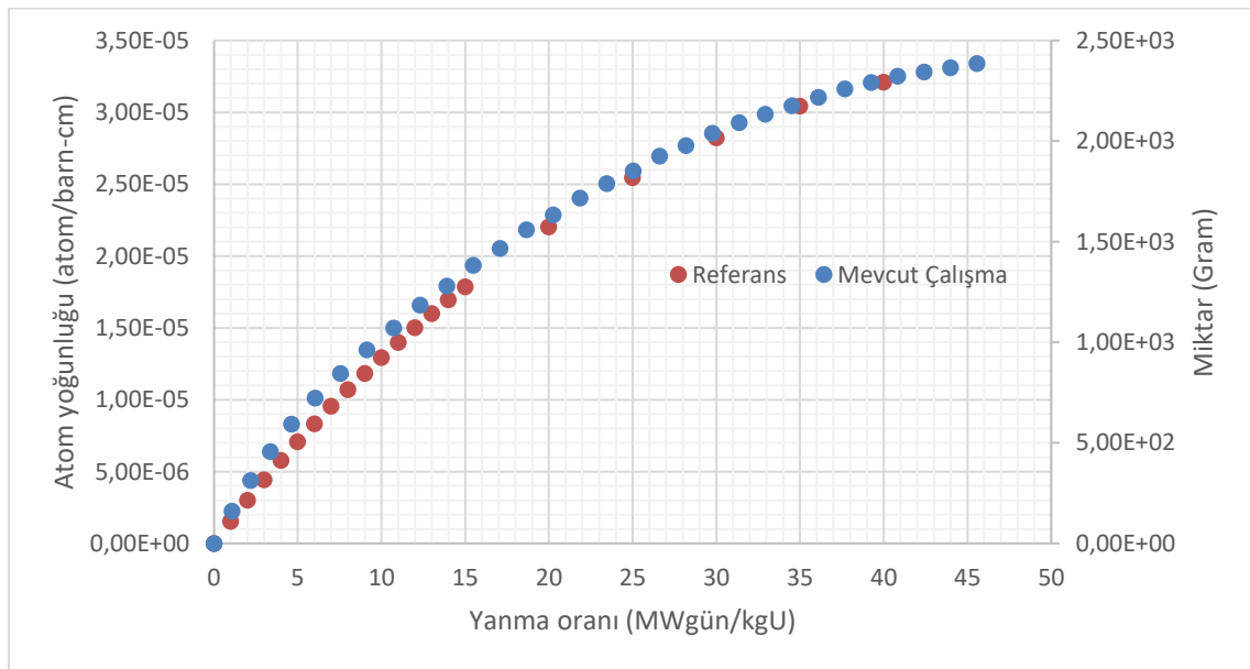
Şekil 5.8. YD3 düzeninde U-236 miktarı ile yanma oranı arasındaki ilişki
