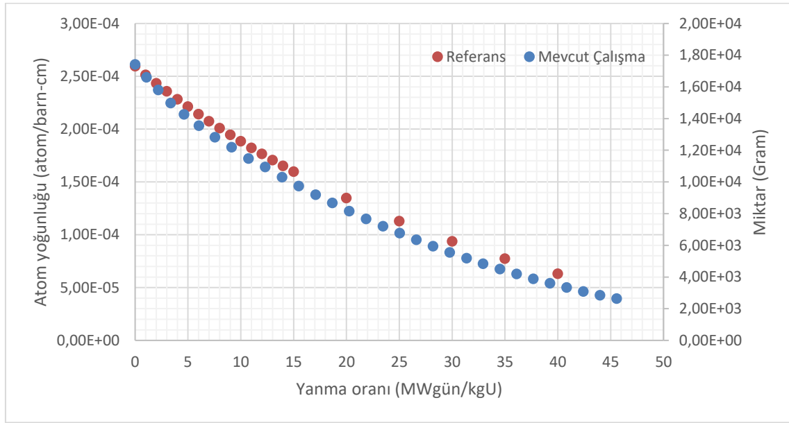
Şekil 5.7. YD3 düzeninde U-235 miktarı ile yanma oranı arasındaki ilişki
