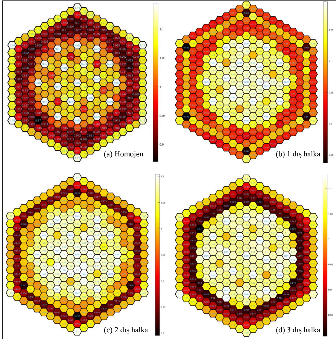
Şekil 6.10. Heterojen bir şekilde dağılmış ( rgPuO_2+ThO_2 ) yakıt bileşiminin D12 işletme koşullarında bağlı güç yoğunluğu dağılımı
