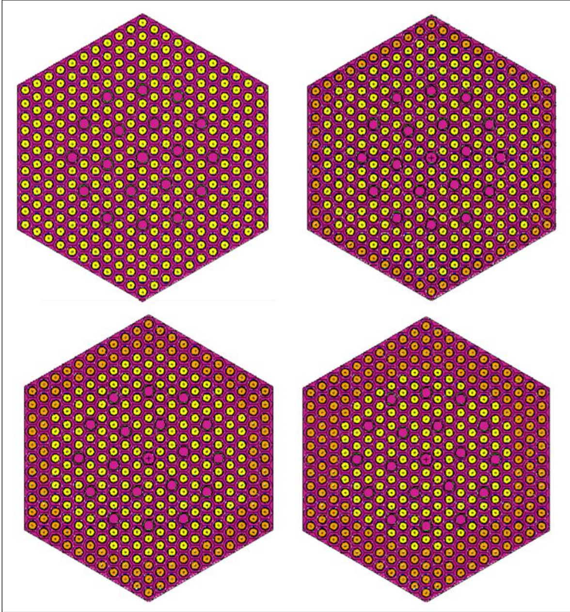
Şekil 6.1. Homojen, 1 dış halkalı heterojen, 2 halkalı heterojen ve 3 dış halkalı heterojen yakıt demeti düzeni
