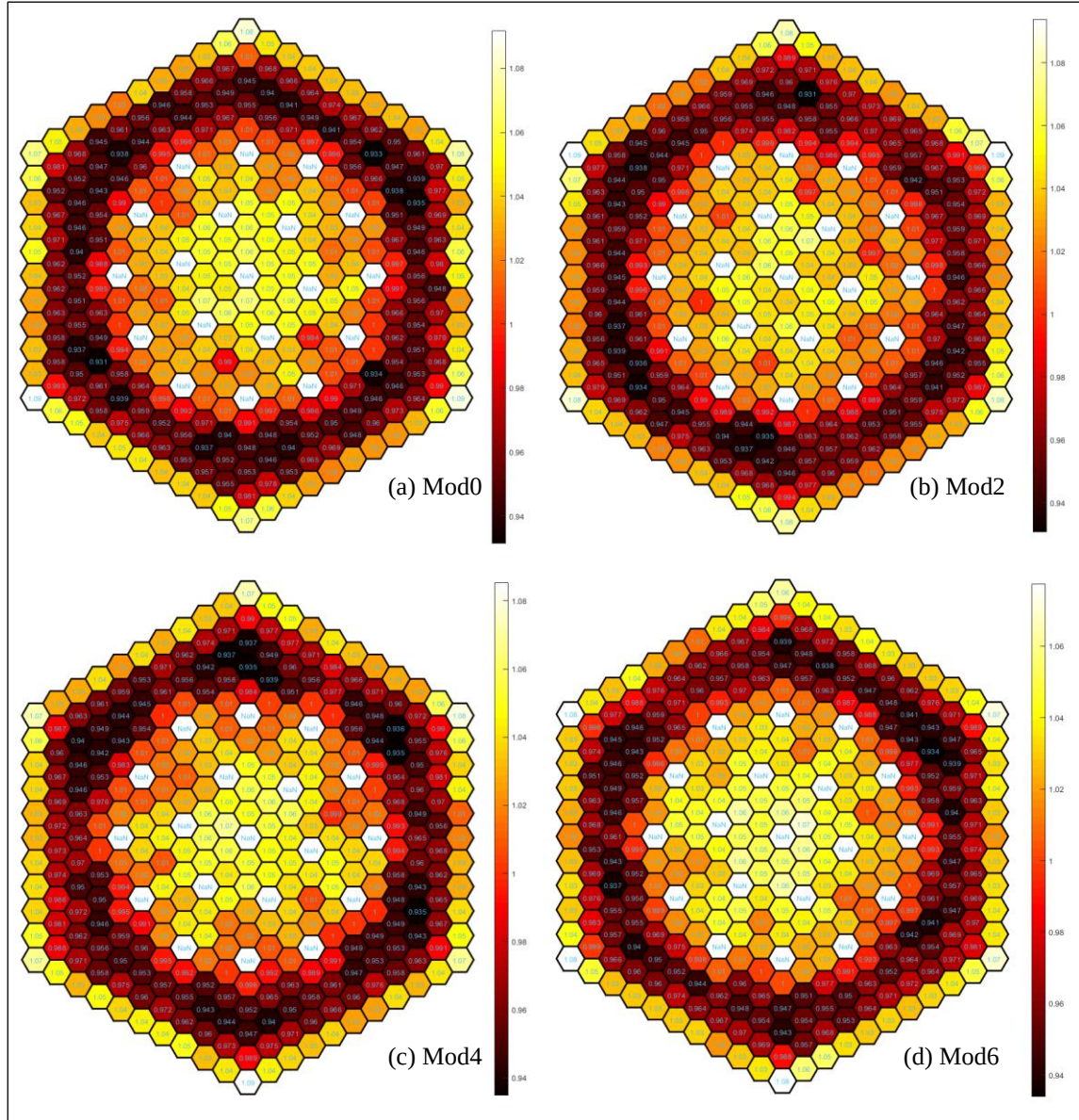
Şekil 6.7. Homojen bir şekilde dağılmış ( \text{UO}_2 + \text{ThO}_2 ) yakıt bileşimlerinin D12 işletme koşullarında bağıl güç yoğunluğu dağılımları
