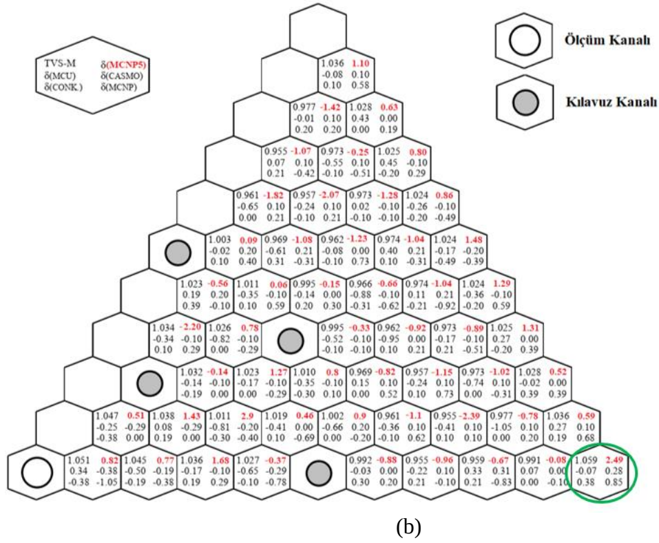
Şekil 5.2. Yakıt demeti 1 için bağıl güç yoğunluk değeri ve diğer kodlar ile sapma yüzdelerinin karşılaştırılması
