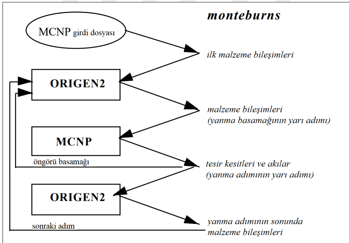
Şekil 4.3. Monteburns kodunun MCNP ve ORIGEN2 ile etkileşimi [71]
