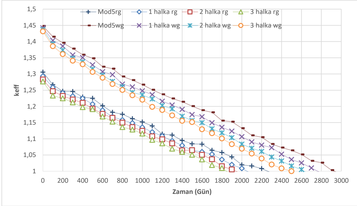
Şekil 6.6. Heterojen dizilime sahip ( rgPuO_2+ThO_2 ) ve ( wgPuO_2+ThO_2 ) yakıt bileşimlerinin D12 işletme koşullarında zamana bağlı olarak etkin çoğaltma faktörünün değişimi
