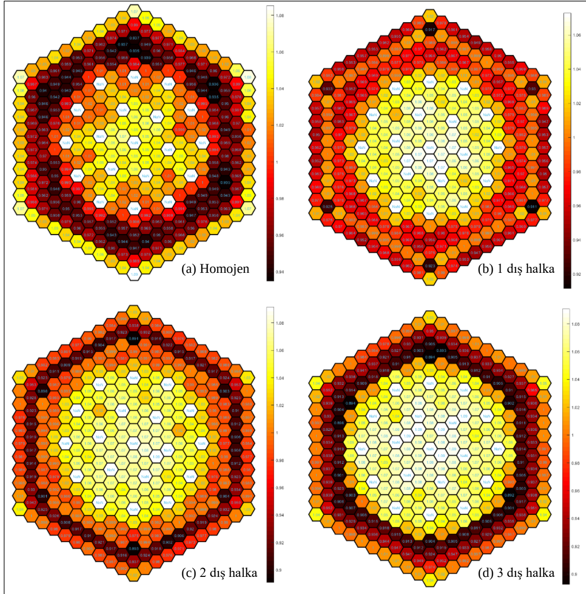
Şekil 6.8. Heterojen bir şekilde dağılmış ( \text{UO}_2 + \text{ThO}_2 ) yakıt bileşimlerinin D12 işletme koşullarında bağlı güç yoğunluğu dağılımı
