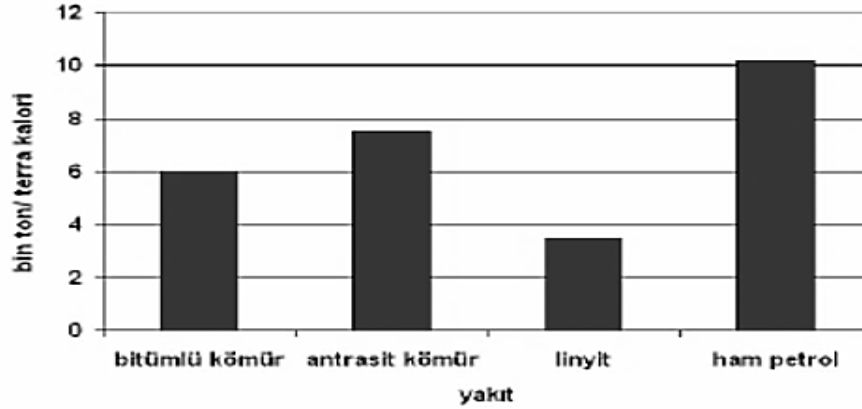
Şekil 7: Yakıtların Enerji İçeriklerinin Karşılaştırılması (Ağırlık Olarak)
