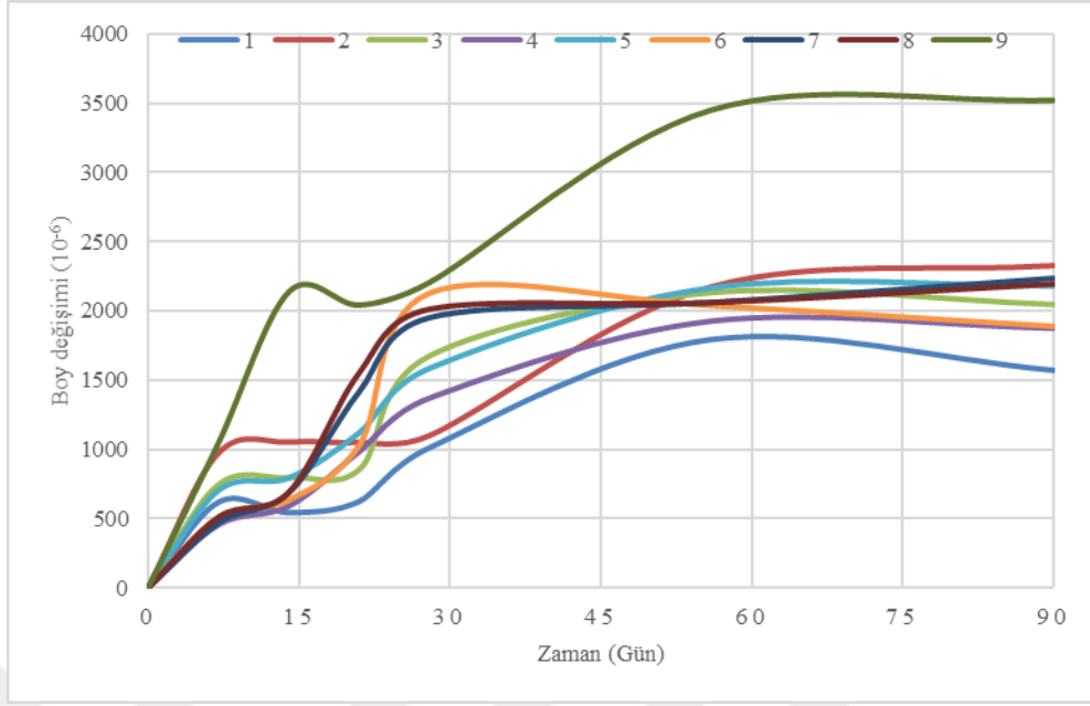
Şekil 4.15 6 mm uzunluğundaki liflerden üretilen karışımların kuruma büzülmesi özellikleri
