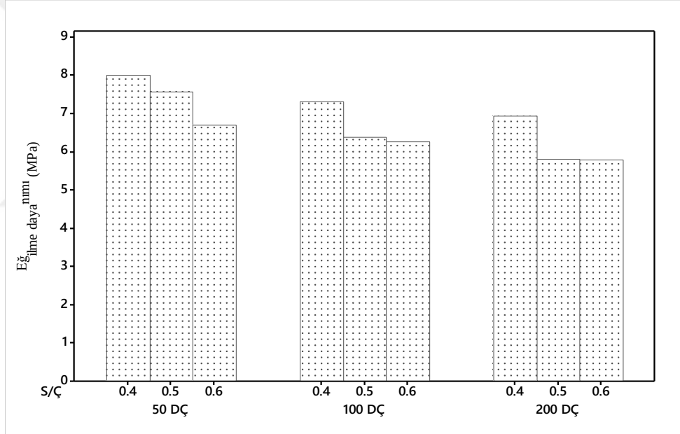
Şekil 4.20 S/Ç etkisinin donma-çözülme sonrasındaki eğilme dayanımına etkisi
