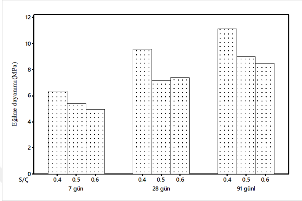
Şekil 4.9 S/Ç oranının eğilme dayanımına etkisi
