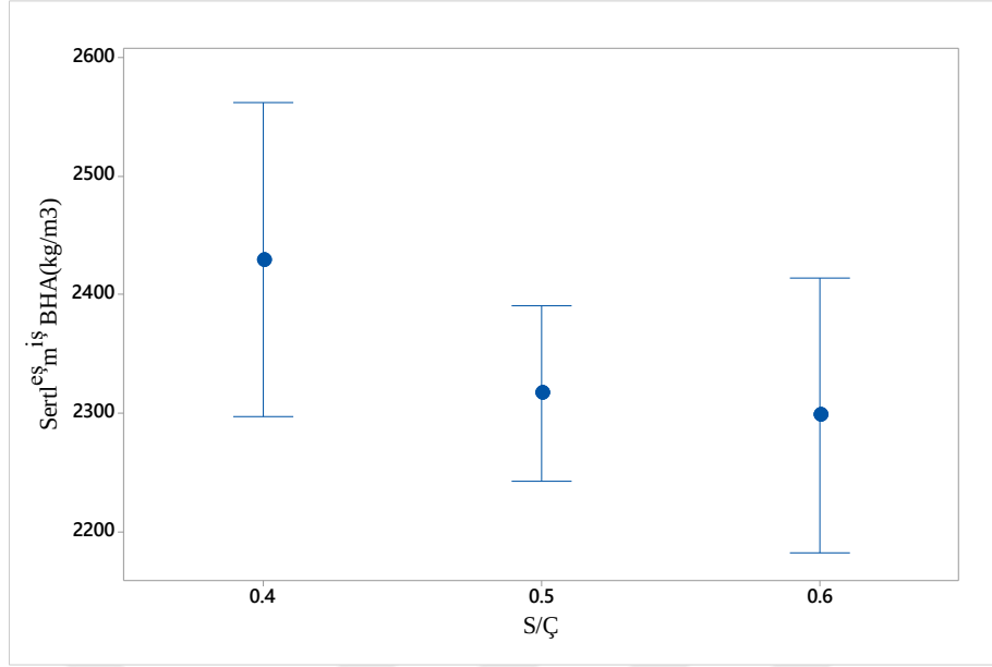
Şekil 4.7 S/Ç oranının BHA üzerindeki etkisi
