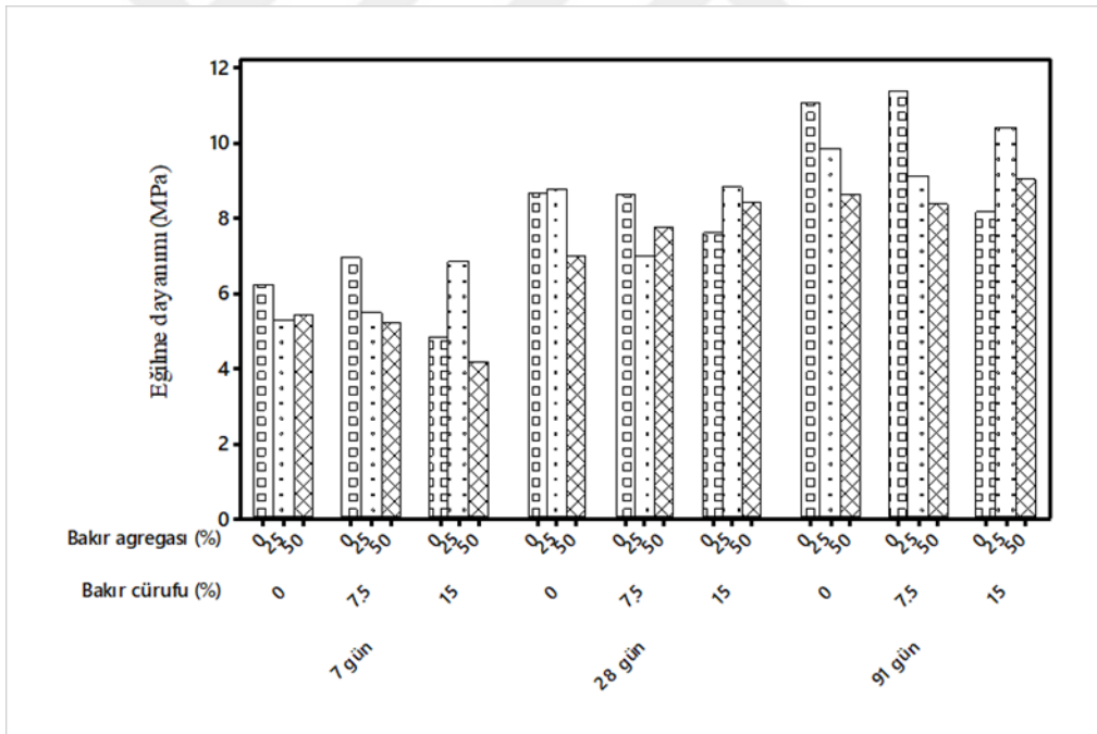
(b) Bakır atıklarının etkisi
