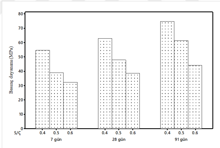
Şekil 4.11 S/Ç oranının basınç dayanımına etkisi
