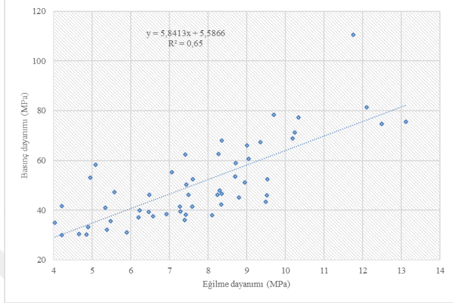
Şekil 4.12 Basınç ve eğilme dayanımı arasındaki ilişki
