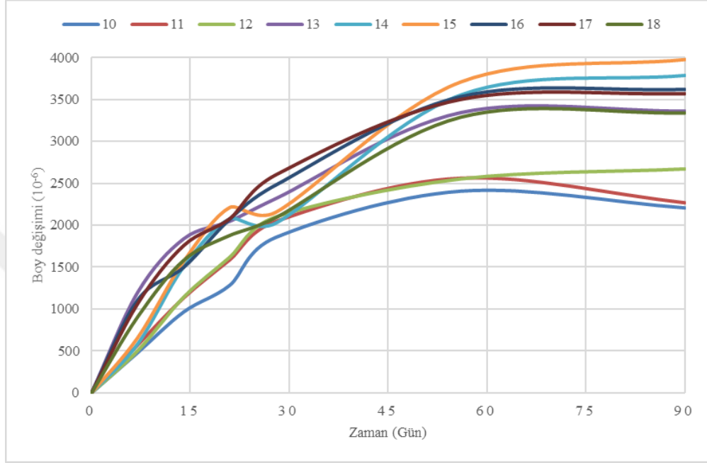
Şekil 4.16 12 mm uzunluğundaki liflerden üretilen karışımların kuruma büzülmesi özellikleri
