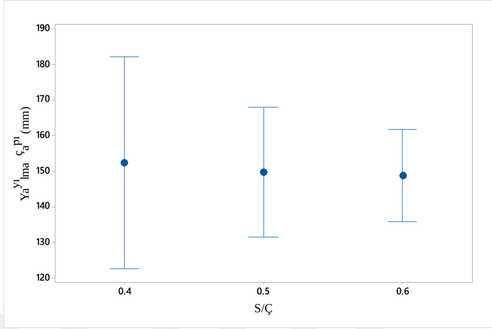
Şekil 4.4 S/Ç oranının yayılma çapı üzerindeki etkisi
