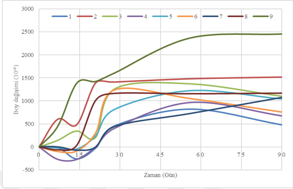
Şekil 4.17 6 mm uzunluğundaki liflerden üretilen karışımların sodyum sülfat etkisindeki özellikleri
