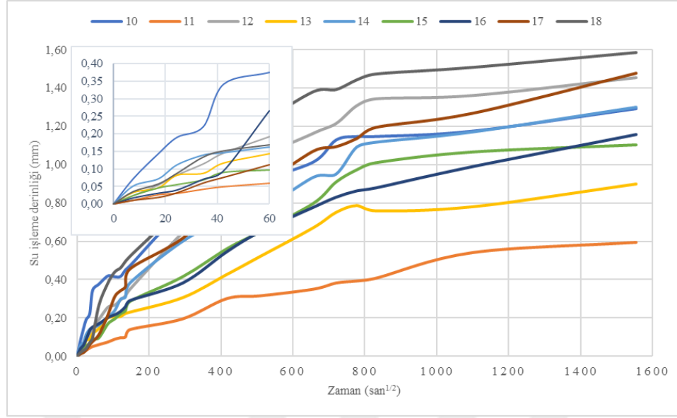
Şekil 4.14 12 mm uzunluğundaki liflerden üretilen karışımların kapilarite özellikleri
