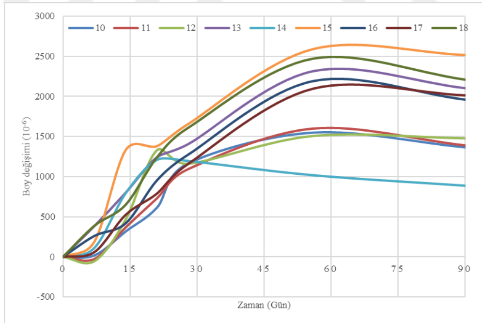
Şekil 4.18 12 mm uzunluğundaki liflerden üretilen karışımların sodyum sülfat etkisindeki özellikleri
