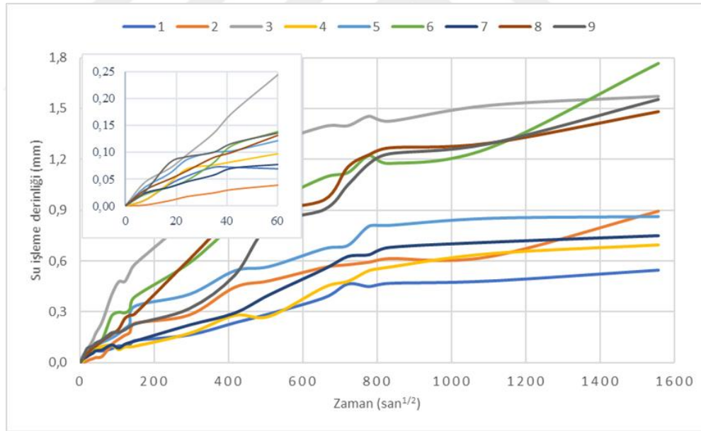
Şekil 4.13 6 mm uzunluğundaki liflerden üretilen karışımların kapilarite özellikleri
