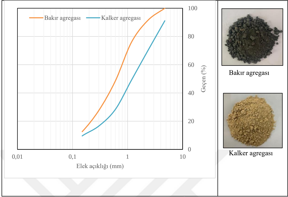
Şekil 3.1 Agregalara ait tane dağılımları
