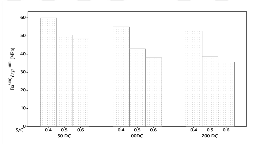
Şekil 4.22 S/Ç etkisinin donma-çözülme sonrasındaki basınç dayanımına etkisi
