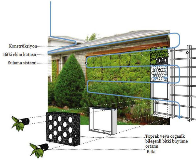
Şekil 4.24. Yeşil duvar (Huber, 2010'dan uyarlanmıştır).
