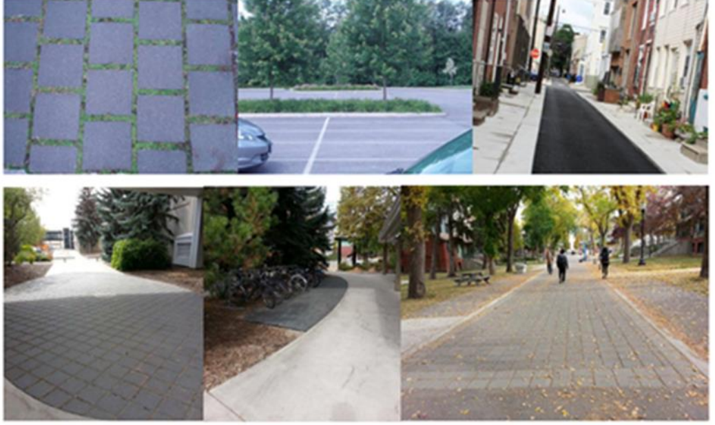
Şekil 4.13. Geçirimli kaplama uygulama örnekleri (The City of Edmonton, 2014’den uyarlanmıştır).
