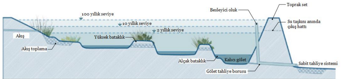
Şekil 4.27. Sulak alan kesit (Team Sponge, 2019'dan uyarlanmıştır).
