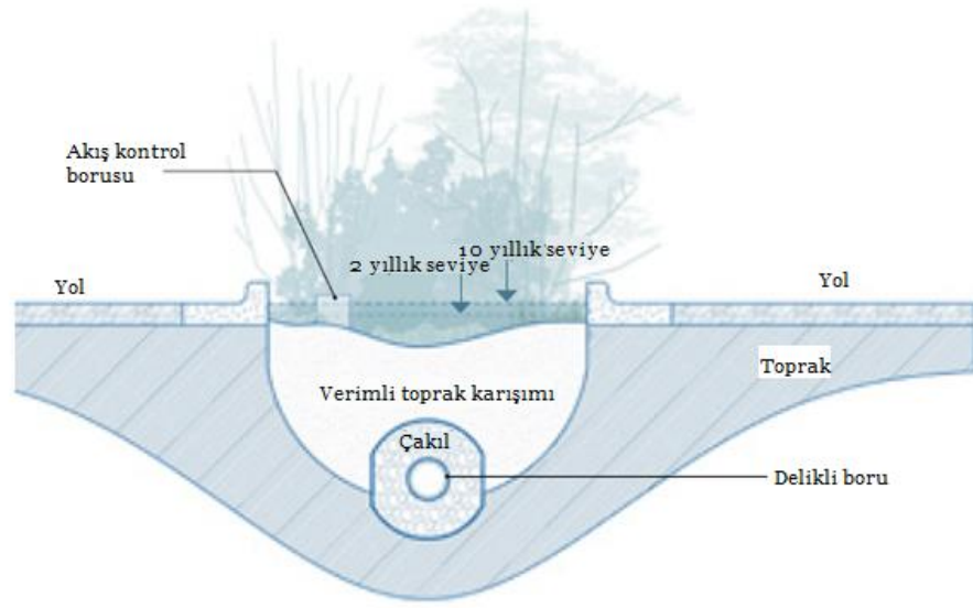
Şekil 4.10. Bitkili su hendeği kesiti (Team Sponge, 2019'dan uyarlanmıştır).
