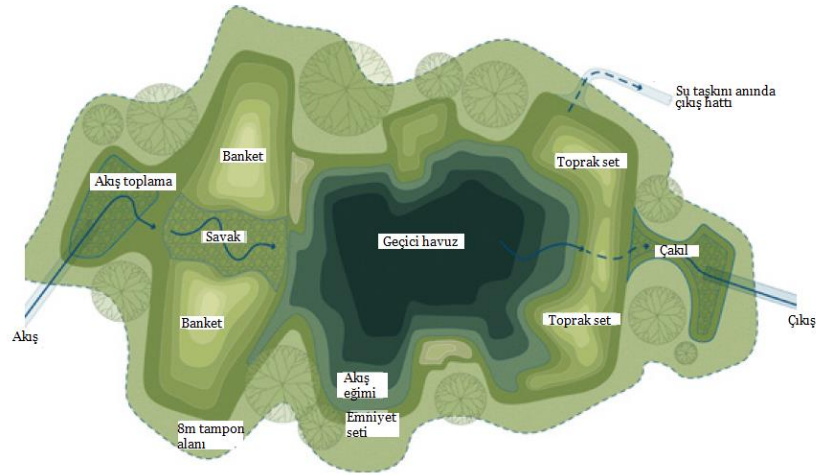
Şekil 4.26. Yapay sulak alan planı (Team Sponge, 2019'dan uyarlanmıştır).
