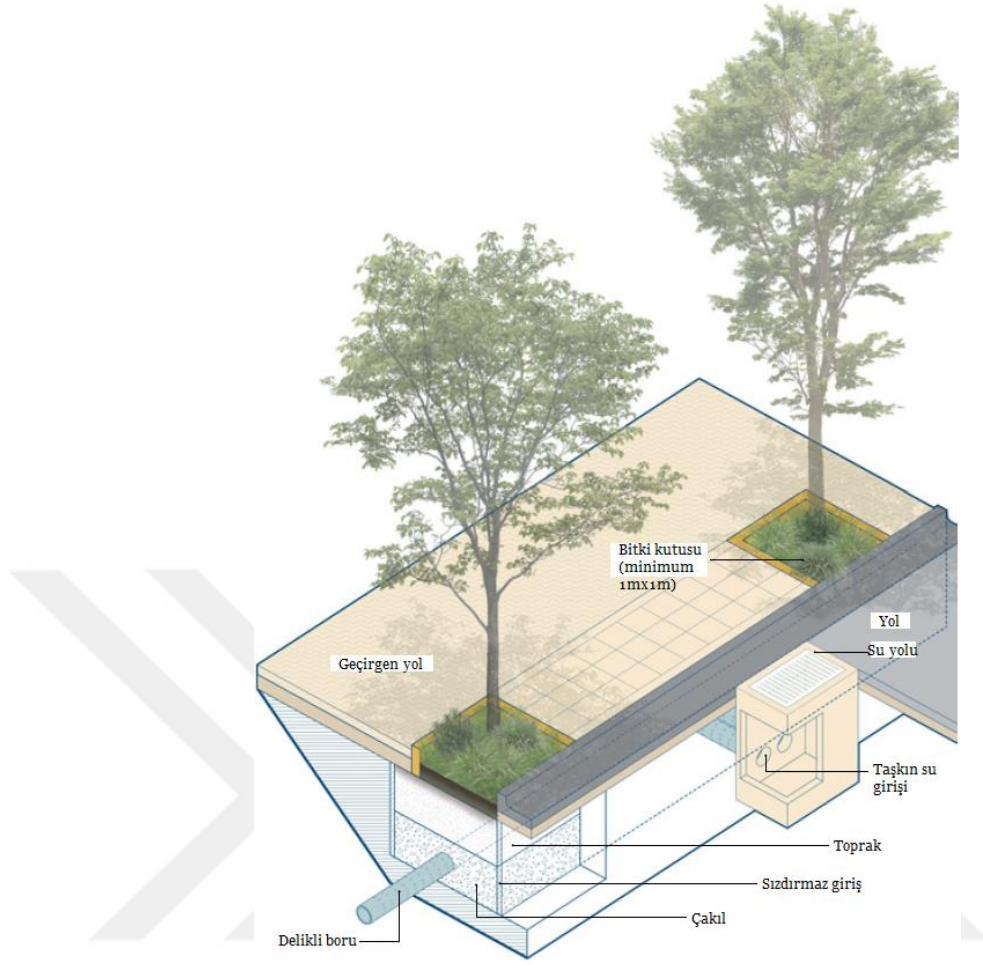
Şekil 4.30. Yol ağacı kesit (Team Sponge, 2019'dan uyarlanmıştır).
