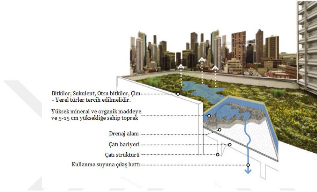
Şekil 4.18. Yeşil çatı (Huber, 2010'dan uyarlanmıştır).
