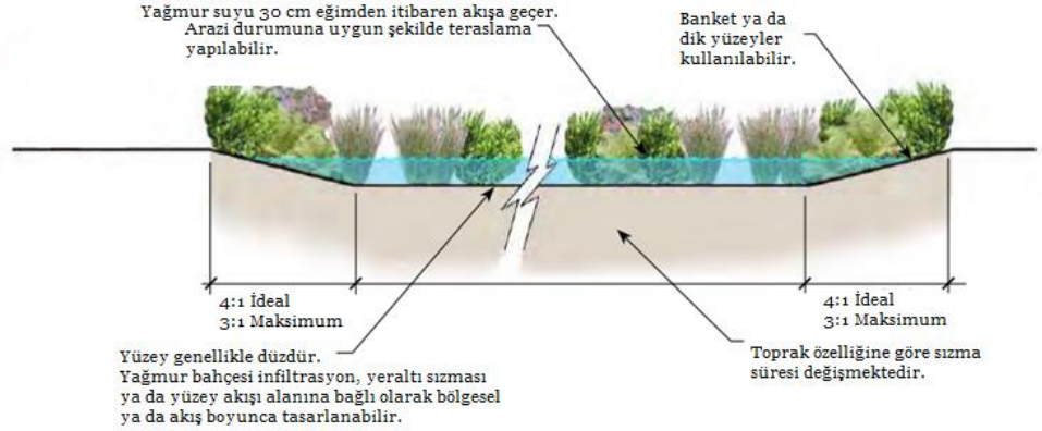
Şekil 4.6. Yağmur bahçesi kesiti (Water Pollution Prevention Program, 2019'dan uyarlanmıştır).
