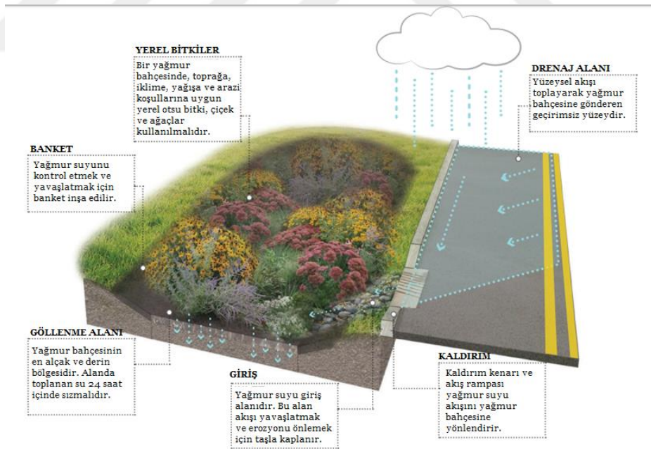
Şekil 4.4. Yağmur bahçesi (Rutgers, 2016'dan uyarlanmıştır).
