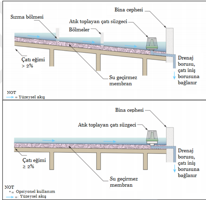
Şekil 4.21. Bölmeli ve bölmesiz mavi çatı profili (Blick, Kelly, Skupien, 2004'den uyarlanmıştır).
