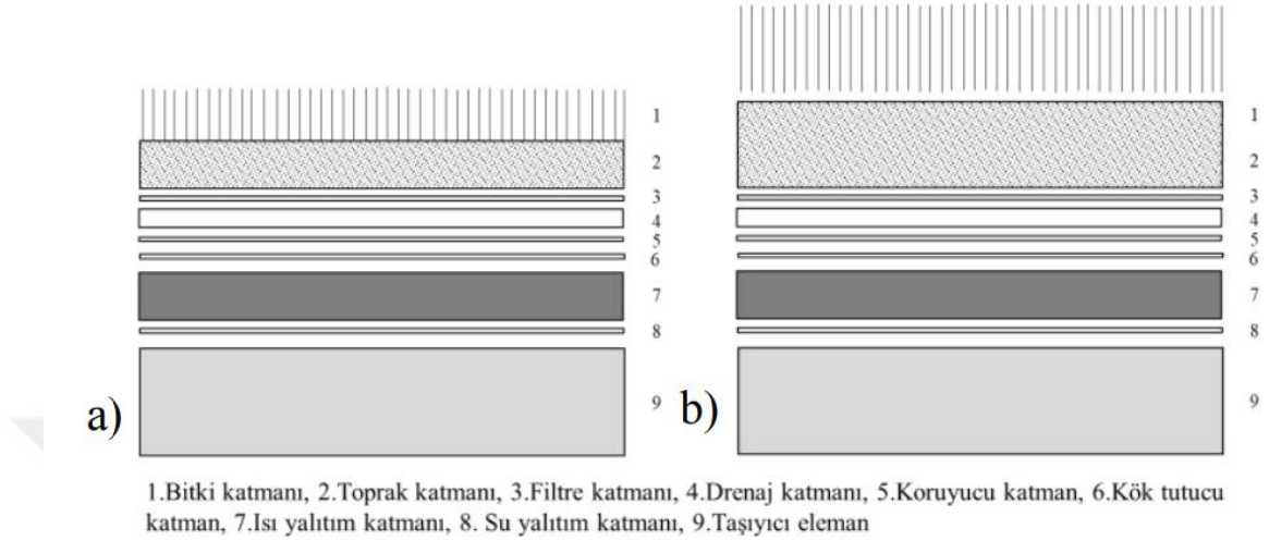
Şekil 4.16. Yeşil çatı konstrüksiyonu a) ekstensif yeşil çatı b) intensif yeşil çatı (Kalfa, Haydararslan, Yaşar, 2018).
