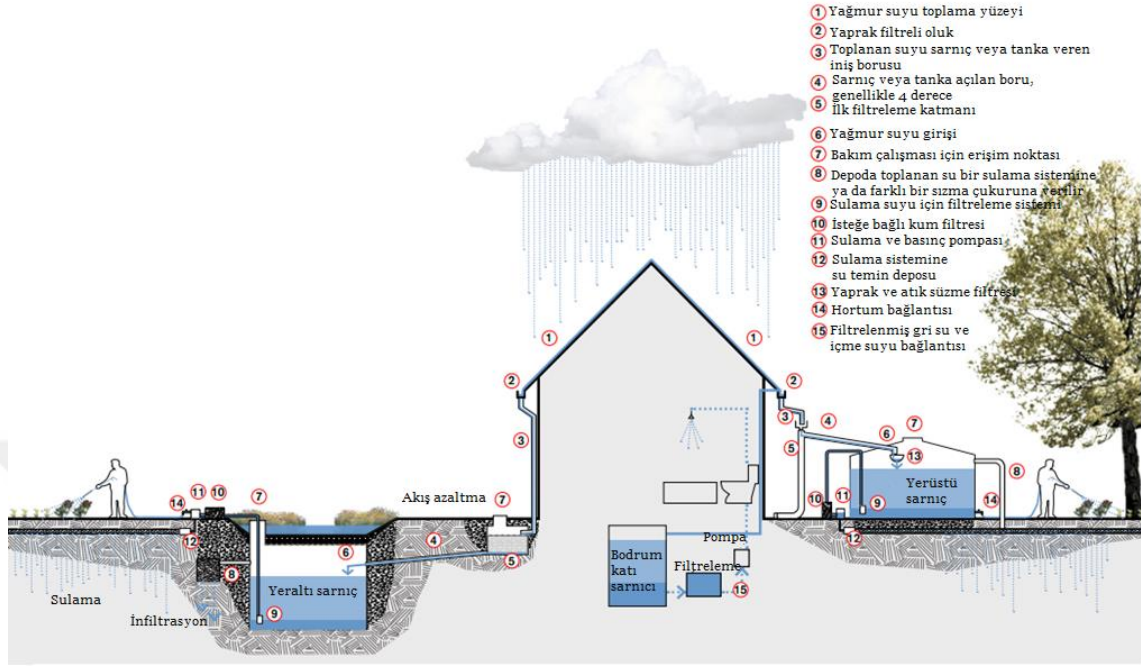
Şekil 4.2. Yağmur suyu sistemi detayı (University of Arkansas Community Design Center, 2010'dan uyarlanmıştır).
