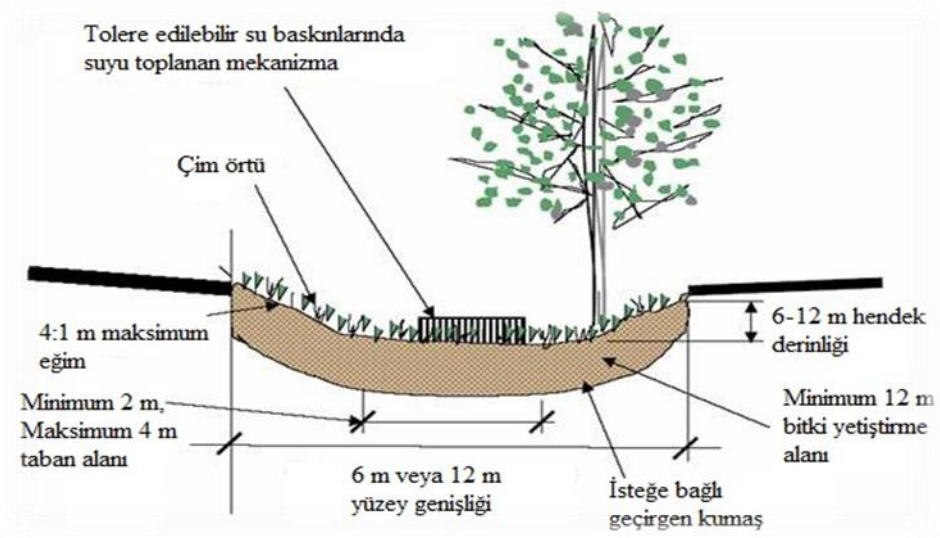
Şekil 4.8. Bitkili su hendeği tasarımı (Ellis vd., 2014’den uyarlanmıştır)
