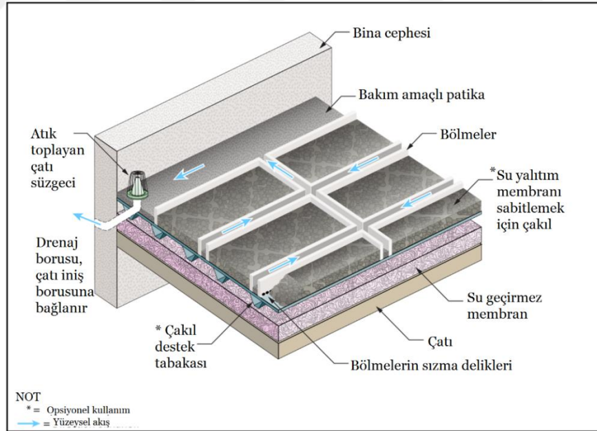
Şekil 4.20. Mavi çatı ve bölmelendirilmesi (Blick, Kelly, Skupien, 2004'den uyarlanmıştır).
