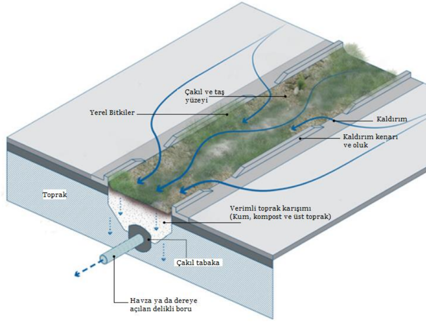
Şekil 4.9. Bitkili su hendeği (Team Sponge, 2019’ dan uyarlanmıştır).
