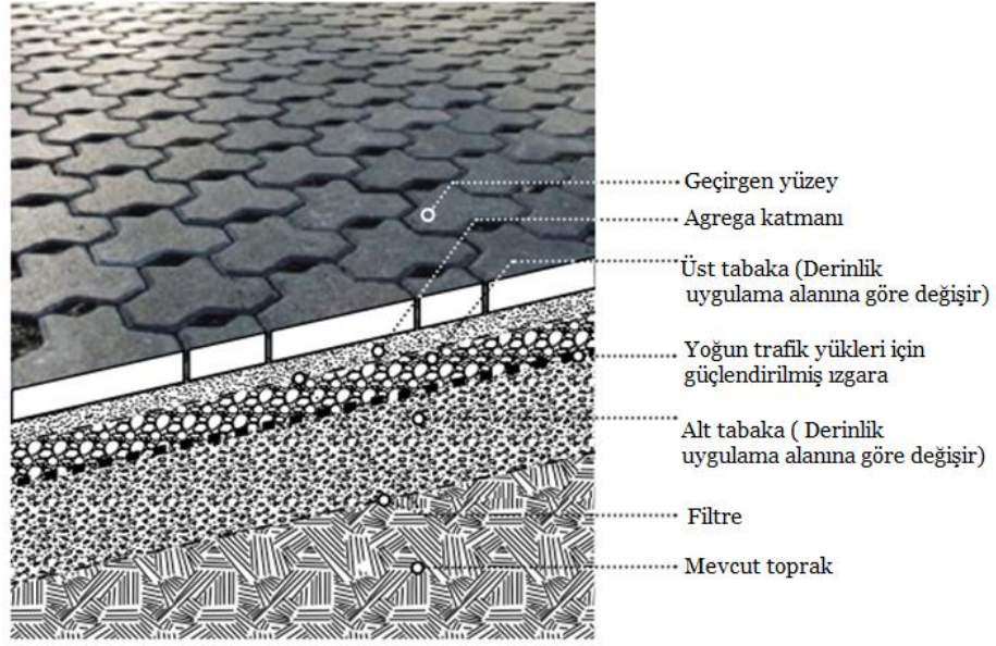
Şekil 4.12. Geçirgen kaplama detayı (University of Arkansas Community Design Center, 2010'dan uyarlanmıştır).
