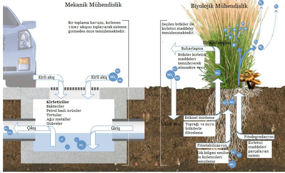
Şekil 2.3. Düşük etkili gelişim modeli (Huber, 2010'dan uyarlanmıştır)
