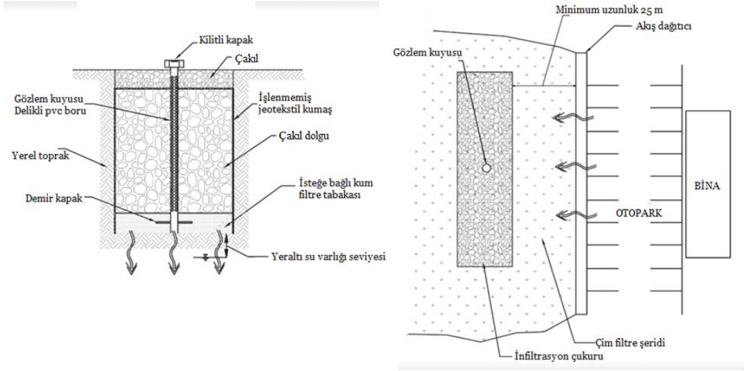
Şekil 4.14. İnfiltrasyon haznesi/hendeği (Burack, Walls, Stewart, 2008'den uyarlanmıştır).
