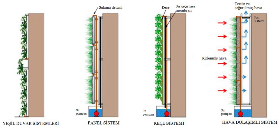
Şekil 4.23. Yeşil duvar uygulama yöntemi örnekleri (Pérez-urrestarazu vd., 2016'dan uyarlanmıştır).
