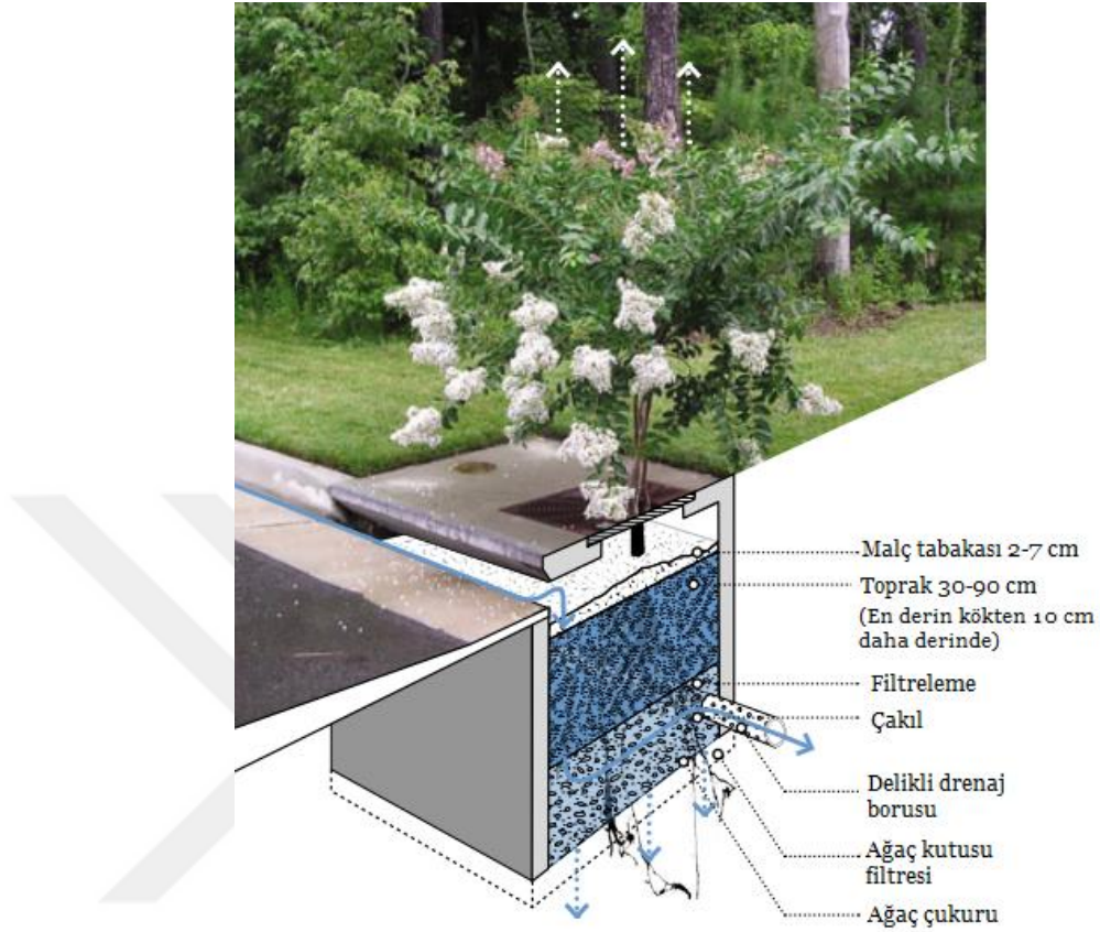
Şekil 4.29. Yol ağacı bitki kutusu detayı (Huber, 2010'dan uyarlanmıştır).
