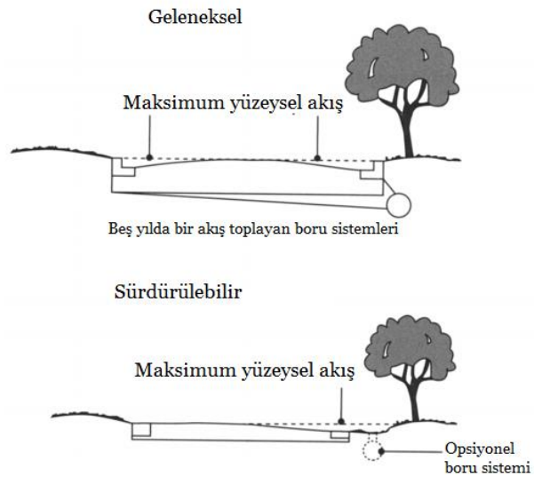
Şekil 1.14. Yol kesiti (Victoria Stormwater Committee, 1999'dan uyarlanmıştır).
