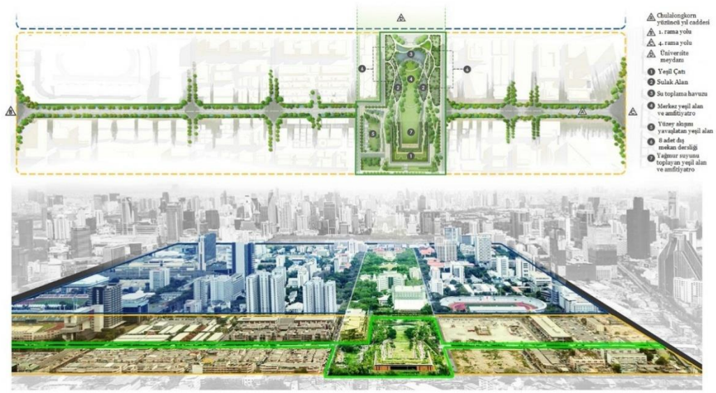
Şekil 5.2. Chulalongkorn Yüzüncü Yıl Parkı planı (ASLA, 2019'dan uyarlanmıştır).
