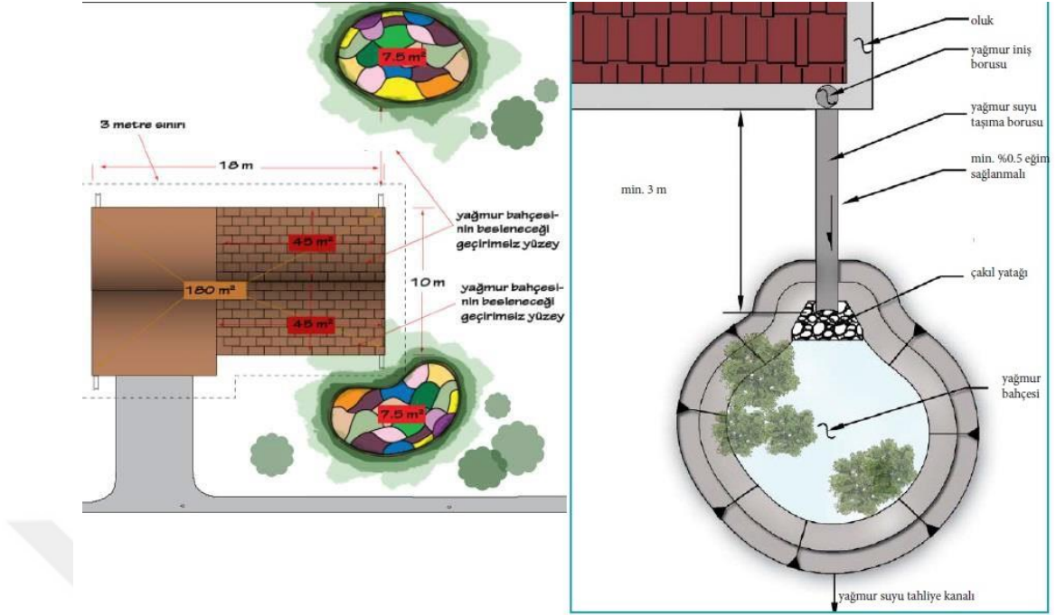
Şekil 4.5. Yağmur bahçesi konumlandırılması (Çevre ve Şehircilik Bakanlığı, 2018b).
