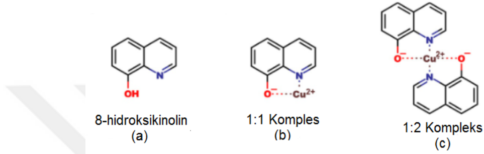
Şekil 4.2. a) 8-HQ yapısı b) 1:1 metal:lingant oranında Cu(II) iyonlarının 8-HQ ile oluşturduğu kompleks c) 1:2 metal:lingant oranında Cu(II) iyonlarının 8-HQ ile oluşturduğu kompleks (Dalecki et al., 2017)
