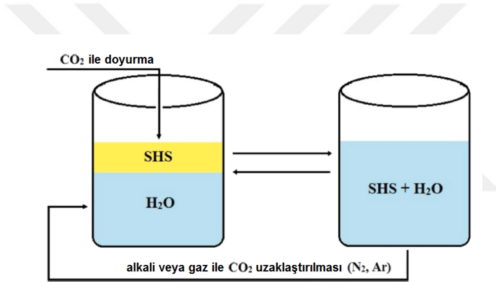
Şekil 2.4. Hidrofilikliğı değiştirilebilir çözücülerin oluşturulması (Bazel et al., 2020).
