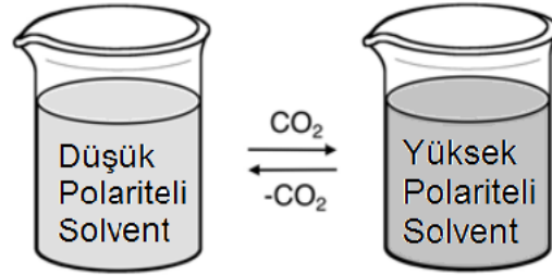
Şekil 2.5. Değiştirilebilir polariteye sahip çözücüler yüksek polariteli çözeltiliye dönüşmek için \text{CO}_2 ile reaksiyona girerler ve \text{CO}_2 nin uzaklaşması ile çözelti eski haline döner (Jessop, 2013)
