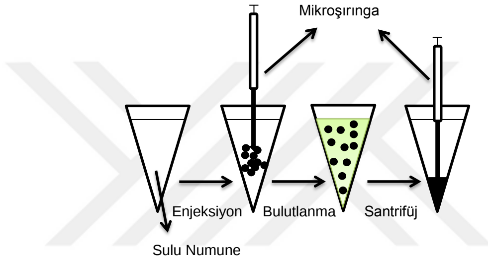
Şekil 2.13. DLLME yöntemi şematik gösterimi
