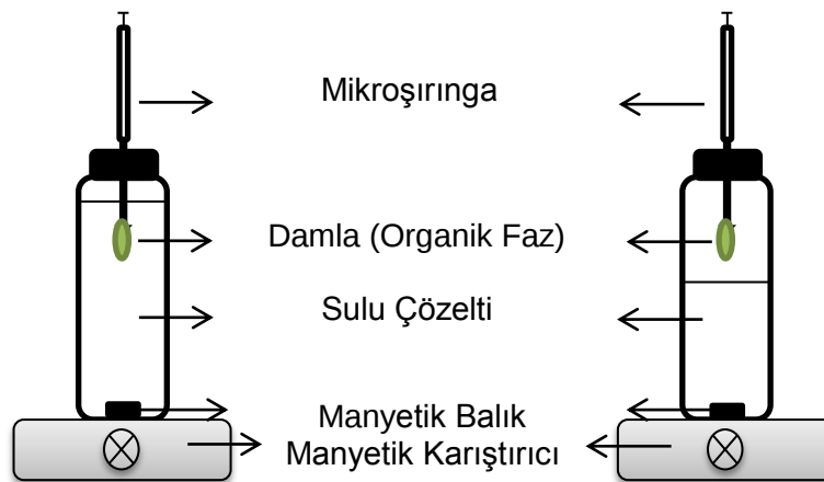
Şekil 2.9. (a) DI-SDME, (b) HS-SDME yöntemi şematik gösterimi
