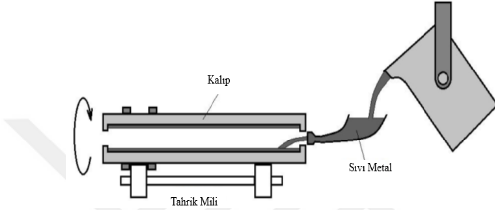
Şekil 3.4. Yatay gerçek santrifüj döküm yönteminin şematik gösterimi [32].
