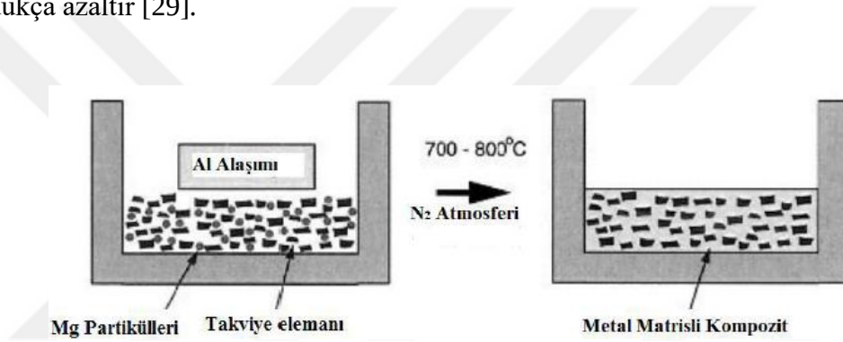
Şekil 3.8. Basıncsız infiltrasyon yöntemi [29].
