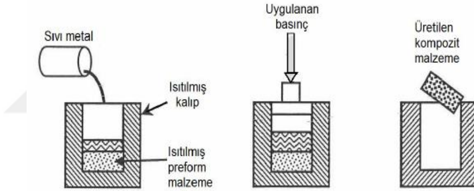
Şekil 3.3. Sıkıştırılmalı döküm tekniğinin üretim aşamaları [18].
