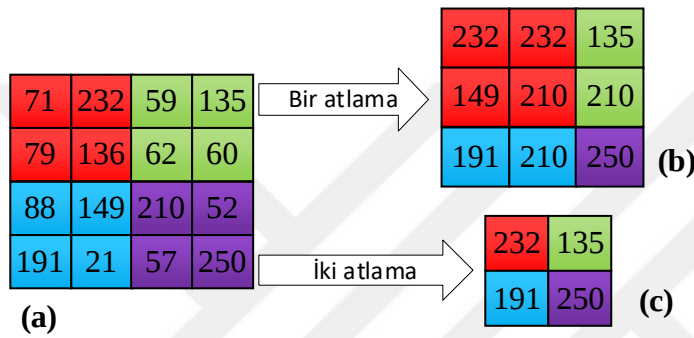
Şekil 2.18. Farklı atlama sayıları ile örnek bir atlama işlemi a) 4x4 giriş hacmi; b) S = 1 adımıyla maksimum 2x2 havuzlama uygulaması; c) S = 2 ile maks. 2x2 havuzlama uygulaması
