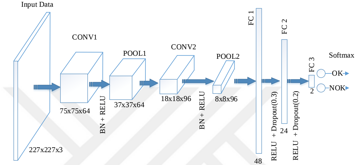
Şekil 3.12. Tohum sınıflandırma problemi için önerilmiş özel ağ yapısı (Custom227)
