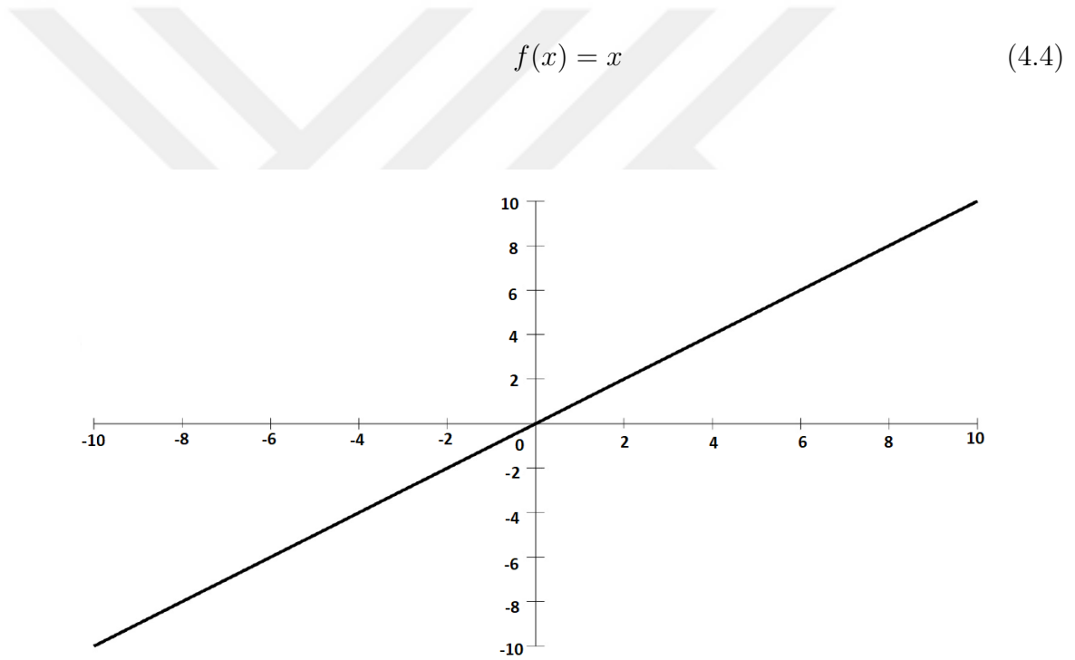
Figure 4.4. Linear function
