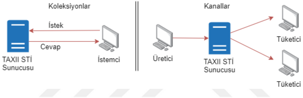
Şekil 2.12. TAXII protokolü ile STİ verisi paylaşım yöntemleri [44]
