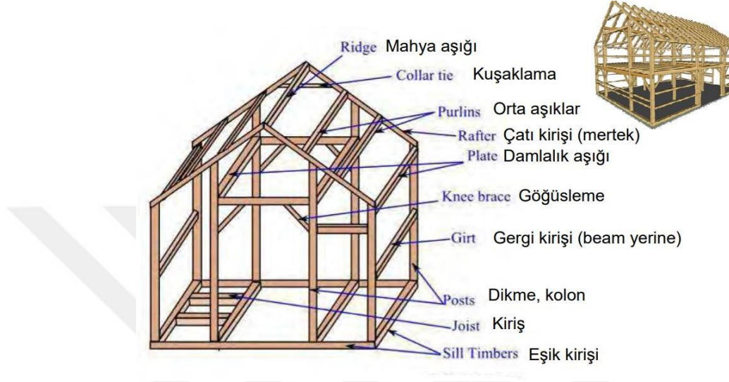
Şekil 6.1. : Ahşap yapı iskeleti [2].
