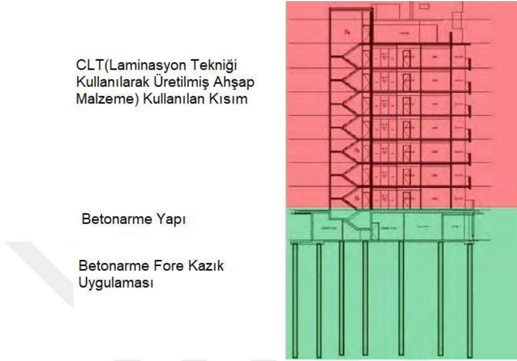
Şekil 9.13. : Forté Living, Avustralya- yapının toprak altında kalan kısımları forekazıklardan oluşurken, giriş katı betonarmeden meydana geliyor [82].
