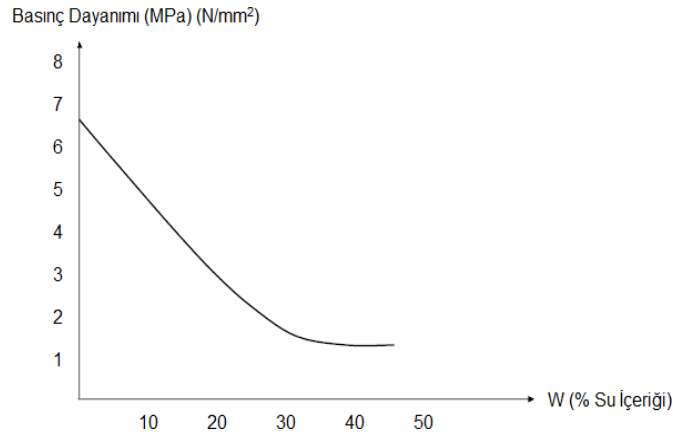
Şekil 2.1. :Birim hacim ağırlığı 0.42 \text{ kg/ dm}^3 olan bir kozalaklı ağacın basınç dayanımının (lifler doğrultusunda) su içeriği ile değişim grafiği [4].
