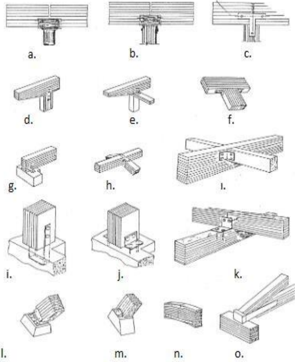
Şekil 5.11. : Laminasyonlu ahşap ile aşık bağlantısında kullanılan bağlantı elemanları [45].
