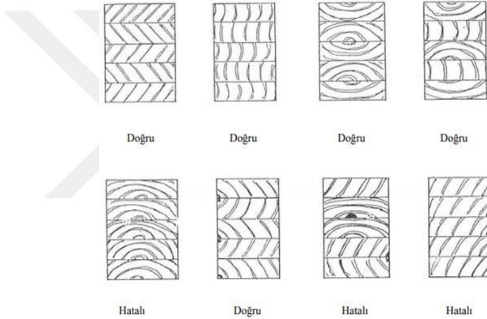
Şekil 4.2. : Laminasyonda katların düzenlenmesi [29].
