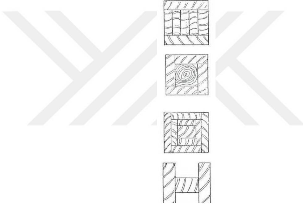
Şekil 4.4. : Liflere paralel basınç yüküne maruz kalan lamine elemanlarda (kolonlarda) katların karışık düzenlenmesi [29].
