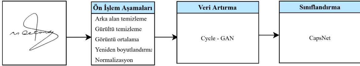
Önerilen Veri Artırma ve İmza Doğrulama Sistemi
