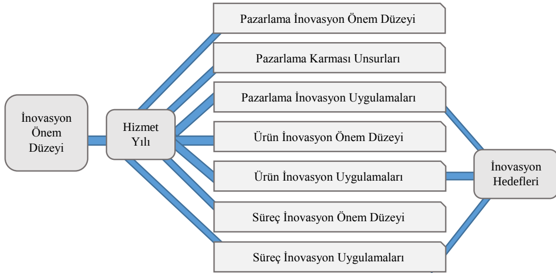
Şekil 3.1. Araştırma Modeli
