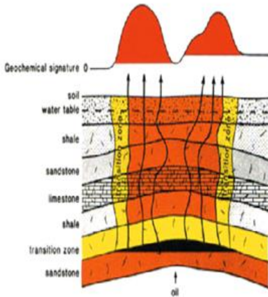
Şekil 2.5. Dikey göç dördüncü aşama (Tedesco, 1995)
