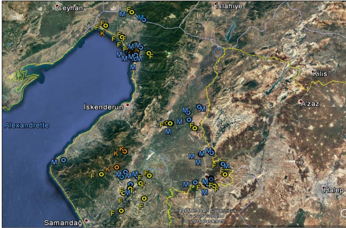
Şekil 3.1. Suların petrol hidrojeokimyası açısından tipleri (F: Fosil, M: Meteorik, K: Karışım)
