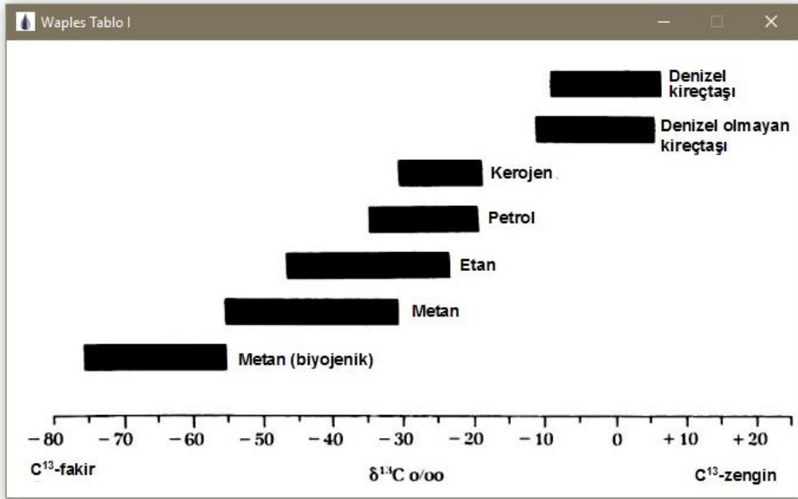
Şekil 3.21. Waples’a göre Karbon 13 izotopunun çeşitli formlardaki dağılım aralıkları
