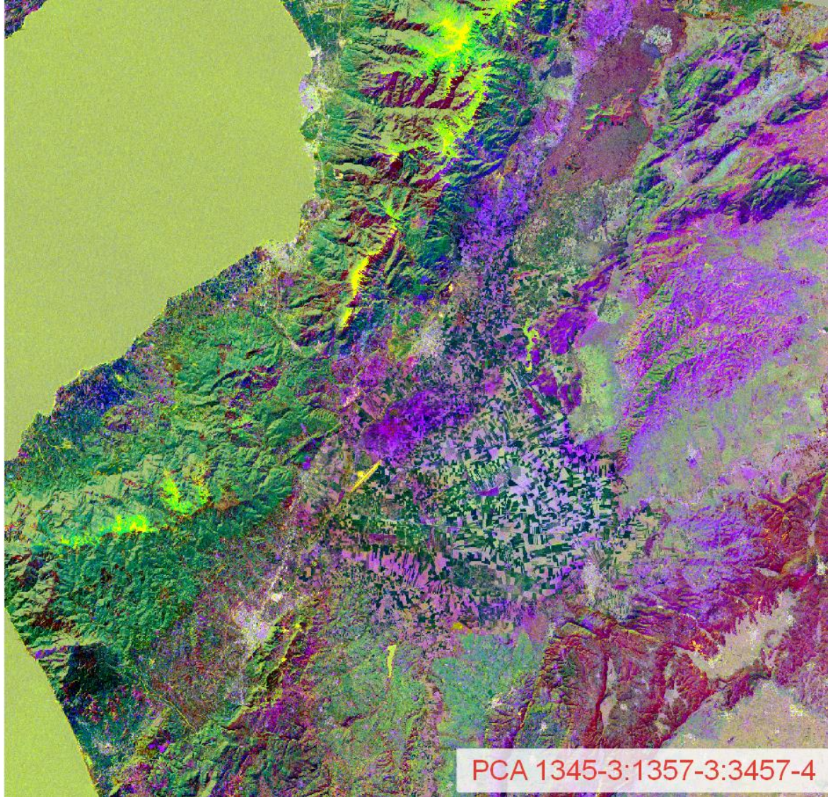
Şekil 3.23. Landsat-7 ETM+ PCA R: 1345-3, G: 1357-3, B: 3457-4 kompozit görüntüsü
