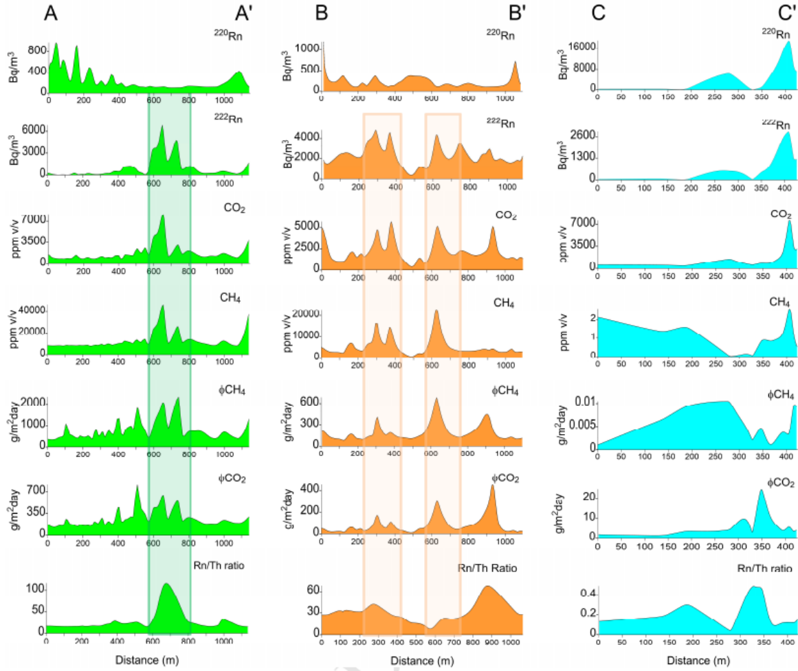
Şekil 2.18. Radon anomali kesitlerinin gösterilişi (Sciara vd., 2017)
