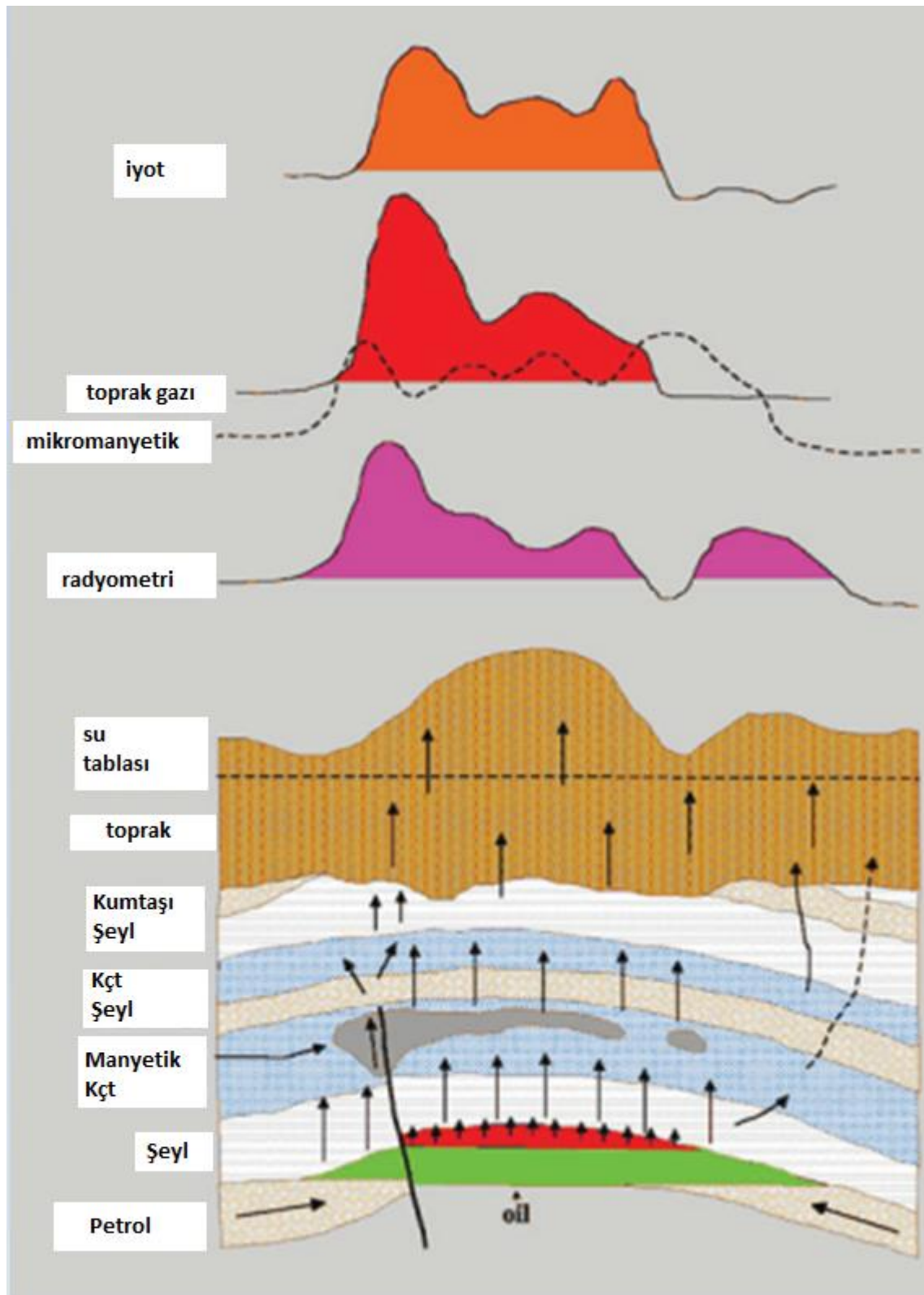
Şekil 2.8. Mikrosızıntı tespitinde kullanılan farklı yöntemlere göre anomali tiplerinin modellenmesi (Tedesco, 1995)
