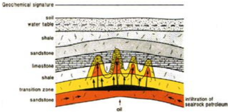
Şekil 2.3. Dikey Göç İkinci Aşama (Tedesco, 1995)
