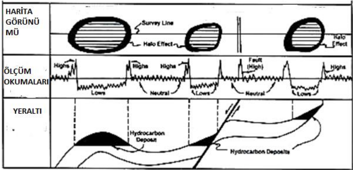
Şekil 2.14. Farklı kapan tiplerine göre Radyometrik halo anomalisi türleri (Fernandez vd., 2015)
