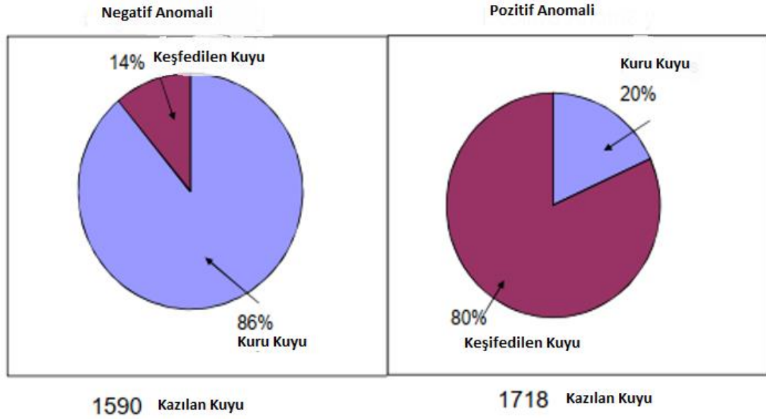
Şekil 1.3. Çeşitli havzalarda şirketlerce çeşitli yöntemlerle kazılan kuyular (Schumacher, 2017)
