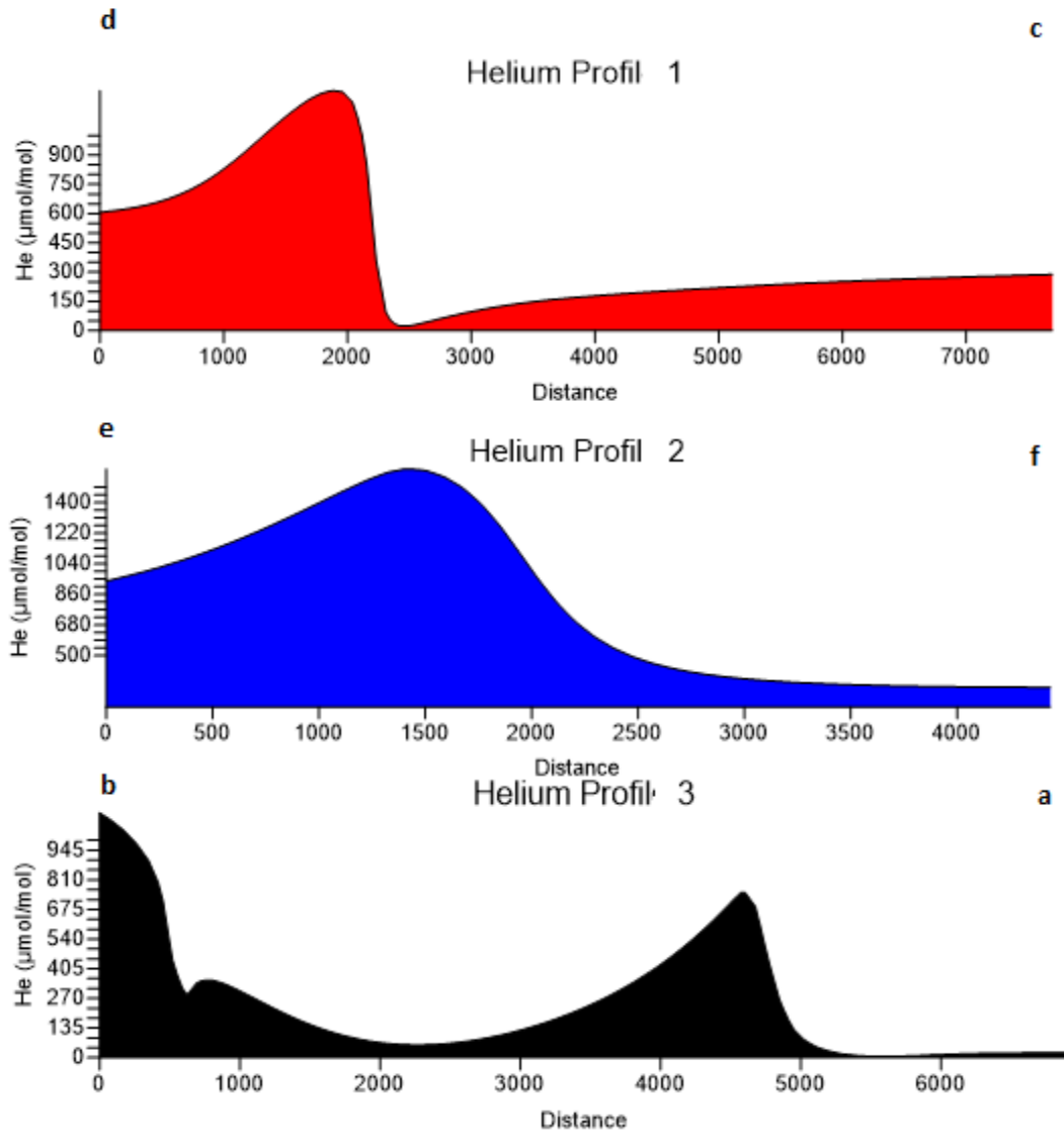
Şekil 3.18. Kırmızı Mavi ve Siyah hatlardan alınan helyum miktarına bağlı profiller.
