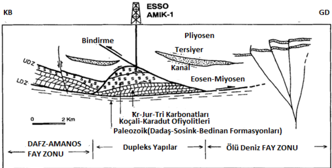
Şekil 3.15. Kuyu yerinin yapısal jeoloji kesiti (Coşkun, 1994)
