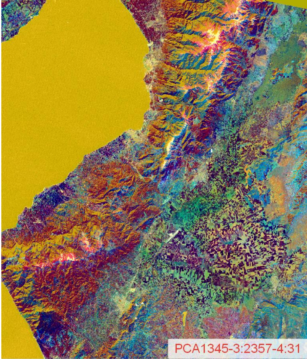
Şekil 3.25. Landsat-7 ETM+ PCA R:1345-3, G: 2357-4, B: 3/1 bant oranı kompozit görüntüsü
