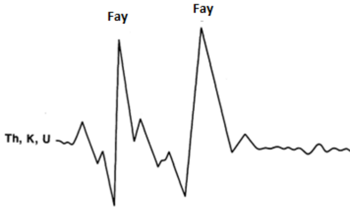
Şekil 2.17. Radyometri profilinin yorumu (Tedesco, 1995)
