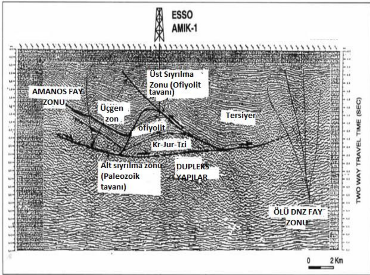
Şekil 3.14. Amik-1 kuyusuna ait sismik kesit (Coşkun,1994)
