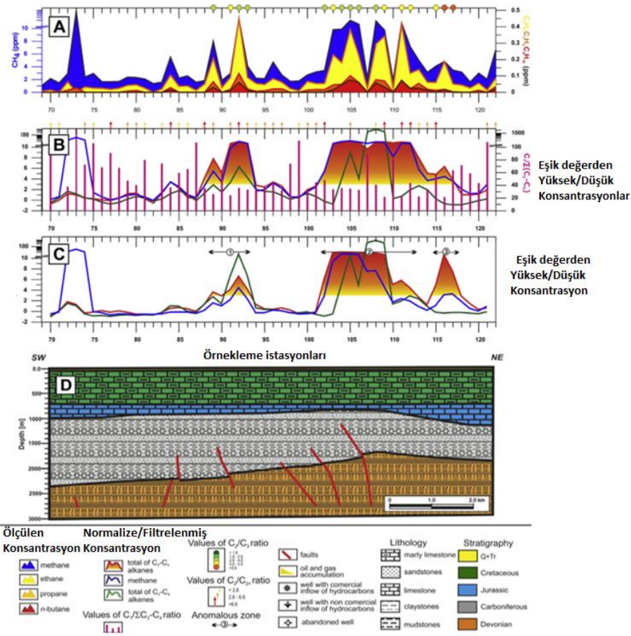
Şekil 2.11. Toprak gazı verilerinin gösterimi (alkanlar) (Sechman vd. 2015)
