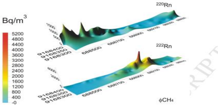
Şekil 2.19. Radon anomali kesitlerinin 3 Boyutlu gösterilişi (Sciara vd., 2017)
