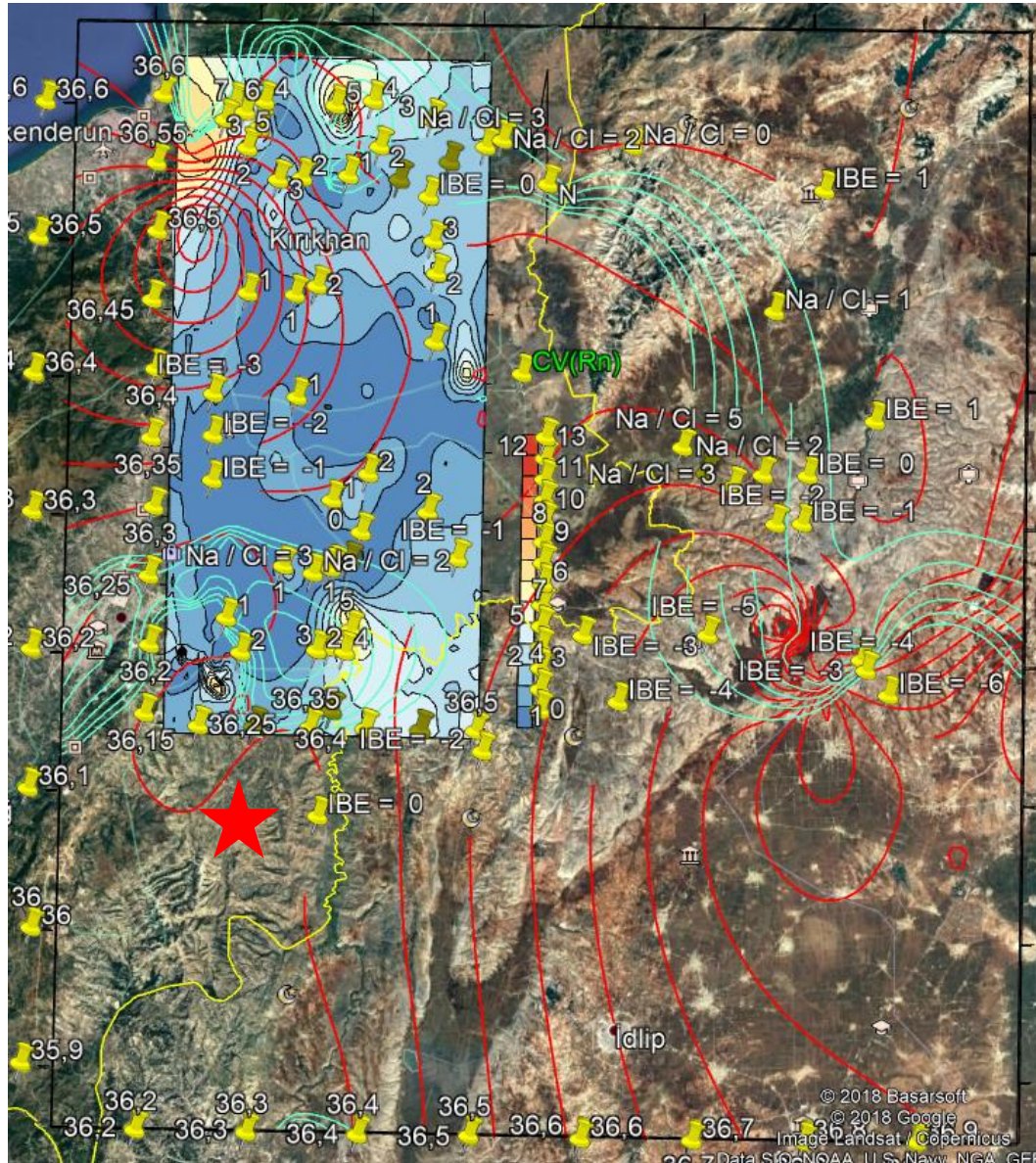
Şekil 3.12. Sulin ve Schoeller hidrohipslerinin üzerine bindirilmiş Radon anomalilerinin Google Earth üzerinde gösterimi.
