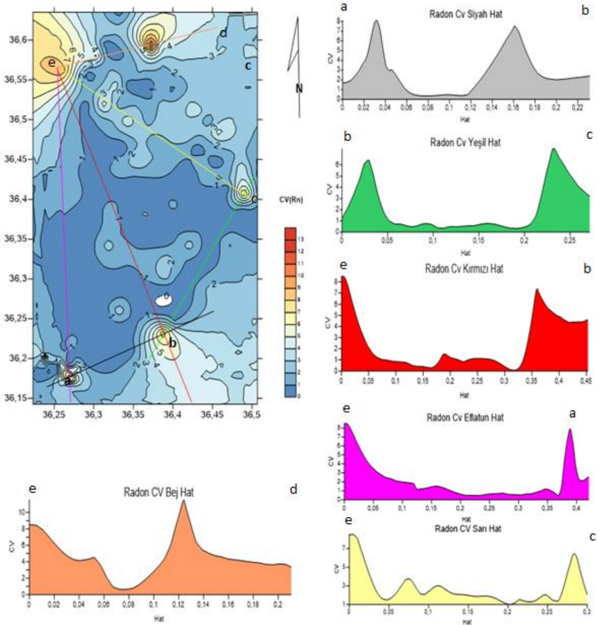
Şekil 3.11. Radon Cv dağılım haritası ve yakalanan halo anomalileri (Krigging yöntemine göre)
