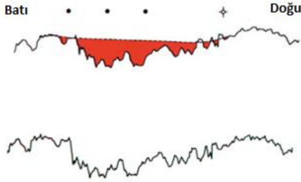
Şekil 2.16. Goldenspike sahası (ABD) radyometrik ölçüm kesiti (Tedesco, 1995)
