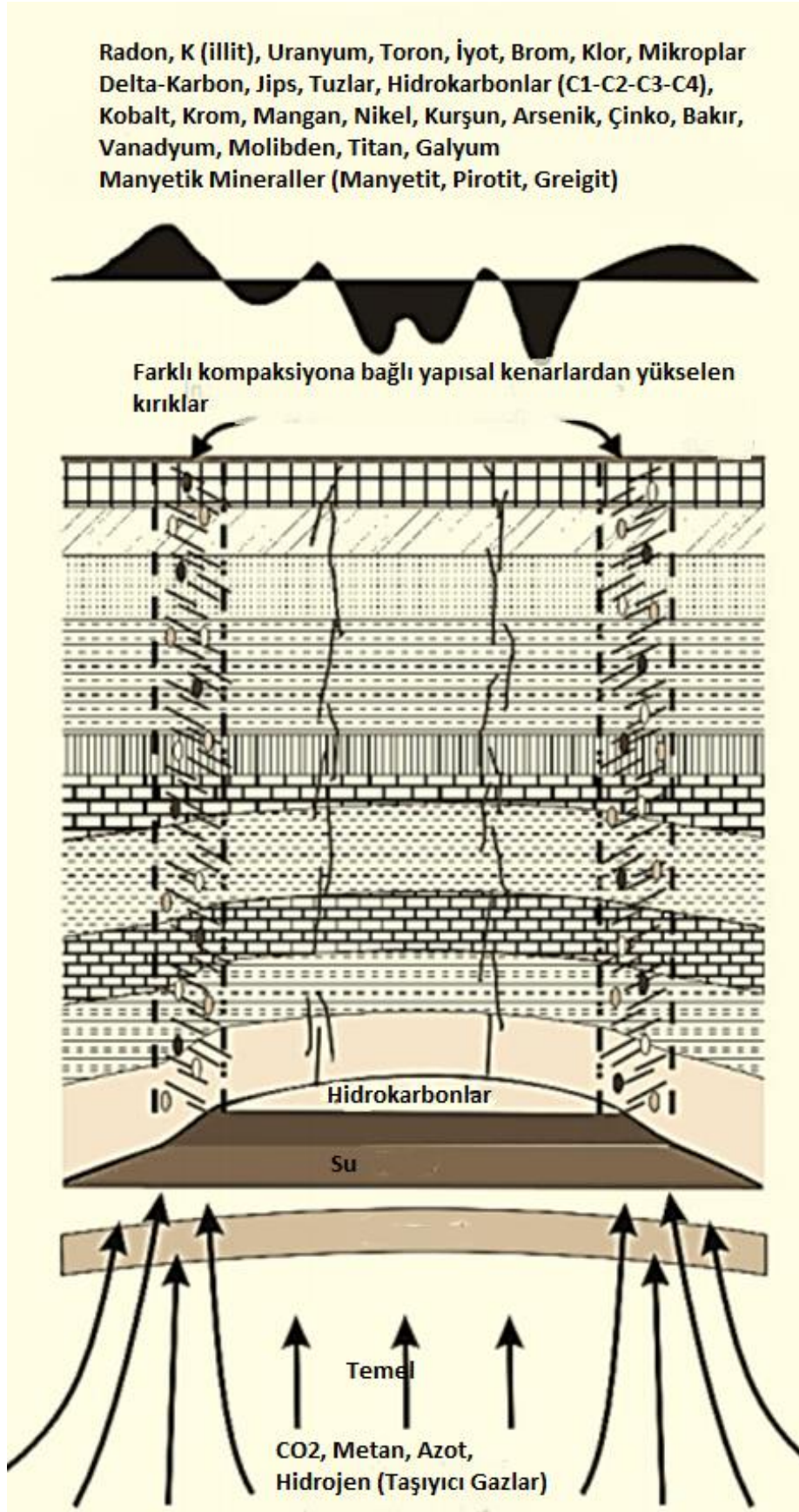
Şekil 2.13. Radyometrik anomali ve kavramsal mikrosızıntı modeli (Fernandez vd., 2015)
