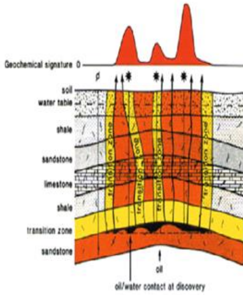
Şekil 2.6. Dikey göç beşinci aşama (Tedesco, 1995)
