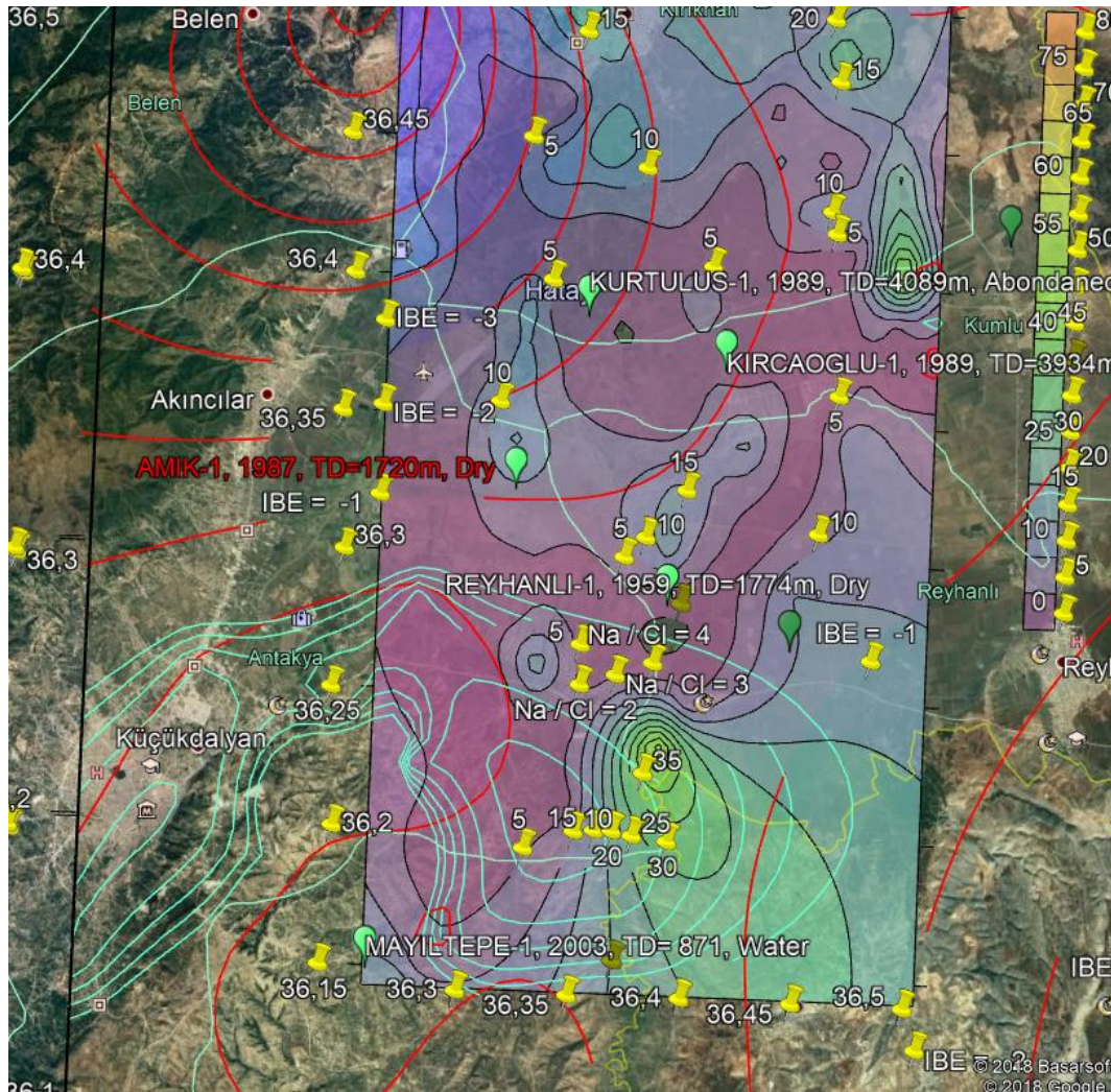
Şekil 3.13. Daha önce açılan sondaj kuyularının yerleri ve radon haritasının Google Earth üzerinde gösterimi
