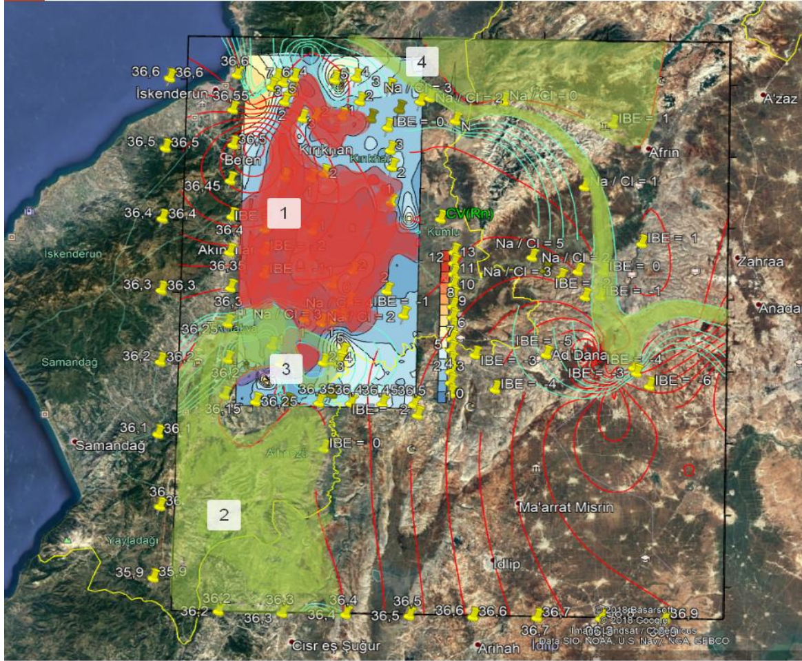
Şekil 3.22. Radon ve Hidrojeokimyasal verilere göre muhtemel rezervuarın olabileceği dört alan. Kırmızı: Radon verileri Yeşil: Hidrojeokimyasal (Sulin ve Shoeller sınıflaması) veriler.
