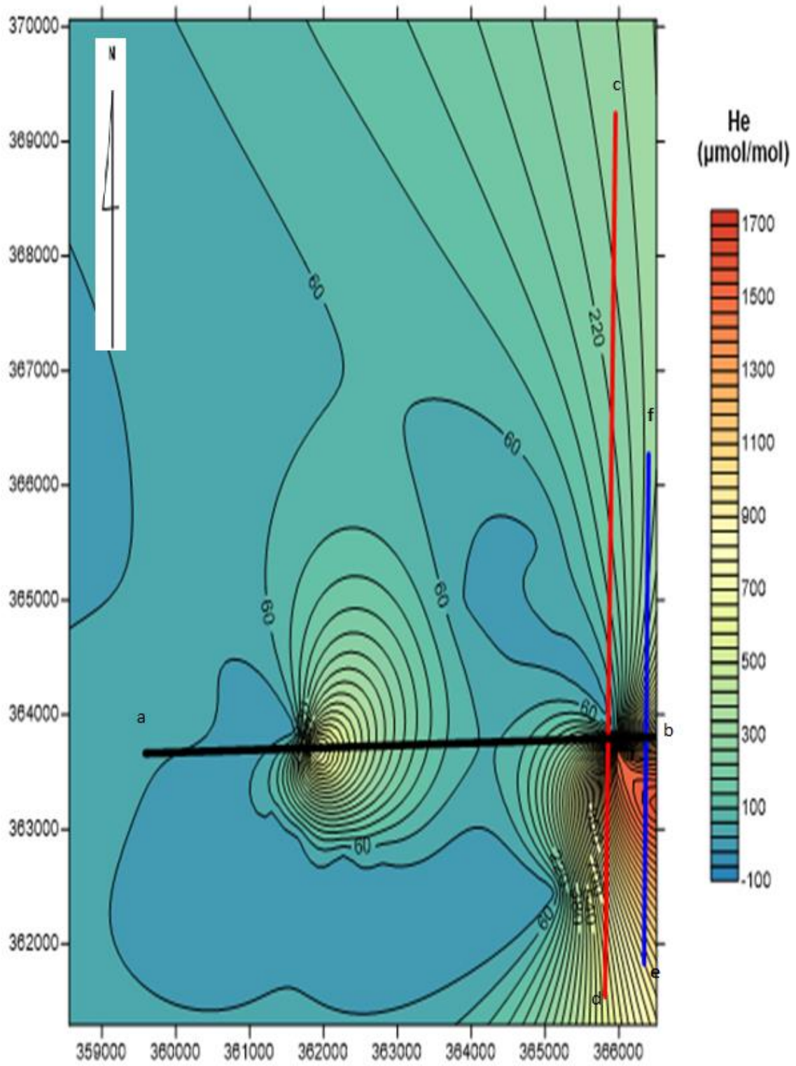
Şekil 3.17. Çalışma alanı Helyum haritası ve renkli helyum profil hatları
