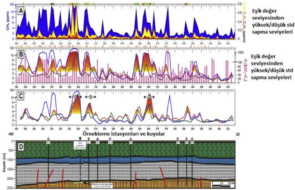
Şekil 2.12. Toprak gazı verilerinin gösterimi (alkenler) (Sechman vd. 2015)
