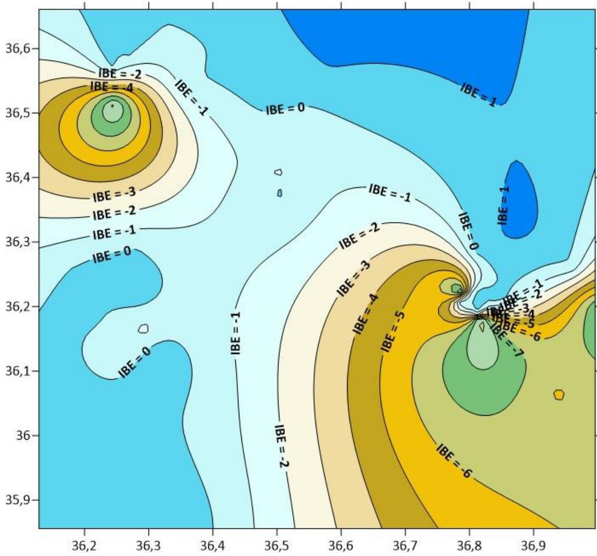
Şekil 3.6. Schoeller Baz Değişim İndeksi (IBE) kontur haritası.
