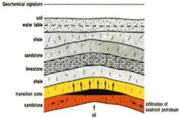
Şekil 2.2. Dikey göç ilk aşaması (Tedesco, 1995)
