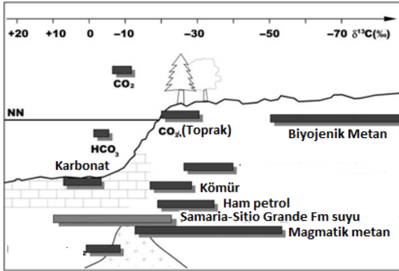
Şekil 3.20. Karbonun çeşitli formlarındaki C-13 izotopunun değeri aralıkları (Birkle vd., 2014)
