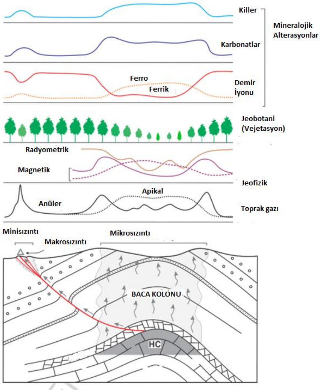
Şekil 2.23. Mikrosızıntı modeline göre mineralojik alterasyonların dağılımları (Assadzadeh, 2017)
