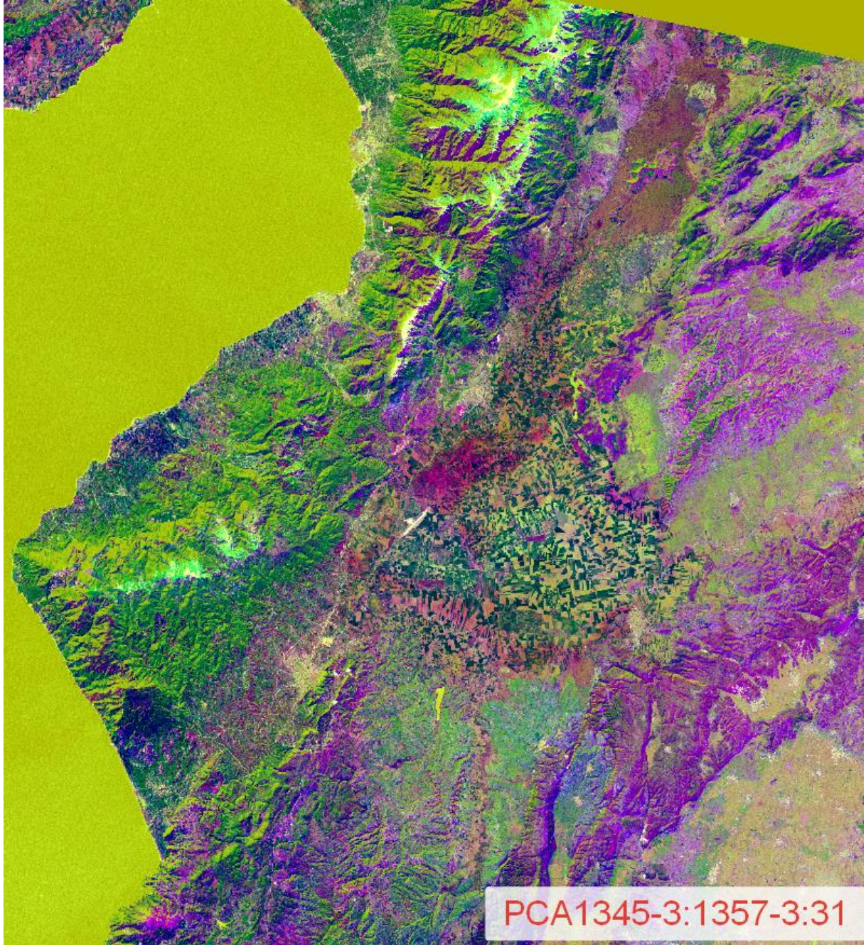
Şekil 3.26. Landsat-7 ETM+ PCA R: 1345-3, G: 1357-3, B: 3/1 bant oranı kompozit görüntüsü
