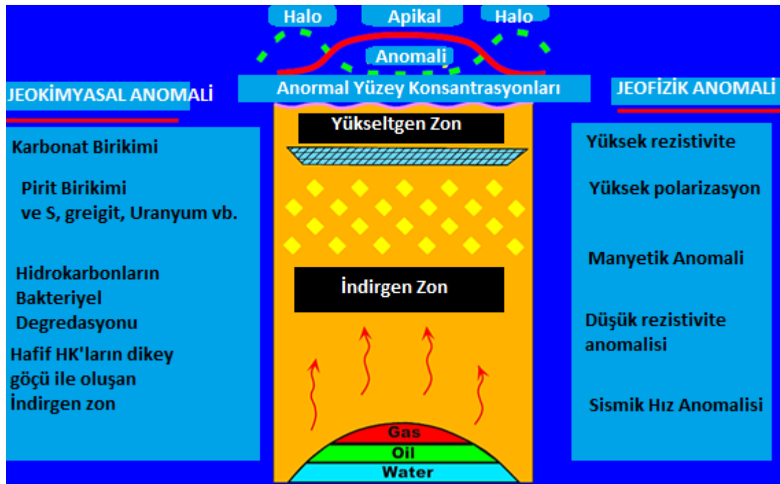
Şekil 2.10. Mikrosızıntılar ve neden oldukları jeokimyasal ile jeofiziksel belirteçler (Schumacher ve Clavereau, 2017)
