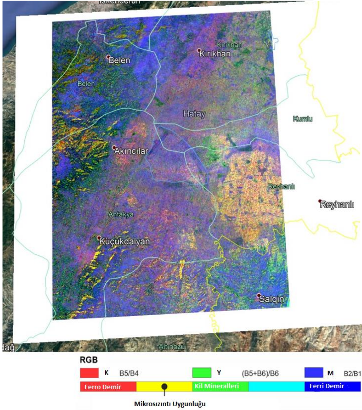
Şekil 3.27. Aster Uydu ile tespit edilen mikrosızıntılar (Hosseinpour, 2020 yöntemine göre)
