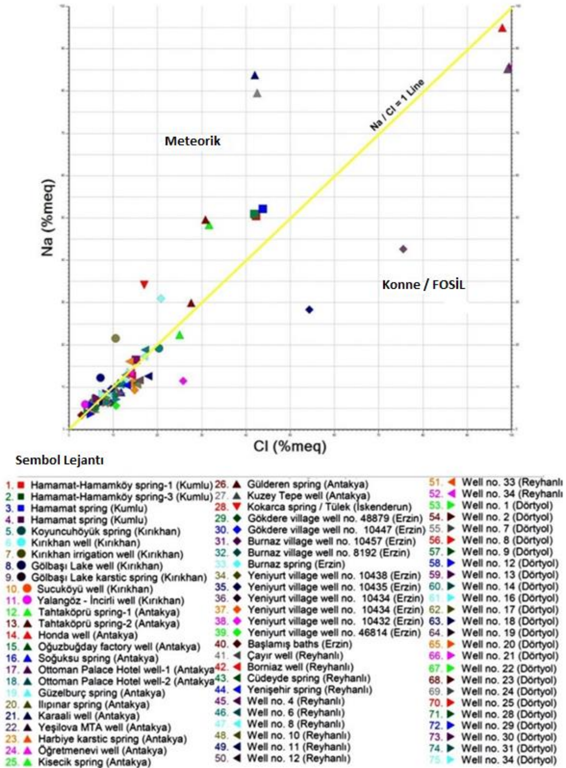
Şekil 3.4. Hatay bölgesi sularının Na/Cl grafiği (1'den küçük olanlar fosil su)
