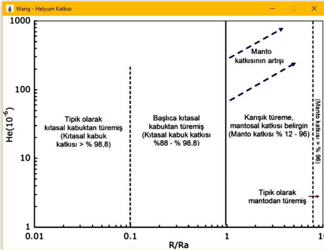
Şekil 3.19. Helyum kökenini değerlendirmek için Hydropet yazılımındaki grafik (Wang vd., 2016)
