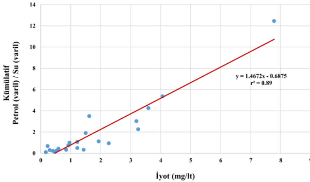
Şekil 2.22. İyot ile petrol/su oranı arasındaki ilişki
