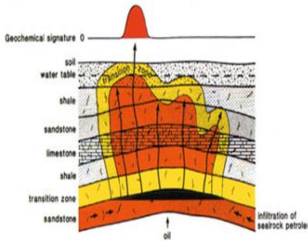
Şekil 2.4. Dikey göç üçüncü aşama (Tedesco, 1995)
