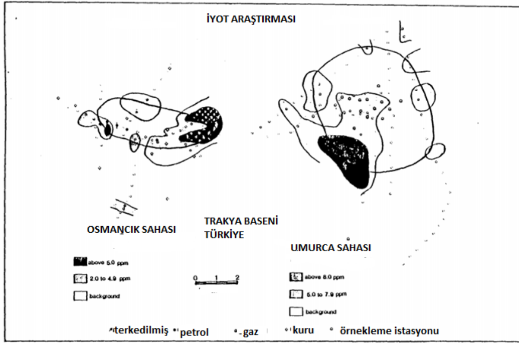
Şekil 2.20. Trakya Baseni Umurca ve Osmancık sahaları iyot araştırması (Allexan vd., 1986)
