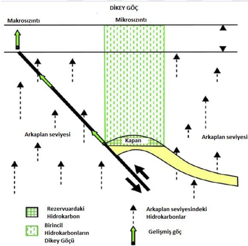
Şekil 2.7. Şematik sızıntı modeli (Rasheed vd., 2015)
