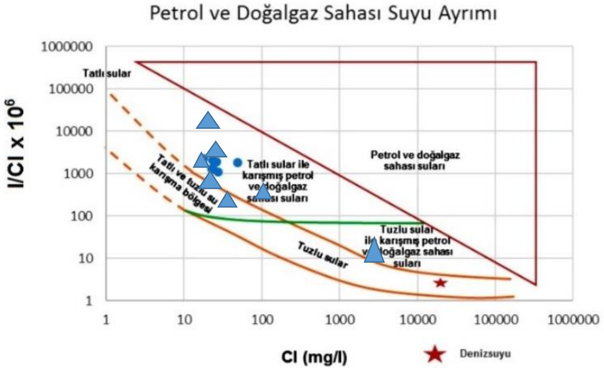
Şekil 3.3. Petrol ve doğalgaz sahası sularının I/Cl –Cl grafiğindeki yeri (Özdemir,2018)
