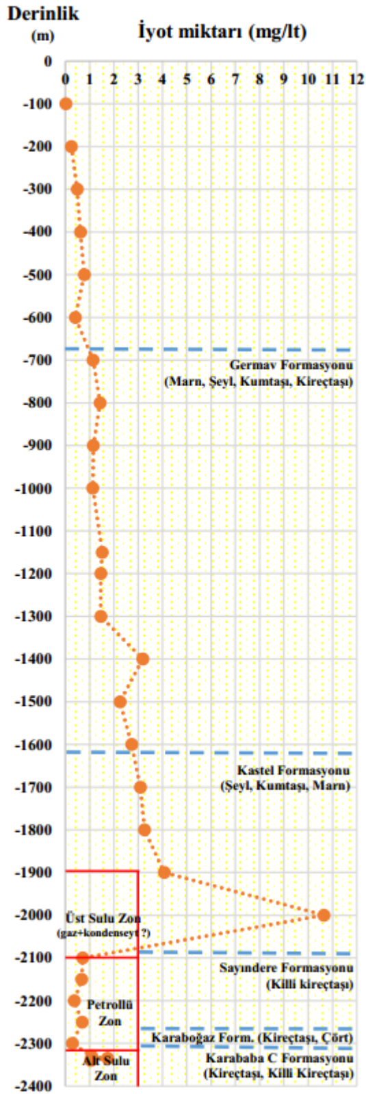
Şekil 2.21. Petrol sondajı esnasında sondaj çamurundan alınan iyot örneklerinin derinliğe bağlı dağılımı (Özdemir, 2018)
