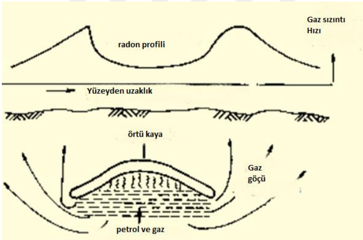
Şekil 2.15. Mikrosızıntı ve Radon anomali kesiti (Fernandez vd., 2015)
