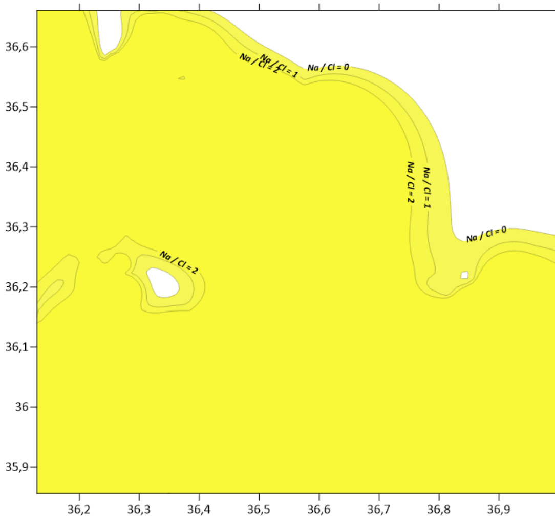
Şekil 3.7. Eş Na/Cl(epm) kontur haritası
