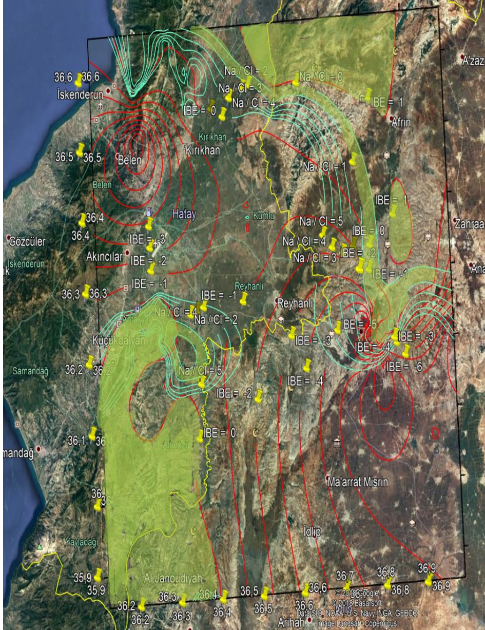
Şekil 3.8. Sulin ve Schoeller sınıflamalarının Google Earth üzerinde gösterimi
