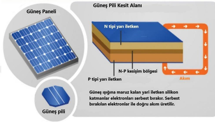
Şekil 1.4. Güneş Pilinin çalışma mekanizması
