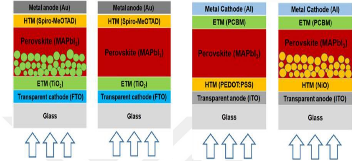
Şekil 1.10. Doğrudan perovskit güneş pillerinin mezogözenekli yapılar için ters modda perovskit güneş pillerinin genel şeması
