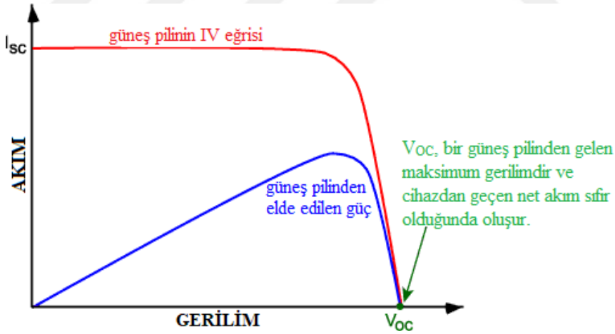
Şekil 2.6. Açık devre gerilimi, güneş pili I-V karakteristiği
