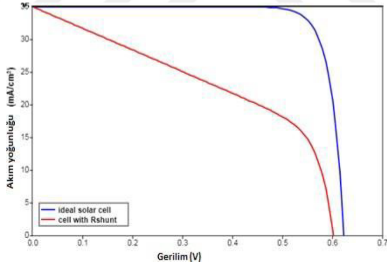
Şekil 2.9. Bir güneş pilinde şönt direncinin dolum faktörüne etkisi, hücre alanı 1cm 2 , T=300K, RSH=30 ohm.cm 2
