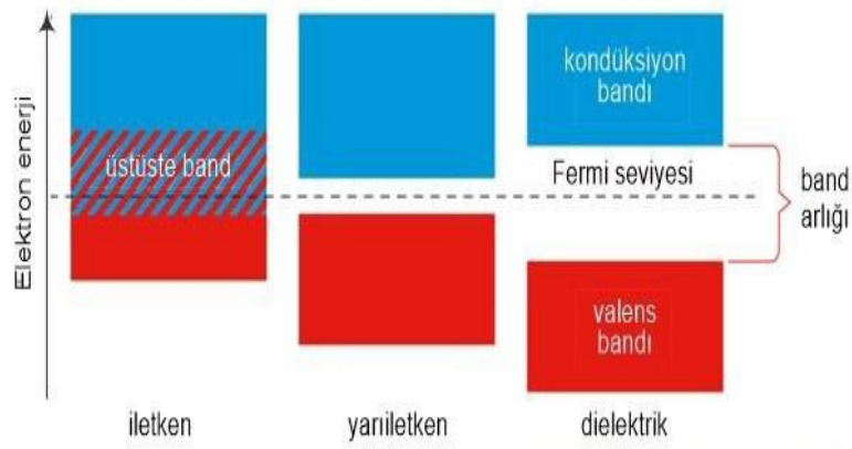
Şekil 1.5. Katı cisim bant teorisinin şeması
