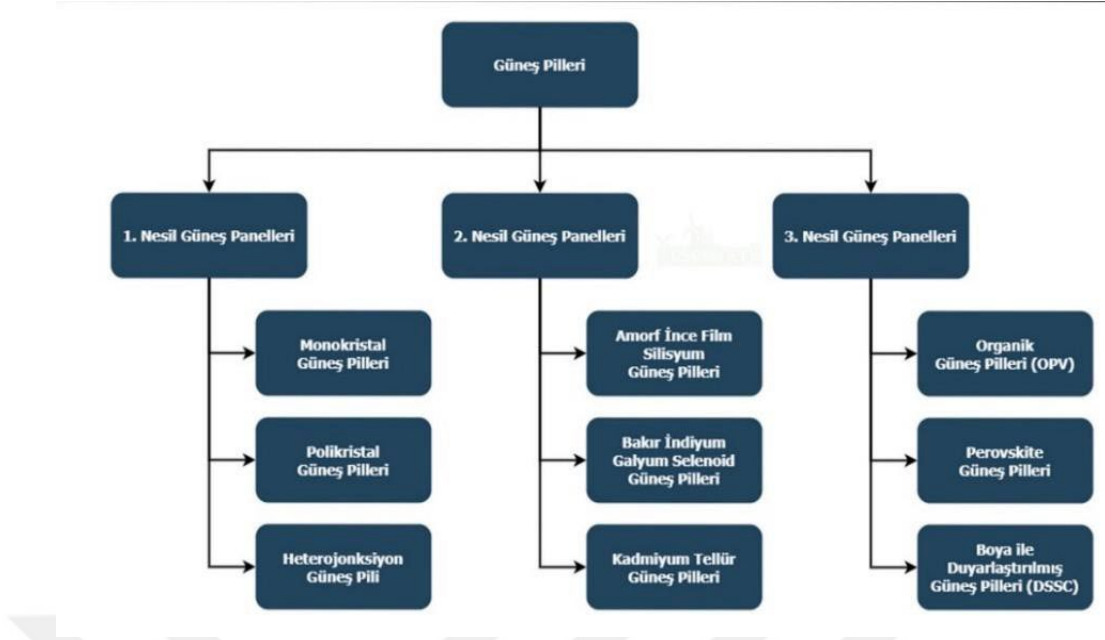
Şekil 1.7. Farklı nesil güneş pillerinin bölünmesinin ağaç diyagramı.
