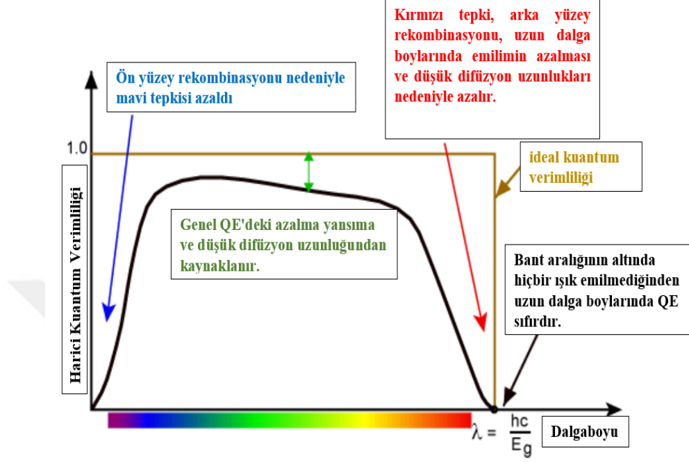
Şekil 2.11. Kuantum verimliliği örnek grafik
