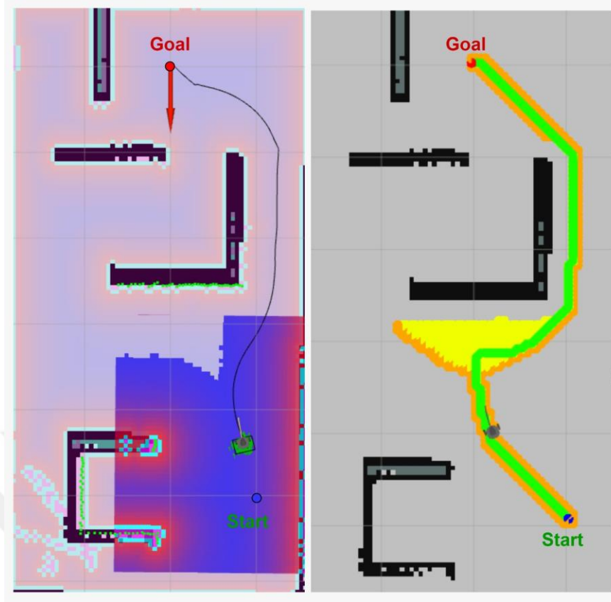
Şekil 6.2. (A) haritasında navigasyon – sol: DWA, sağ: A*.
