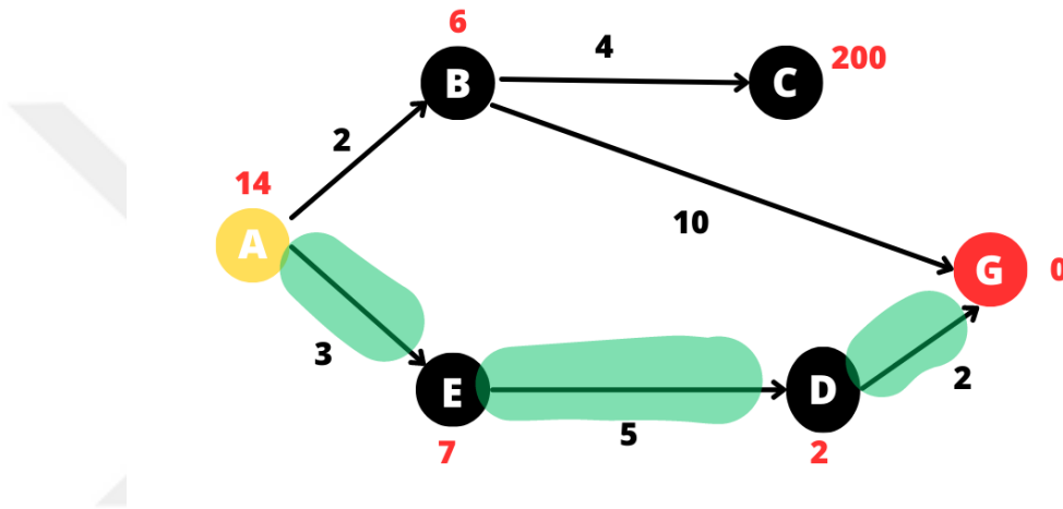
Şekil 3.11. A* ile en kısa yolu bulması.
