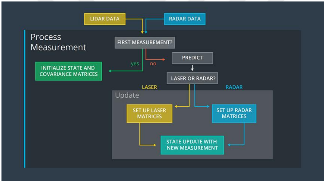
Şekil 3.8. Radar- LiDAR entegreli EKF için çalışma prensibi.
