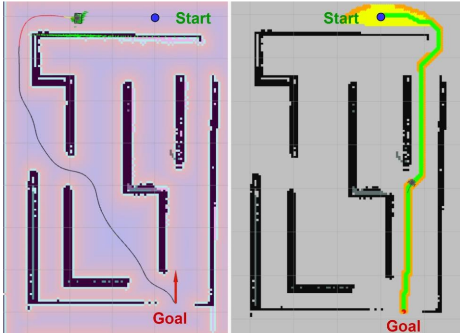
Şekil 6.3. (B) haritasında navigasyon – sol: DWA, sağ: A*.
