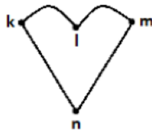
Şekil 3.1. Graf örneği
