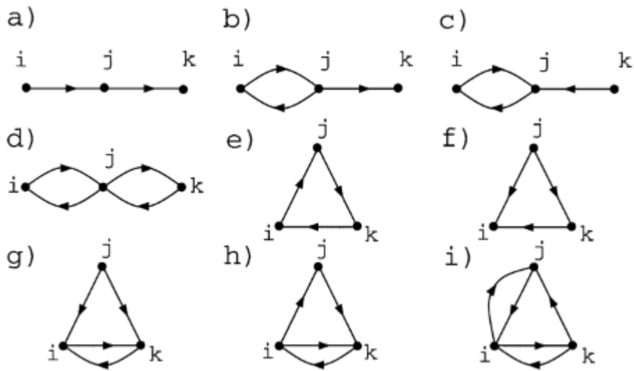
Şekil 4.5. Yasaklı konfigürasyonlar
