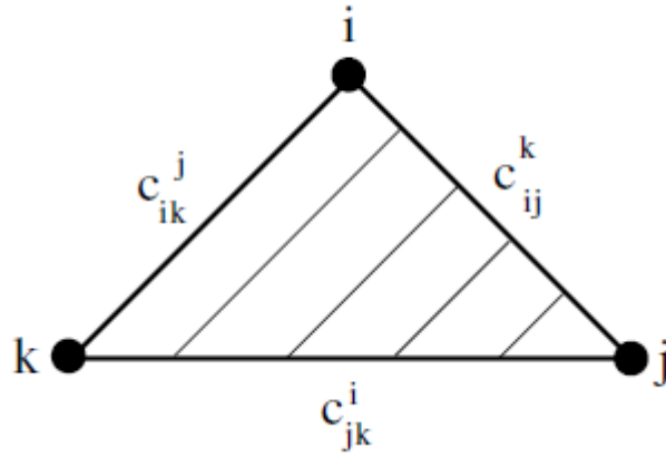
Şekil 4.4. Tam üçgen
