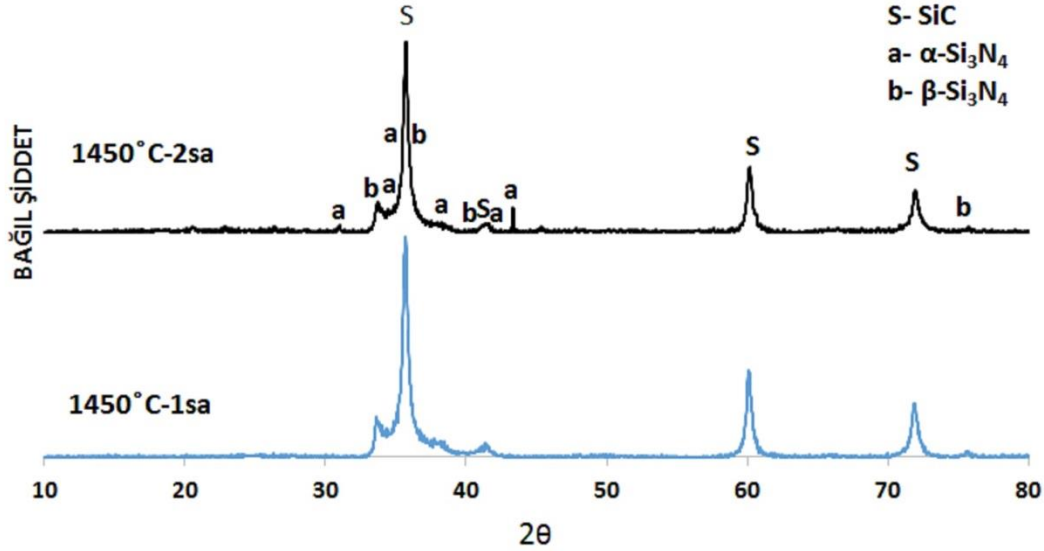
Şekil 6.10. 1450°C’de 1 ve 2 saat \text{N}_2 , 1500°C’de 1 saat Ar atmosferinde dinamik termokimyasal işlem sonrasında elde edilen XRD analizleri
