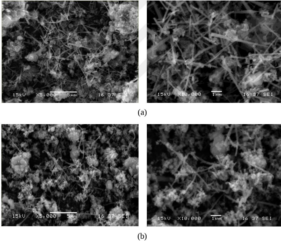
Şekil 6.16. 1500 °C'de 1 saat \text{N}_2 ve 1500 °C'de 1 saat Ar atmosferinde a) dinamik ve b) statik işlem sonucunda elde edilen ürünlerin SEM görüntüleri
