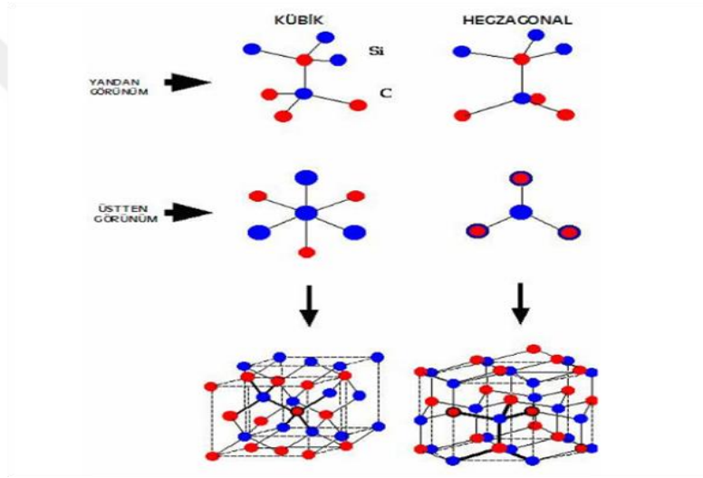
Şekil 3.4. kübik ve hegzagonal SiC yapısı
