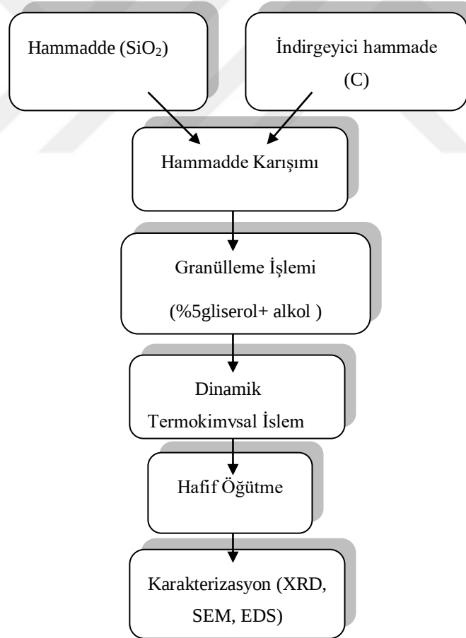
Şekil 5.2. Dinamik termokimyasal ile \text{Si}_3\text{N}_4/\text{SiC} toz üretim işlemlerinin iş akış şeması
