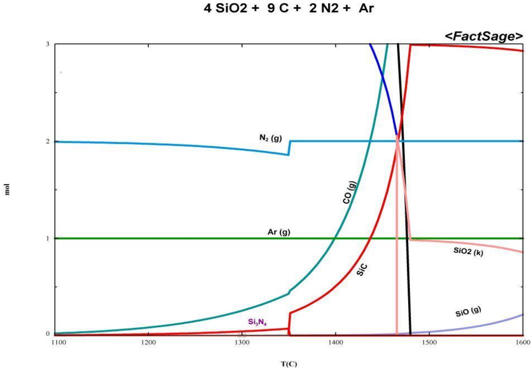
Şekil 6.2. 1 atm basınçta 4\text{SiO}_2+9\text{C} olan 1 mol Ar ve 2 mol \text{N}_2 gazı altındaki mol-sıcaklık grafiği (yakın)
