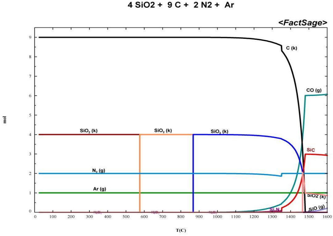
Şekil 6.1. 1 atm basınçta 4\text{SiO}_2+9\text{C} olan 1 mol Ar ve 2 mol \text{N}_2 gazı altındaki mol-sıcaklık grafiği
