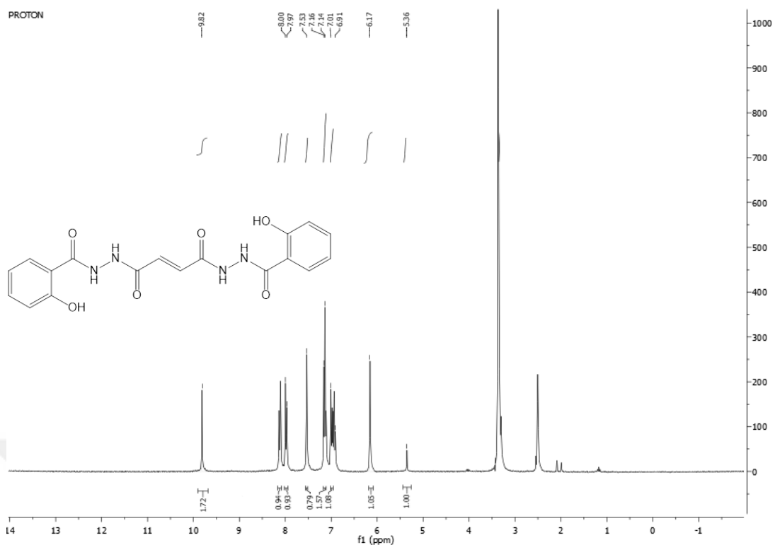
Şekil A.9. N'1,N'4-bis(2-hidroksibenzoil)fumarohidrazit (DSHM) ^1\text{H} NMR spektrumu (300 MHz, DMSO- \text{d}_6 ).
