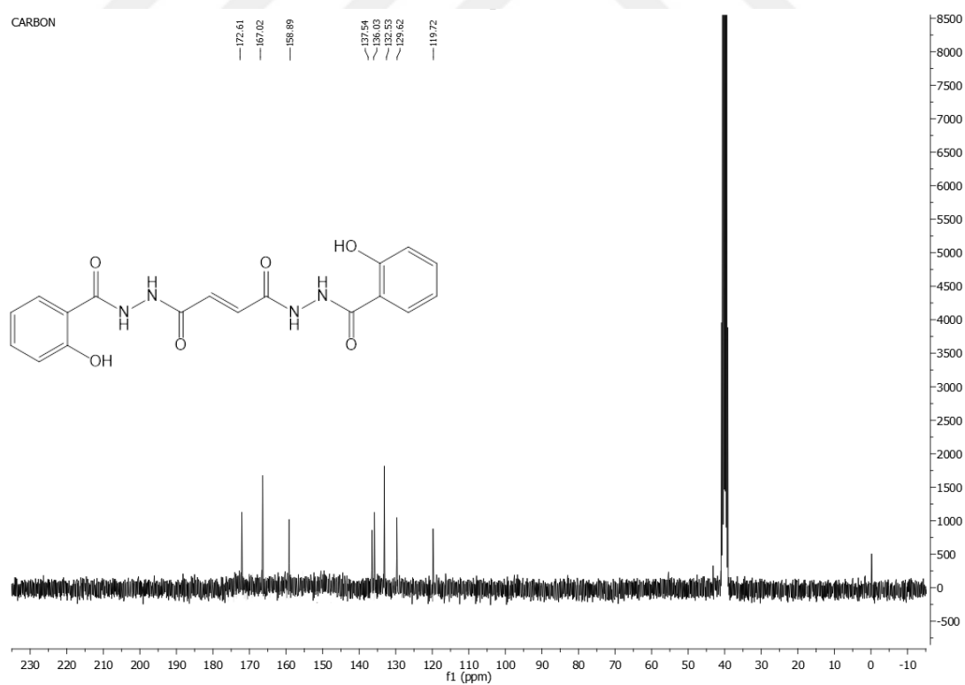
Şekil A.10. N'1,N'4-bis(2-hidroksibenzoil)fumarohidrazit (DSHM) ^{13}\text{C} NMR spektrumu (75 MHz, DMSO- \text{d}_6 ).
