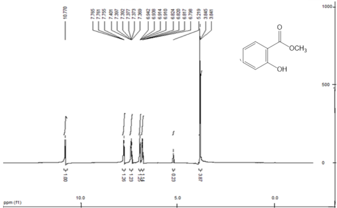
Şekil A.2. Metil salisilat (1)'in 1 H NMR spektrumu.
