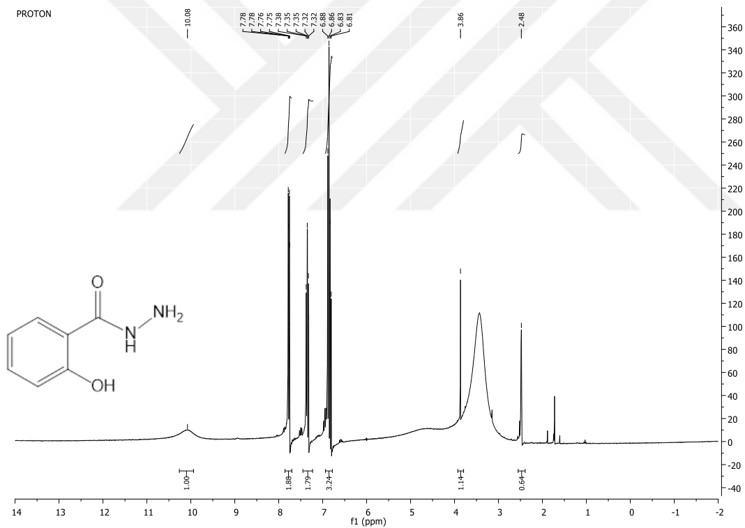
Şekil A.4. 2-hidroksibenzohidrazit (2)'in 1 H NMR spektrumu (300 MHz, DMSO-d 6 ).
