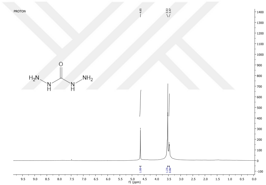
Şekil A.6. Karbohidrazit (3) (300 MHz, CDCl 3 ).
