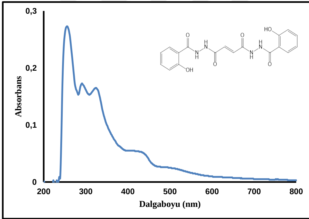
Şekil A.12. N'1,N'4-bis(2-hidroksibenzoil)fumarohidrazit (DSHM) UV-Vis spektrumu.
