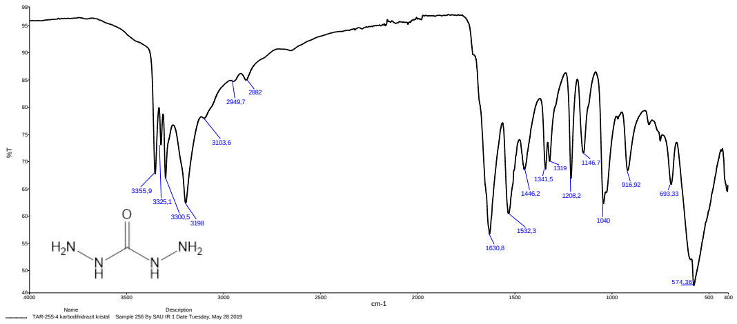
Şekil A.5 Karbohidrazit (3) FT-IR spektrumu.
