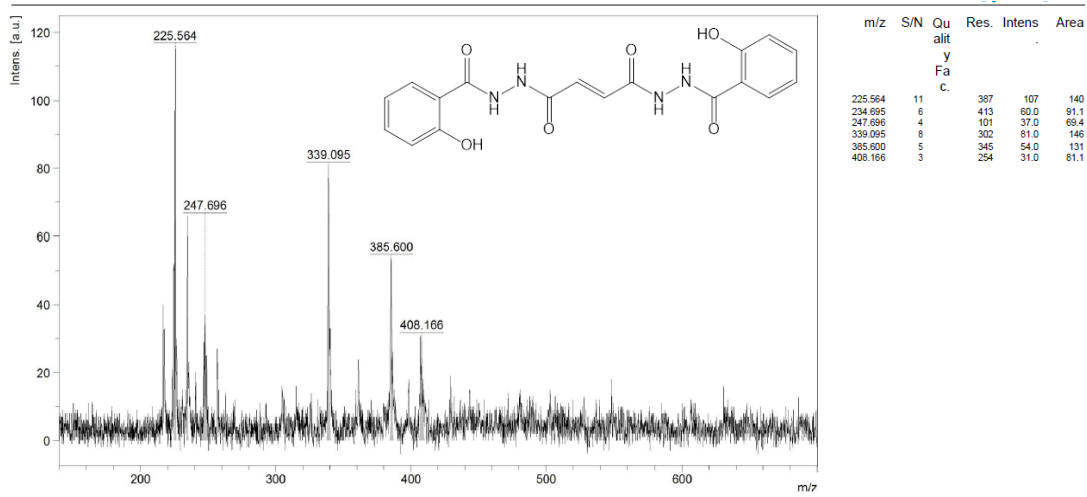
Şekil A.11. N'1,N'4-bis(2-hidroksibenzoil)fumarohidrazit (DSHM) kütle spektrumu.
