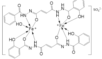
Ekil A.18. N'1,N'4-bis(2-hidroksibenzoil)fumarohidrazit demir kompleksi (Fe) FT-IR spektrumu.
