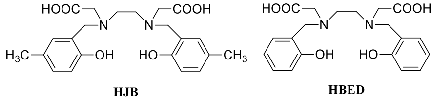
Şekil 2.5. HJB ve HBED ligandlarının molekül yapıları.
