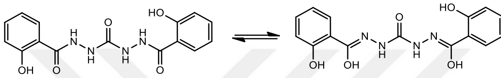
Şekil 4.2. KDHDS ligandının enol-keto tautomerisi.
