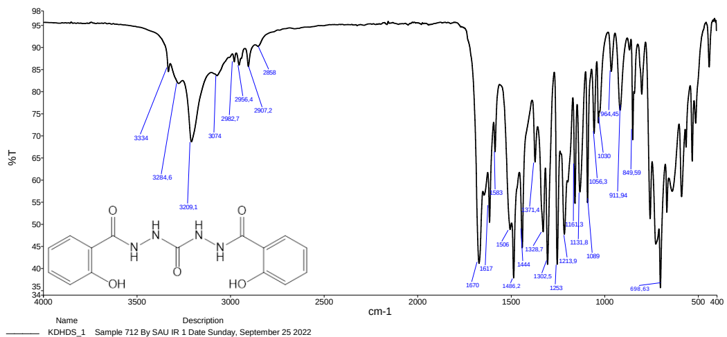
Şekil A.13. N,N''-bis(2-hidroksibenzoil)metanedihidrazit (KDHDS) FT-IR spektrumu.
