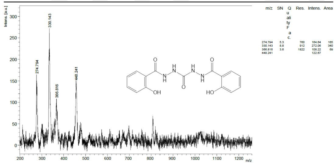
Şekil A.16. N,N''-bis(2-hidroksibenzoil)metanediidrazit (KDHDS) kütle spektrumu.
