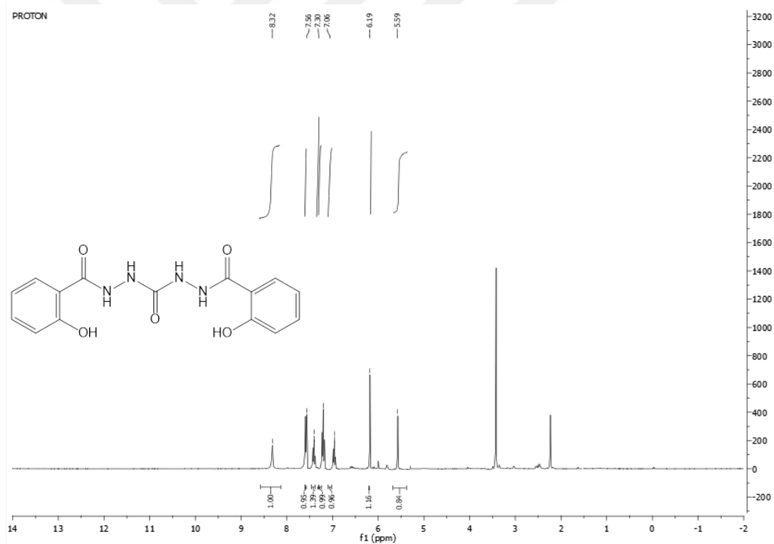
Şekil A.14. N,N''-bis(2-hidroksibenzoil)metanedihidrazit (KDHDS) ^1\text{H} NMR spektrumu (300 MHz, \text{CDCl}_3 ).
