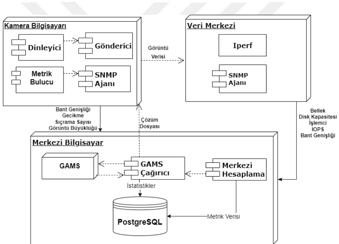
Şekil 5.1. Bileşen diyagramı
