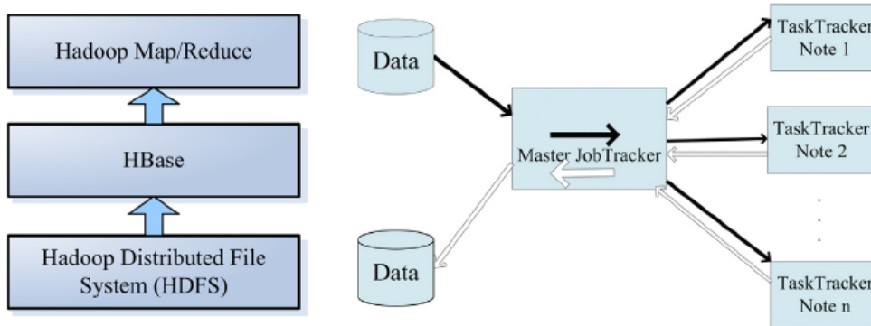
Şekil 3.12. Hadoop ekosistemi
