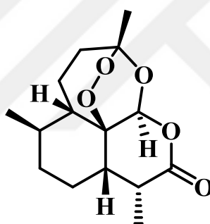
Artemisinin 4
