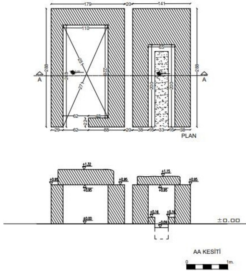
M23-M24 Plan Kesit Çizimleri
