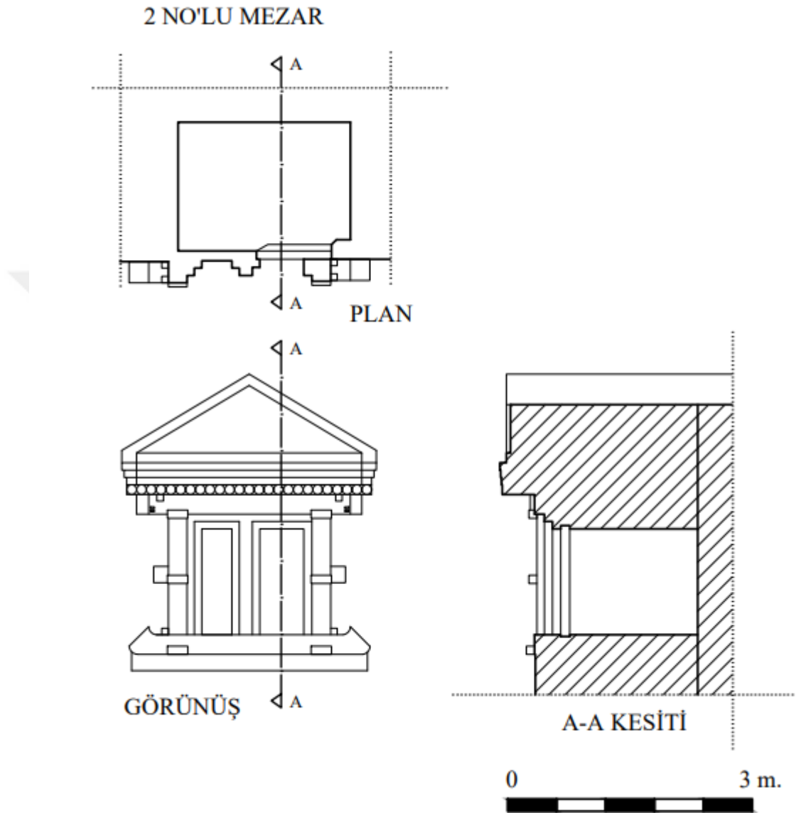
KM2 Plan Kesit Çizim
