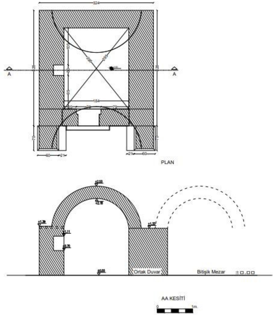
M22 Plan Kesit Çizimleri
