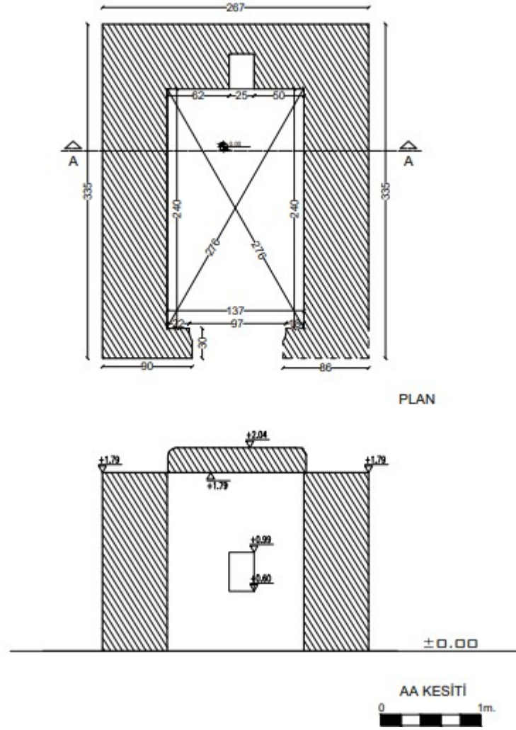
M25 Plan Kesit Çizimleri
