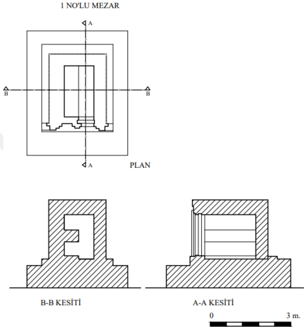
KM1 Plan Kesit Çizim
