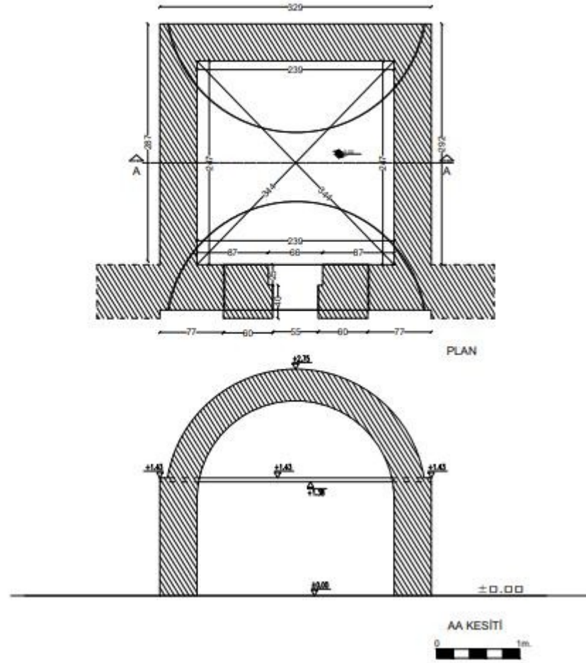
M09 plan kesit çizim
