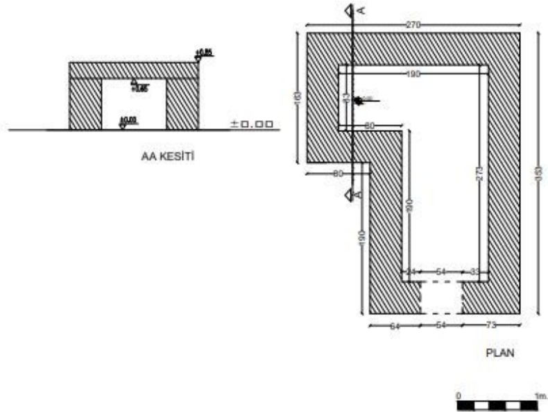
M123 Plan Kesit Çizimi
