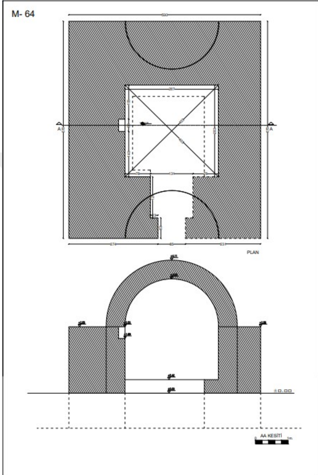
M64 Plan Kesit Çizimleri
