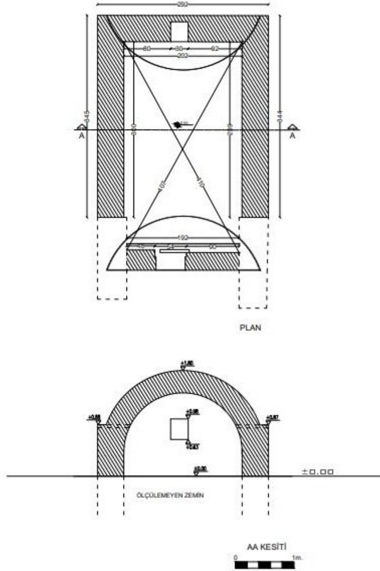
M08 plan kesit çizim
