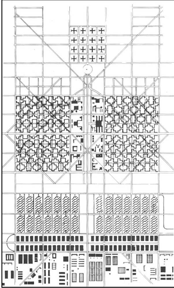
Resim 3.3. Radiant City ( Ville Radieuse ), 1931, Le Corbusier ve Jeanneret; koşt bantlarda bölgelemeyi gösteren plan [Frampton, 1992]
