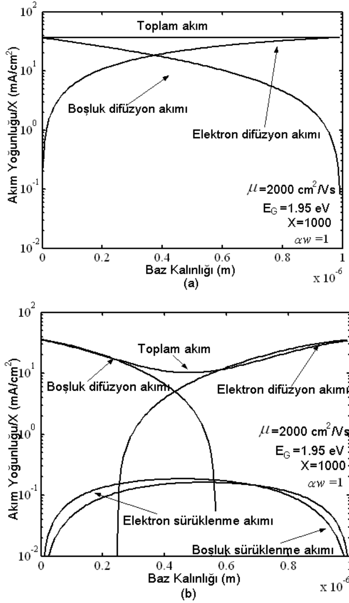
Şekil 4.30. E_G=1,95 \text{ eV} için \alpha w=1 'de elektrik alanın/sürüklenme akımının ihmal (a) ve dahil (b) edilmesi halinde difüzyon ve toplam akım yoğunluklarının baz bölgesi boyunca değişimi
