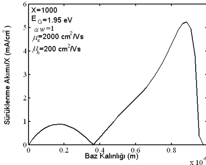
Şekil 4.36. E_G=1,95 eV için, \mu_e=2000 cm 2 /V ve \mu_h=200 cm 2 /V durumunda, sürüklenme akımının baz bölgesi boyunca değişimi
