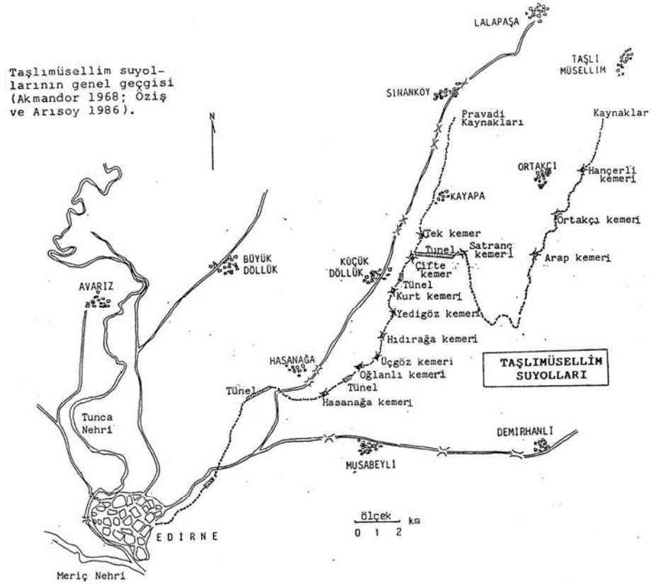
Şekil 3: Taşlı Müsellim Su Yolları Genel Geçgisi (Öziş-Arısoy'dan)
