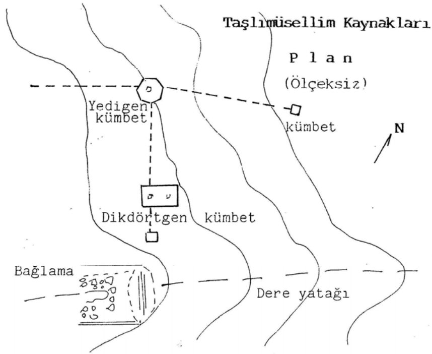
Şekil 2: Taşlı Müsellim Su Kaynakları Yerleşim Krokisi (Öziş'ten)
