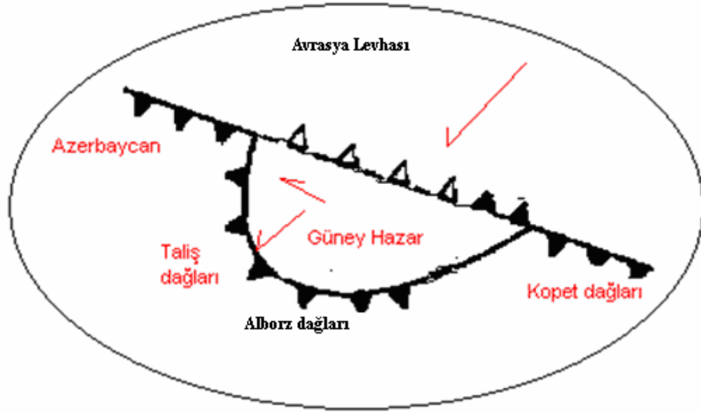
Şekil 2. 3 Hazar mikrolvhası
