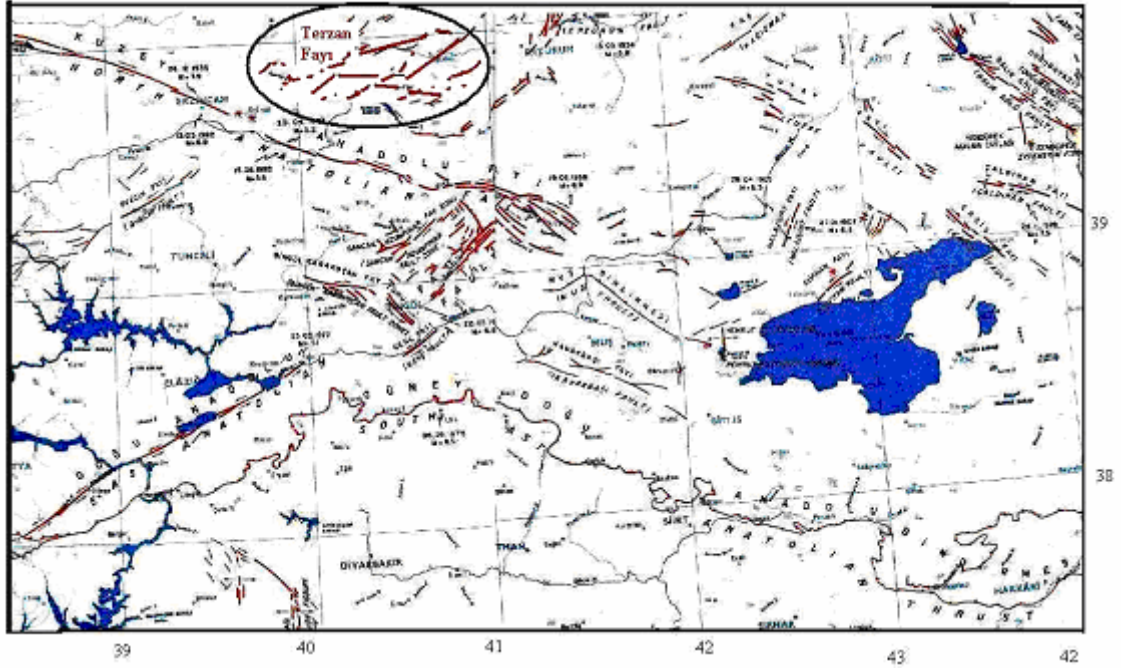
Şekil 2.42 Tercan-Aşkale fay zone
