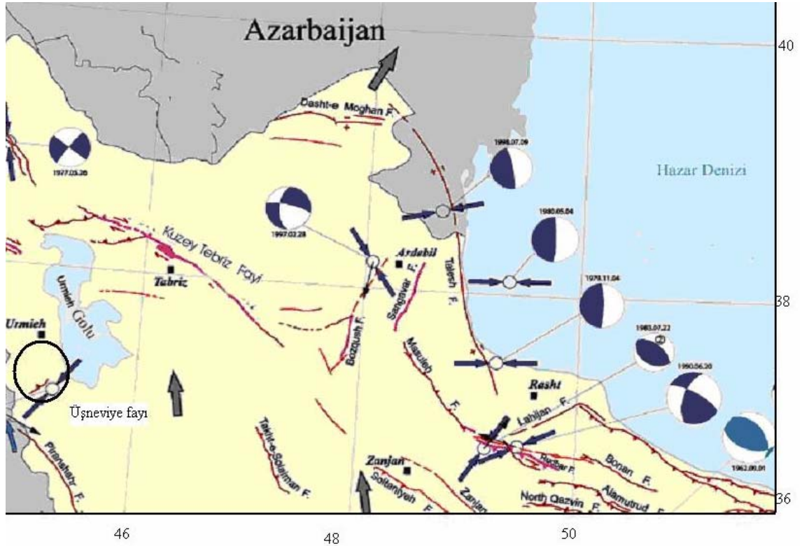
Şekil 2.10. Üşneviye fayı
