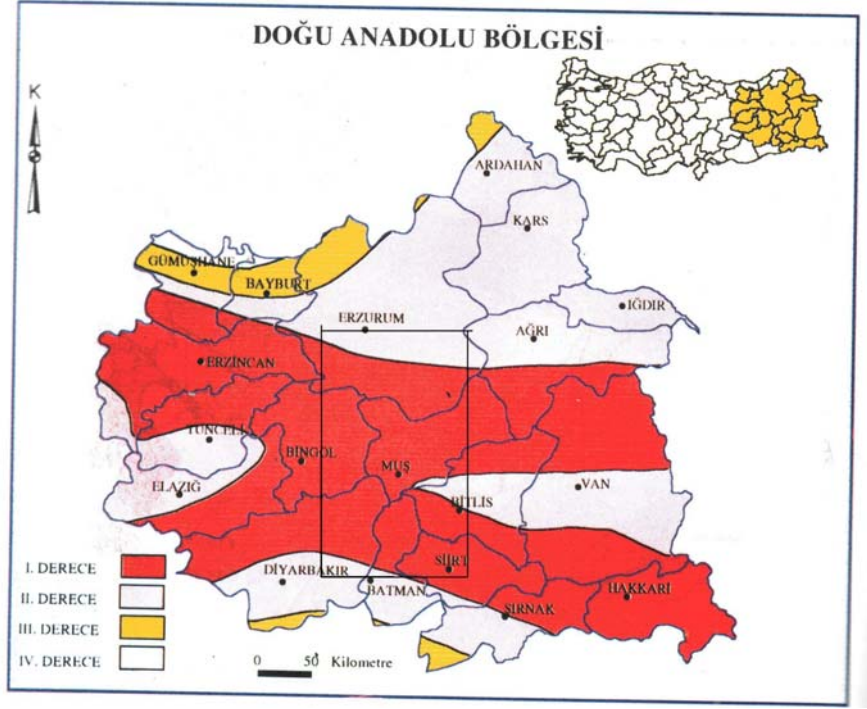
Şekil 4.34 Doğu Anadolu’nun orta zon
