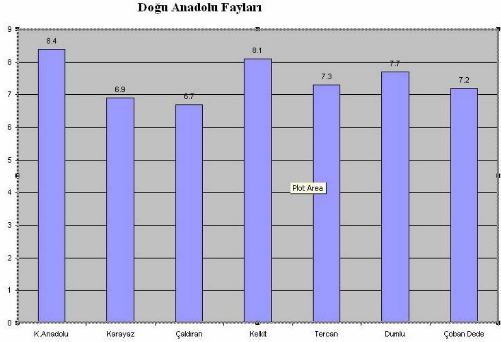
Şekil 4.20. Doğu Anadolu'nun büyük faylarının maksimum üretebileceği büyüklük
