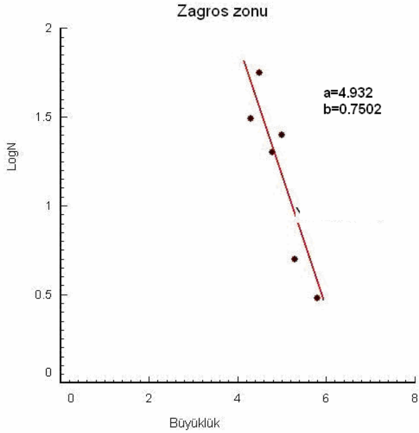
Şekil 4.24 Zagros Zonunda M-LogN ilişkileri ve eğrisi
