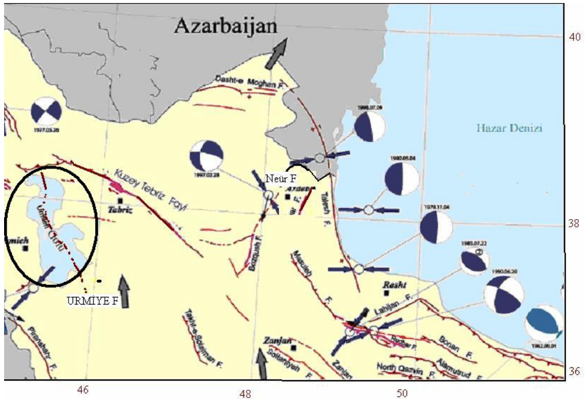
Şekil2.8 Urmیه gölü fay hattı
