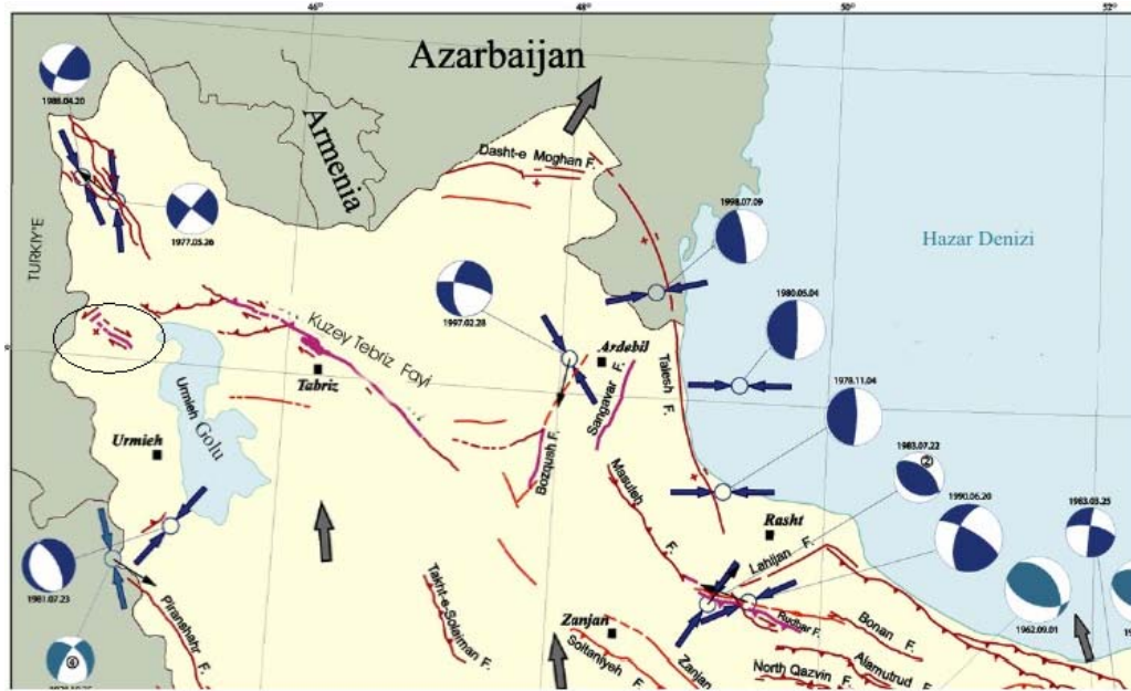
Şekil 4.29 Hoy-Salmas zonu
