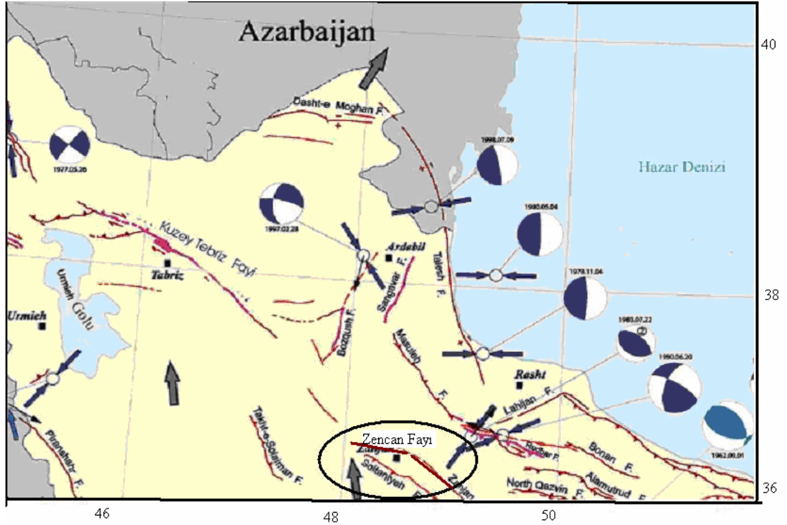
Şekil 2.17 Zencan fayı
