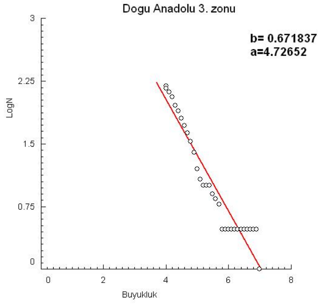
Şekil 4.37 Doğu Anadolu'nun Doğu zonuu M-LogN ilişkileri
