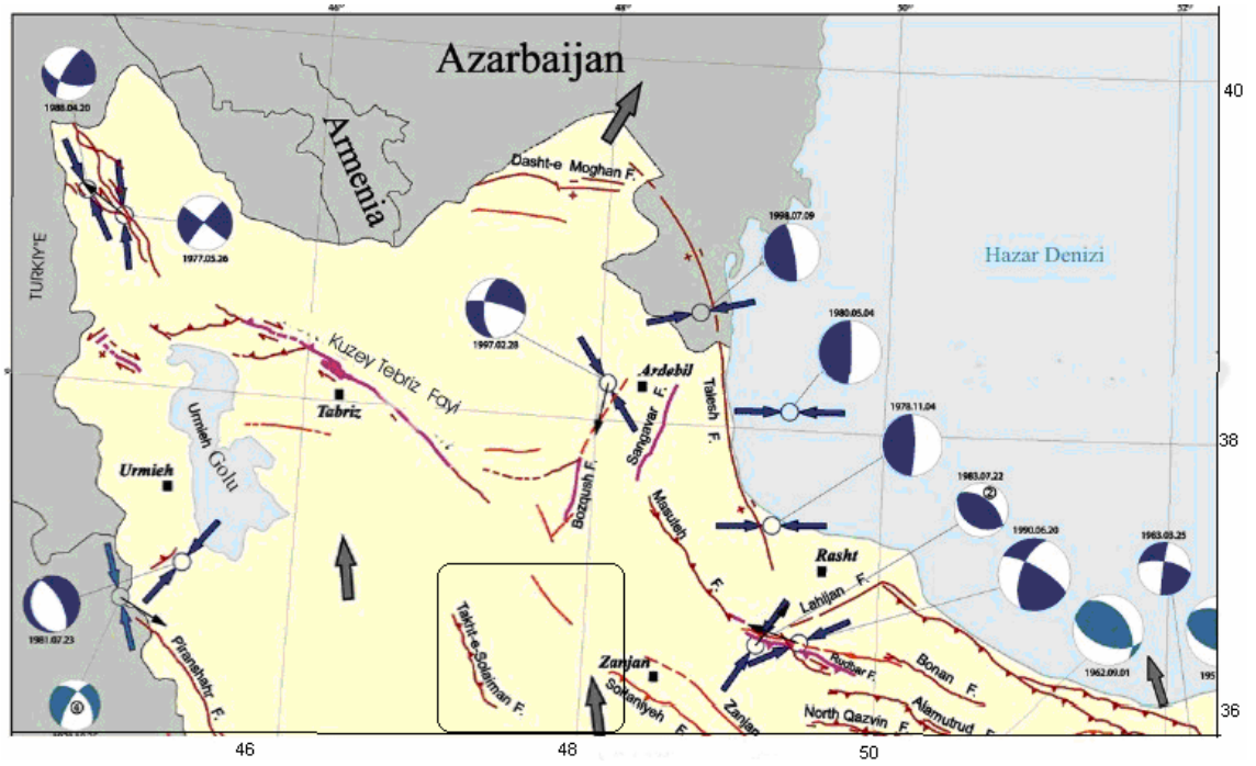
Şekil 4.23 Zagros zonu
