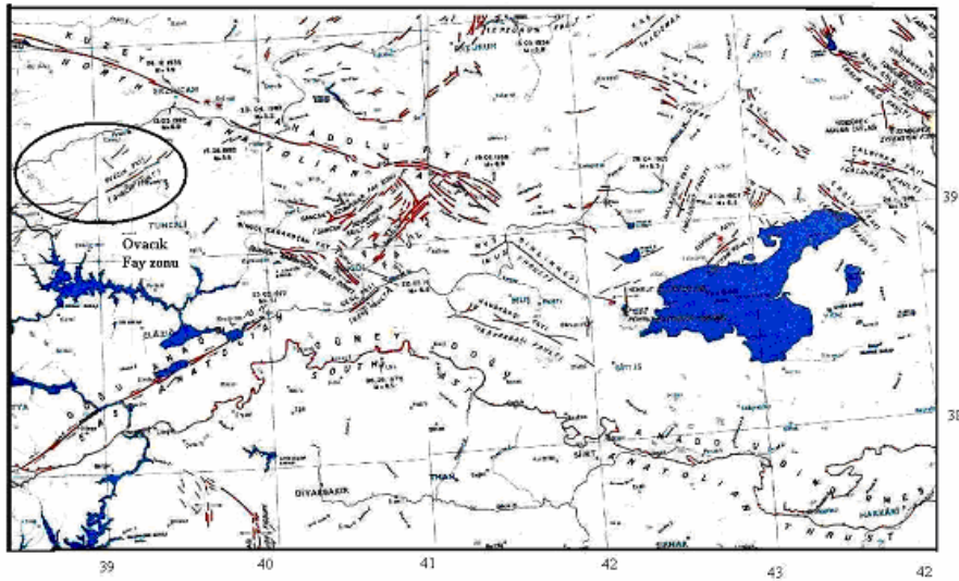
Şekil 2.44 Ovacık fay zone
