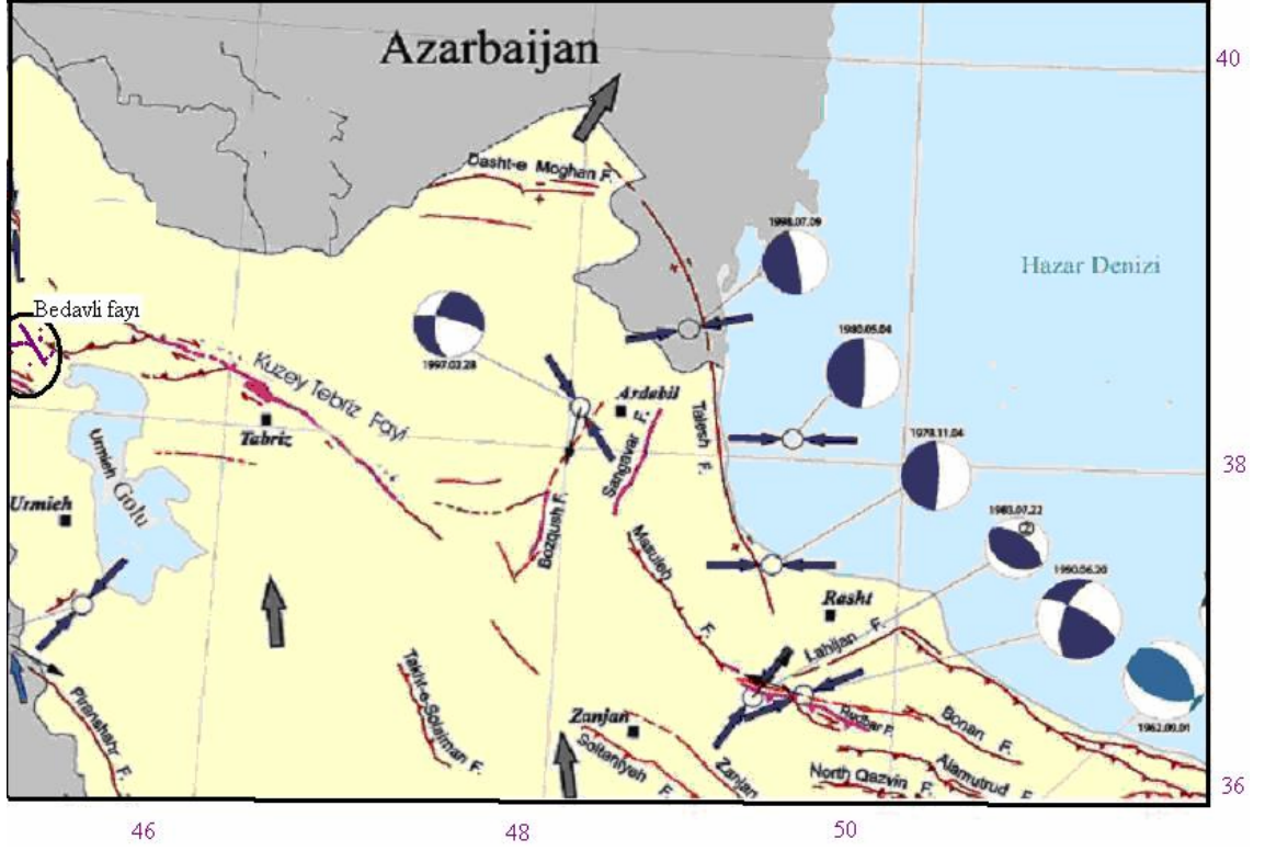
Şekil 2.12 Bedavlı fayı
