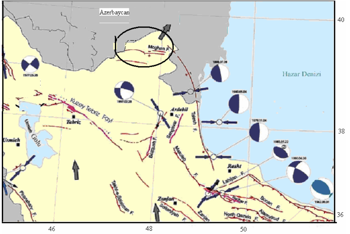
Şekil 2.22 Moğan fayı
