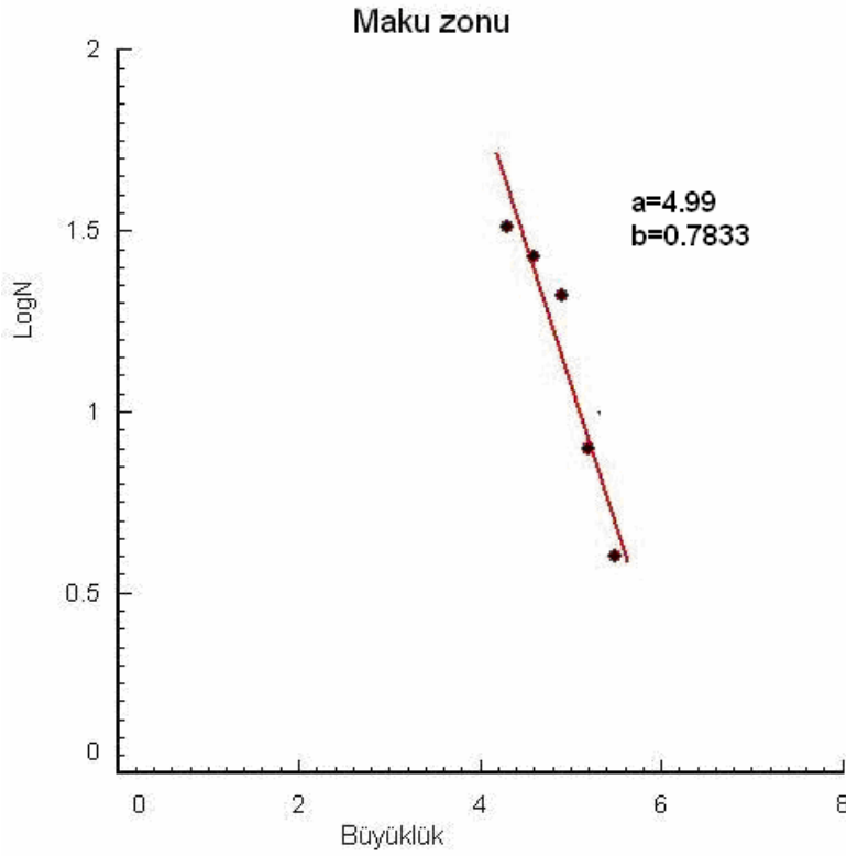
Şekil 4.28 Makı zonunda M-LogN ilişkileri
