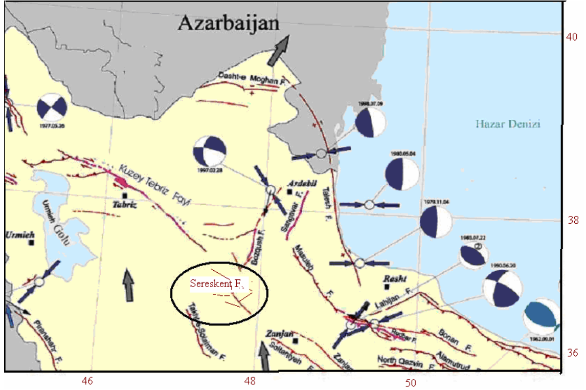
Şekil 2.18 Sereskent fayı
