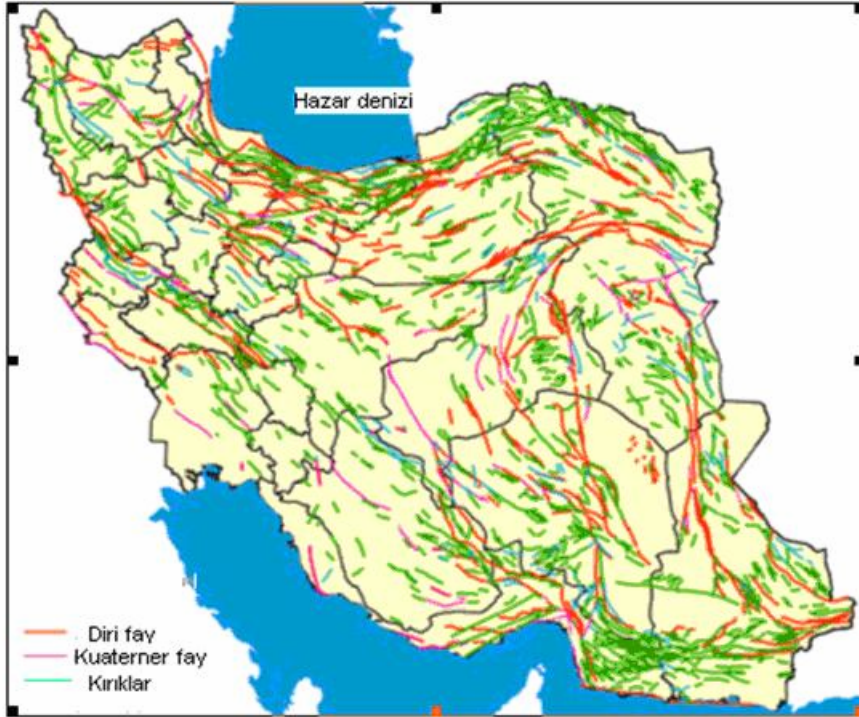
Şekil 2.5 İran faylarının genel haritası
