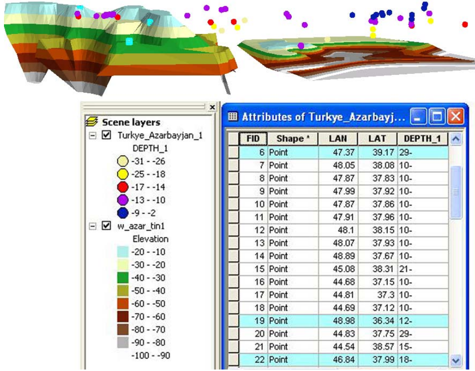
Şekil 4.14 Azerbaycan ve Doğu Anadolu'daki kabuk -deprem derinliğinin İncelenmesi ve karşılaştırılması
