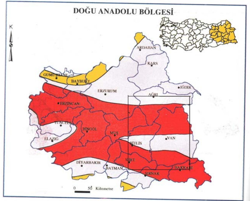
Şekil 4.36 Doğu Anadolu'nun Doğu zonu
