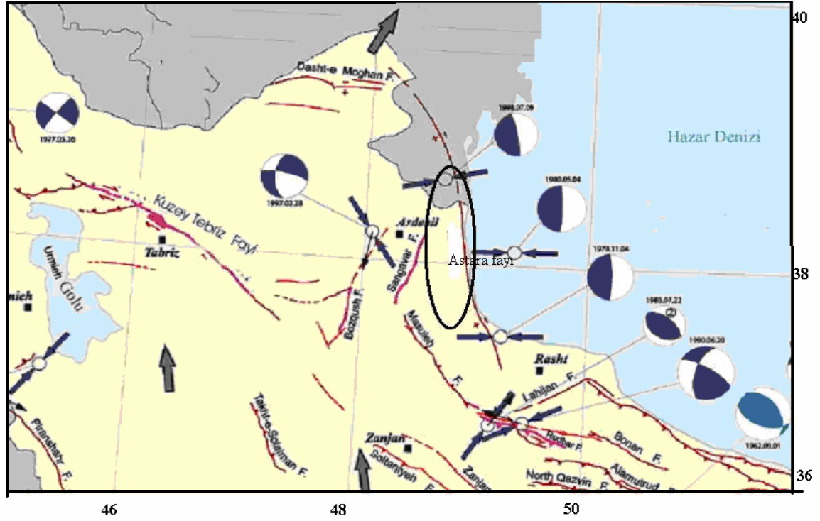
Şekil 2.6 Astara fayı
