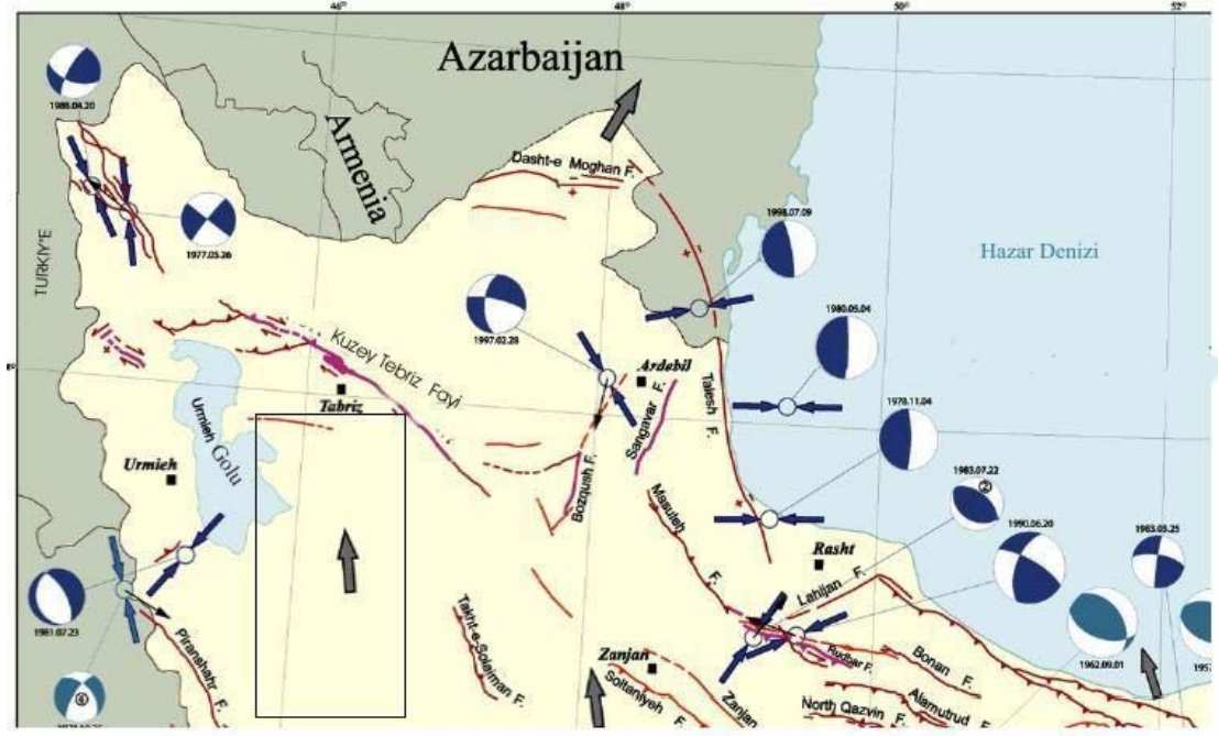
Şekil 4.21 Orta Azerbaycan Zonu
