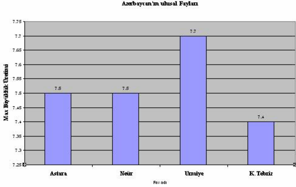
Şekil 4.19 Azerbaycan faylarının maksimum üretebileceği büyüklükler
