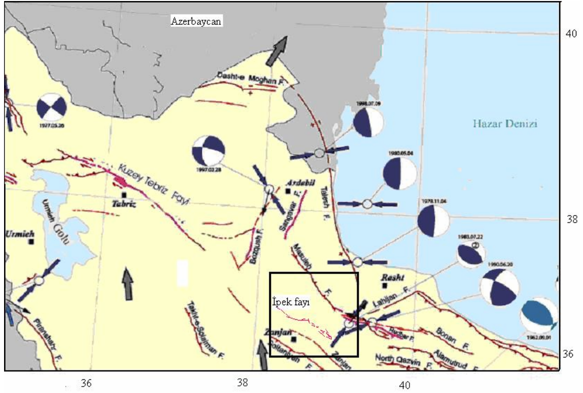
Şekil 2.11. İpek fayı
