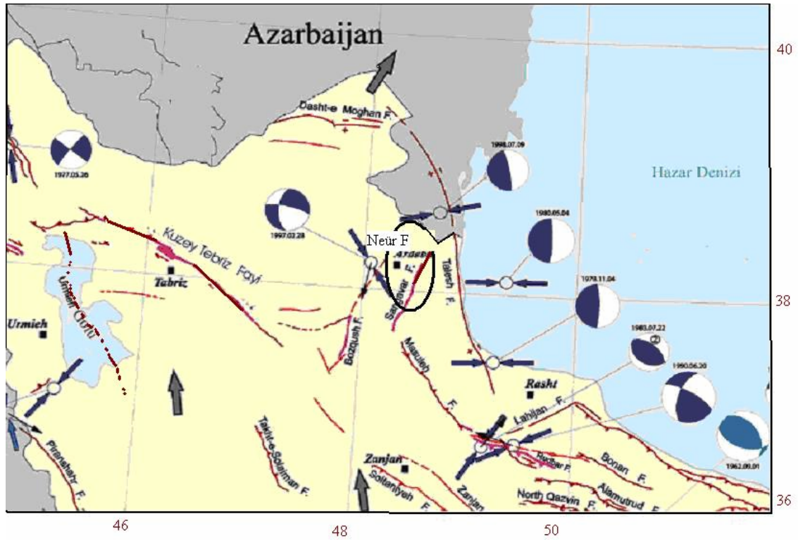
Şekil 2.7 Neür Fayı
