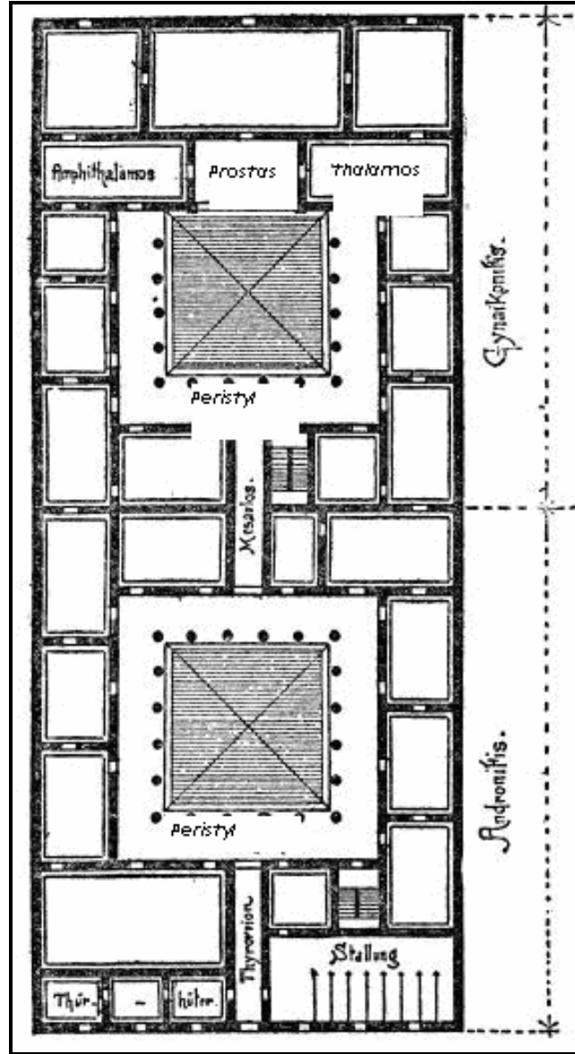
Vitruvius'a Göre Yunan Evi Planı.
