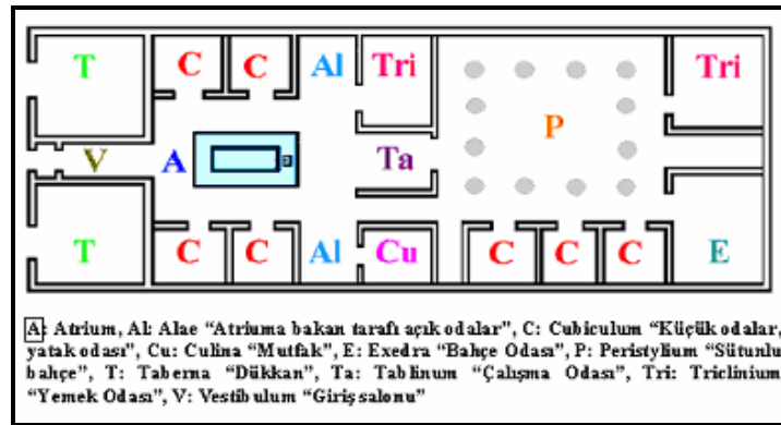
c- Domus Kent Evi Planı.
