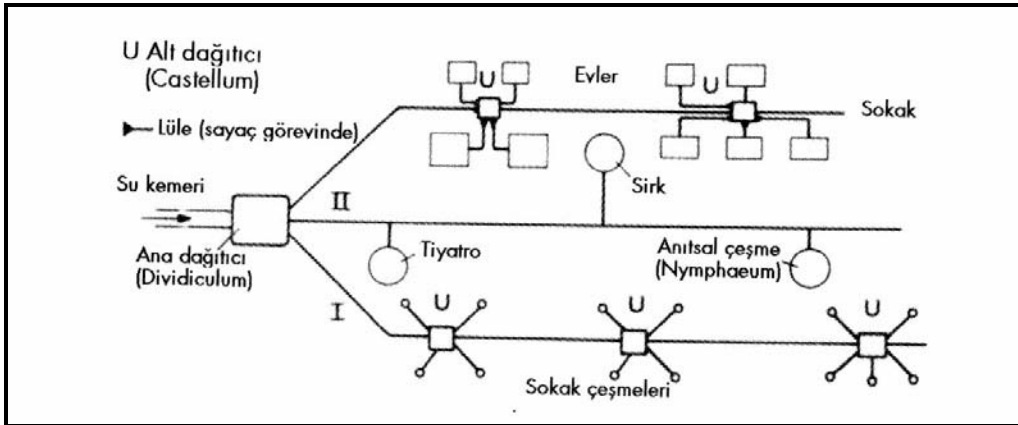
d-Antikçağ Roma Su Dağılım Şeması.
