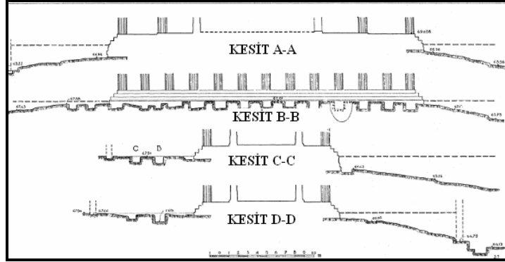
a- Hephaistos Tapınağı'nın Güney Bahçesinin Kesiti.
