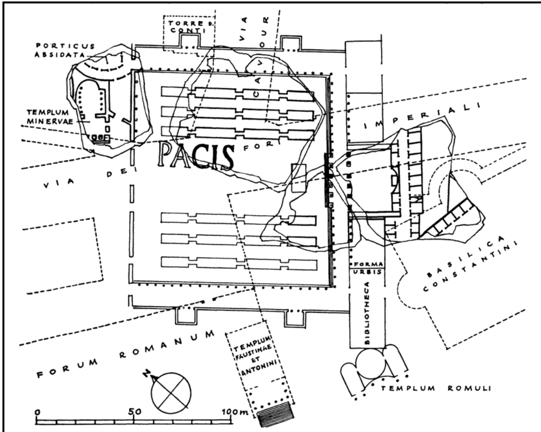
b- Peace Forumunun Rekonstrüksiyon Çizimi.
