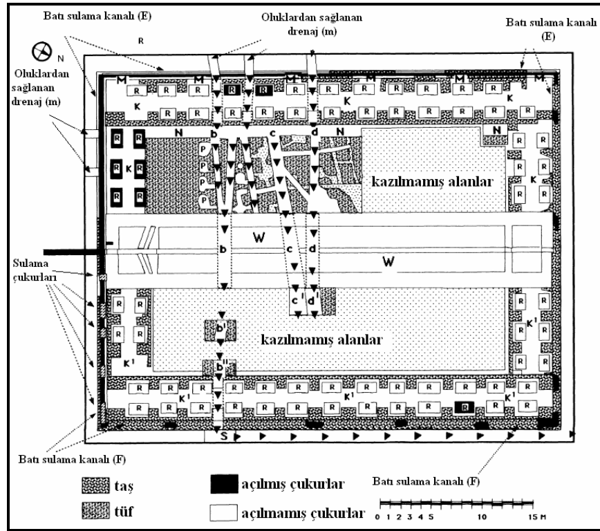
a-Hadrian Villasının Piazza D'oro Bölümünün Bahçesinin Planı.
