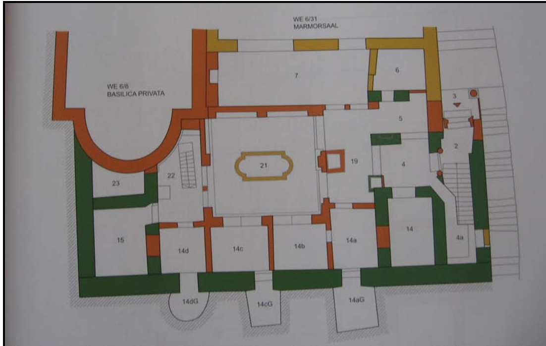
b- Efes Yamaç Evi 2/21 nolu Atrium Planı.
