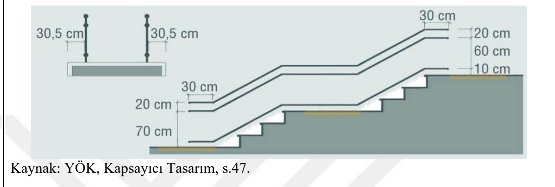
Şekil 6: Korkuluk, Tırabzan ve Tutamak Standartları
