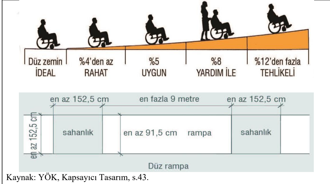
Şekil 3: Rampa Standartları
