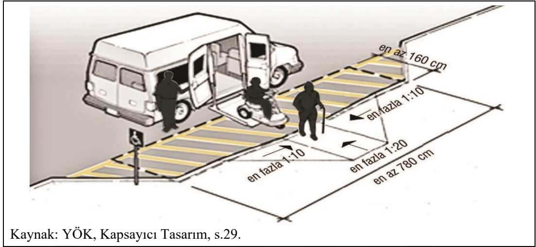
Şekil 1: Yolcu İndirme-Bindirme Alanlarının Standartları
