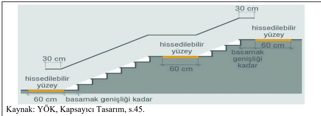
Şekil 5: Merdiven Standartları
