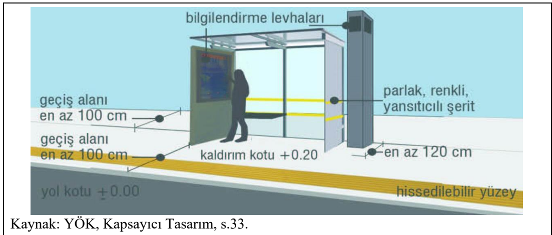
Şekil 2: Durak Standartları
