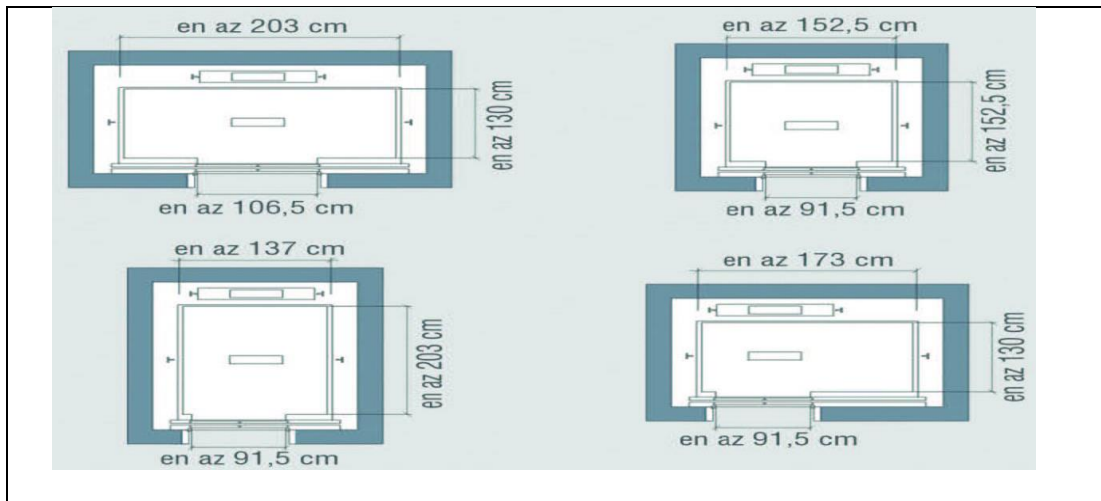
Şekil 7: Asansör Standartları
