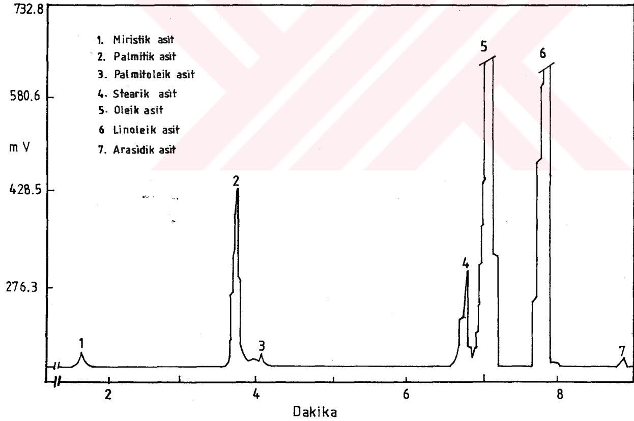
Şekil 2. Gaz kromatografisinde yağ asitlerinin ayrışımı
