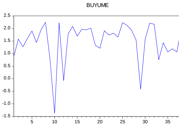
Şekil 6. Büyüme Durağanlık Grafiği
