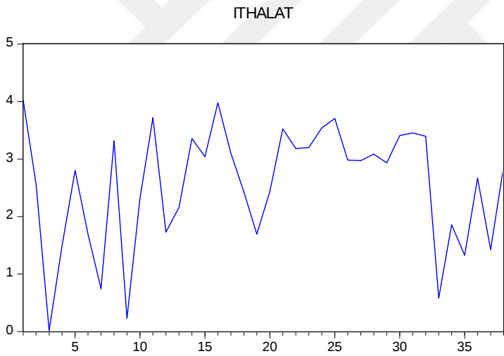
Şekil 8. İthalat Durağanlık Grafiği
