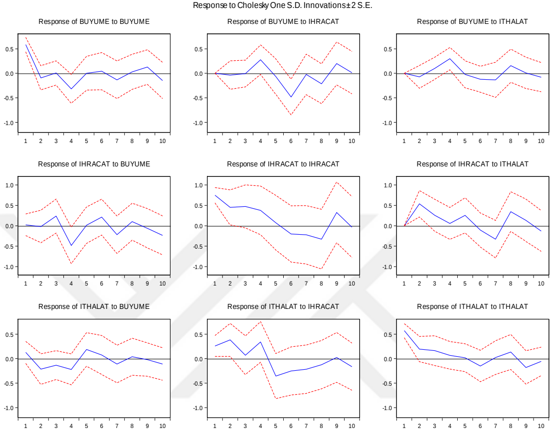
Şekil 10. Etki-Tepki Analiz Sonuçları
