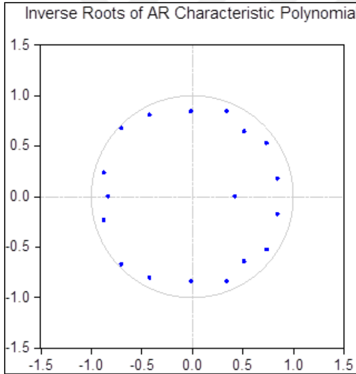
Şekil 9. AR Karakteristik Polinomu
