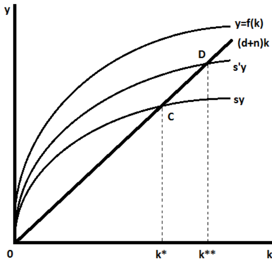
Şekil 4. Durağan Durum Dengesi
