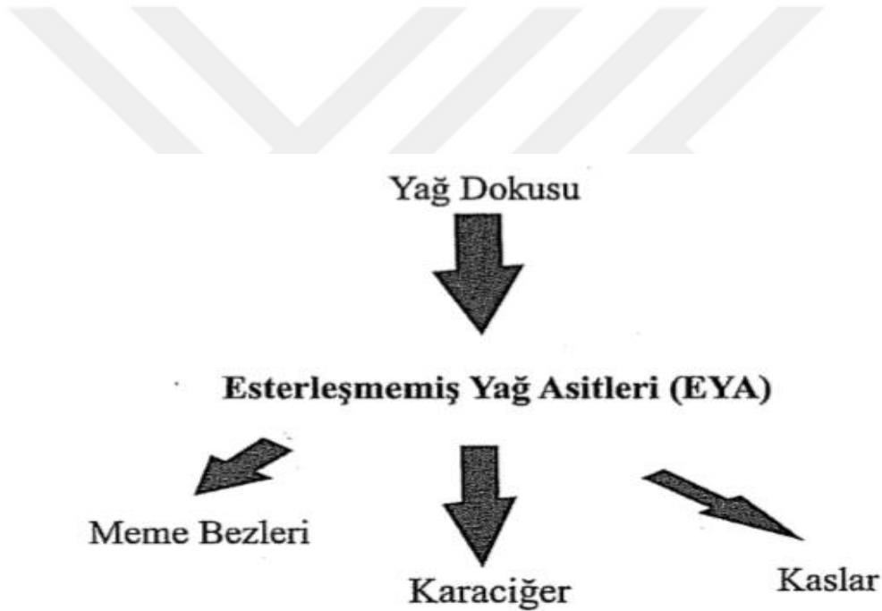
Şekil.5 Esterleşmemiş yağ asitlerinin metabolizması
