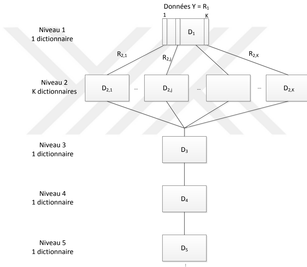
FIGURE 3.6 – La structure en “cerf-volant” (exemple de paramétrage imposant une fermeture après le deuxième niveau).
