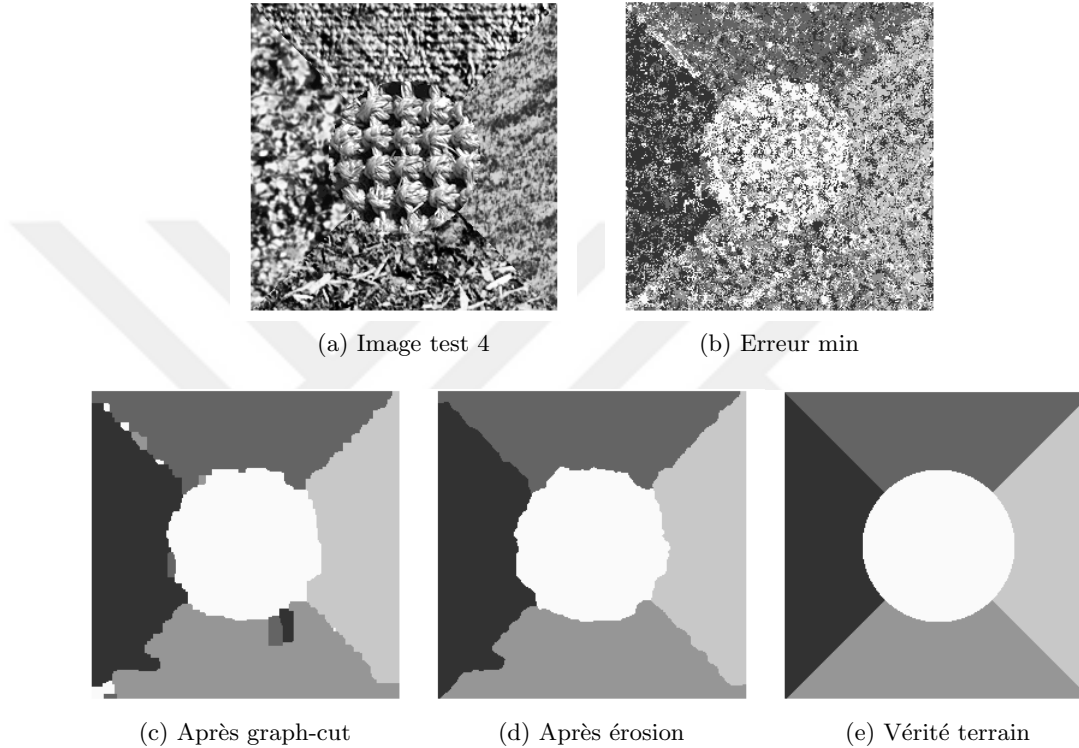
FIGURE 6.2 – Image test 4 aux différentes étapes de l'algorithme de classification/segmentation.
