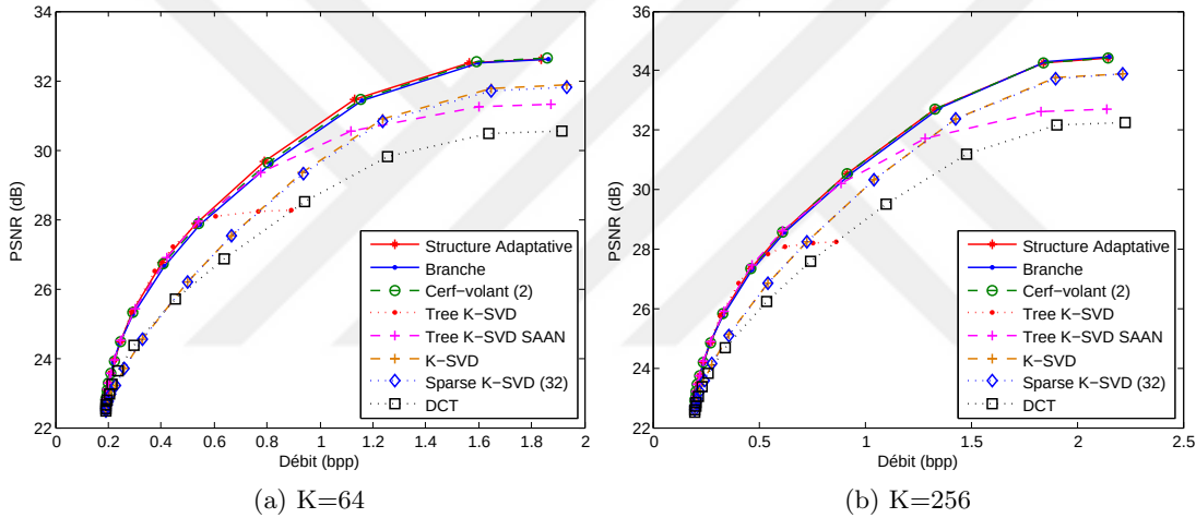
FIGURE 4.1 – Performances de codage des différentes structures de dictionnaires pour K=64 et K=256 sur New York .
