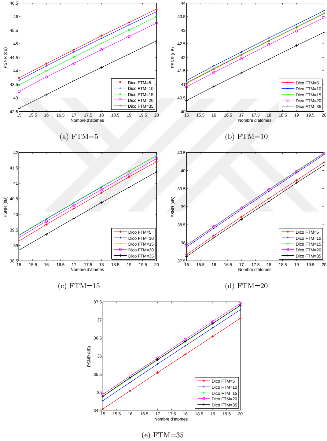
FIGURE 5.3 – Tests sur New York .
