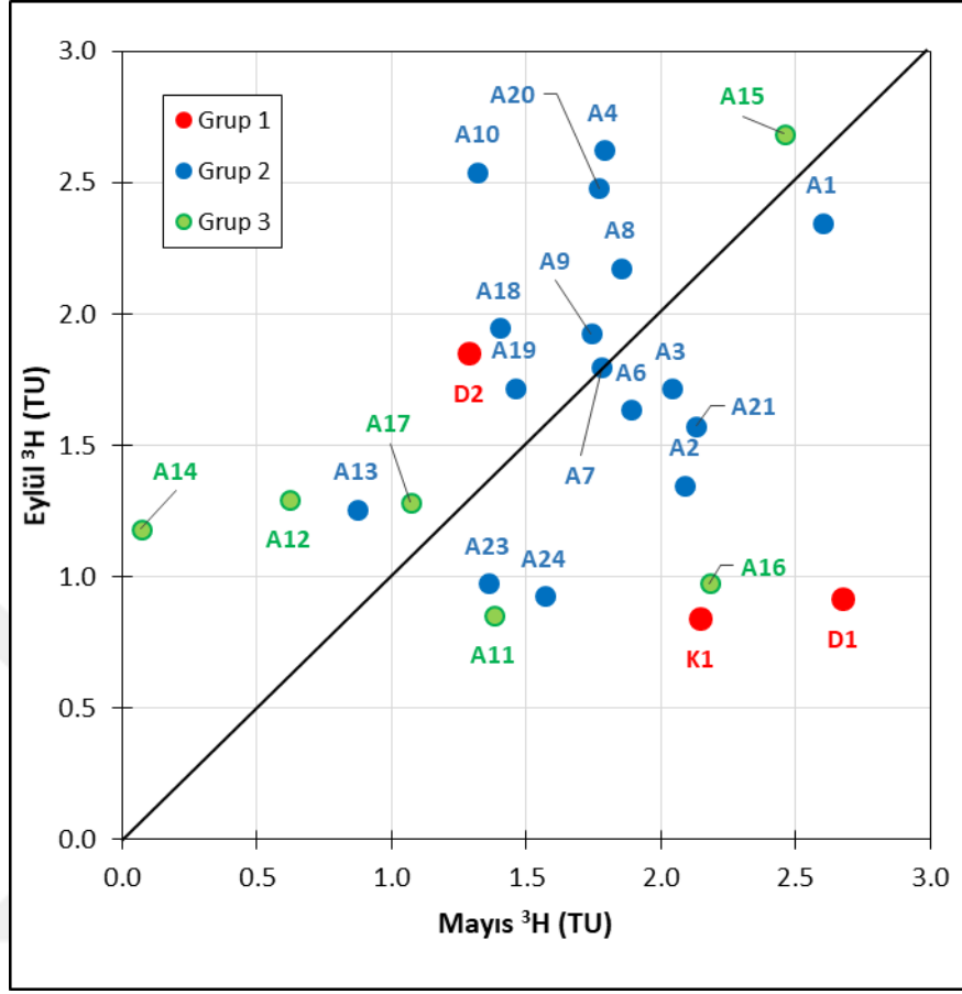
Şekil 4.20. ^3\text{H} içeriklerinin Mayıs ve Eylül dönemlerinde değişimi.
