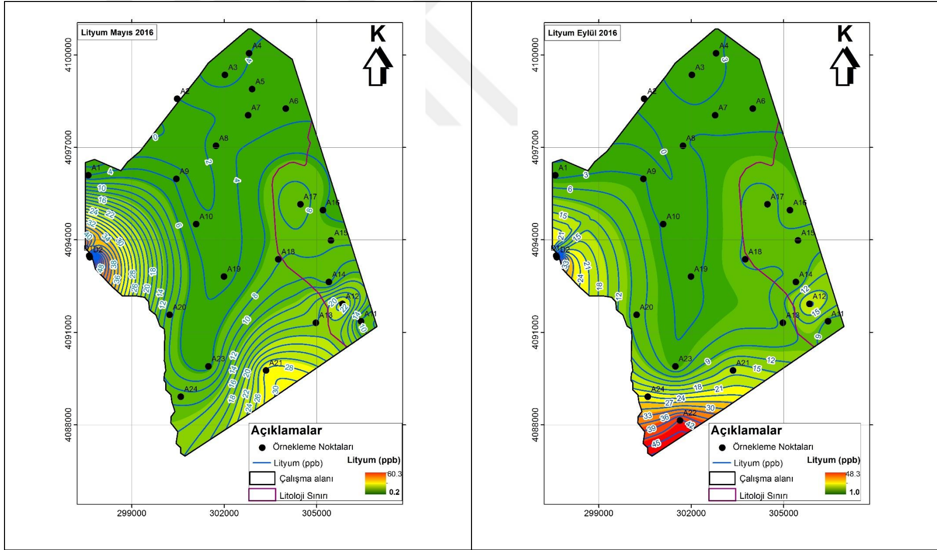
Şekil 4.15. Çalışma alanında Li derişimlerinin alansal değışimi.
