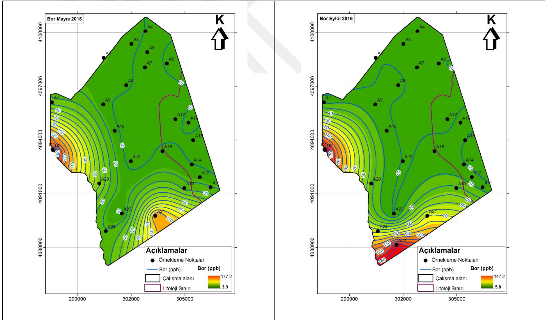
Şekil 4.16. Çalışma alanında B derişimlerinin alansal değışimi.
