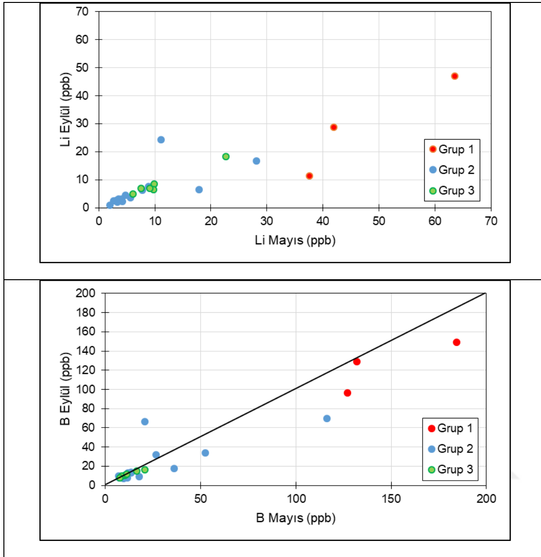
Şekil 4.14. Yağışlı ve kurak dönemlerde Li ve B derişimlerinin değışimi
