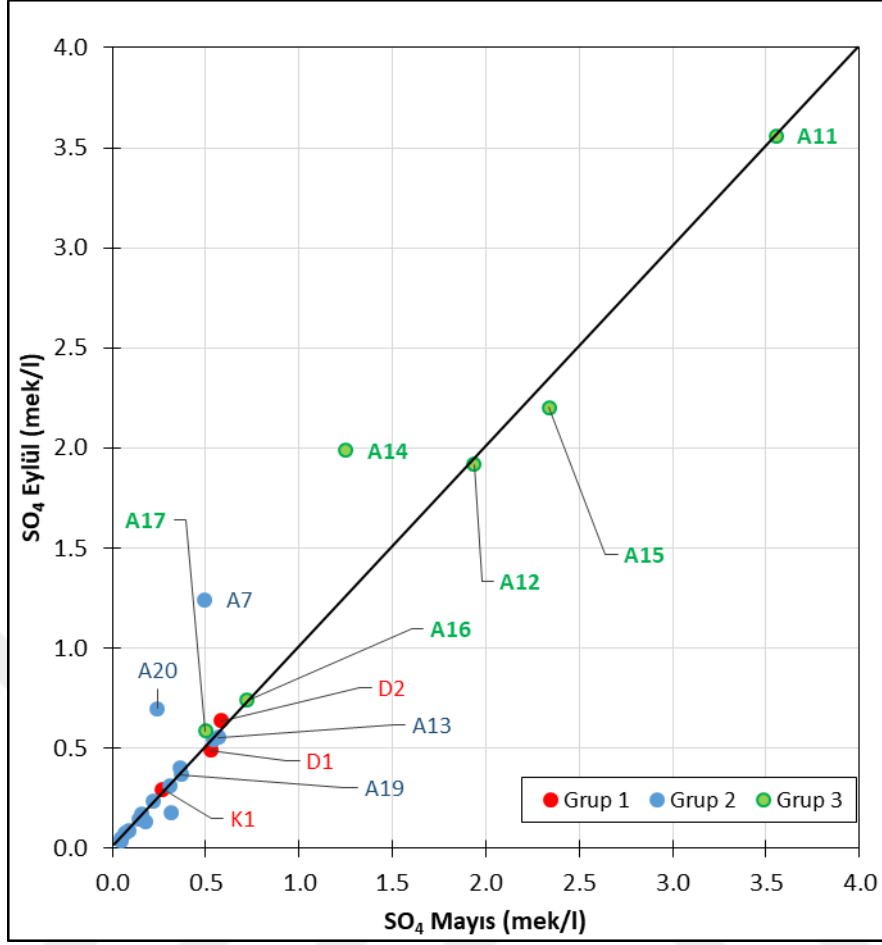
Şekil 4.10. Yağışlı ve kurak dönemlerde SO 4 -2 derişimlerinin değışimi.
