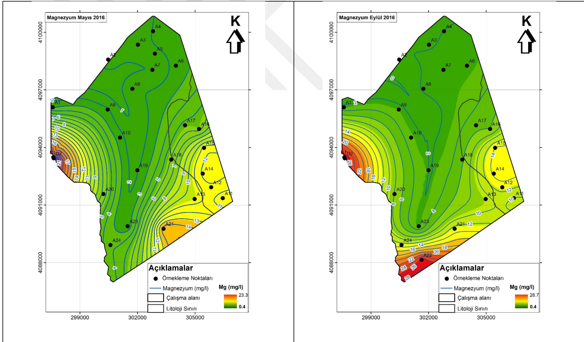
Şekil 4.12. Yağışlı ve kurak dönemlerde Mg^{+2} derişimlerinin alansal deęiřimi.
