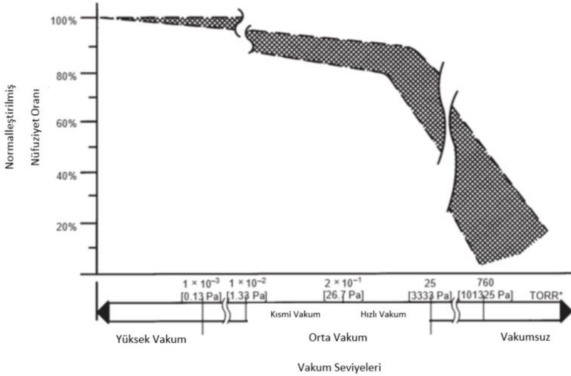
Şekil 1.6 Kaynak nüfuziyet miktarı ve vakum seviyesi ilişkisi [1]
