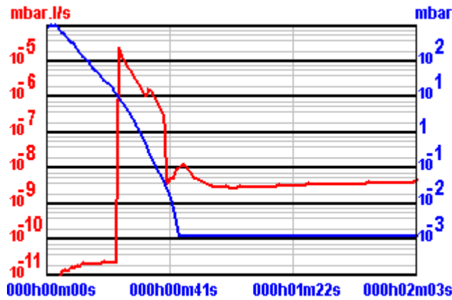
Şekil 5.63 Çizelge 5-9 1 numaralı basınçlı tüp He kaçak seviyesi, 3.5 \times 10^{-9} \frac{\text{mbar.lit}}{\text{s}}
