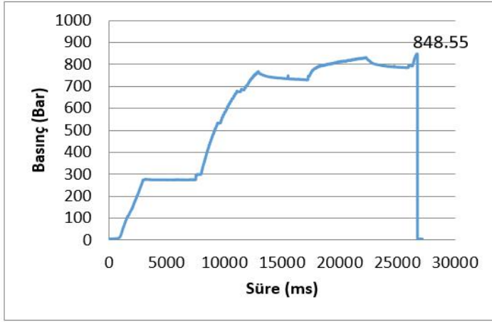
Şekil 5.30 8 numaralı basınçlı tüpün patlama basıncı-zaman grafiği ve prototip
