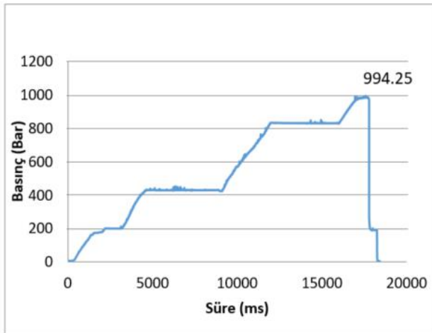
 ekil 5.58  izelge 5-8 2 numaralı basıncılı t p n patlama basıncı-zaman grafi i ve prototip
