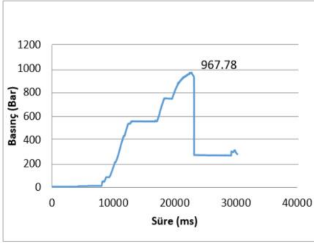
 ekil 5.57  izelge 5-8 1 numaralı basıncılı t p n patlama basıncı-zaman grafi i ve prototip
