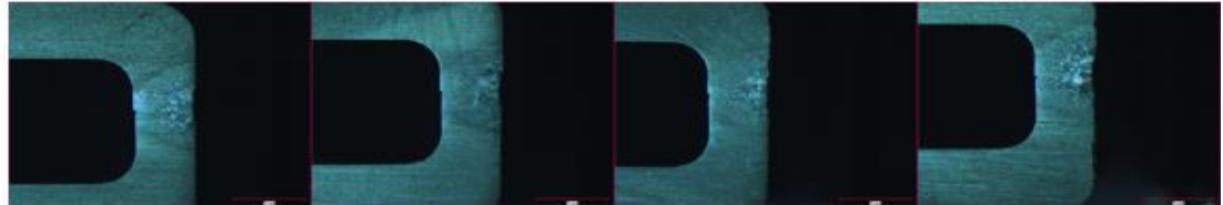
Şekil 5.46 Çizelge 5-6 Kupon 5 sırasıyla A,B,C ve D kesitleri X-ray makro görüntüleri (Ortalama KN: 1.39)
