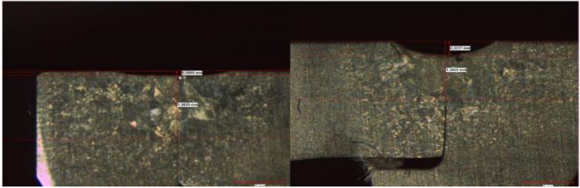
Şekil 5.34 Çizelge 5-3 ve Şekil 5.29 da belirtilen 7 numaralı basınçlı tüpün patlama olmayan yüzeyinden alınan numunelerin X-ray makro görüntüsü, kaynak bölgesi 1 (Kaynak nüfuziyeti 1.58 ile 1.34 mm arasında çevresel olarak değişiklik göstermektedir.)
