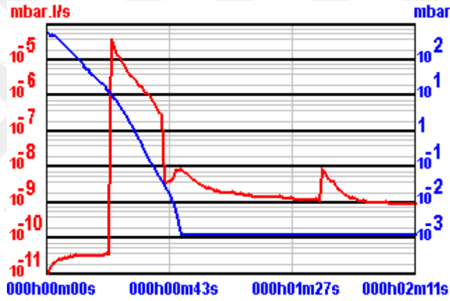
Şekil 5.62 Vakum odası He kaçak seviyesi, 3.2 \times 10^{-10} \frac{\text{mbar.lit}}{\text{s}}
