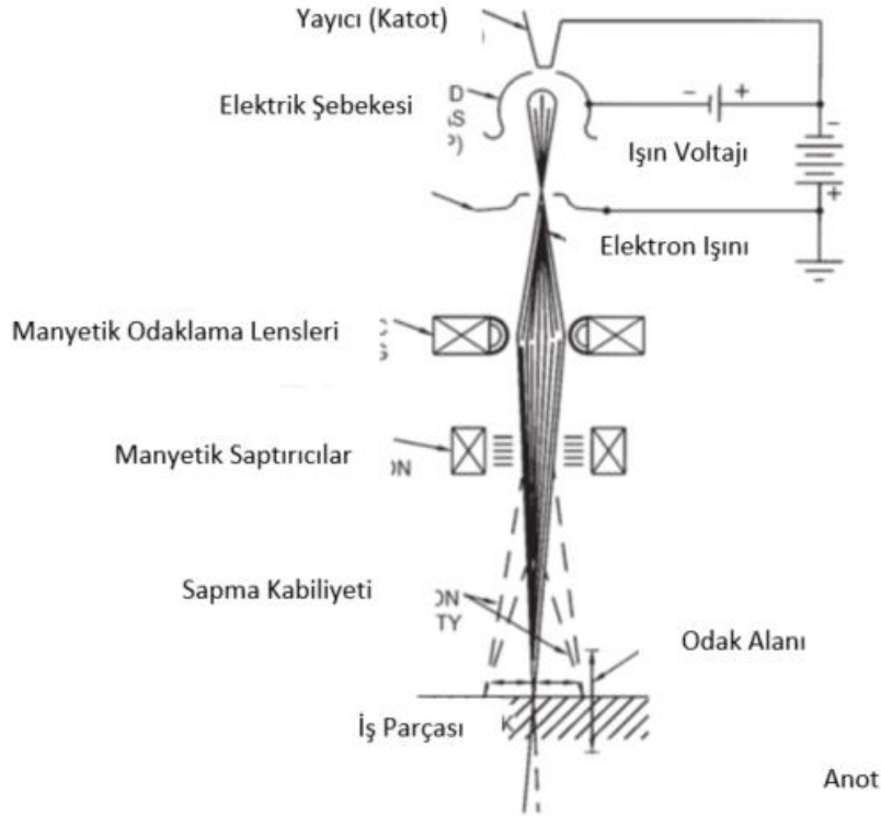
Şekil 1.1 Elektron ışın tabancasının çalışma şematifi [1]
