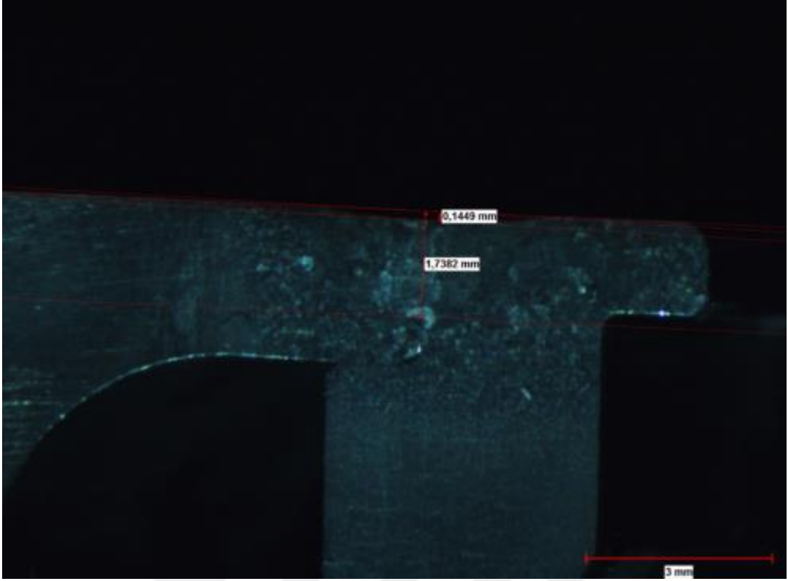
Şekil 5.14 Kupon 7 kesiti makro görüntü (KN: 1.74, KYÇ: 0.15) / Kaynak bölgesi 1
