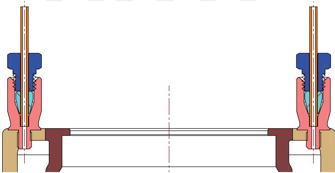
 ekil 3.2 Basıncılı t p  zeri pn matik aray zler kesit g r n m 
