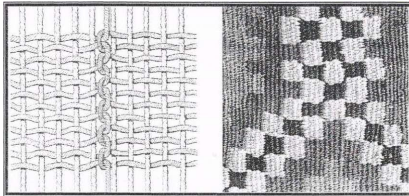
Şekil 11-a: Çift Kenetleme İle İliklerin Yok Edilmesi (Acar, 1982 s:)
