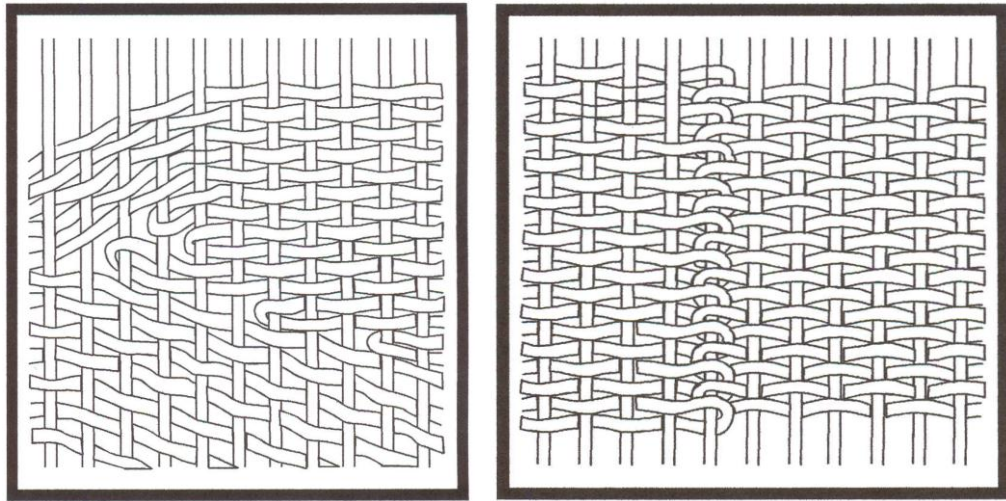
řekil 9: Atkılarının Aynı Çözg¼den Geri Dönmesi İle İliklerin Yok Edilmesi (Acar, 1982 s:)
