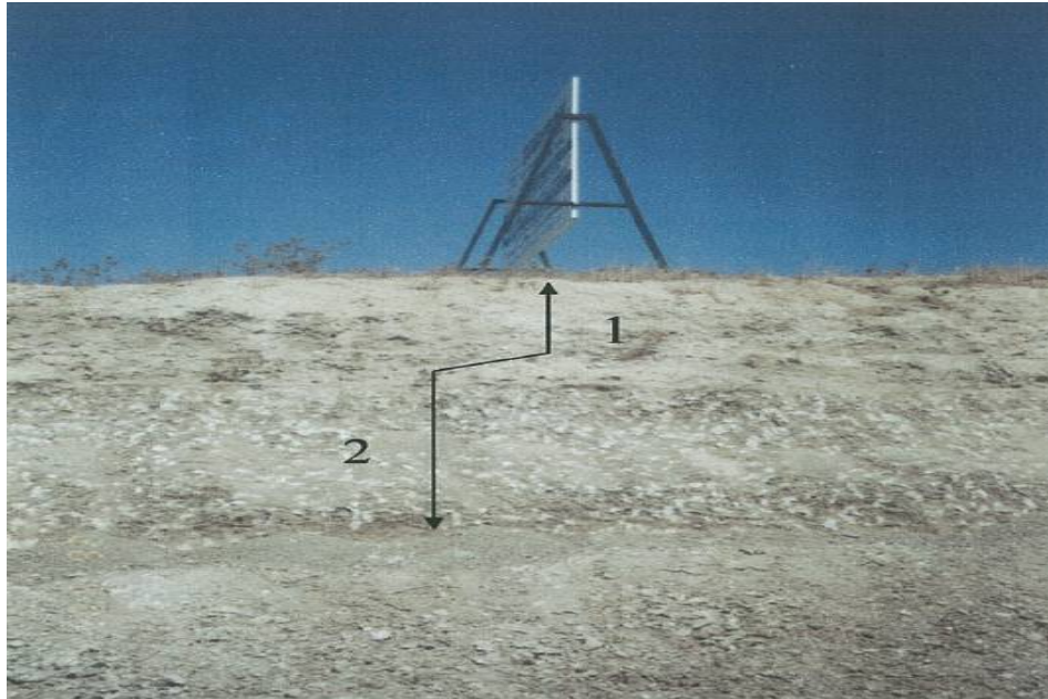
Fotoğraf 1.1. Karasal seki'yi oluşturan ve ikincil kireçtaşı yumruları içeren eski alüvyon (2). Karasal seki üzerinde yer alan kumlu alüvyon (1)
