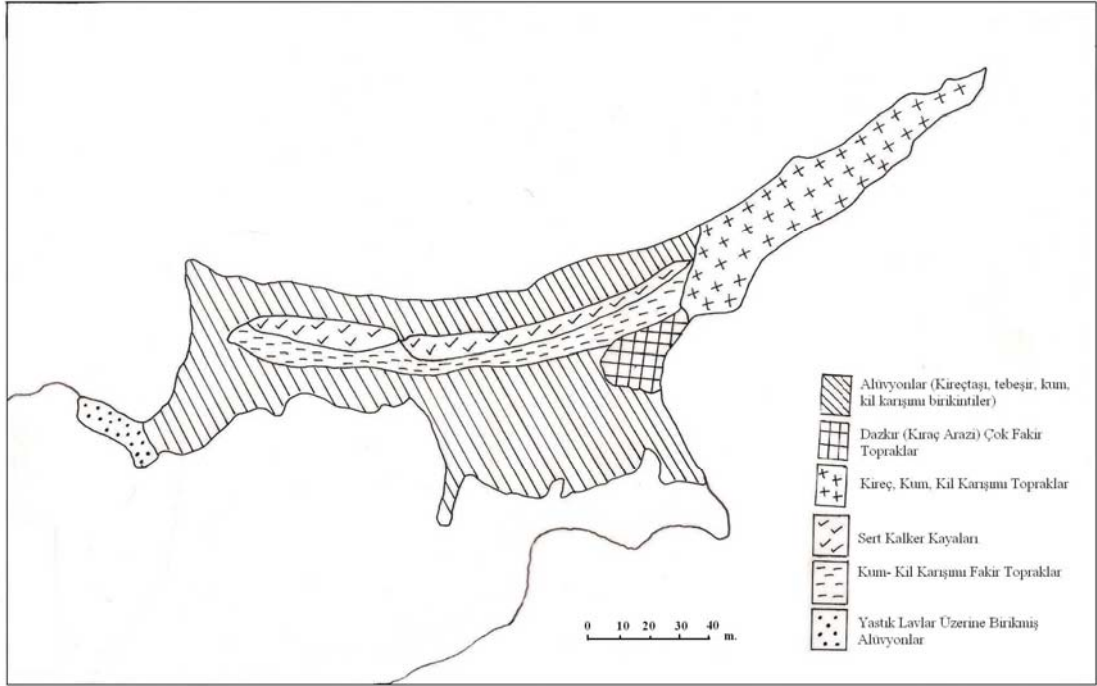
Harita 8. KKTC'nin toprak haritası
