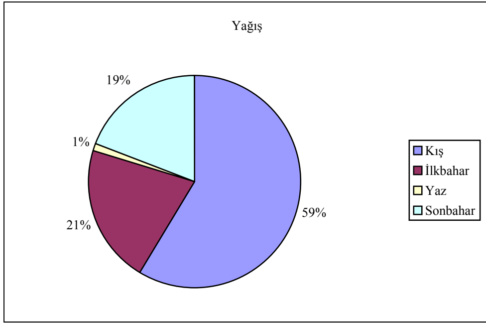
Şekil 1.3. Yağışın mevsimlere göre dağılışı
