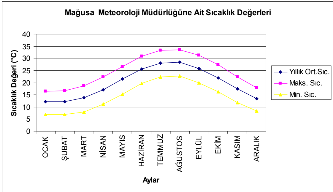
Şekil 1.1. Gazimağusa'da sıcaklık değerlerinin yıllık durumu
