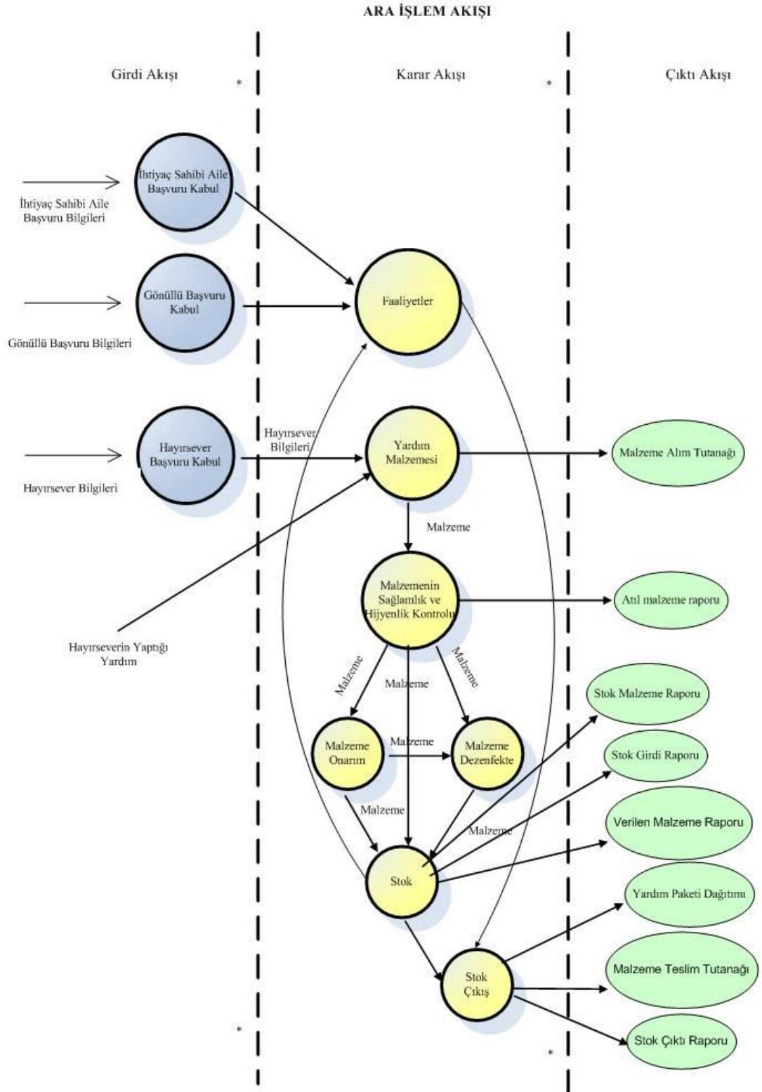
Şekil 7.1.3.2 Dönüştürme İşlem Akışı Şemaları
