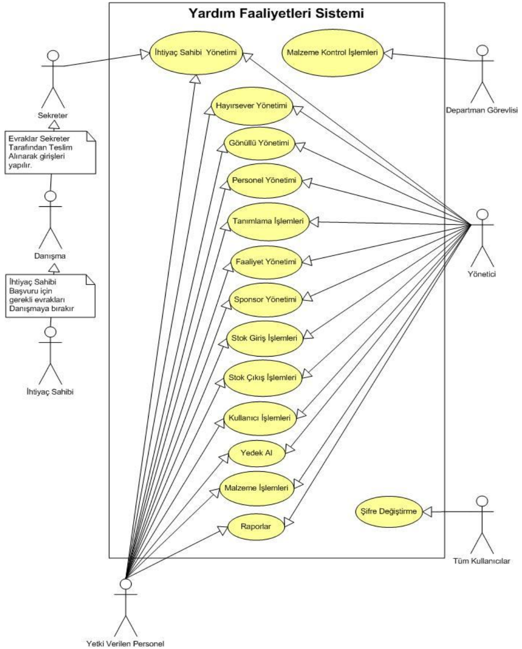
Şekil 6.1.2.1 Sistemin Use Case Diyagramı
