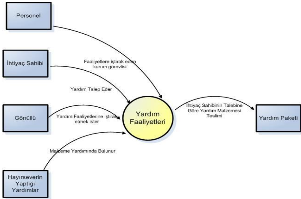
Şekil 6.1.7.1.1 Veri Akış Diyagramı (Düzey 0)
