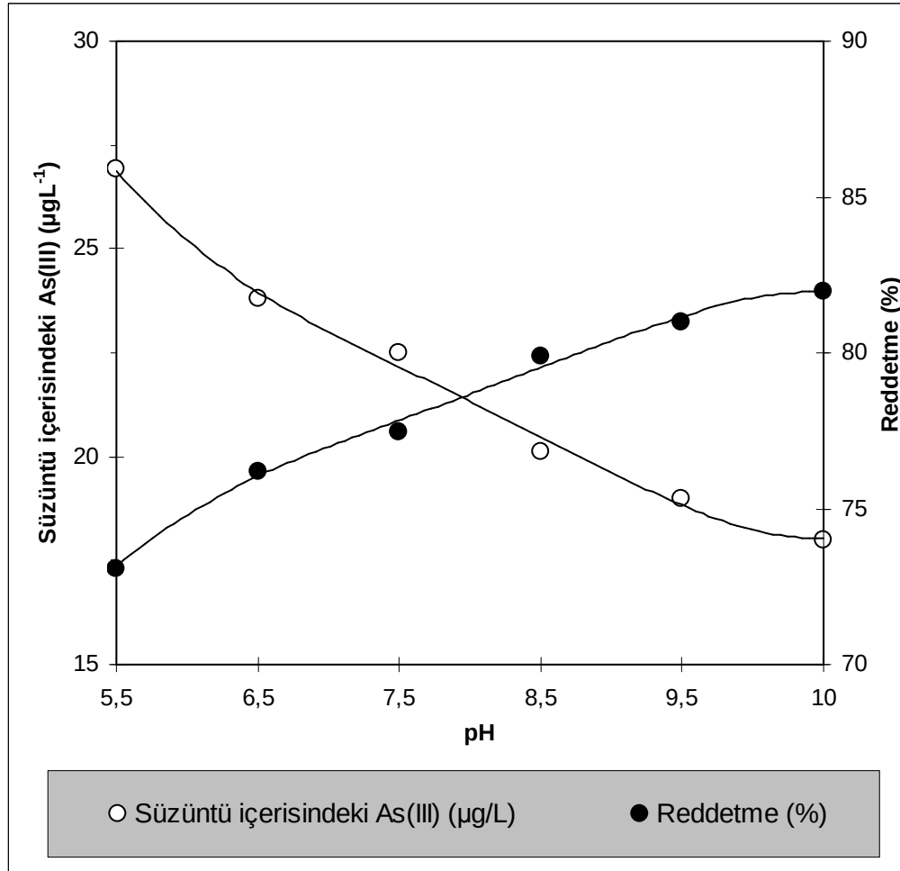
Şekil 8.23. Ters osmoz SWHR membranı ile arsenit uzaklaştırılması üzerine pH etkisi çalışması (Besleme çözelti konsantrasyonu: 100 ppb, basınç: 20 bar, sıcaklık: 25°C)
