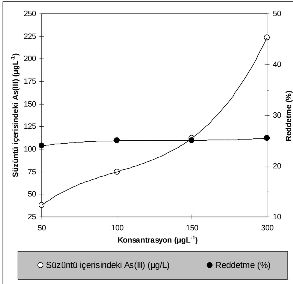
Şekil 8.17. Nanofiltrasyon NF 270 membranı ile arsenit uzaklaştırılması üzerine konsantrasyon etkisi çalışması (Basınç: 20 bar, sıcaklık: 25°C, pH: 6,75)
