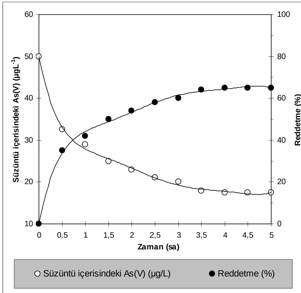
Şekil 9.5. NF 270 Membranı ile gerçek su numunesinde arsenat gideriminin zamana bağlı değişimi (besleme konsantrasyonu Gölbahçe: 50 \pm 2,7 µg/L, besleme çözeltisi pH'sı Gölbahçe: 7,1; sıcaklık: 25 °C)
