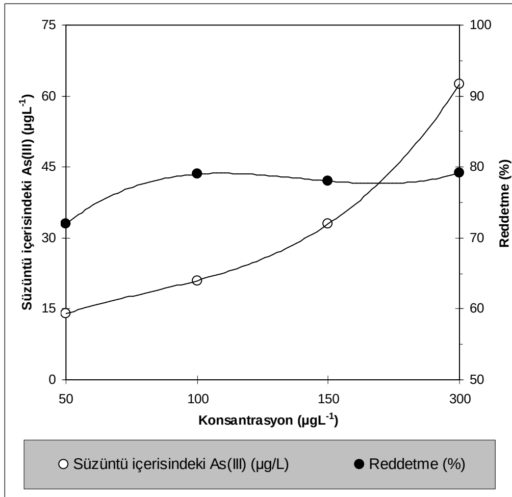
Şekil 8.21. Ters osmoz SWHR membranı ile arsenit uzaklaştırılması üzerine konsantrasyon etkisi çalışması (Besleme çözelti konsantrasyonu: 100 ppb, basınç: 20 bar, sıcaklık: 25°C, pH: 6,75)
