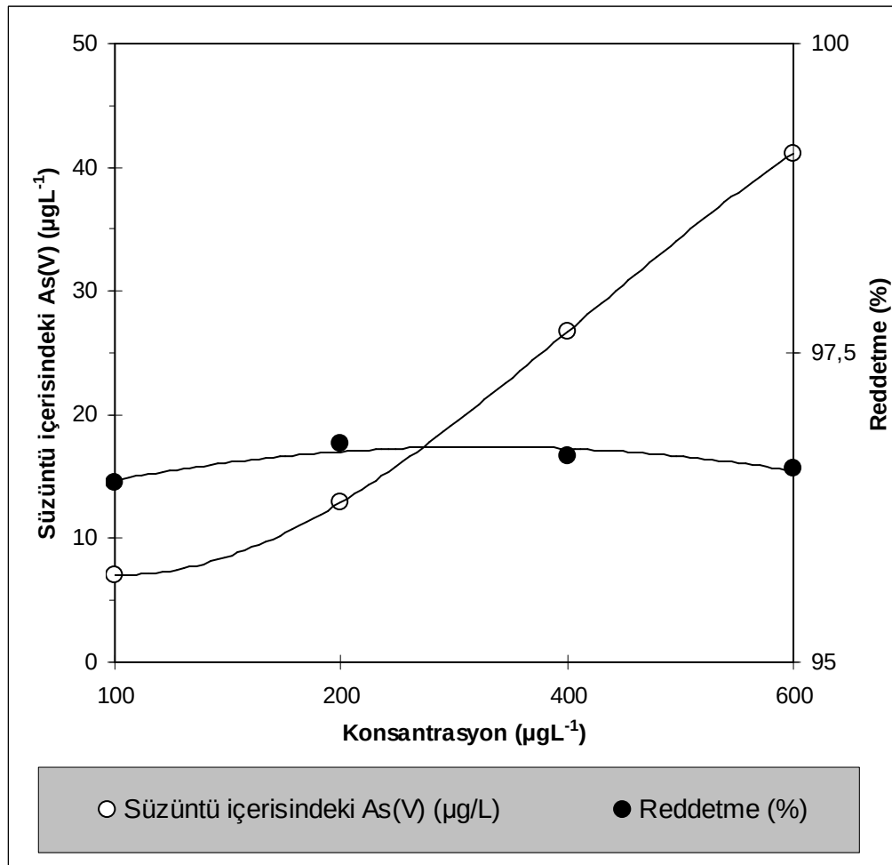
Şekil 8.9. Ters Osmoz SWHR membranı ile arsenat uzaklaştırılması üzerine konsantrasyon etkisi çalışması (Basınç: 20 bar, sıcaklık: 25°C, pH: 6,75)
