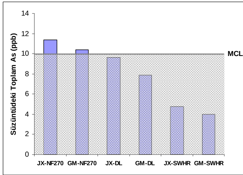
Şekil 10.4. Hibrit membranlar ile yapılan denemelerde süzüntüdeki toplam arsenik miktarının MCL ile kıyaslanması
