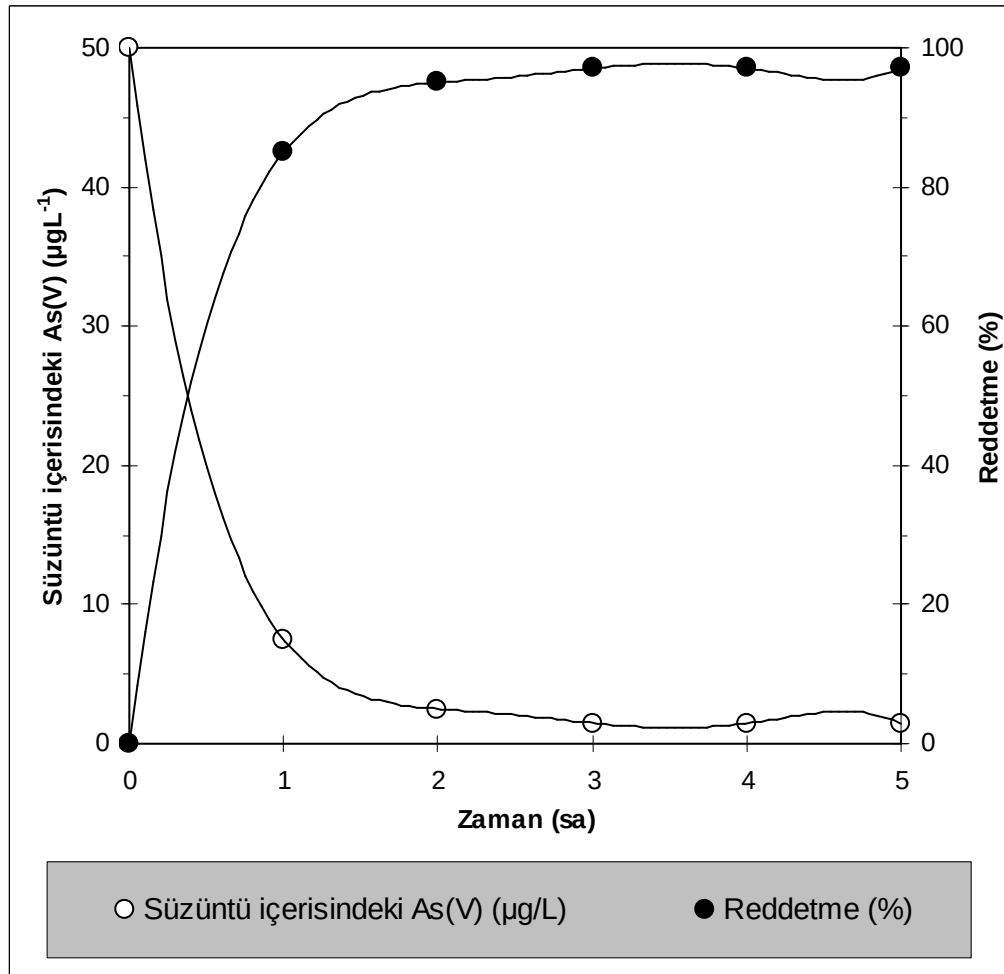
Şekil 9.18. UF-GM / RO-SWHR Hibrit membran prosesi ile gerçek su numunesinden arsenit gideriminin zamana bağlı değişimi (besleme konsantrasyonu Gölpazarı: 12 \pm 2 µg/L, besleme çözeltisi pH'sı Gölpazarı : 7,1; sıcaklık:25 °C)
