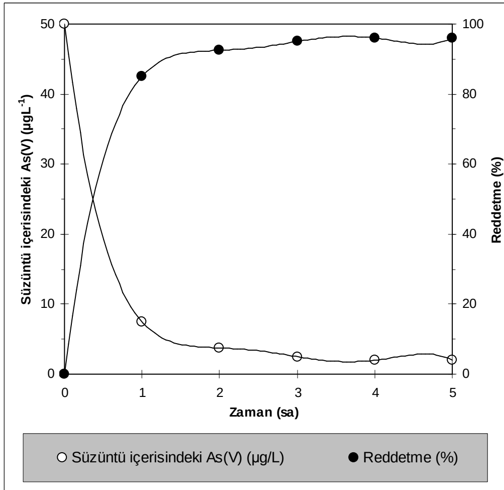
Şekil 9.17. MF-JX / RO-SWHR Hibrit membran prosesi ile gerçek su numunesinden arsenat gideriminin zamana bağlı değişimi (besleme konsantrasyonu Gölpazarı: 12 \pm 2 µg/L, besleme çözeltisi pH'sı Gölpazarı : 7,1; sıcaklık:25 °C)
