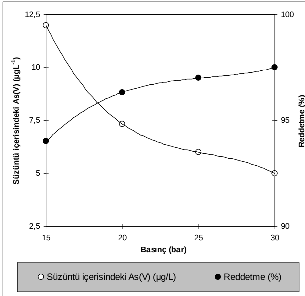
Şekil 8.10. Ters Osmoz SWHR membranı ile arsenat uzaklaştırılması üzerine basınç etkisi çalışması (Besleme çözelti konsantrasyonu: 200 ppb, sıcaklık: 25°C, pH: 6,75)
