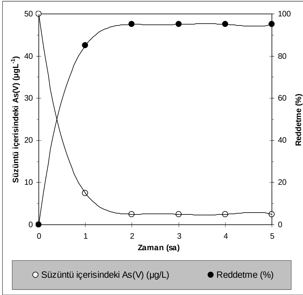
Şekil 9.14. UF-GM / NF-DL Hibrit membran prosesi ile gerçek su numunesinden arsenat gideriminin zamana bağlı değişimi (besleme konsantrasyonu Gölpazarı: 12 \pm 2 µg/L, besleme çözeltisi pH'sı Gölpazarı : 7,1; sıcaklık:25 °C)
