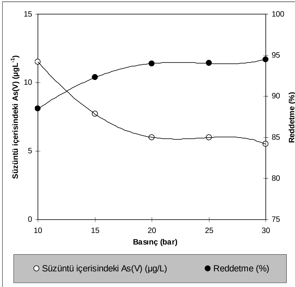
Şekil 8.6. Nanofiltrasyon NF 270 membranı ile arsenat uzaklaştırılması üzerine basınç etkisi çalışması (Besleme çözelti konsantrasyonu: 100 ppb, sıcaklık: 25°C, pH: 6,75)
