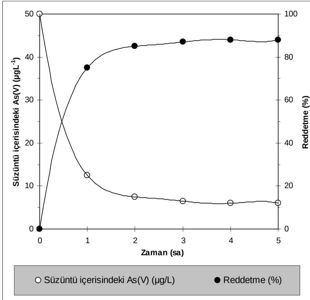
Şekil 9.15. MF-JX / NF-NF 270 Hibrit membran prosesi ile gerçek su numunesinden arsenat gideriminin zamana bağlı değişimi (besleme konsantrasyonu Gülbahçe: 12 \pm 2 µg/L, besleme çözeltisi pH'sı Gülbahçe : 7,1; sıcaklık:25 °C)
