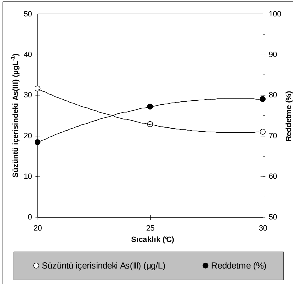
Şekil 8.24. Ters osmoz SWHR membranı ile arsenit uzaklaştırılması üzerine sıcaklık etkisi çalışması (Besleme çözelti konsantrasyonu: 100 ppb, basınç: 20 bar, pH: 6,75)
