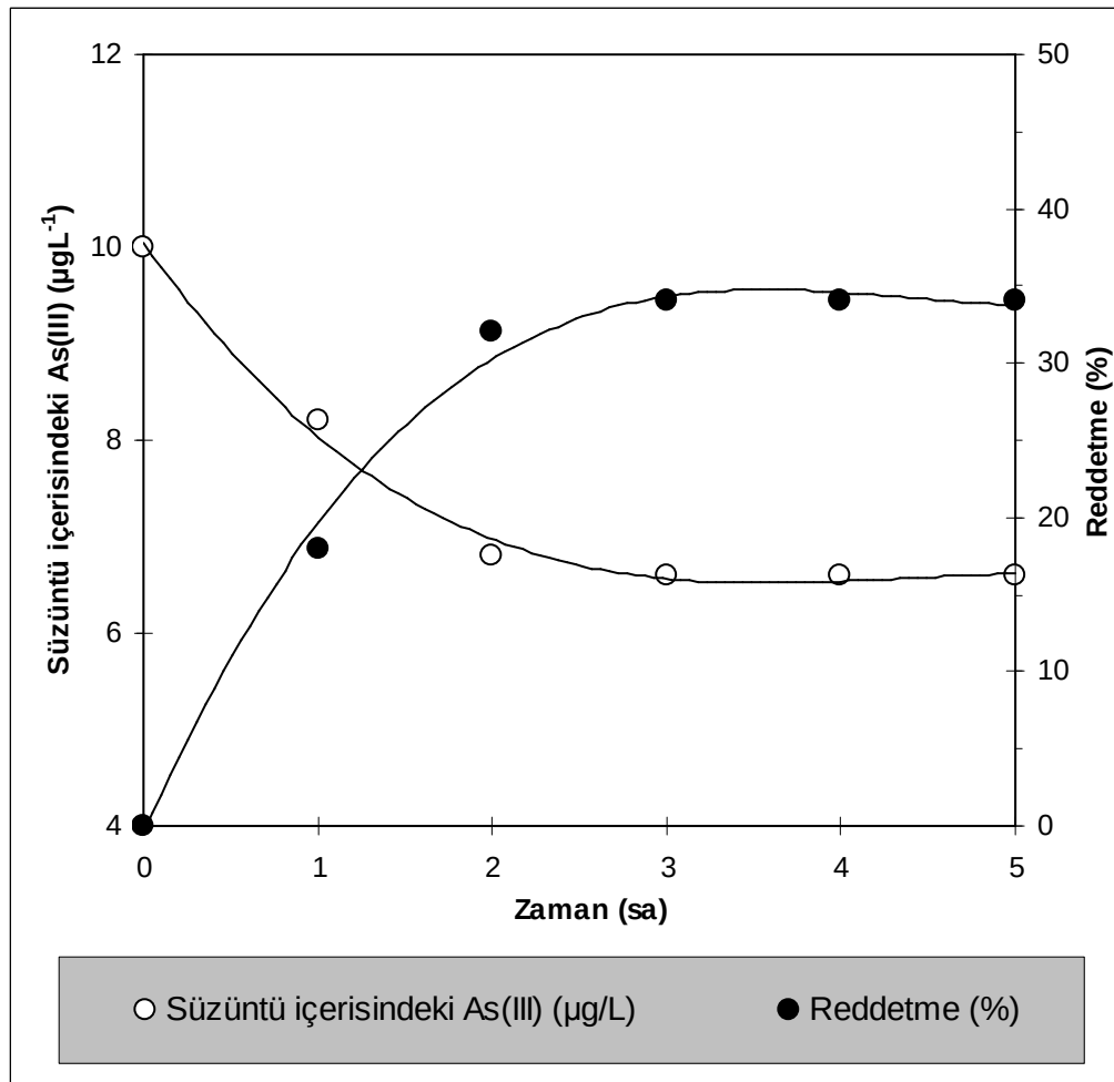
Şekil 9.7. MF-JX / NF-DL Hibrit membran prosesi ile gerçek su numunesinden arsenit gideriminin zamana bağlı değişimi (besleme konsantrasyonu Gölpazarı: 12 \pm 2 µg/L, besleme çözeltisi pH'sı Gölpazarı : 7,1; sıcaklık:25 °C)
