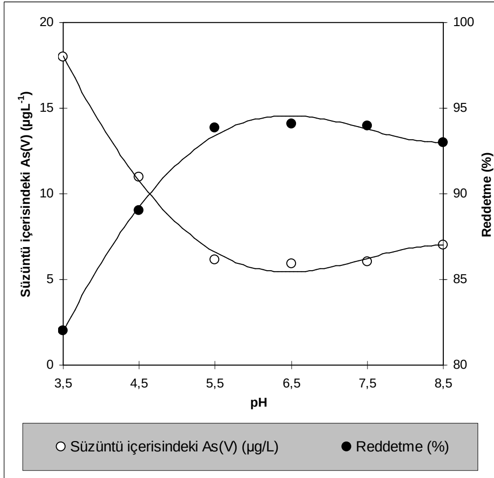
Şekil 8.7. Nanofiltrasyon NF 270 membranı ile arsenat uzaklaştırılması üzerine pH etkisi çalışması (Besleme çözelti konsantrasyonu: 100 ppb, basınç: 20 bar, sıcaklık: 25°C)
