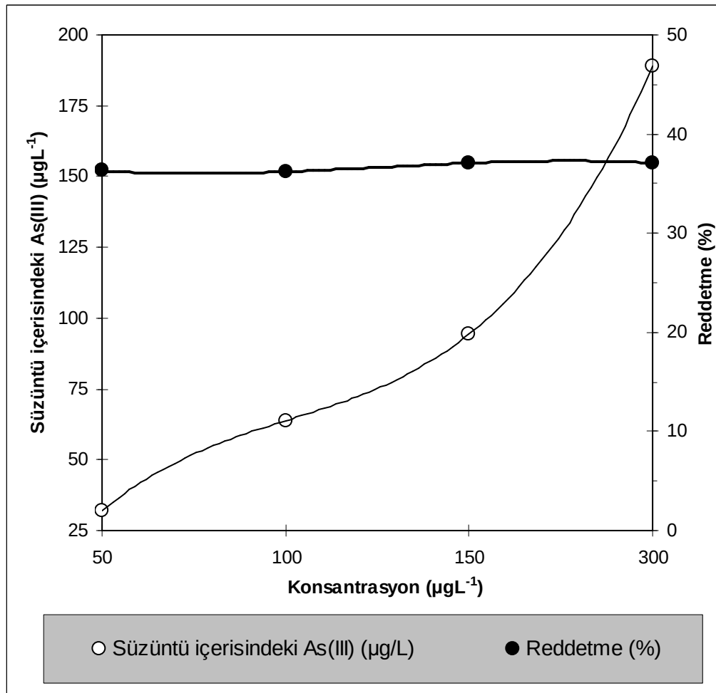
Şekil 8.13. Nanofiltrasyon DL membranı ile arsenit uzaklaştırılması üzerine konsantrasyon etkisi çalışması (Basınç: 20 bar, sıcaklık: 25°C, pH: 6,75)
