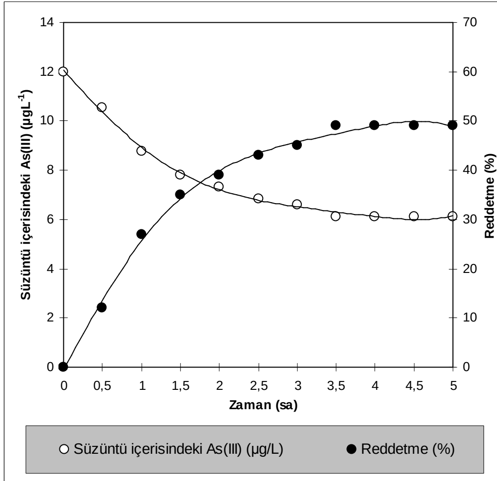
Şekil 9.3. SWHR Membranı ile gerçek su numunesinde arsenit gideriminin zamana bağlı değişimi (besleme konsantrasyonu Gölbahçe: 12 ±2 μg/L, besleme çözeltisi pH'sı Gölbahçe: 7,1; sıcaklık:25 °C)
