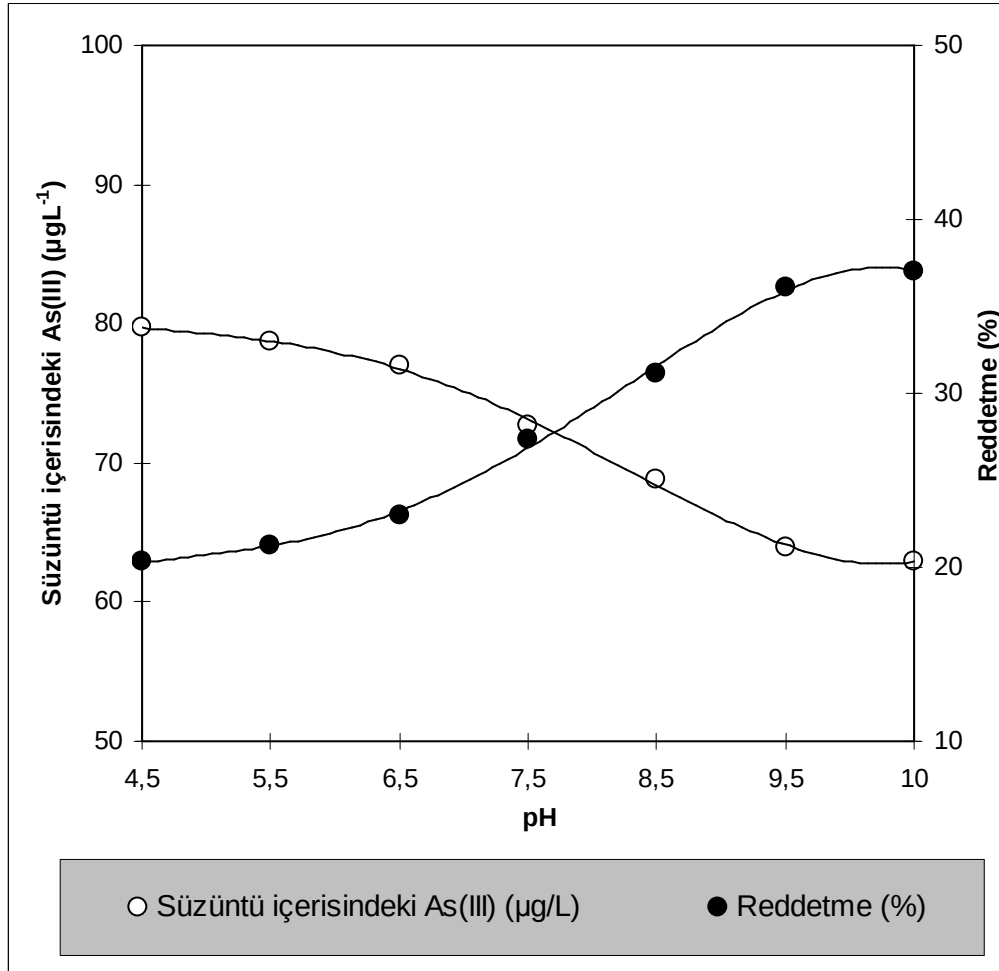
Şekil 8.15. Nanofiltrasyon DL membranı ile arsenit uzaklaştırılması üzerine pH etkisi çalışması (Besleme çözelti konsantrasyonu: 100 ppb, basınç: 20 bar, sıcaklık: 25°C)
