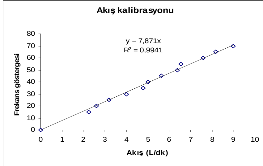
Şekil 7.2. Pilot sistem frekans göstergesi akış hızı kalibrasyon grafiği (TÜBİTAK Proje No:106Y299)
