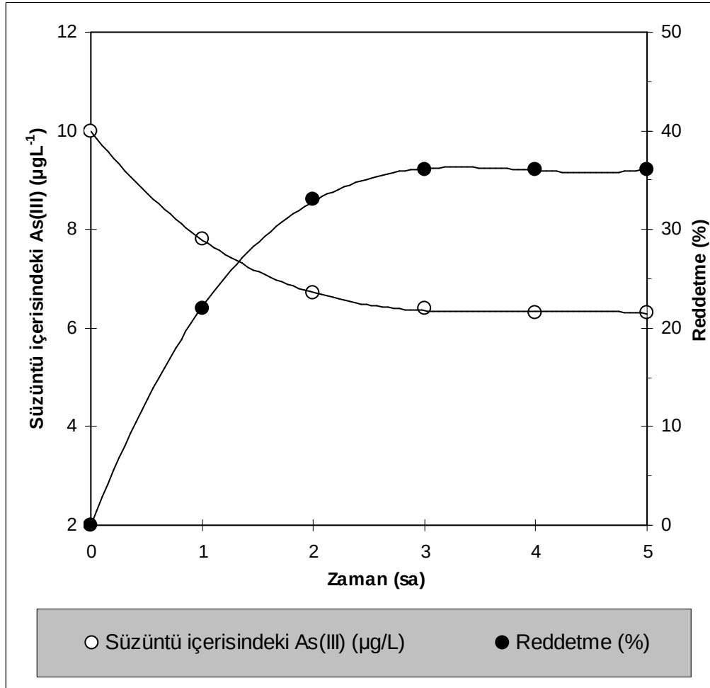
Şekil 9.8. UF-GM / NF-DL Hibrit membran prosesi ile gerçek su numunesinden arsenit gideriminin zamana bağlı değişimi (besleme konsantrasyonu Gölpazarı: 12 \pm 2 µg/L, besleme çözeltisi pH'sı Gölpazarı : 7,1; sıcaklık:25 °C)
