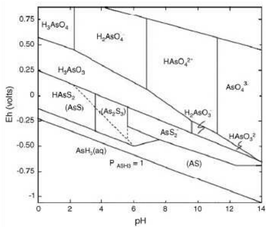
Şekil 2.6. Arsenik İçin Eh-pH Grafiği ( Ferguson, 1972; Pookrod, 2004; Mohan, 2007).
