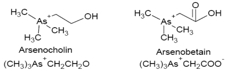
Şekil 2.3(b). Organik Arsenik Türlerine Ait Kimyasal Formül ve Yapılar
