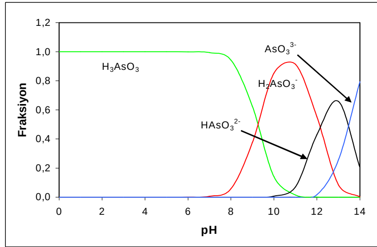
Şekil 10.7 As(III) iyonlarının asit-baz kimyası (Aragon, 2004).
