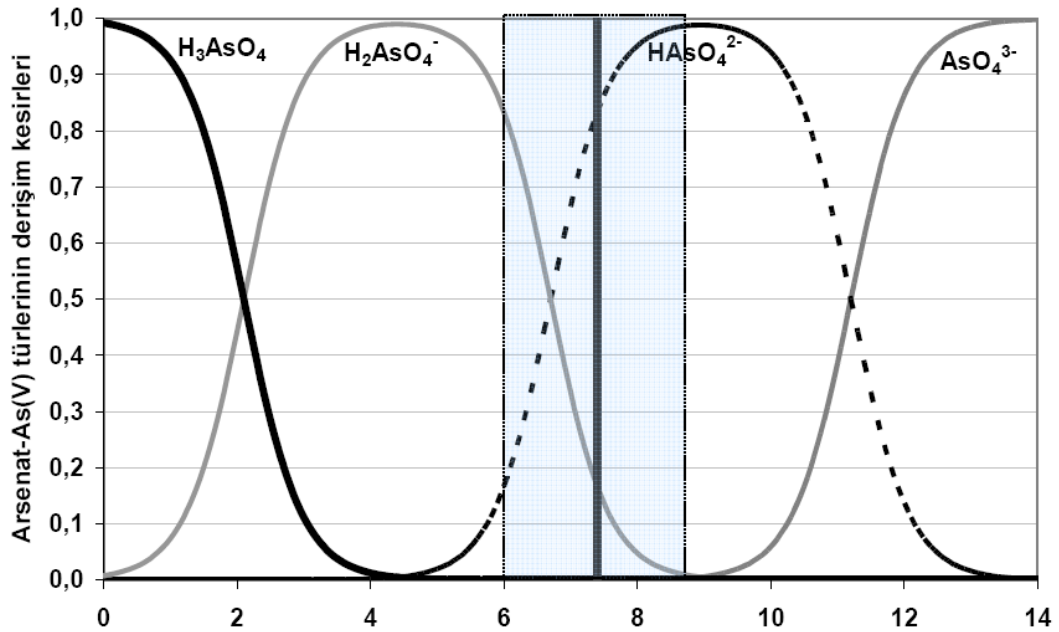
Şekil 2.5. Beş Değerlikli Arsenik Türlerinin pH İle Değişen Bulunma Kesirleri (Demircioğlu, 2009)
