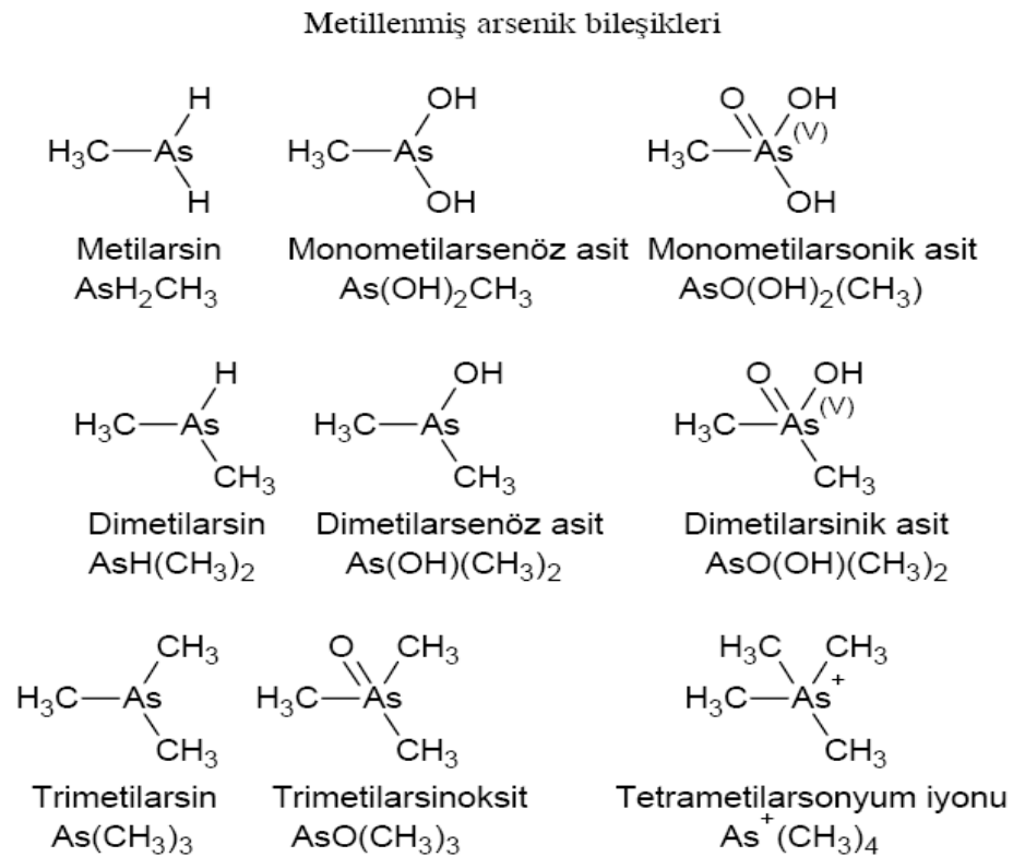
Şekil 2.3(a). Metillenmiş Arsenik Türlerine Ait Kimyasal Formül ve Yapılar
