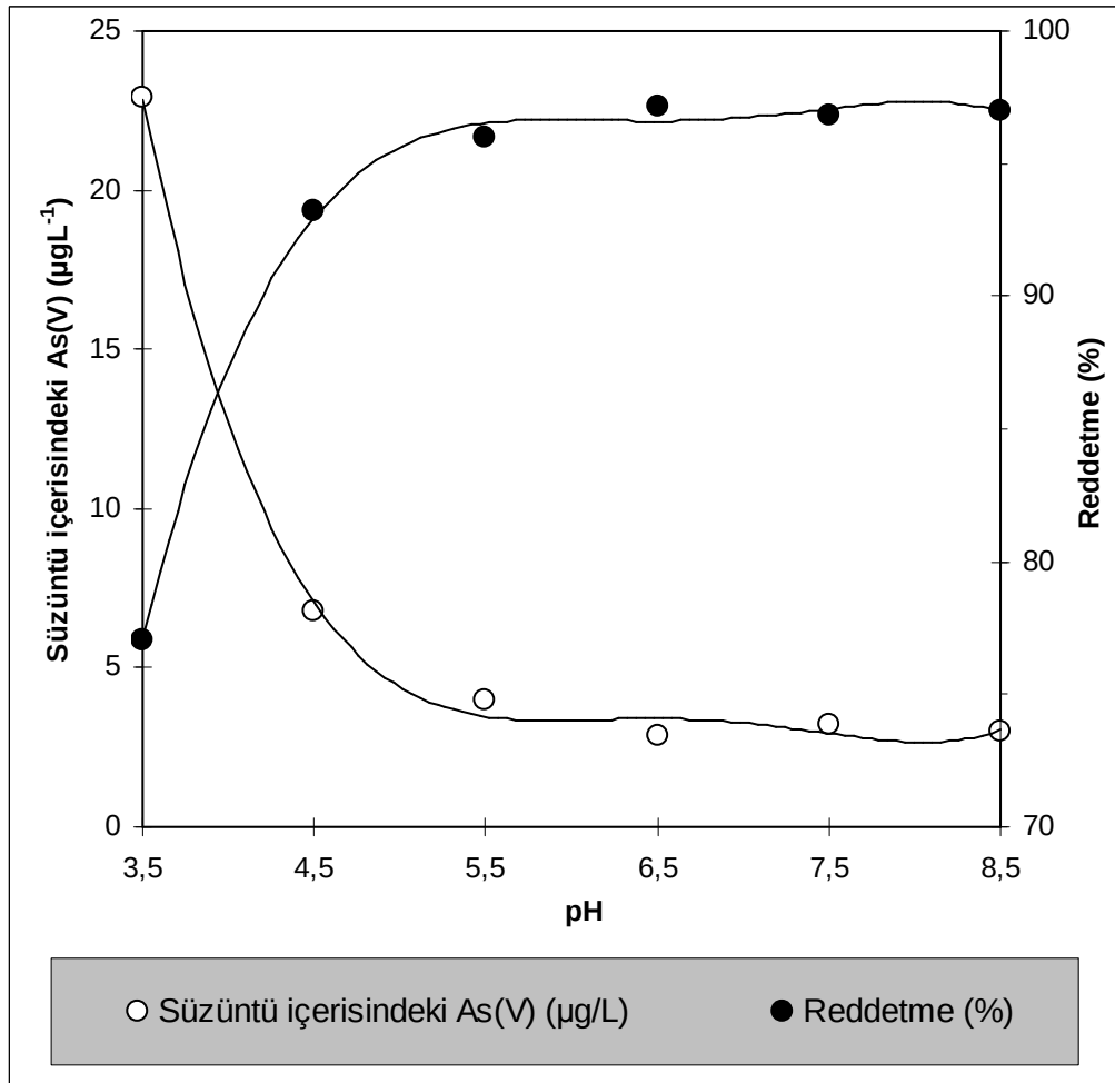
Şekil 8.3. Nanofiltrasyon DL membranı ile arsenat uzaklaştırılması üzerine pH etkisi çalışması (Besleme çözelti konsantrasyonu: 100 ppb, basınç: 20 bar, sıcaklık: 25°C)
