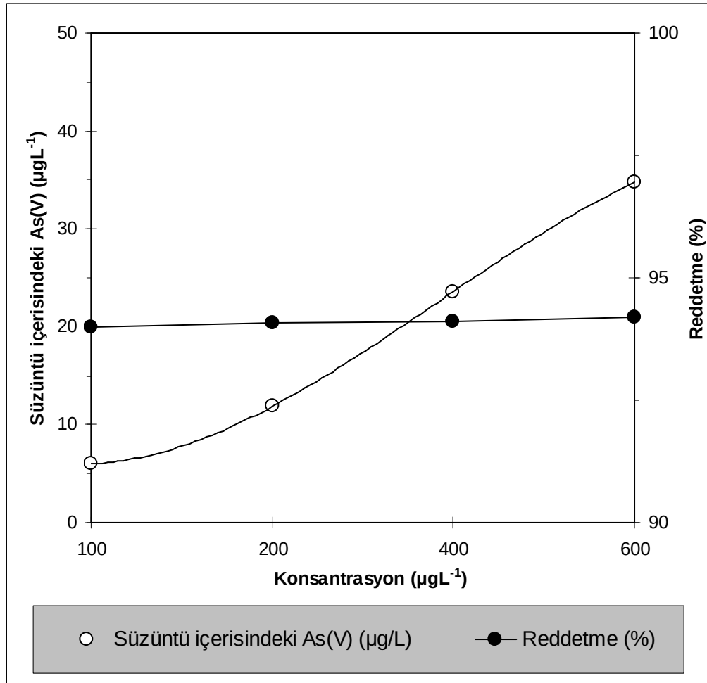
Şekil 8.5. Nanofiltrasyon NF 270 membranı ile arsenat uzaklaştırılması üzerine konsantrasyon etkisi çalışması (Basınç: 20 bar, sıcaklık: 25°C, pH: 6,75)
