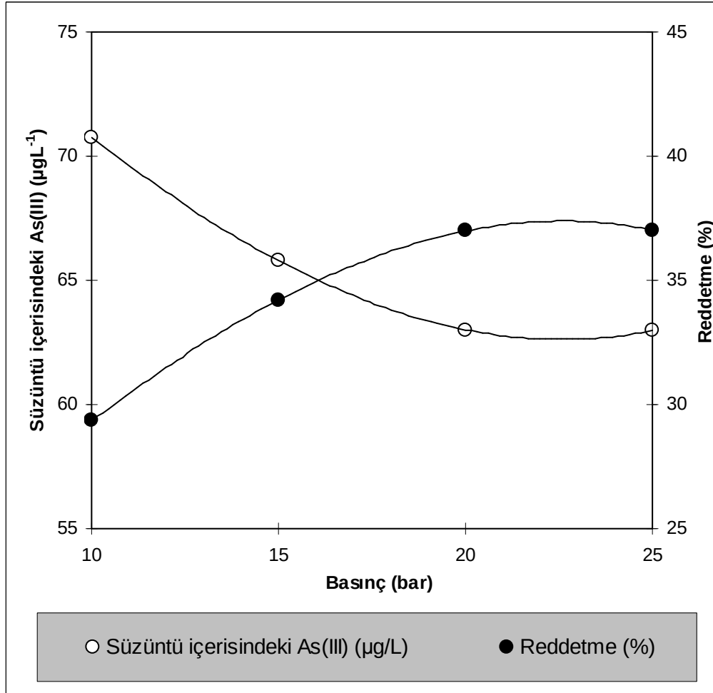
Şekil 8.14. Nanofiltrasyon DL membranı ile arsenit uzaklaştırılması üzerine basınç etkisi çalışması (Besleme çözelti konsantrasyonu: 100 ppb, sıcaklık: 25°C, pH: 6,75)
