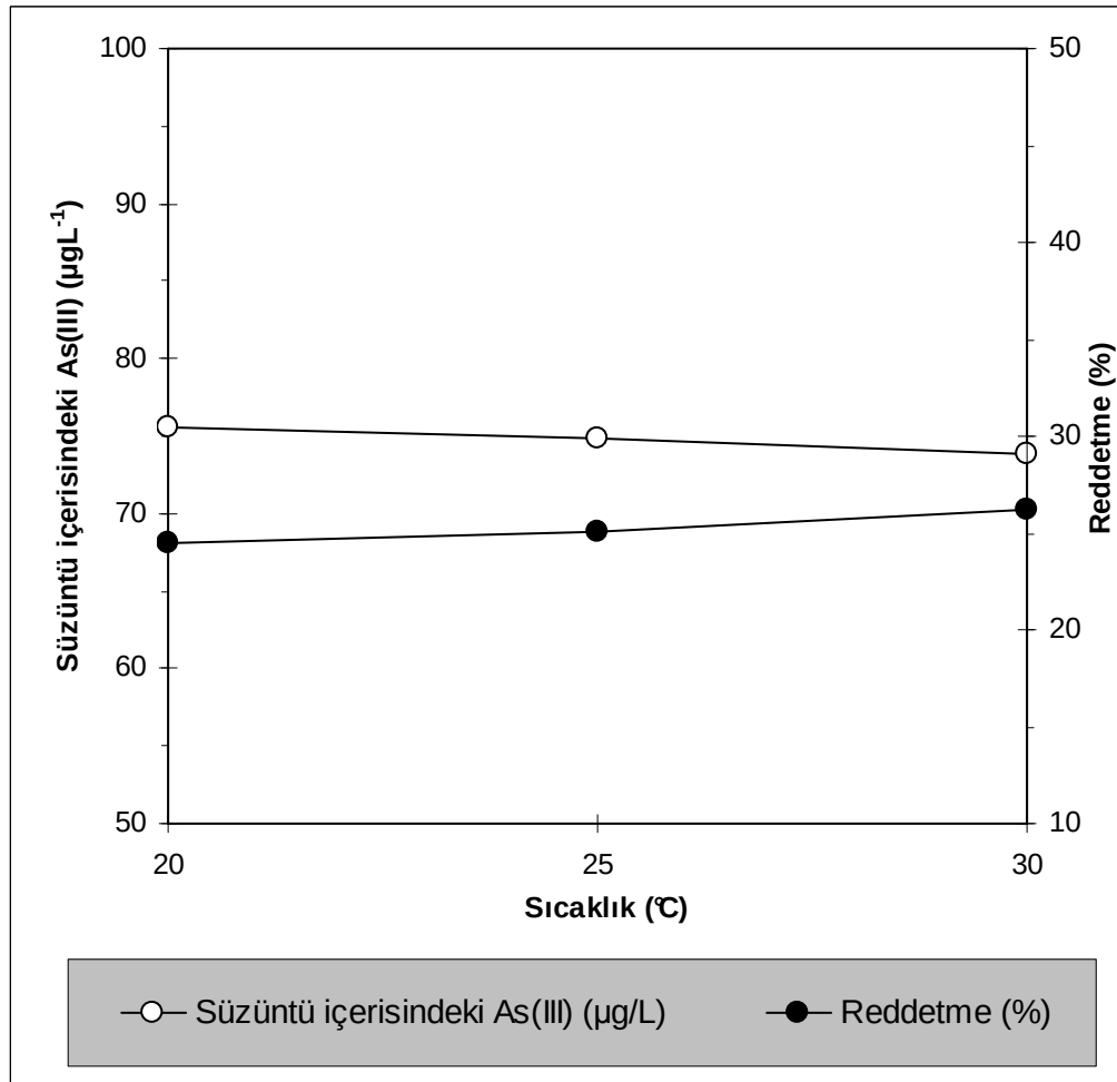
Şekil 8.20. Nanofiltrasyon NF 270 membranı ile arsenit uzaklaştırılması üzerine sıcaklık etkisi çalışması (Besleme çözelti konsantrasyonu: 100 ppb, basınç: 20 bar, pH: 6,75)
