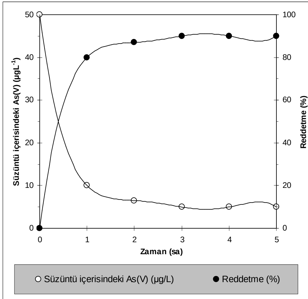
Şekil 9.16. UF-GM / NF-NF 270 Hibrit membran prosesi ile gerçek su numunesinden arsenat gideriminin zamana bağlı değişimi (besleme konsantrasyonu Gülbahçe: 12 \pm 2 µg/L, besleme çözeltisi pH'sı Gülbahçe : 7,1; sıcaklık:25 °C)
