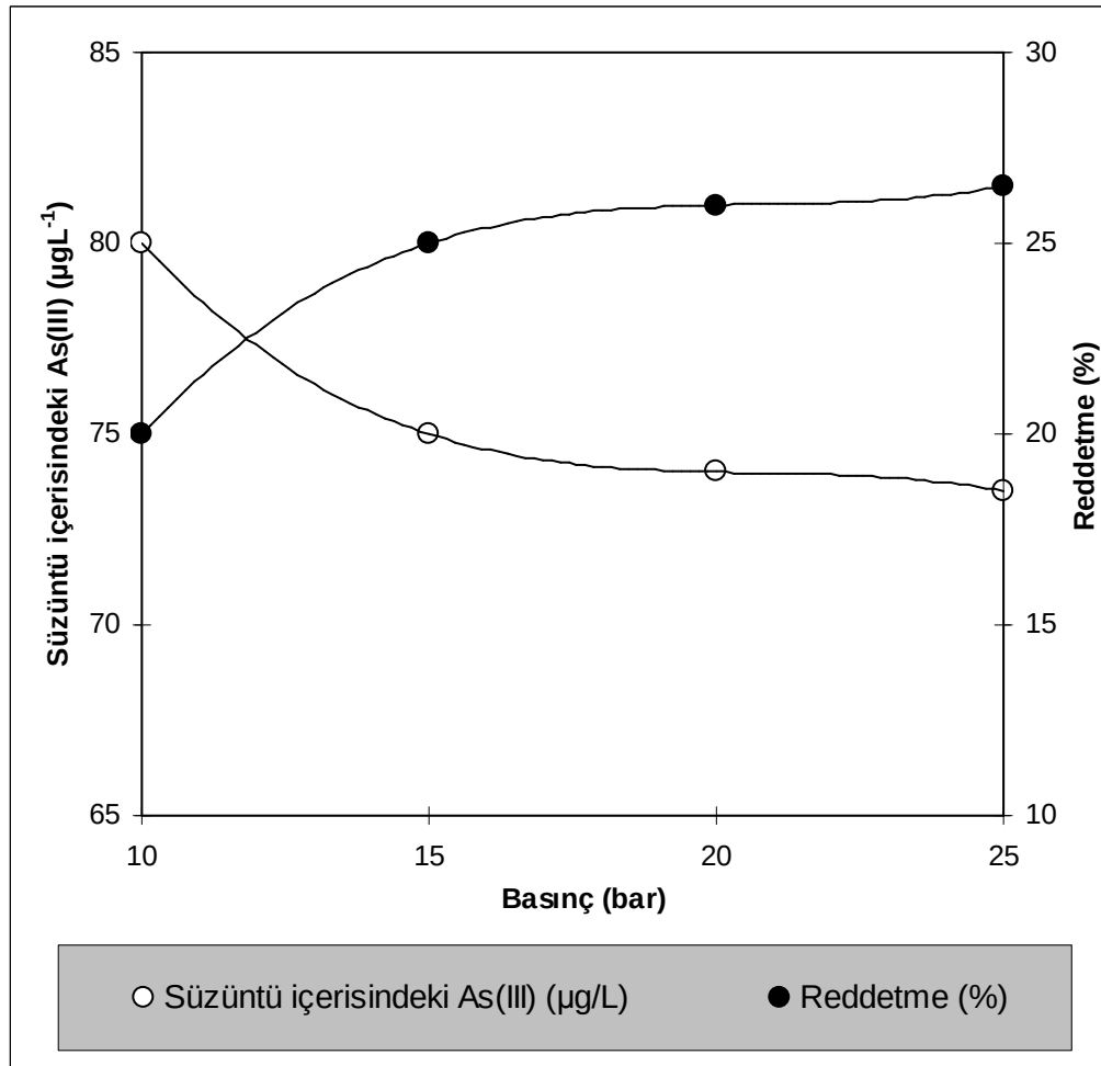
Şekil 8.18. Nanofiltrasyon NF 270 membranı ile arsenit uzaklaştırılması üzerine basınç etkisi çalışması (Besleme çözelti konsantrasyonu: 100 ppb, sıcaklık: 25°C, pH: 6,75)
