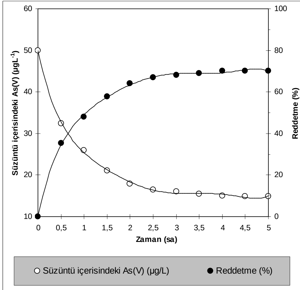
Şekil 9.4. DL Membranı ile gerçek su numunesinde arsenat gideriminin zamana bağlı değişimi (besleme konsantrasyonu Gölbahçe: 50 ±2,7 µg/L, besleme çözeltisi pH'sı Gölbahçe: 7,1; sıcaklık:25 °C)
