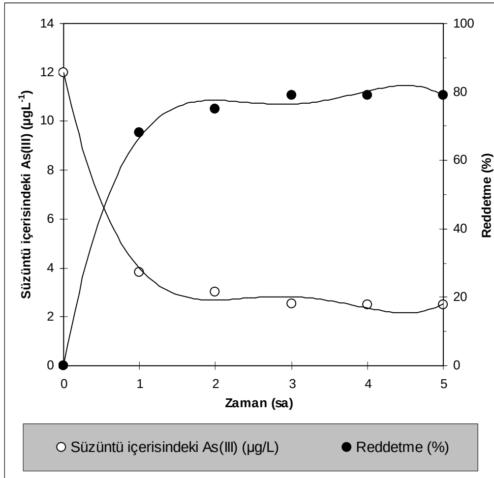
Şekil 9.12. UF-GM / RO-SWHR Hibrit membran prosesi ile gerçek su numunesinden arsenit gideriminin zamana bağlı değişimi (besleme konsantrasyonu Gölpazarı: 12 ±2 µg/L, besleme çözeltisi pH'sı Gölpazarı : 7,1; sıcaklık:25 °C)
