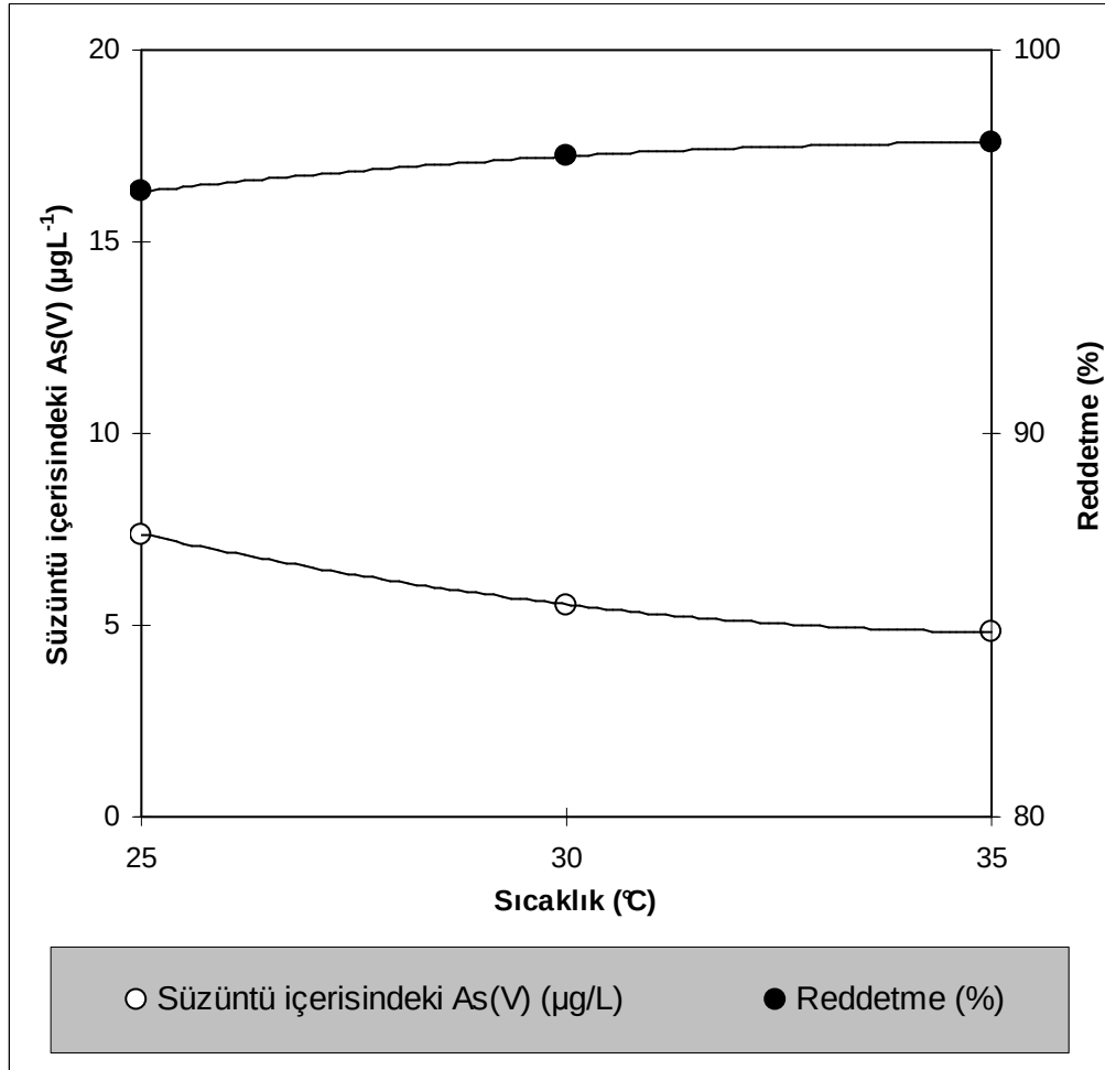
Şekil 8.12. Ters Osmoz SWHR membranı ile arsenat uzaklaştırılması üzerine sıcaklık etkisi çalışması (Besleme çözelti konsantrasyonu: 200 ppb, basınç: 20 bar, pH: 6,75)
