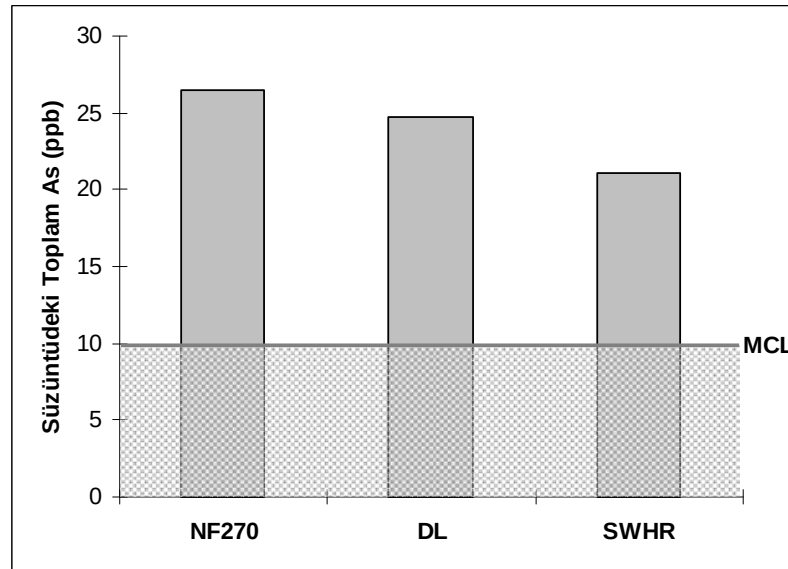
Şekil 10.2. Süzüntüdeki toplam arsenik miktarının MCL ile kıyaslanması
