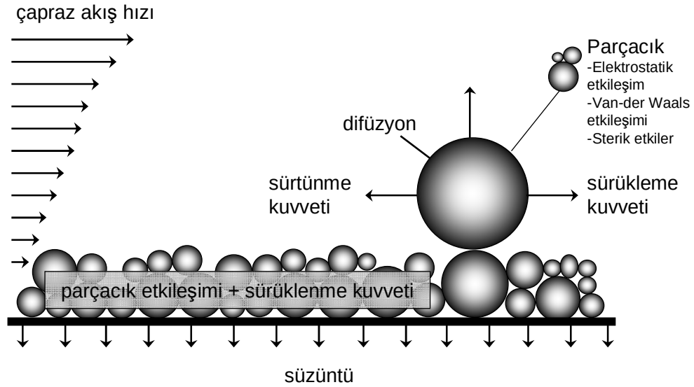
Şekil 5.2. Membran malzemesi üzerinde tutulan parçacıklara etki eden kuvvetler (Ripperger ve Altmann 2002)
