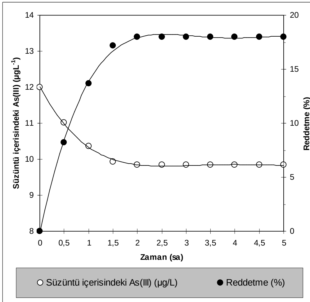
Şekil 9.1. DL Membranı ile gerçek su numunesinde arsenit gideriminin zamana bağlı değişimi (besleme konsantrasyonu Gölbahçe: 12 \pm 2 \mu\text{g/L} , besleme çözeltisi pH'sı Gölbahçe : 7,1; sıcaklık: 25 °C)
