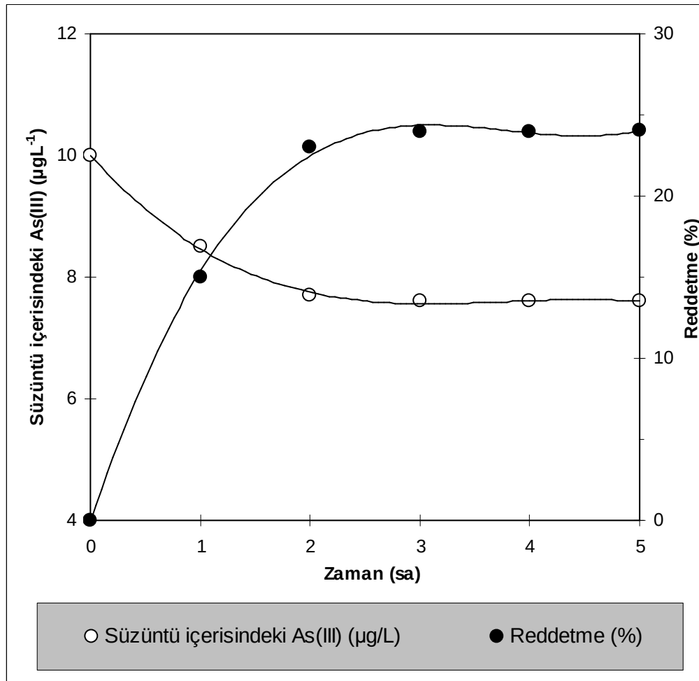
Şekil 9.9. MF-JX / NF 270 Hibrit membran prosesi ile gerçek su numunesinden arsenit gideriminin zamana bağlı değişimi (besleme konsantrasyonu Gülbahçe: 12 \pm 2 µg/L, besleme çözeltisi pH'sı Gülbahçe : 7,1; sıcaklık:25 °C)
