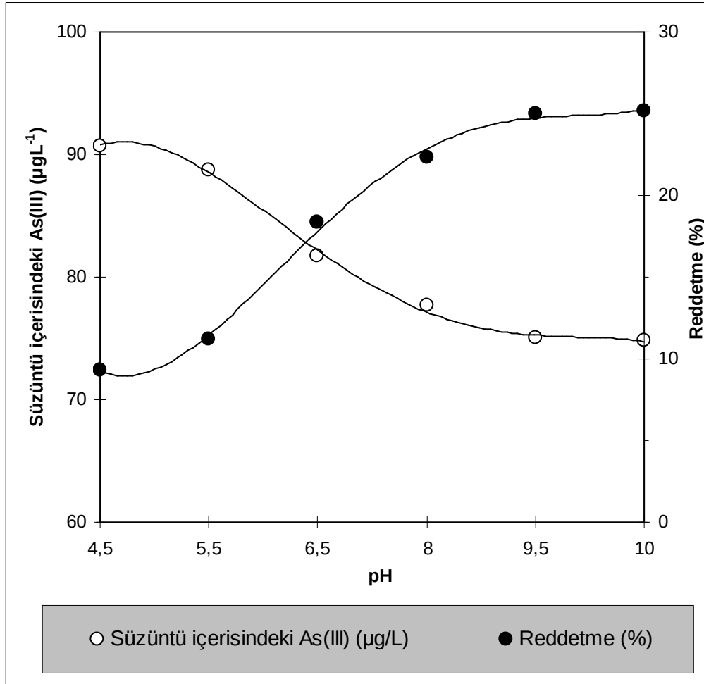
Şekil 8.19. Nanofiltrasyon NF 270 membranı ile arsenit uzaklaştırılması üzerine pH etkisi çalışması (Besleme çözelti konsantrasyonu: 100 ppb, basınç: 20 bar, sıcaklık: 25°C)
