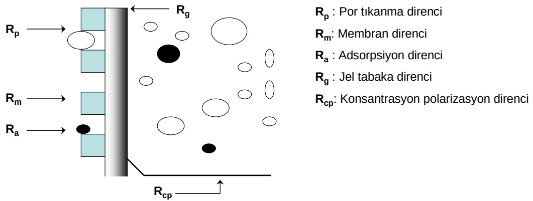
Şekil 5.3. Membran yüzeyinde meydana gelen direnç türleri (Mulder, 1996)
