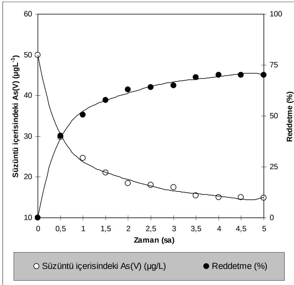
Şekil 9.6. SWHR Membranı ile gerçek su numunesinde arsenat gideriminin zamana bağılı değışimi (besleme konsantrasyonu Gölbahçe: 50 ±2,7 µg/L, besleme çözeltilisi pH'sı Gölbahçe: 7,1; sıcaklık:25 °C)
