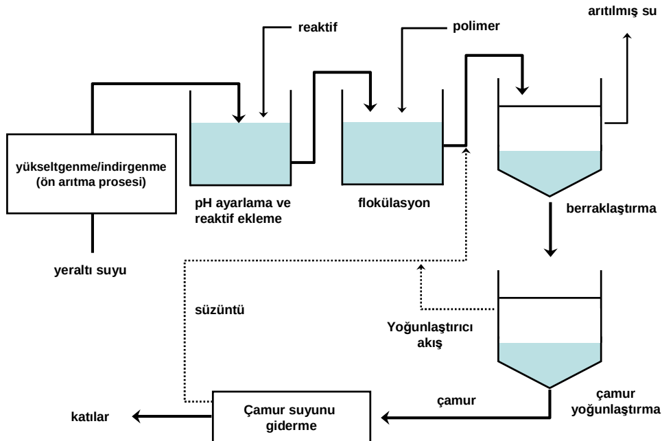
Şekil 2.8. Birlikte çöktürme tekniği ile arsenik arıtımının şematik gösterilişi
