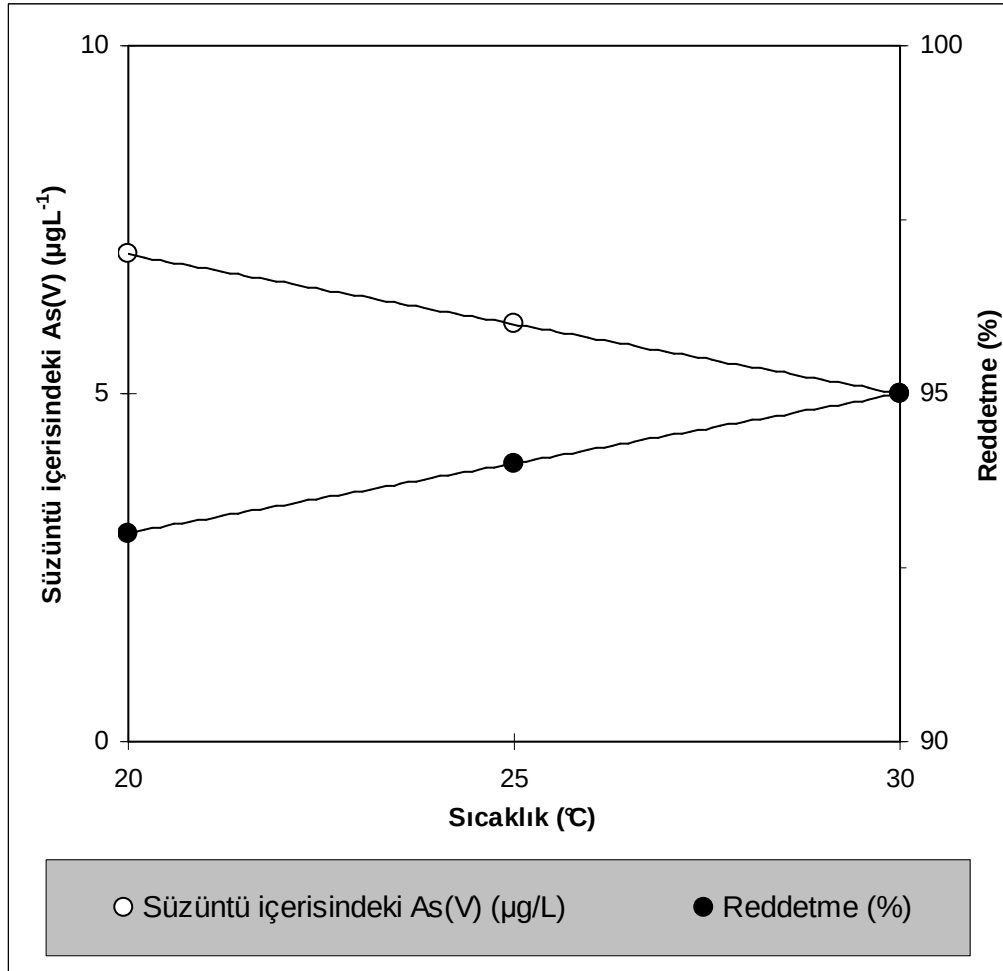
Şekil 8.8. Nanofiltrasyon NF 270 membranı ile arsenat uzaklaştırılması üzerine sıcaklık etkisi çalışması (Besleme çözelti konsantrasyonu: 100 ppb, basınç: 20 bar, pH: 6,75)
