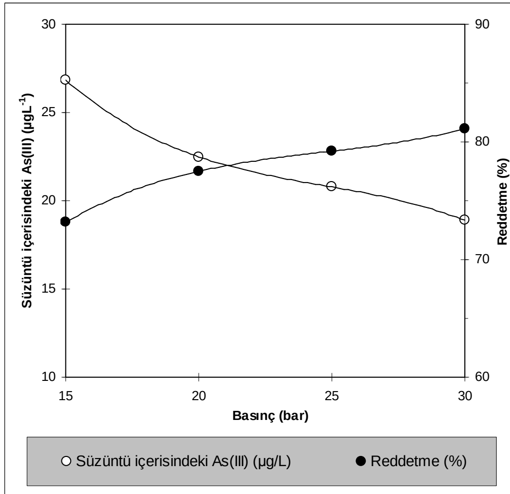
Şekil 8.22. Ters osmoz SWHR membranı ile arsenit uzaklaştırılması üzerine basınç etkisi çalışması (Besleme çözelti konsantrasyonu: 100 ppb, sıcaklık: 25°C, pH: 6,75)
