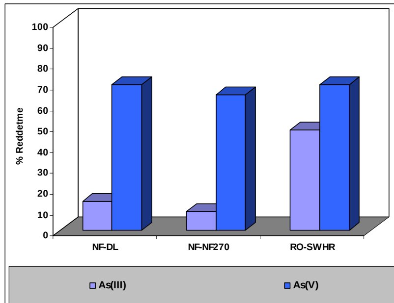
Şekil 10.1. As(III) ve As(V) Gerçek su numune çözeltileri ile yapılan giderim çalışmaları
