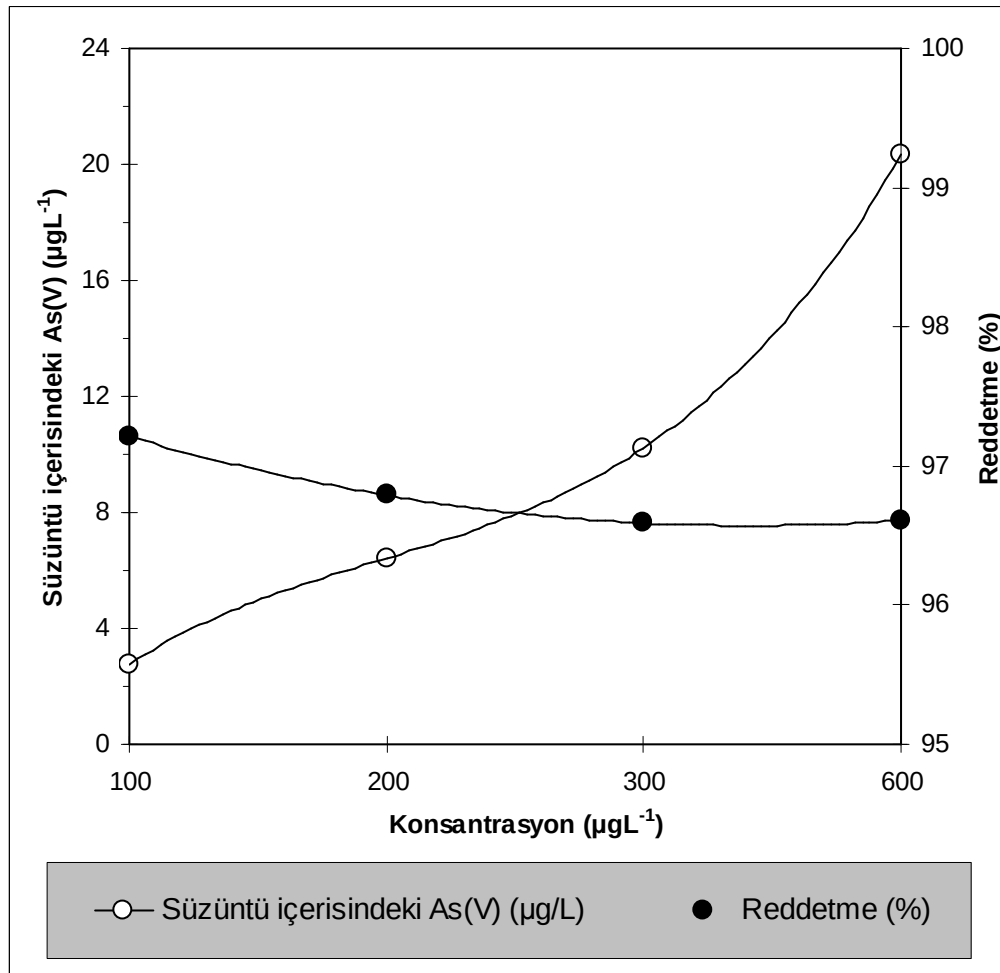
Şekil 8.1. Nanofiltrasyon DL membranı (Osmonics) ile arsenat uzaklaştırılması üzerine konsantrasyon etkisi çalışması( Basınç: 20 bar, sıcaklık: 25°C, pH: 6,75)
