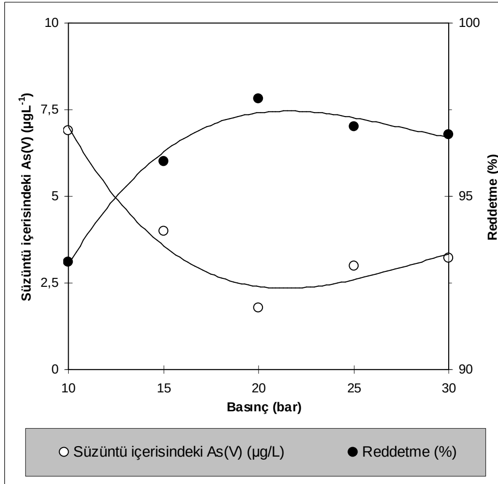
Şekil 8.2. Nanofiltrasyon DL membranı ile arsenat uzaklaştırılması üzerine basınç etkisi çalışması (Besleme çözelti konsantrasyonu: 100 ppb, sıcaklık: 25°C, pH: 6,75)
