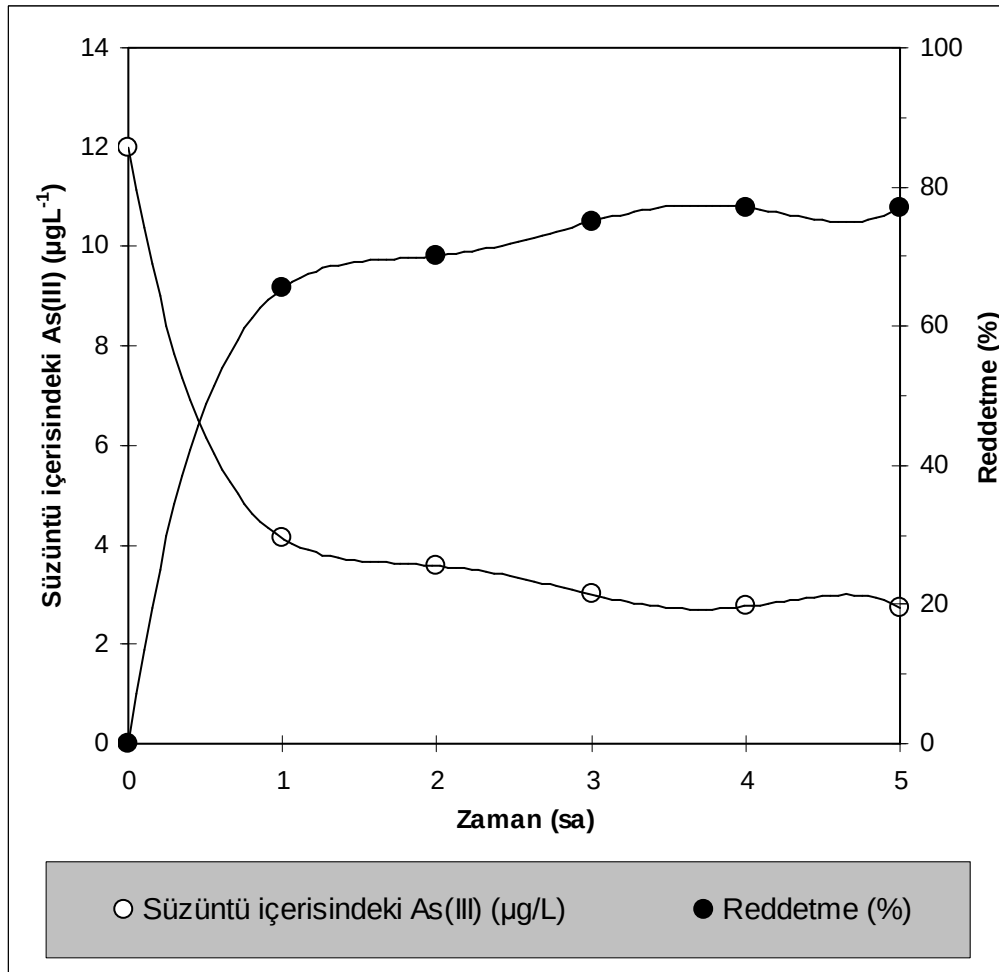
Şekil 9.11. MF-JX / RO-SWHR Hibrit membran prosesi ile gerçek su numunesinden arsenit gideriminin zamana bağlı değişimi (besleme konsantrasyonu Gölpazarı: 12 ±2 µg/L, besleme çözeltisi pH'sı Gölpazarı : 7,1; sıcaklık:25 °C)
