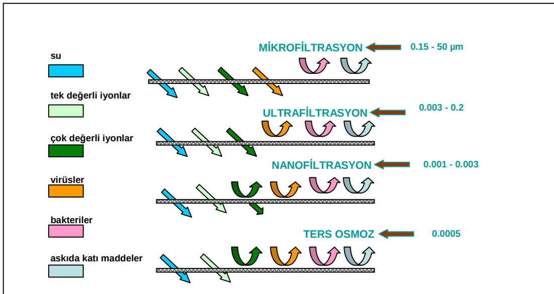
Şekil 4.1. Süzülen madde, gözenek çapı ve membran prosesleri arasındaki ilişki
