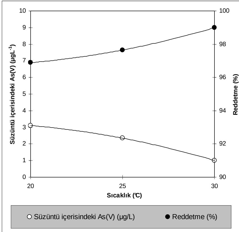
Şekil 8.4. Nanofiltrasyon DL membranı ile arsenat uzaklaştırılması üzerine sıcaklık etkisi çalışması (Besleme çözelti konsantrasyonu: 100 ppb, işletme basıncı: 20 bar, pH: 6,75)
