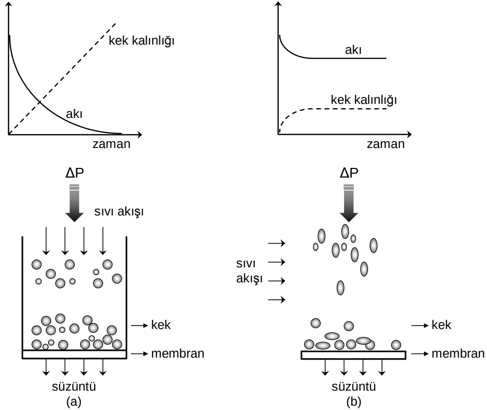
Şekil 5.1. Klasik ve çapraz akış filtrasyonunda akı azalması ve kek kalınlığının zamanla değişimi (a) Klasik filtrasyon (b) Çapraz akış filtrasyonu (Keskinler 1997)
