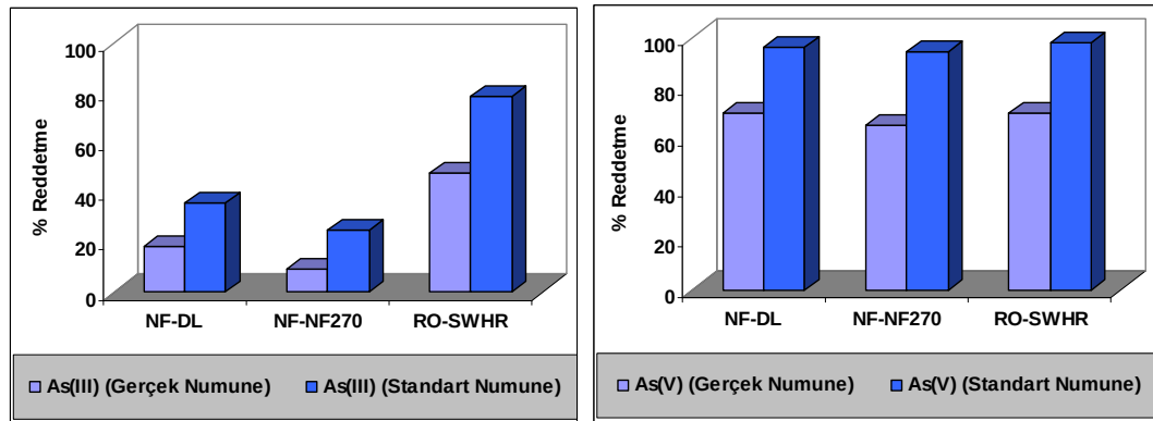
Şekil 10.9 As(III) ve As(V) Standart çözeltilerle yapılan giderim denemeler
