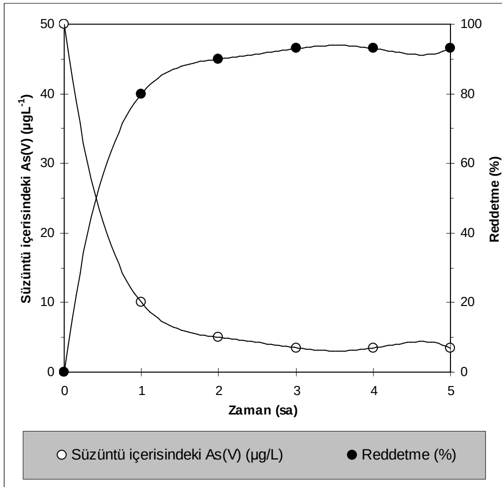
Şekil 9.13. MF-JX / NF-DL Hibrit membran prosesi ile gerçek su numunesinden arsenat gideriminin zamana bağlı değişimi (besleme konsantrasyonu Gölpazarı: 12 \pm 2 µg/L, besleme çözeltisi pH'sı Gölpazarı : 7,1; sıcaklık:25 °C)
