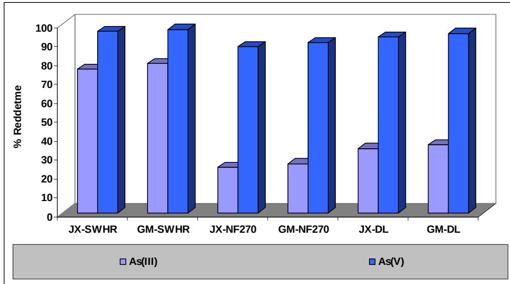
Şekil 10.3. Gerçek su numunelerinde hibrit membranlarla yapılan As(III) ve As(V) giderim çalışmaları
