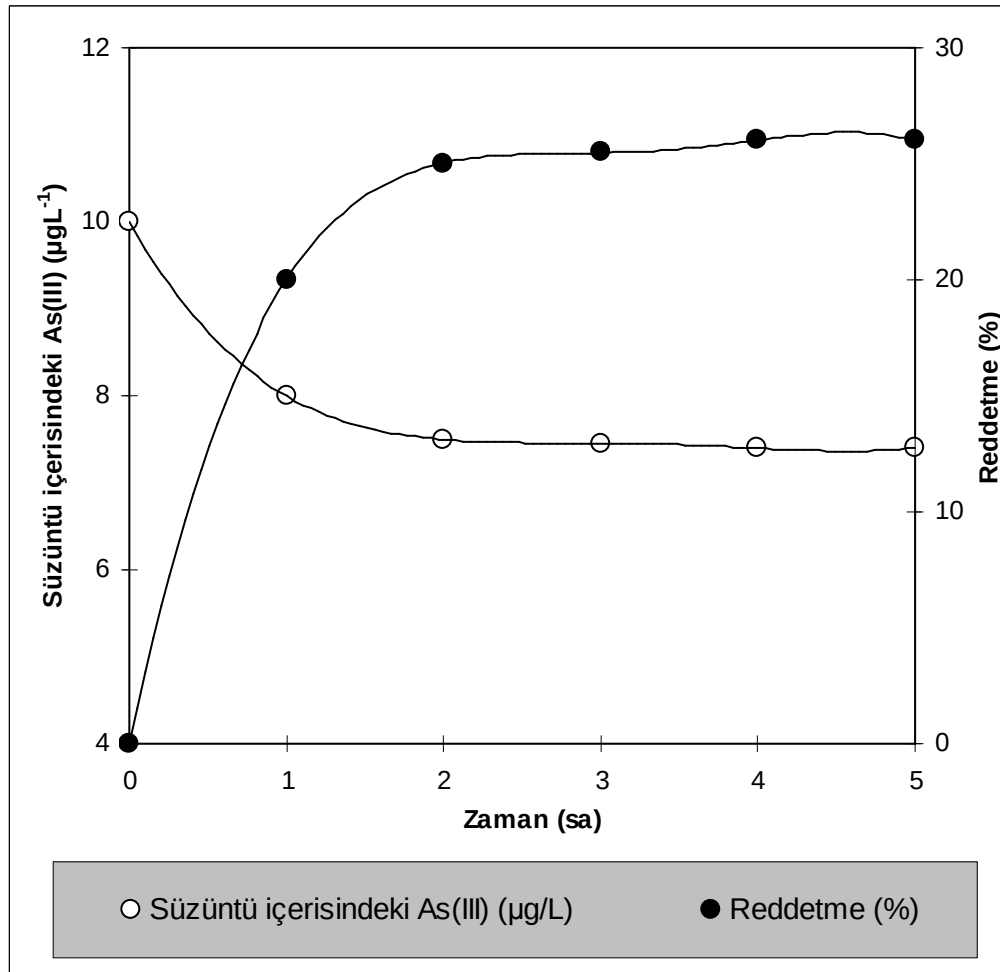
Şekil 9.10. UF-GM/ NF-NF 270 Hibrit membran prosesi ile gerçek su numunesinden arsenit gideriminin zamana bağlı değişimi (besleme konsantrasyonu Gölpazarı: 12 ±2 µg/L, besleme çözeltisi pH'sı Gölpazarı : 7,1; sıcaklık:25 °C)
