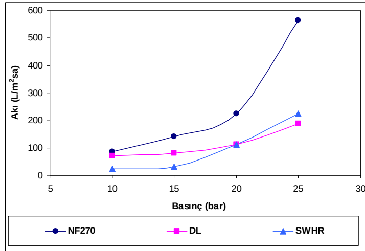
Şekil 10.6.Basınç artışı ile akı arasındaki ilişki
