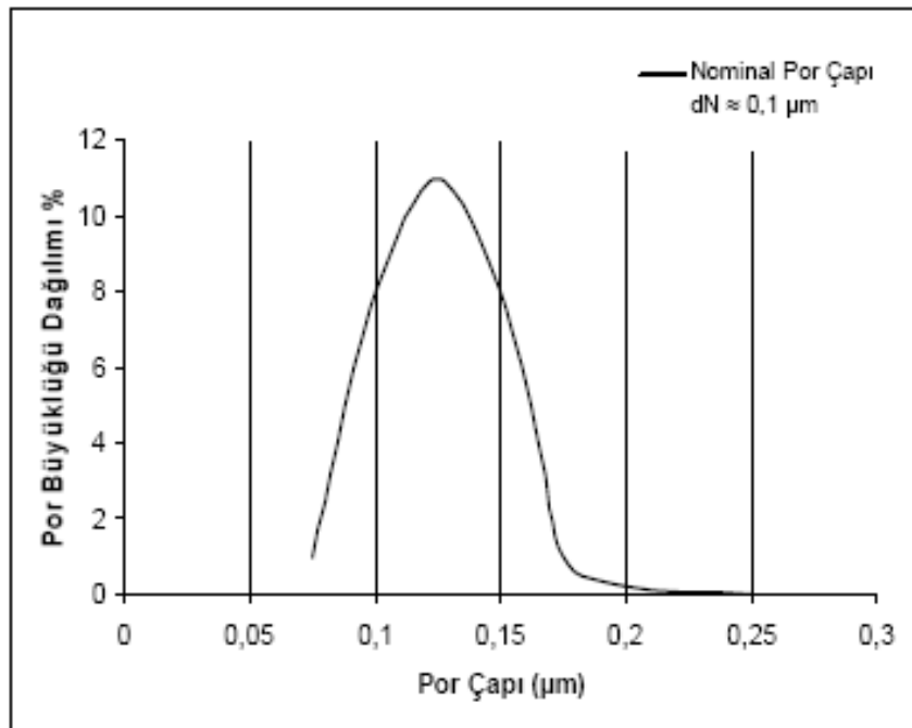
Şekil 4.2. Mikrofiltrasyon membranlarında por büyüklüğü dağılımı
