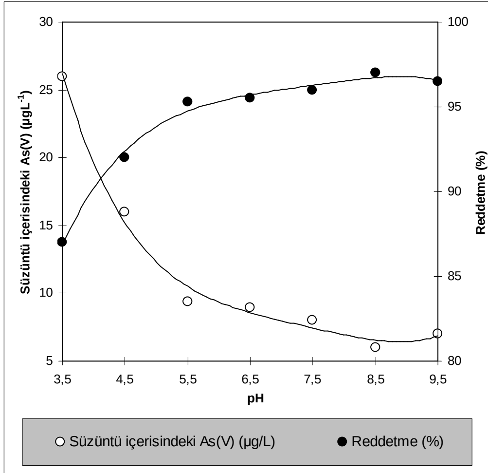
Şekil 8.11. Ters Osmoz SWHR membranı ile arsenat uzaklaştırılması üzerine pH etkisi çalışması (Besleme çözelti konsantrasyonu: 200 ppb, basınç: 20 bar, sıcaklık: 25°C)
