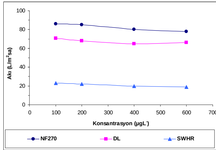
Şekil 10.5. Besleme konsantrasyonunun artışı ile akı arasındaki ilişki
