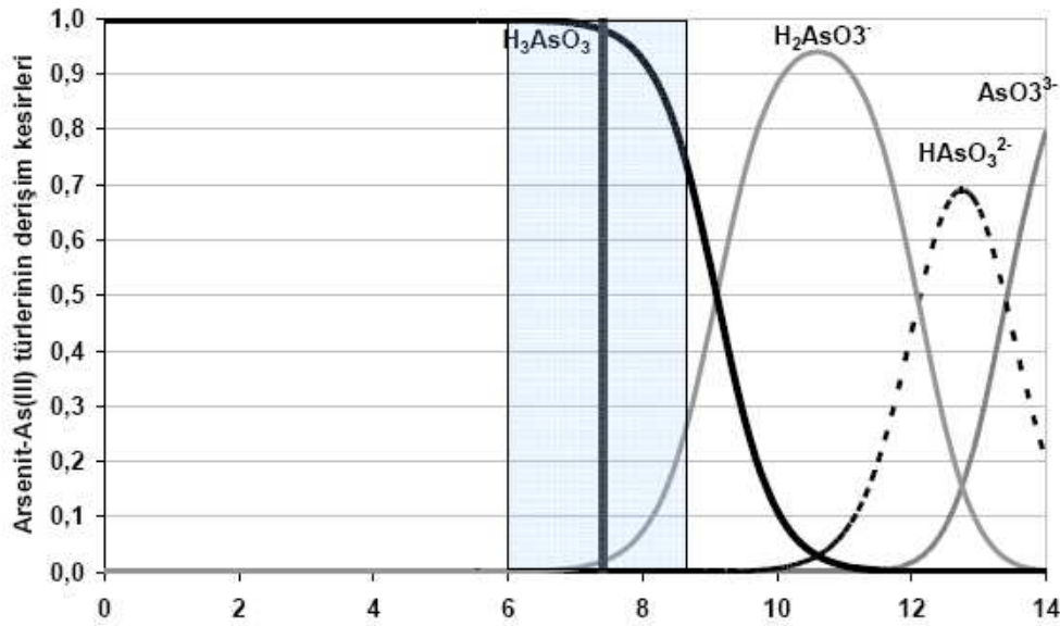
Şekil 2.4. Üç Değerlikli Arsenik Türlerinin pH İle Değişen Bulunma Kesirleri (Demircioğlu, 2009)
