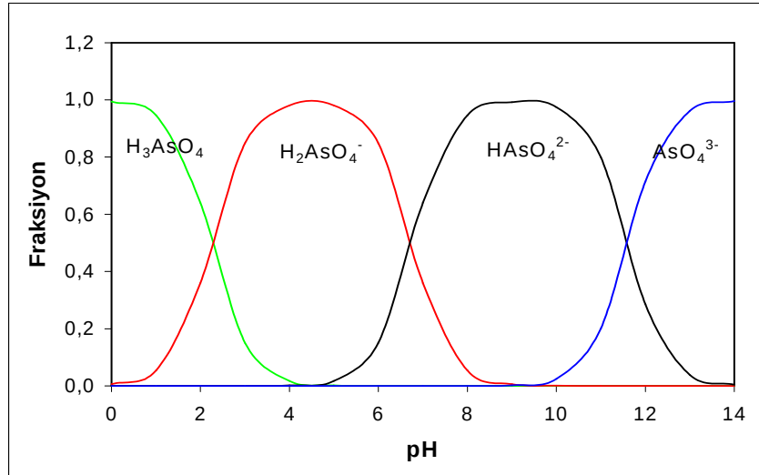
Şekil 10.8 As(V) iyonlarının asit-baz kimyası (Aragon, 2004).
