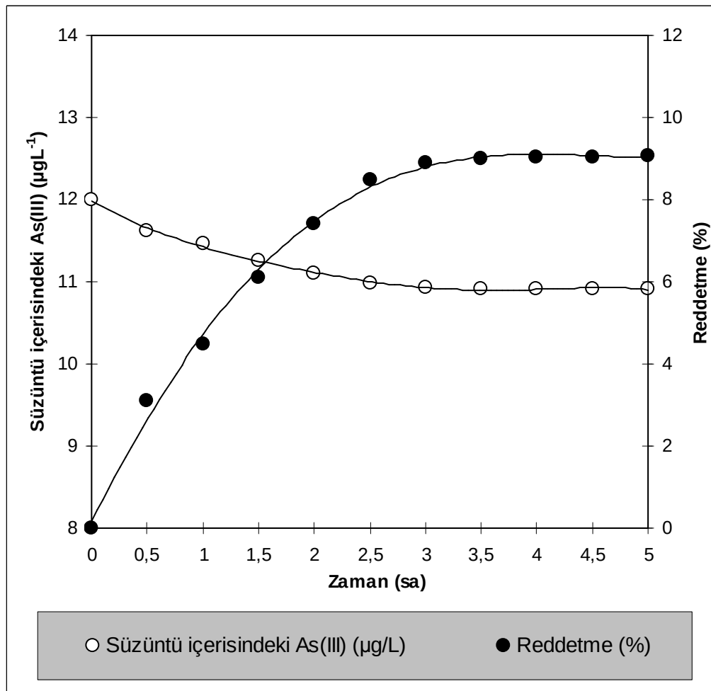
Şekil 9.2. NF 270 Membranı ile gerçek su numunesinde arsenit gideriminin zamana bağlı değişimi (besleme konsantrasyonu Gölpazarı: 12 \pm 2 µg/L, besleme çözeltisi pH'sı Gölpazarı: 7,1; sıcaklık:25 °C)
