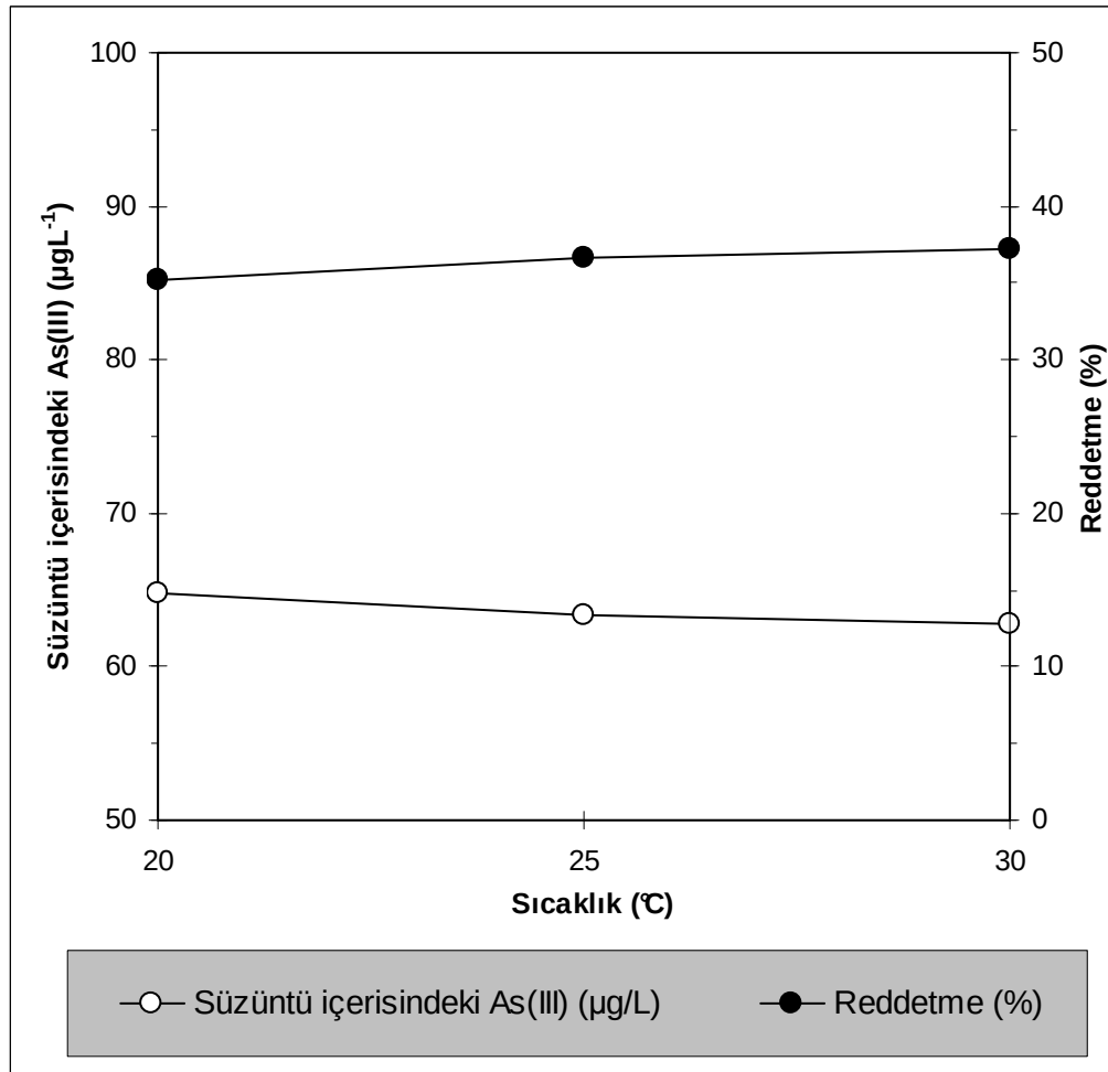
Şekil 8.16. Nanofiltrasyon DL membranı ile arsenit uzaklaştırılması üzerine sıcaklık etkisi çalışması (Besleme çözelti konsantrasyonu: 100 ppb, basınç: 20 bar, pH: 6,75)
