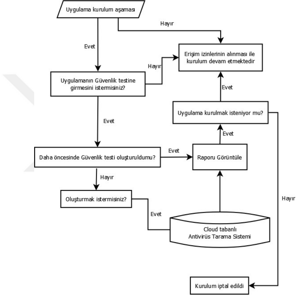
Şekil 30 Güvenilir uygulama kurulum modeli
