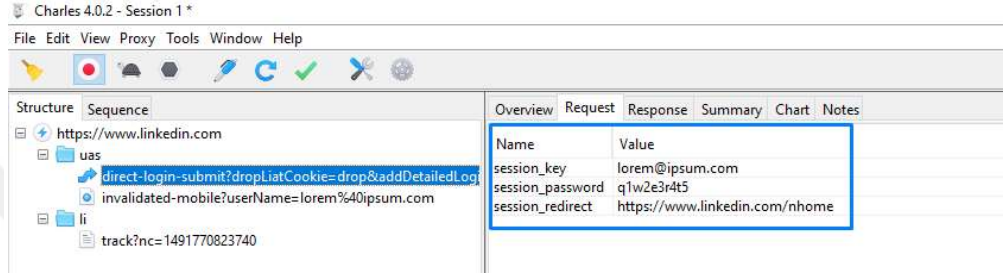
Şekil 23: Charles Proxy: Ağ oturum trafiğini yakalama uygulaması 51
