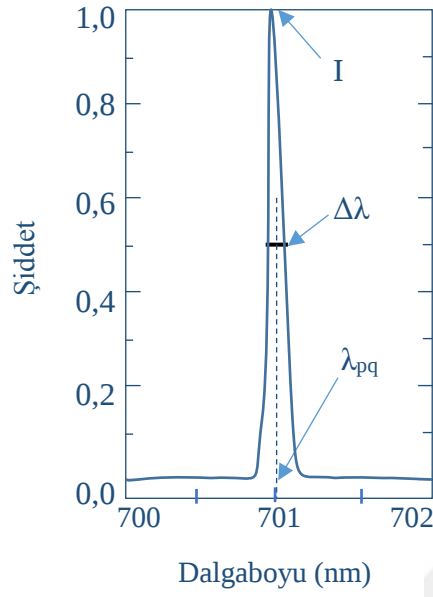
Şekil 3.7. Çizgi ışıma spektrum örneği [78]
