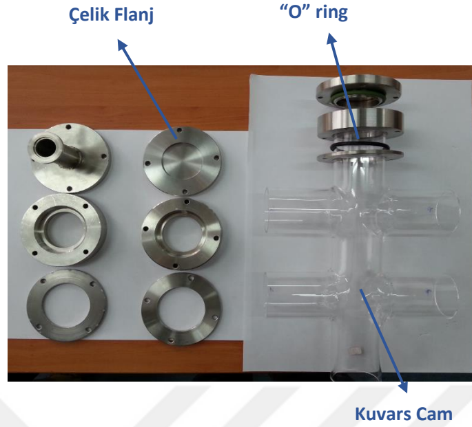
Görsel 4.1. Vakum odasını oluşturmak için kullanılan flanjlardan ve kuvars
