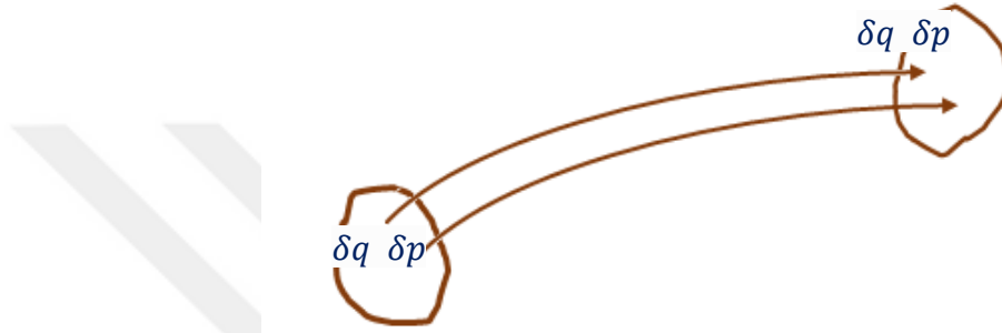
Şekil 2.1. Faz uzayında parçacıkların hareketi
