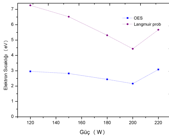
Şekil 4.35. 0,03 lt/dk Ar-0,02 lt/dk H 2 karışım deşarjı için Langmuir prob ve OES ile elde edilen elektron sıcaklıklarının uygulanan güce göre değişimi
