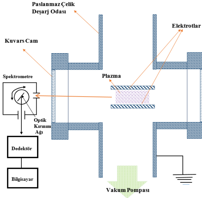
Şekil 3.5. Optiksel büyötmeye sahip plazma spektrumunun kullanıldığı plazma spektroskopisi için deneysel düzenek
