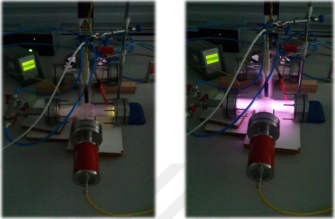
Görsel 4.8. Düşük basınçta kapasitif bağlı radyo frekans sistemi aracılığı ile Ar – O 2 gaz karışımından elde edilen plazmanın deneysel düzeneği
