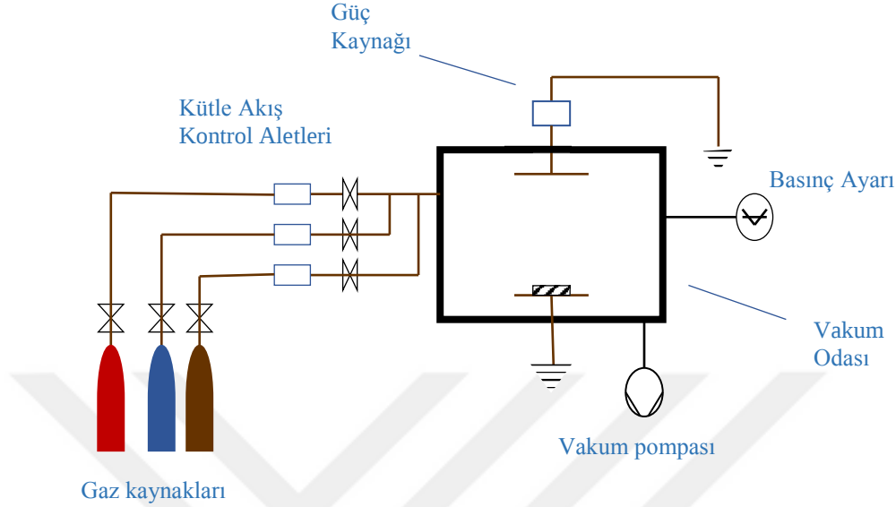
Şekil 1.5. Plazma üretimi için bir sistemin genel şeması
