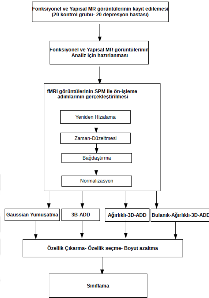
Şekil 3.16. Bu Tez çalışmasında elde edilen fMR görüntülerine uygulanan işlem adımları
