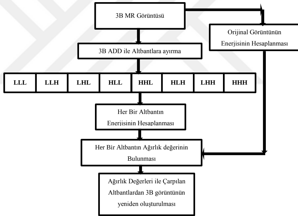
Şekil 2.14. Tez çalışmasında geliştirilen Ağırlıklı 3B-ADD yöntemine ait akış diyagramı
