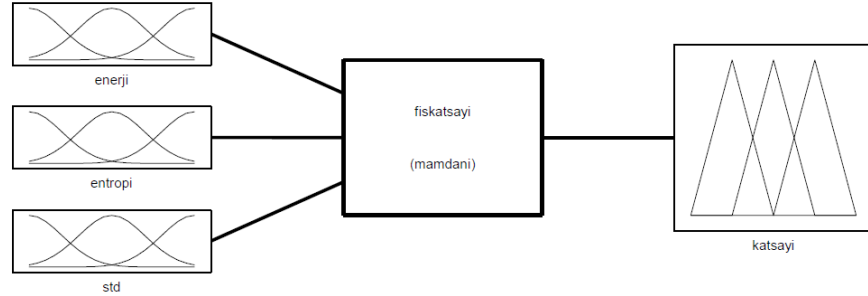
Şekil 3.4. Bulanık Çıkarım Sistemi
