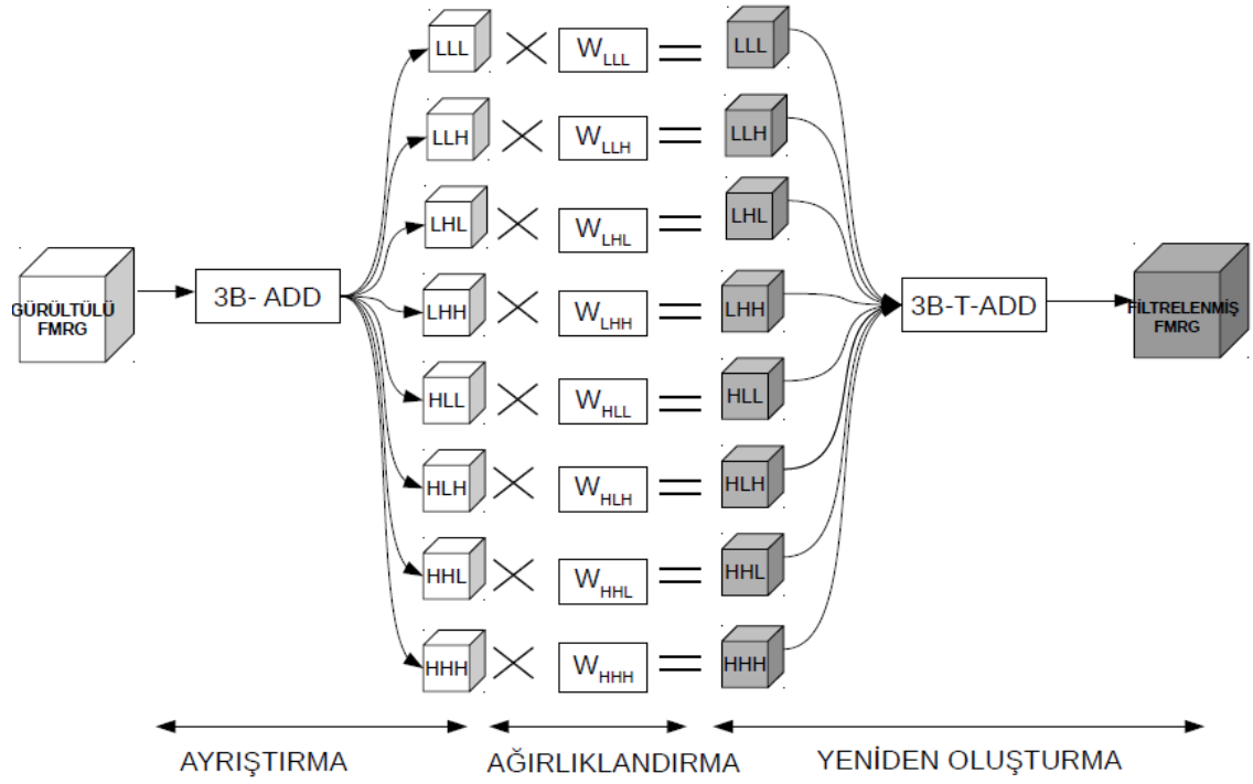
Şekil 2.18. Filtrelenmiş volümün ağırlıklandırılmış altbantlardan elde edilmesi
