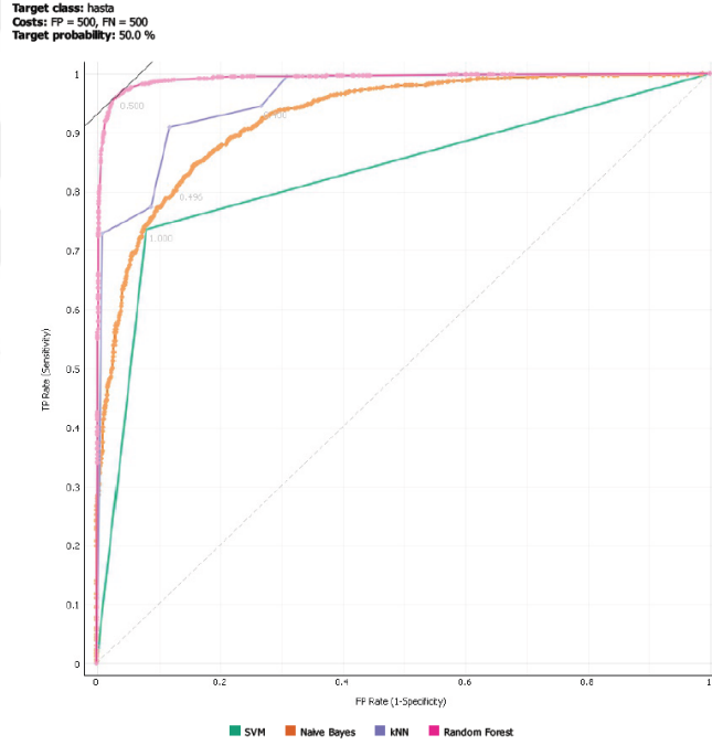
Şekil 3.26. Ağırlıklı-3B-ADD + kesit bazlı yöntem+ TBA kullanılması ile yapılan sınıflama sonuçlarına ait ROC eğrileri
