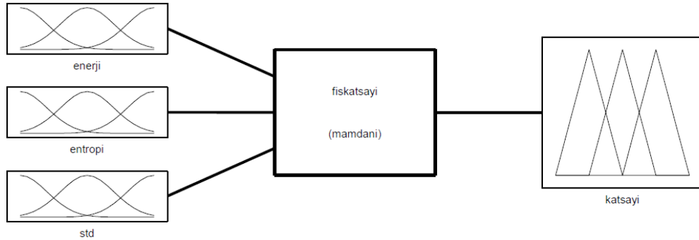
Şekil 2.21. Bulanık Çıkarım Sistemi
