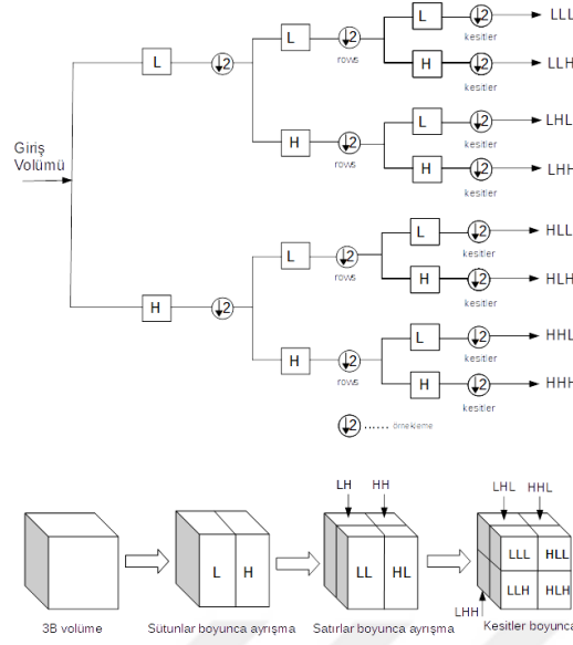
Şekil 2.16. 3B-ADD ile alt-bantların elde edilmesi (Procházka ve ark., 2011)
