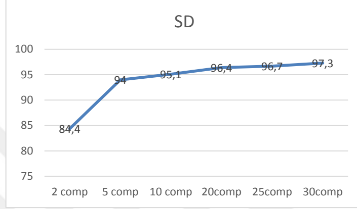
Şekil 3.29. Ağırlıklı-3B ADD ile kullanılan kesit bazlı yöntemde temel bileşen sayıları 2,5,10,20,25,30 için RO değerlendirme sonuçları
