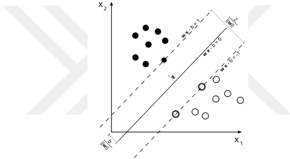
Şekil 2.30. Doğrusal DVM modelini ifade eden grafik (Chen ve ark., 2005)
