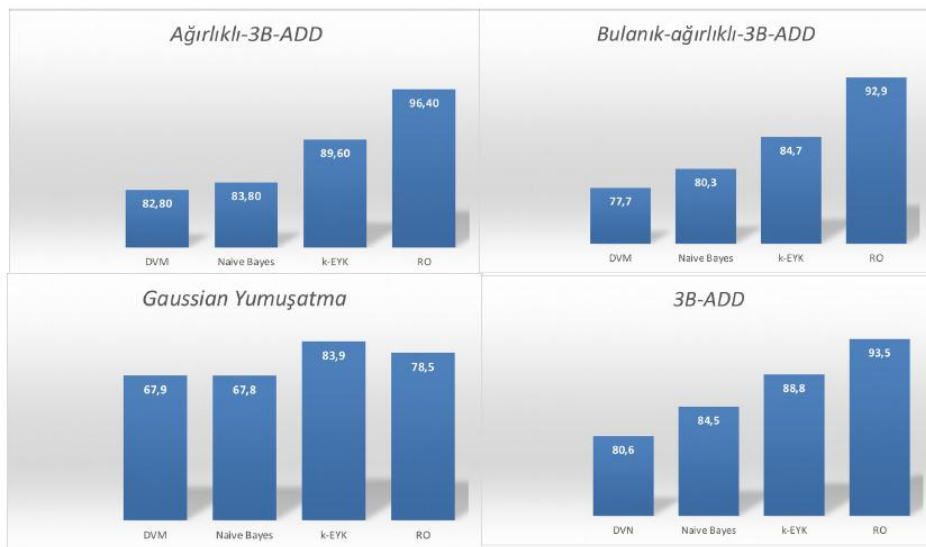
Şekil 3.28. Kesit bazlı elde edilen özelliklere TBA uygulanması sonucu elde edilen sınıflama doğruluğu için grafiksel sonuçlar
