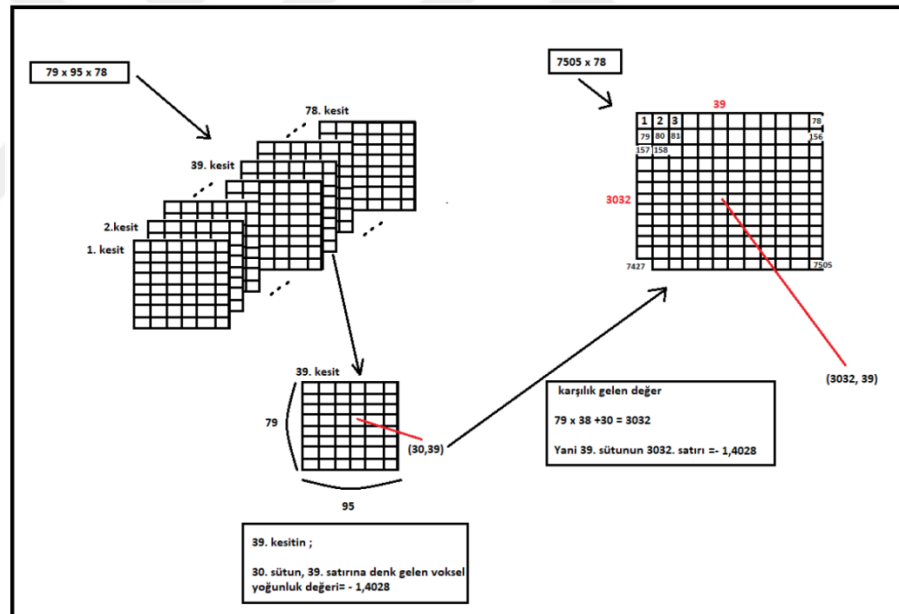
Şekil 2.29. Tez çalışmasında önerilen kesit bazlı özellik seçme yöntemi
