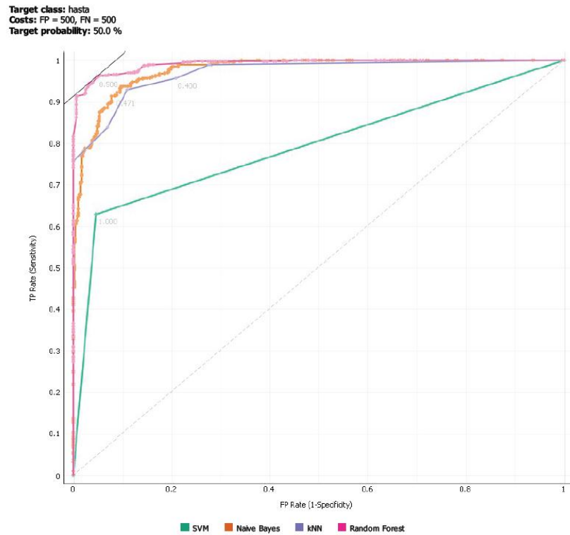
Şekil 3.30. % 30 luk test verisi kullanıldığında RO ile sınıflama doğruluğunun ROC eğrileri ile değerlendirilmesi
