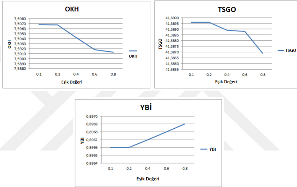
Şekil 3.11. Çizelge 3.12' ye ait değerlendirme parametrelerinin değişiminin izlenmesi
