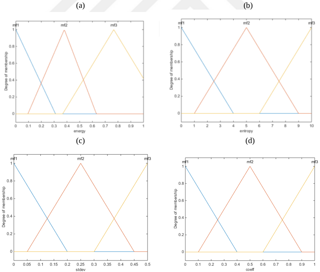
Şekil 2.22. (a) Enerji değeri kullanılarak hesaplanan ağırlık katsayısı için (b) entropi değeri için (c) standart sapma için (d) girdi değerleri ile belirlenen ağırlık değeri için oluşan üyelik fonksiyonları
